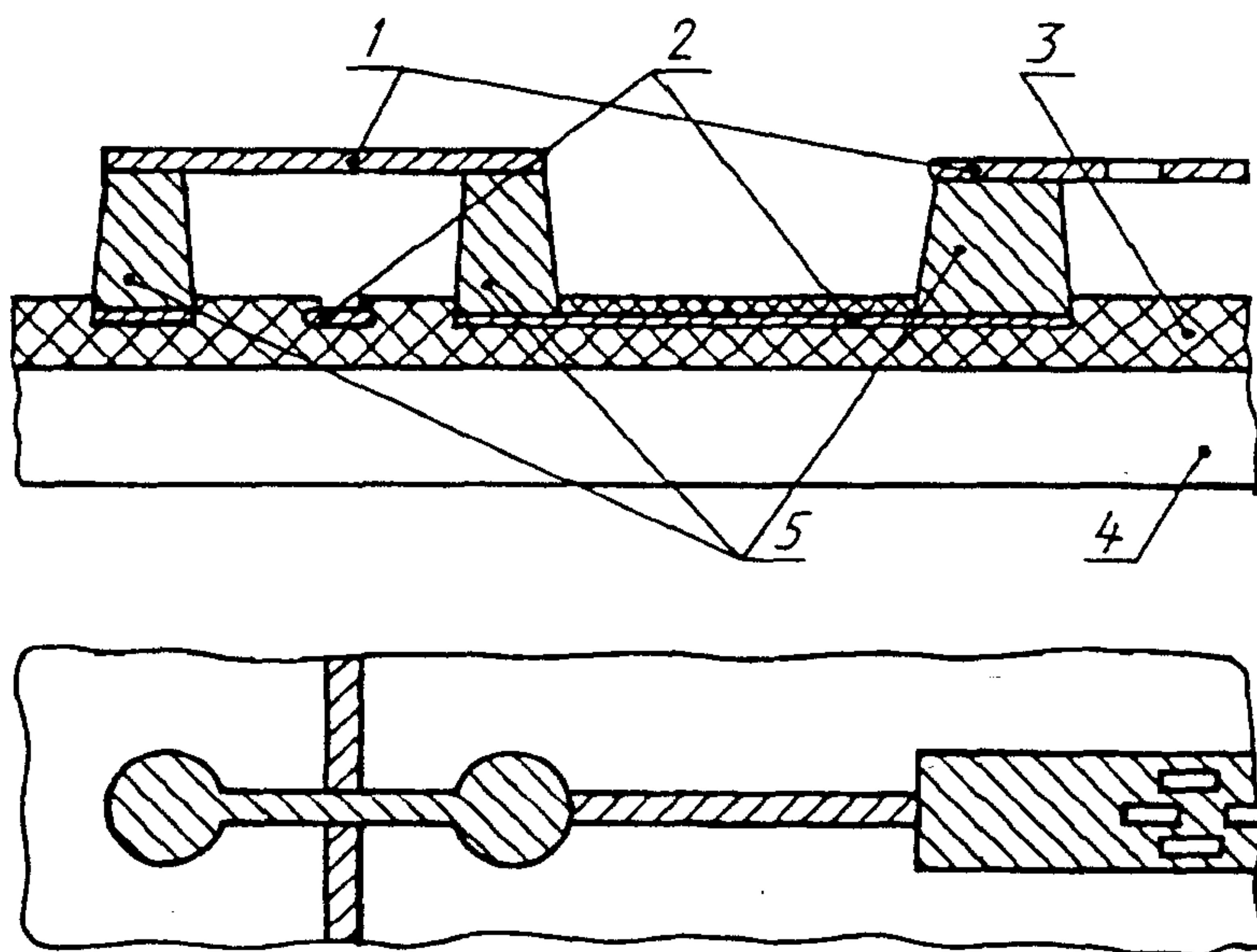
1 — проводящий рисунок, верхний уровень; 2 — проводящий рисунок, нижний уровень; 3 — склеивающая прокладка; 4 — основание МУПП; 5 — опора проводящего рисунка верхнего уровня. Опора может выполнять функции электрического соединения верхнего и нижнего уровней проводящего рисунка
