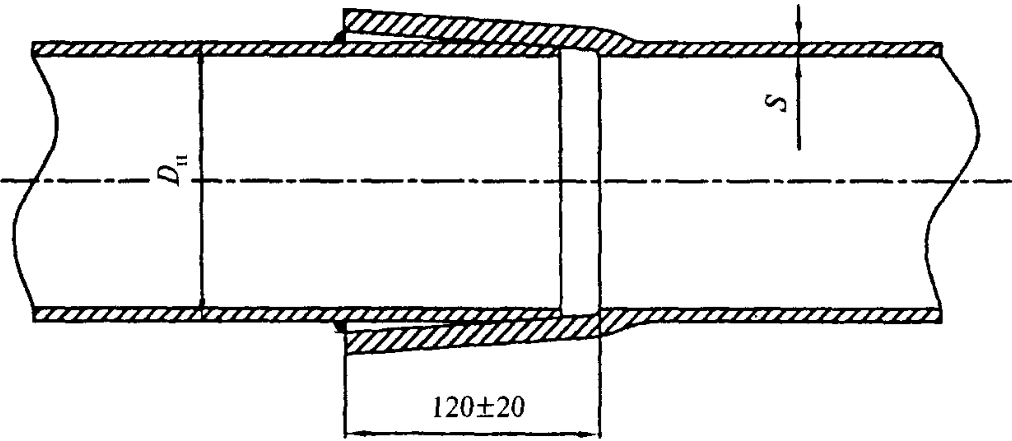
Рисунок А.5 — Схема сварного нахлестного соединения
