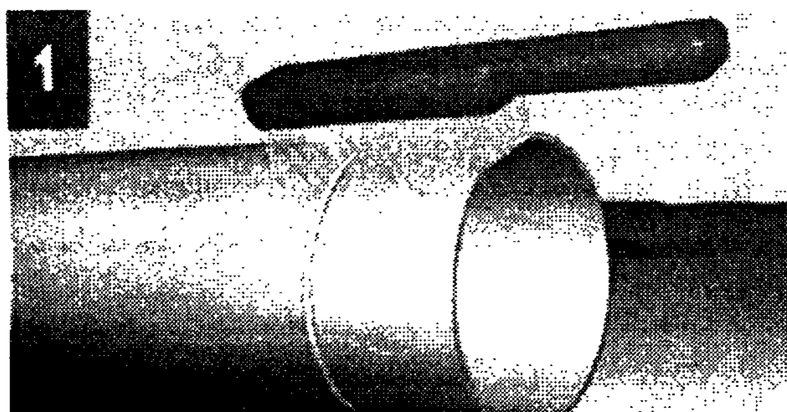
Очистка гладкого конца
