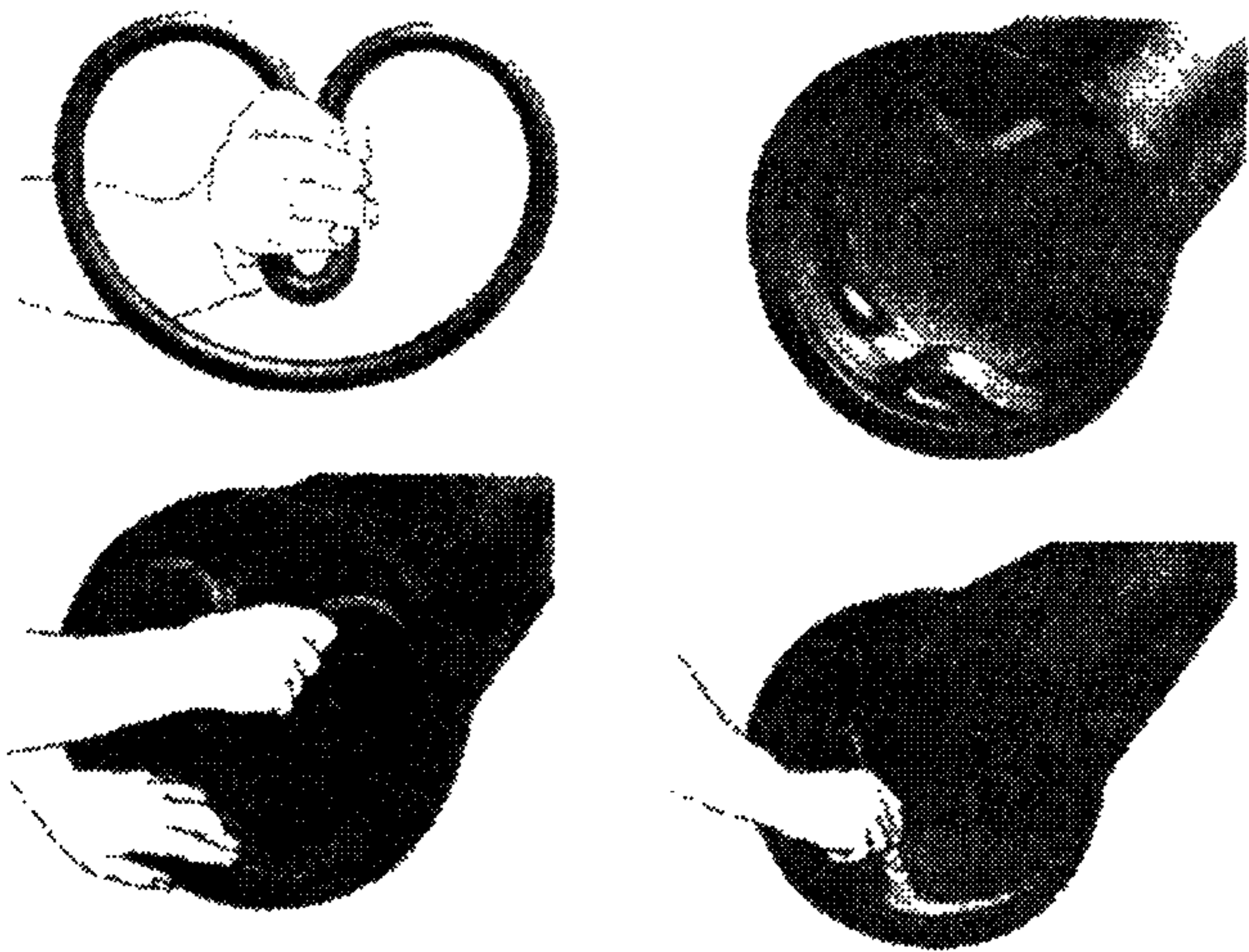
Рисунок 5.3. — Схема укладки уплотнительного резинового кольца
