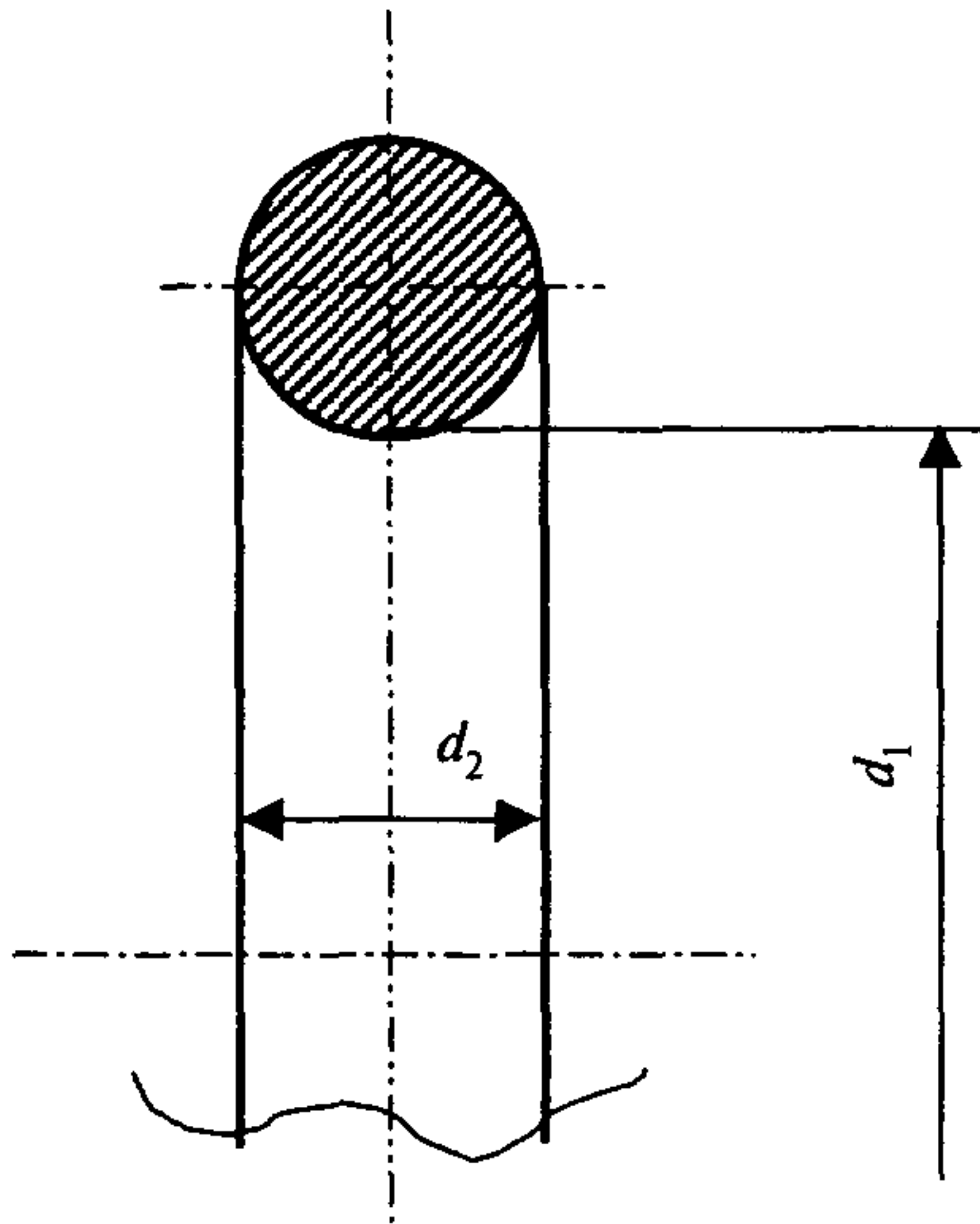
Рисунок А.17 — Уплотнительное резиновое кольцо для муфтового соединения (тип 2)
