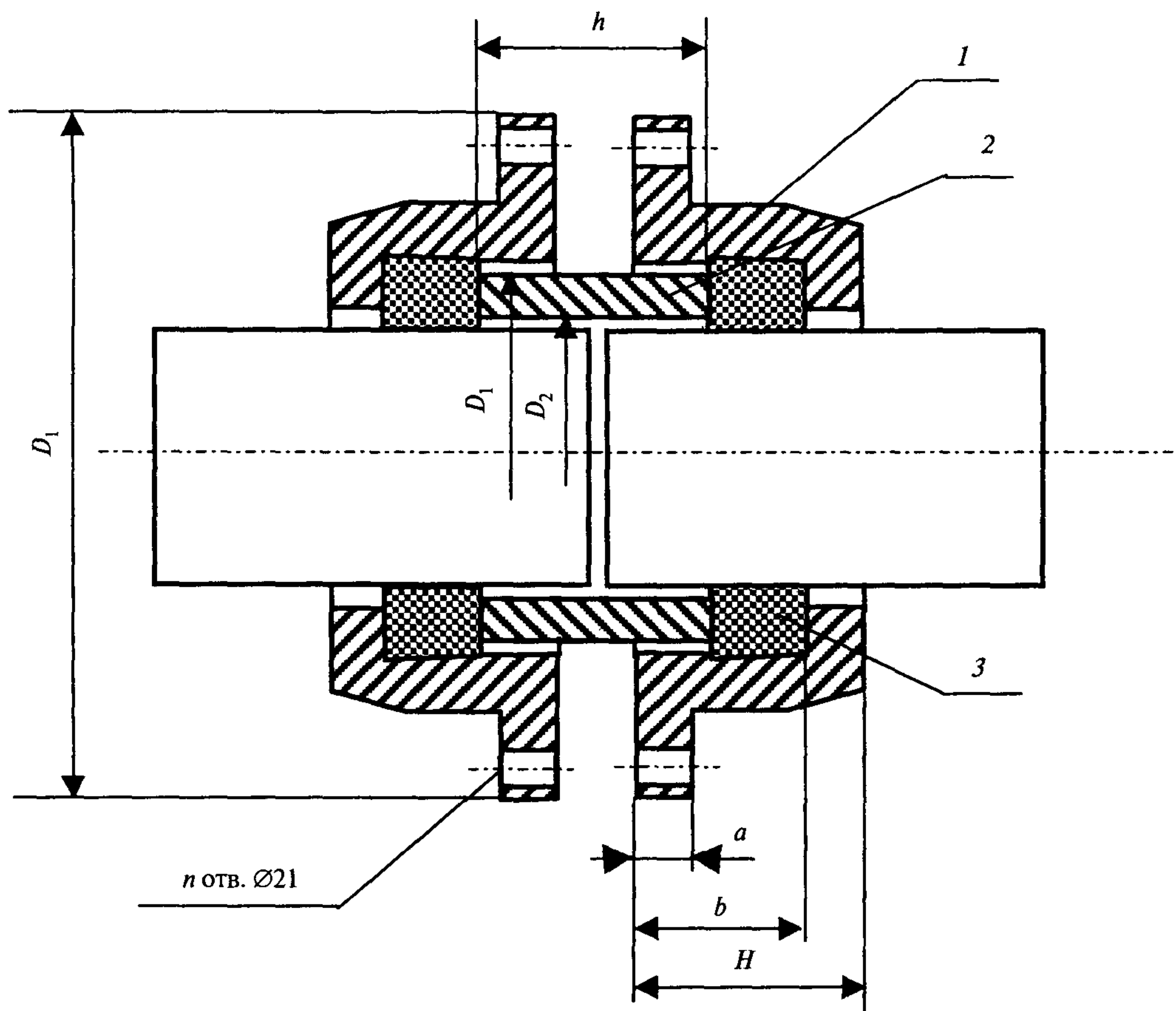
1 — муфта; 2 — втулка; 3 — резиновое кольцо
