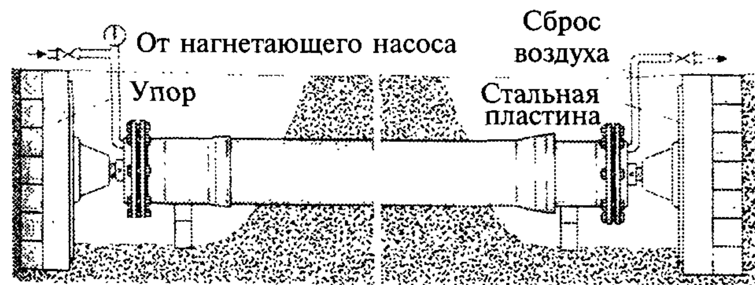
Рисунок 5.11 — Подготовка трубопровода к гидроиспытанию
