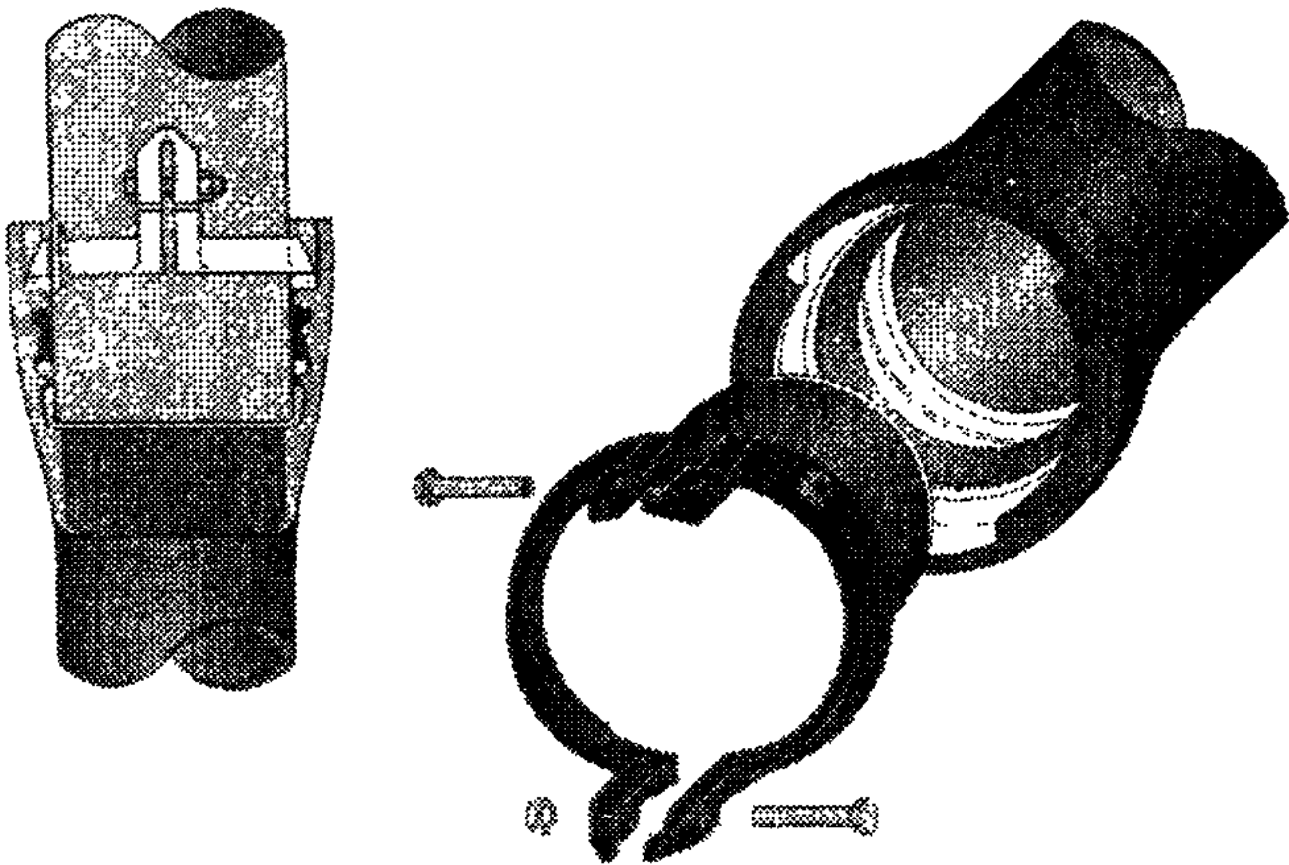
Рисунок 5.4 — Специальное приспособление, заменяющее наплавленный валик
