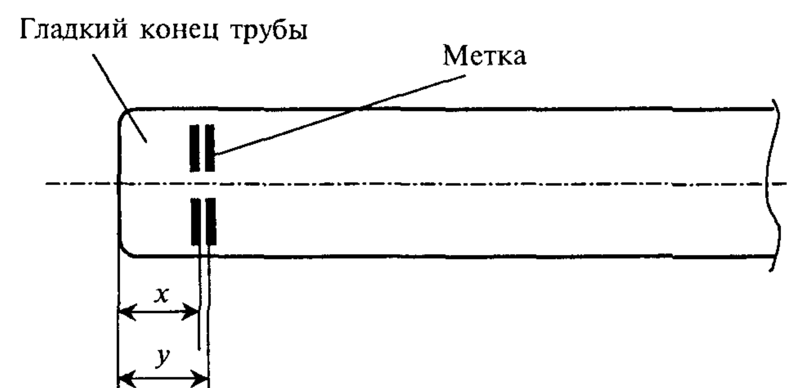
Рисунок 5.2 — Метка на гладком конце трубы
