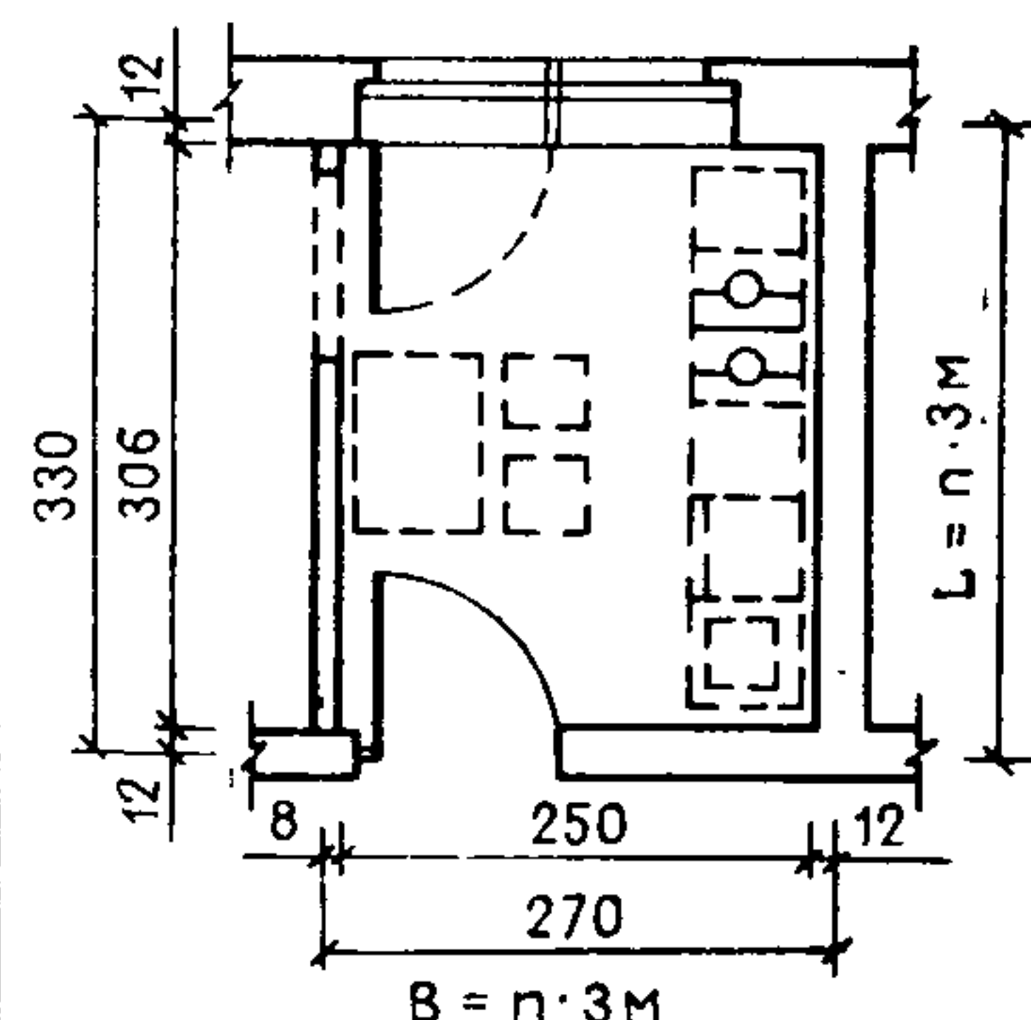
СХЕМА ПЛАНИРОВКИ КУХНИ С ПРИВЯЗКОЙ МОДУЛЬНЫХ ОСЕЙ
