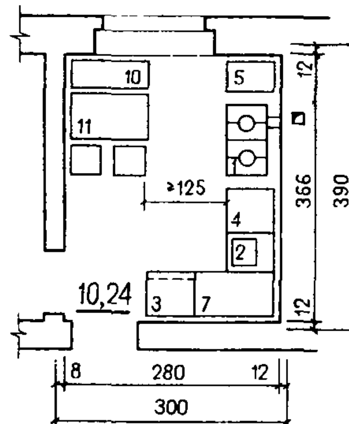
3 УГЛОВОЕ ОБОРУДОВАНИЕ
