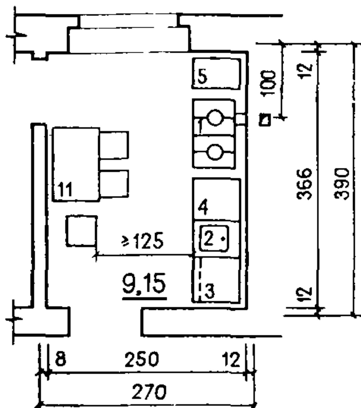
4 П-ОБРАЗНОЕ ОБОРУДОВАНИЕ
