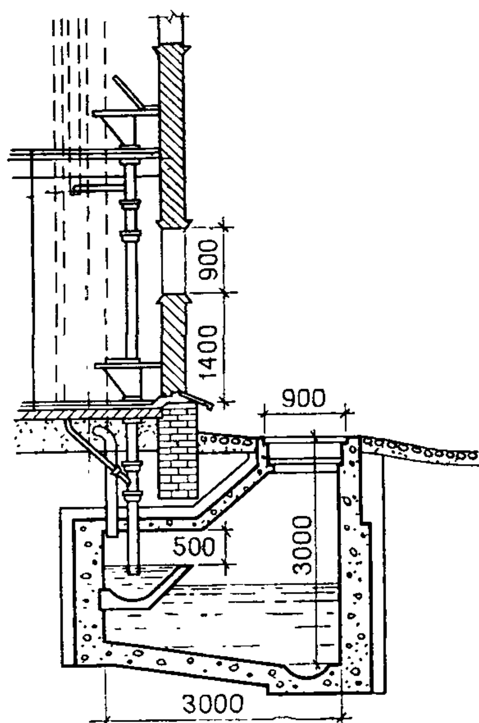
СХЕМА ЛЮФТ-КЛОЗЕТА С ГИДРАВЛИЧЕСКИМ ЗАТВОРОМ В 2-ЭТАЖНОМ ДОМЕ
