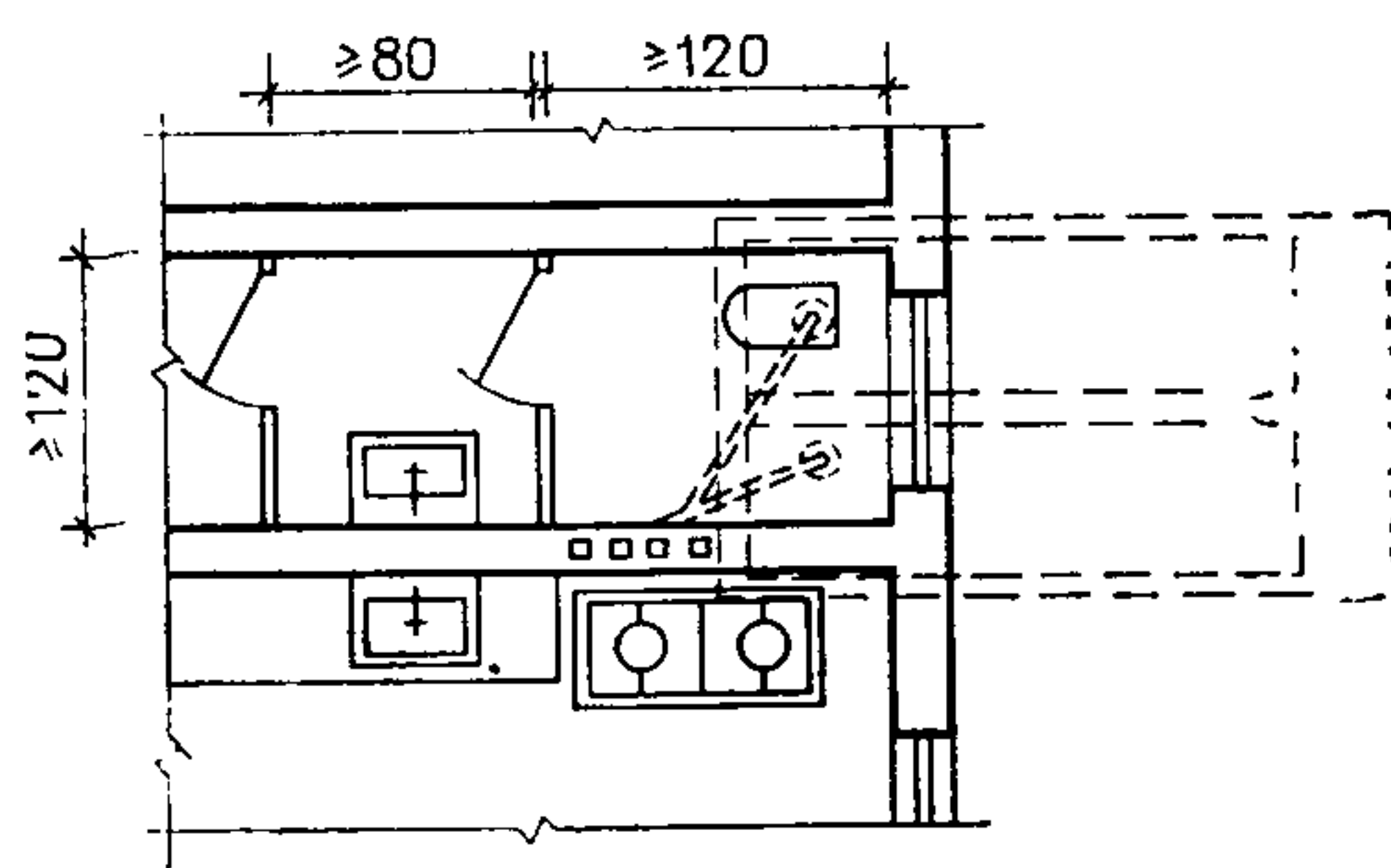
ПЛАН I ЭТАЖА
