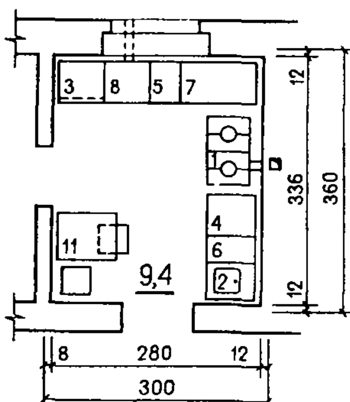
4 П-ОБРАЗНОЕ ОБОРУДОВАНИЕ
