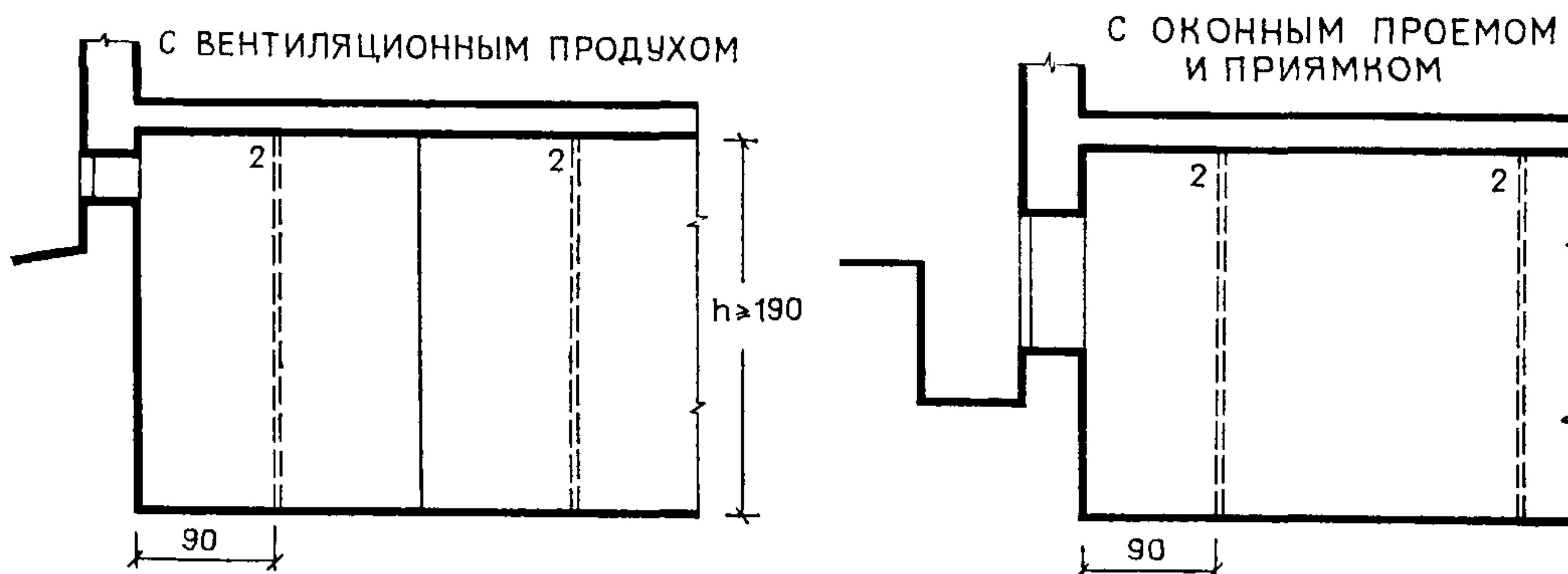
СХЕМЫ РАЗРЕЗОВ ПО ПОДВАЛЬНОМУ ЭТАЖУ
