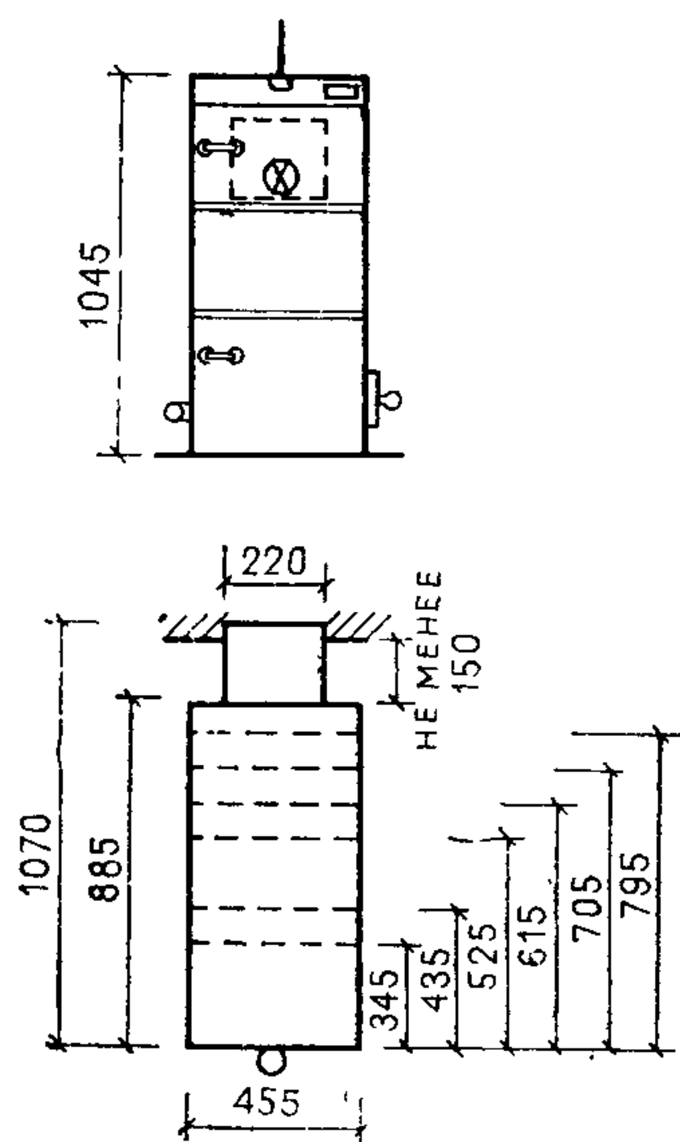
КОТЕЛ-ПЛИТА
