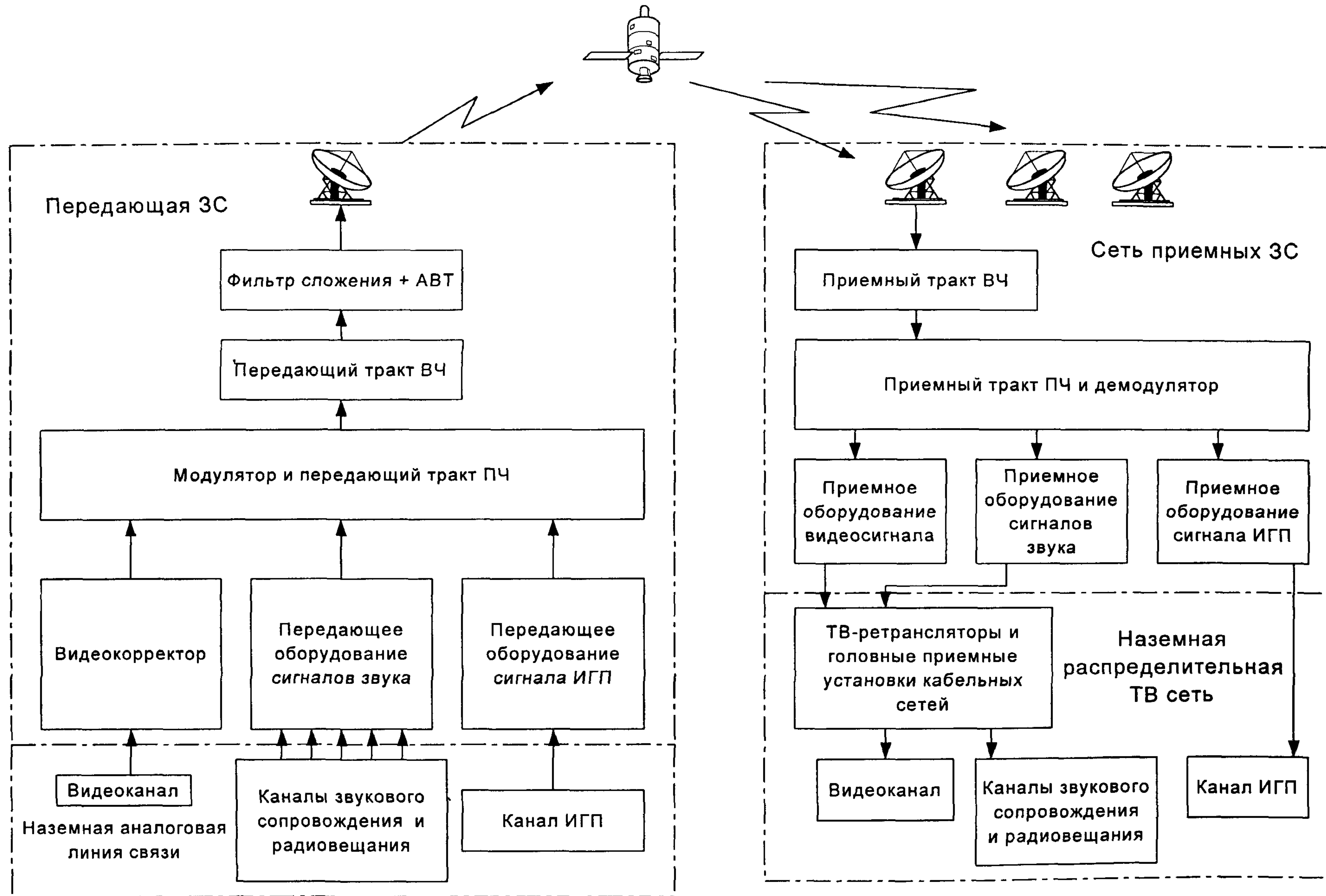
Рис.6.1 Схема передачи аналогового ТВ через спутник
