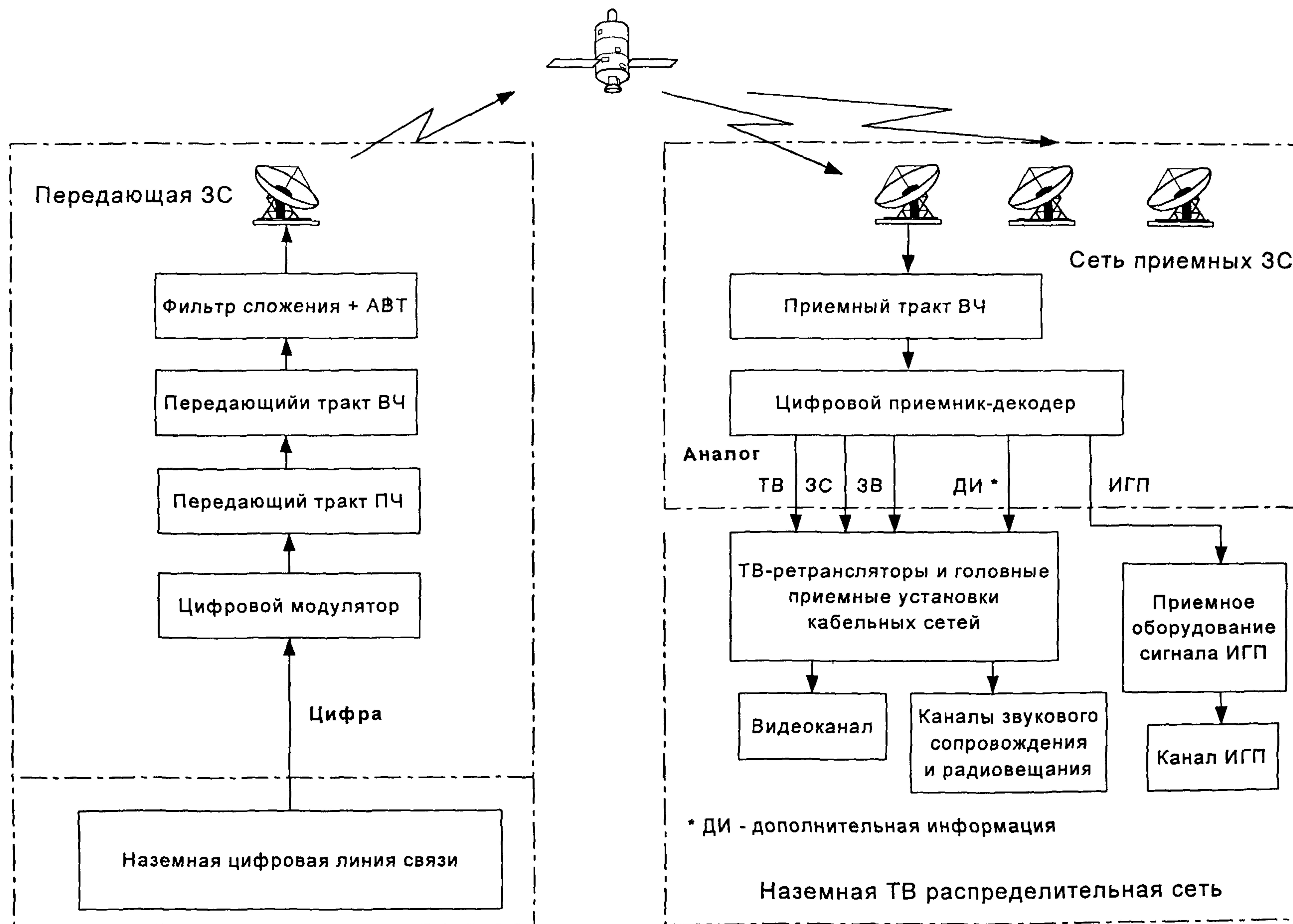
Рис.6.2 Схема передачи цифрового ТВ через спутник
