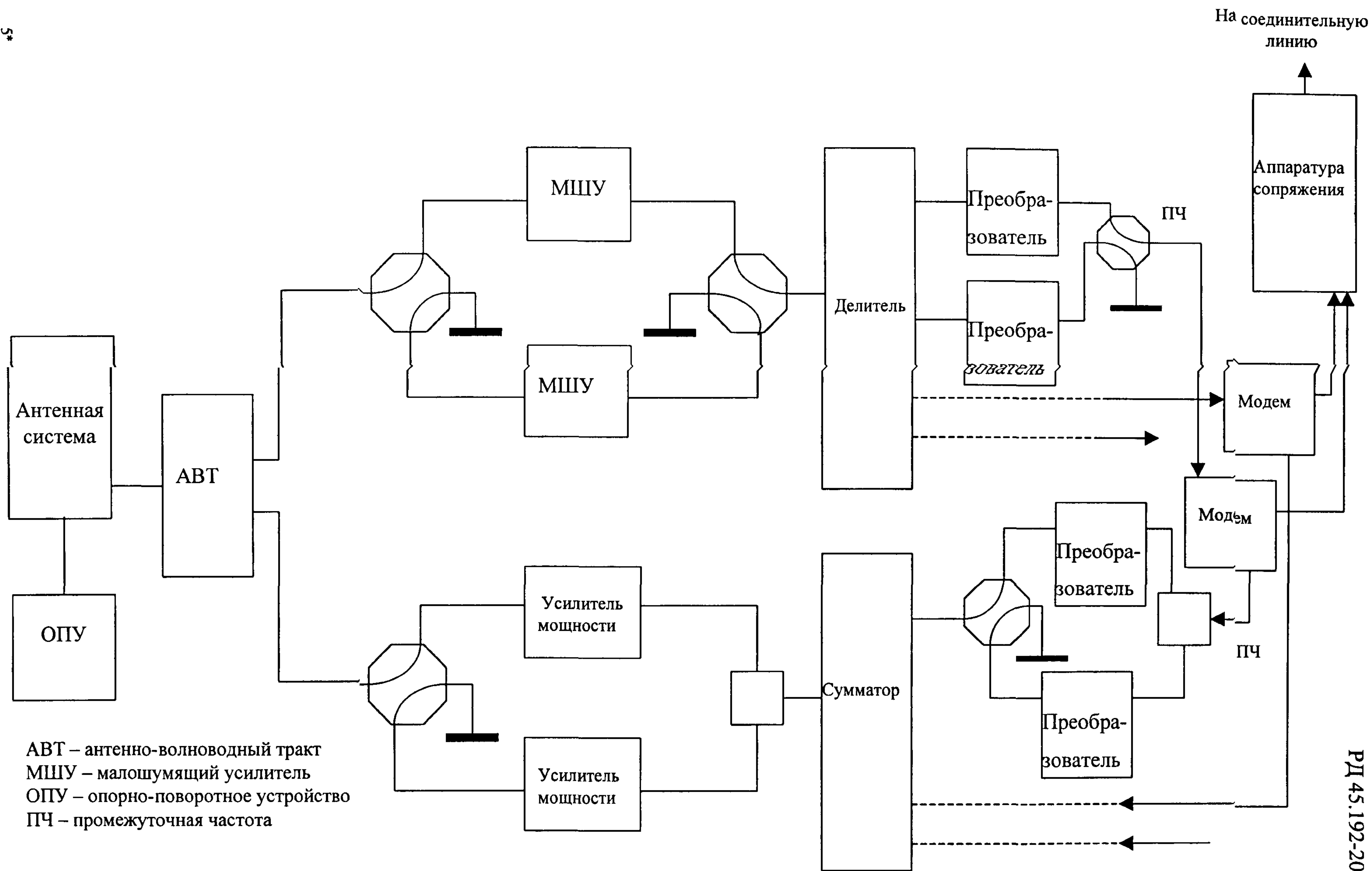
Рис. 3.2 Структурная схема земной станции
