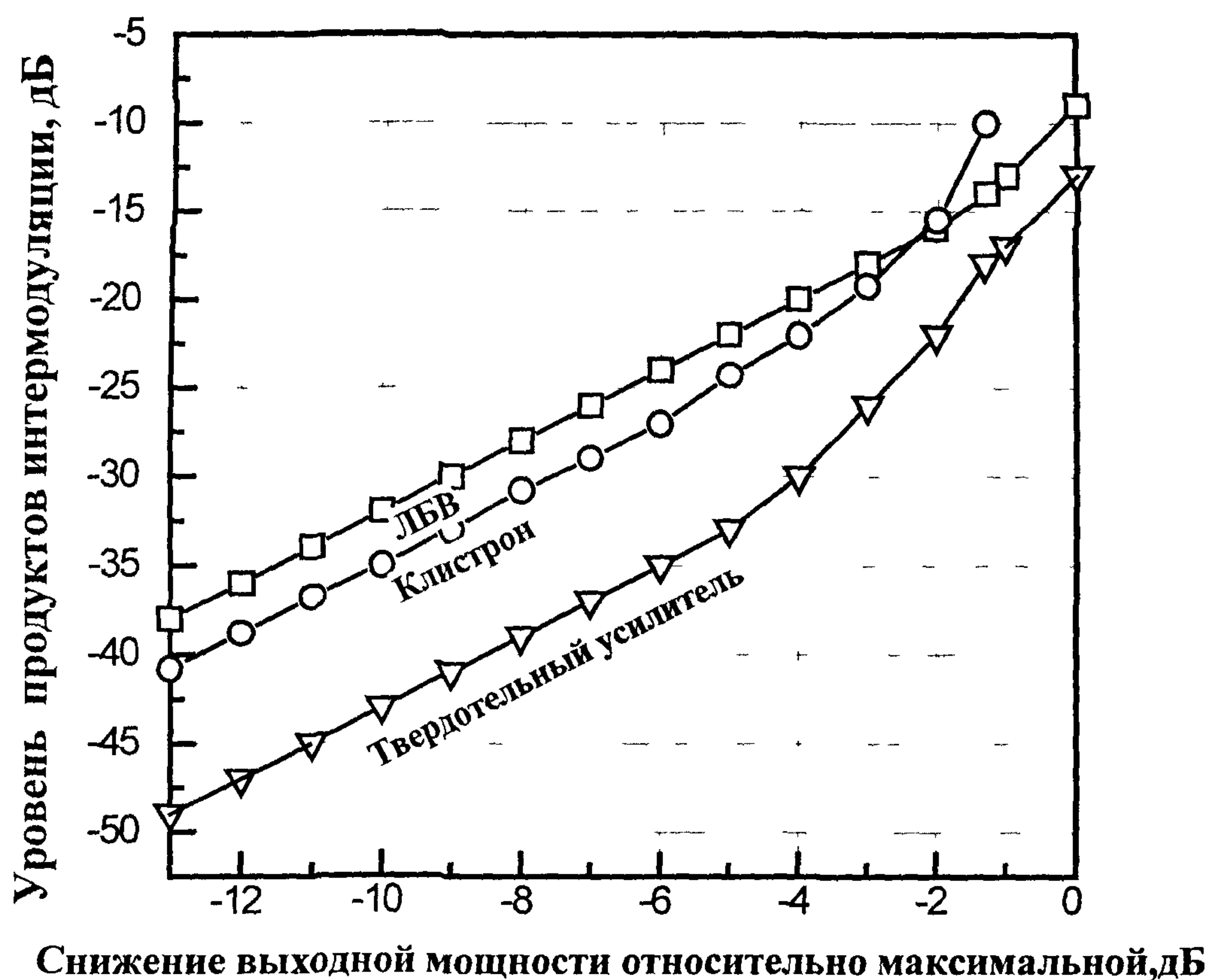
Рис. Ж.1 Зависимость продуктов интермодуляции от снижения мощности усилителя относительно максимальной
