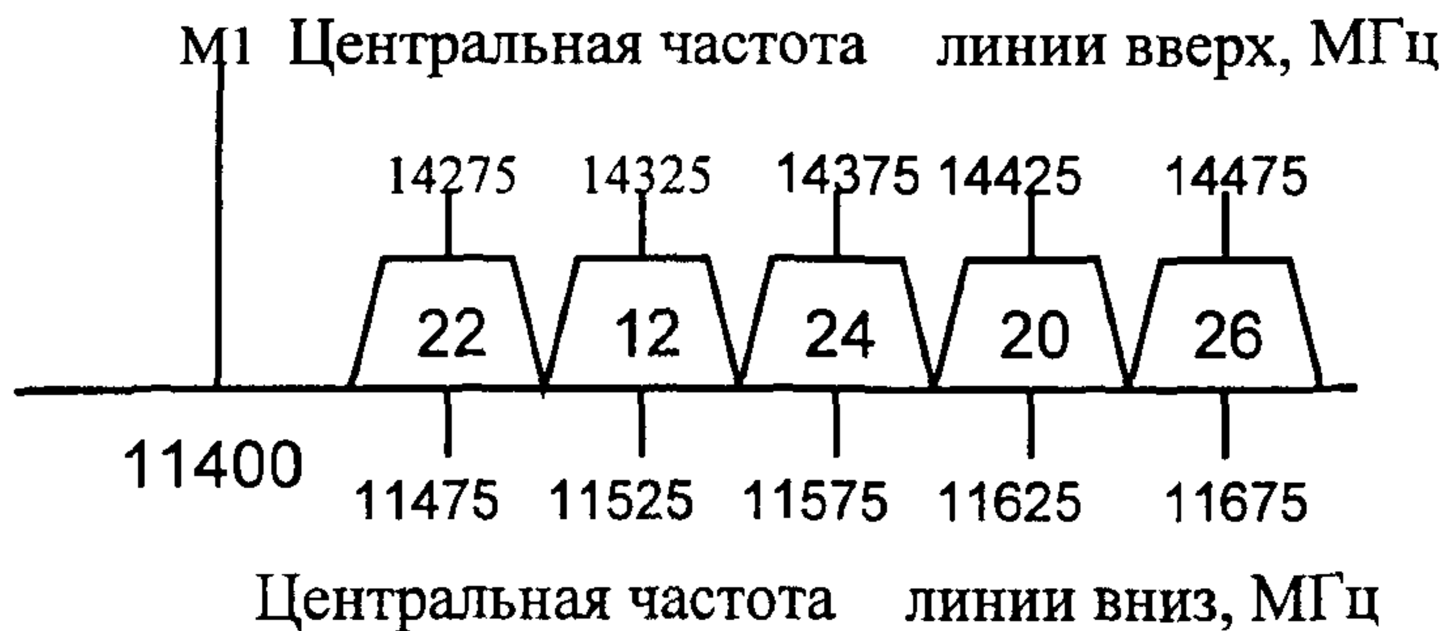
Рис. 3.6.3. Схема частотного плана стволов КА "Экспресс-А"
