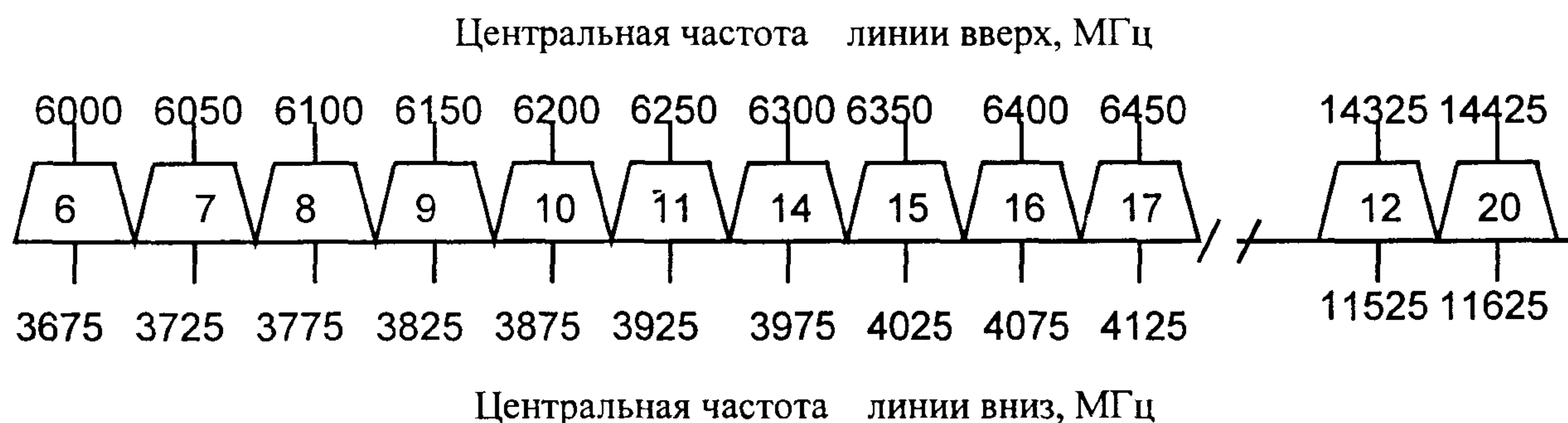
Рис. 3.6.2. Схема частотного плана стволов КА "Экспресс"
