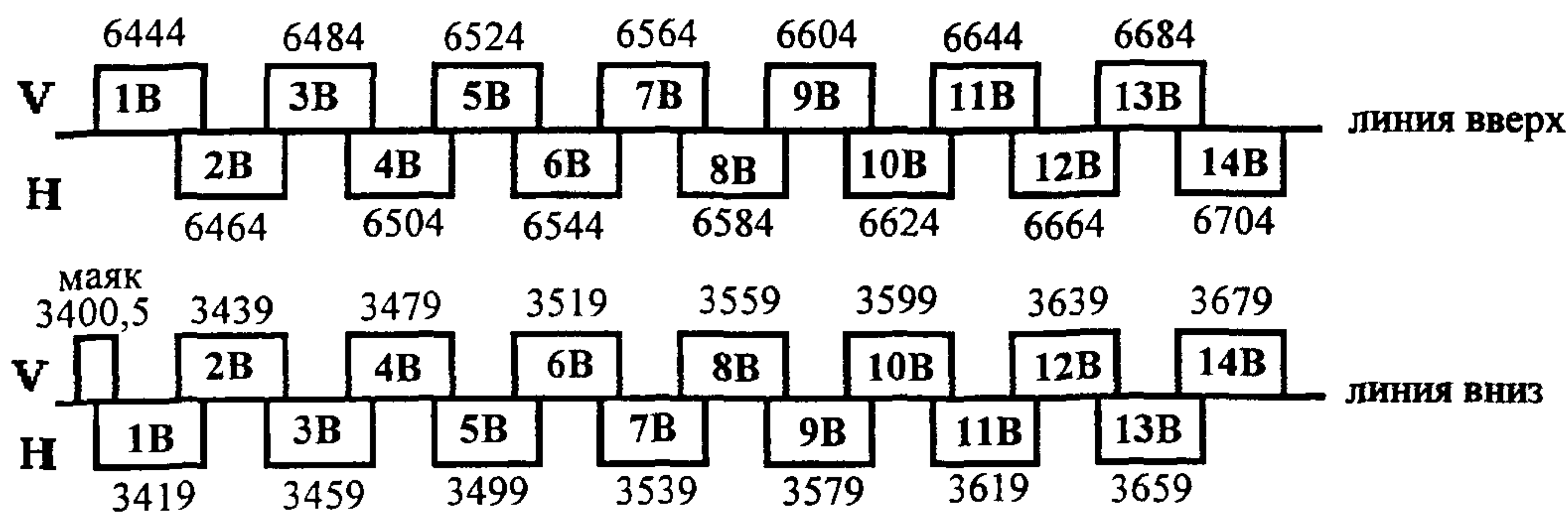
Рис. 3.6.4 Схема частотного плана стволов КА "LMI-1"
