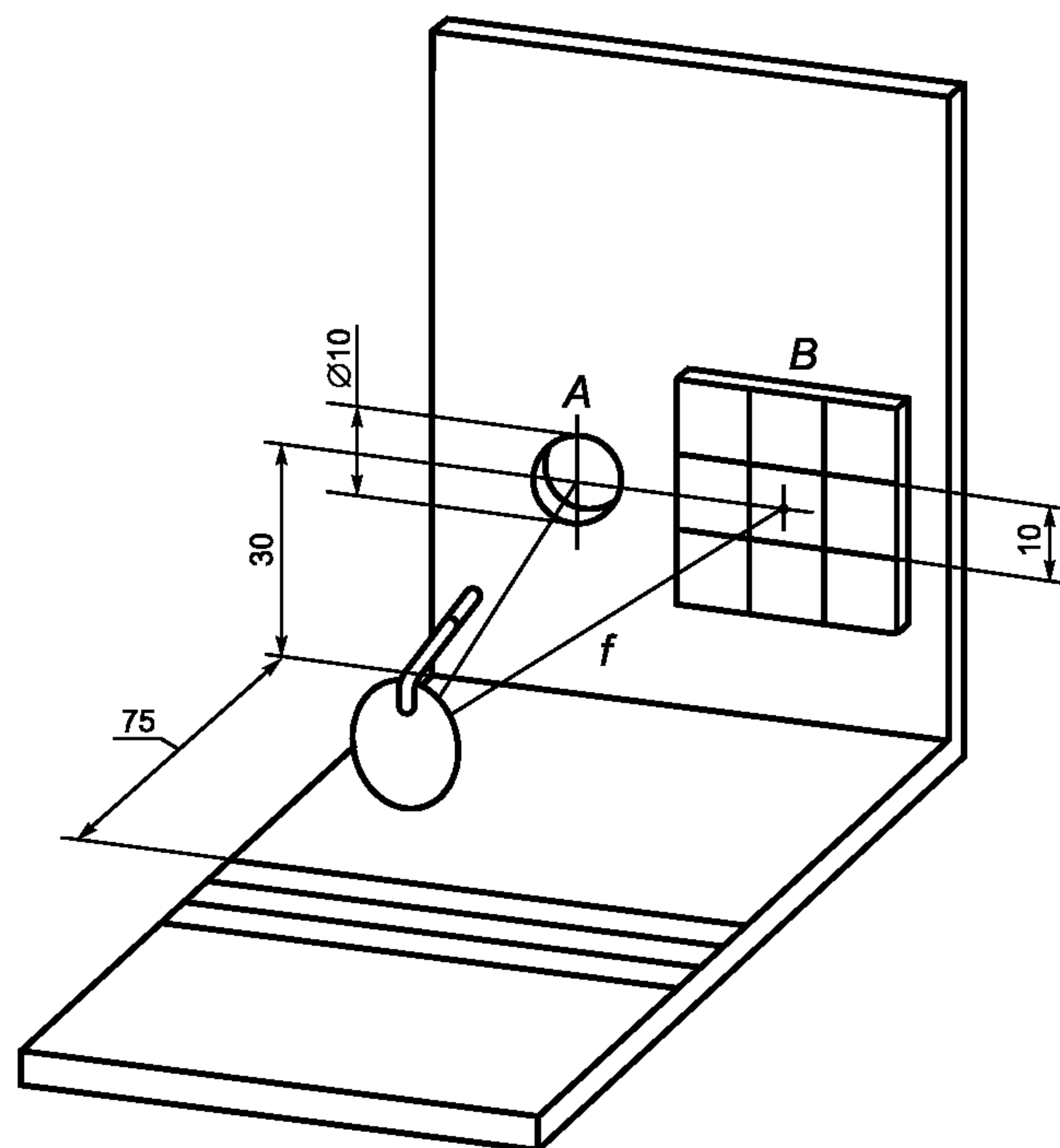
Рисунок 2 — Устройство для определения номинального увеличения
