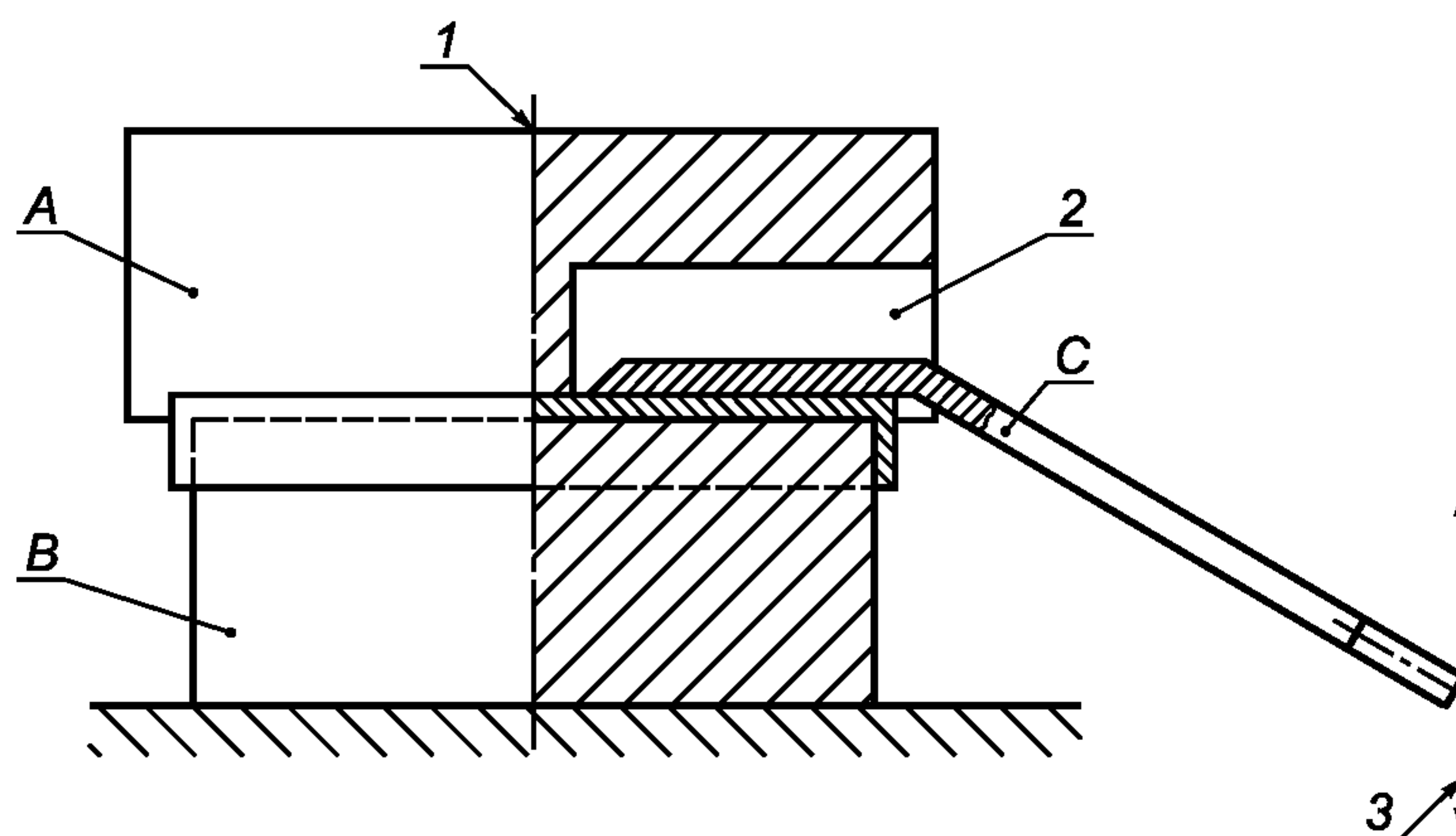
1 — зажим; 2 — паз; 3 — приложение нагрузки
