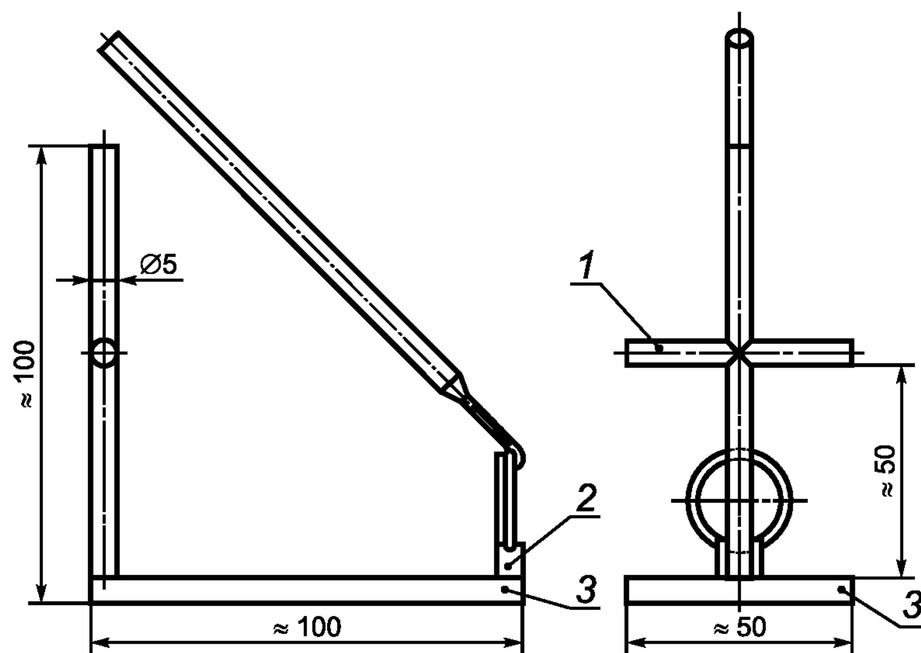
Рисунок 3 — Устройство для проверки искажений (см. 4.3.4)
