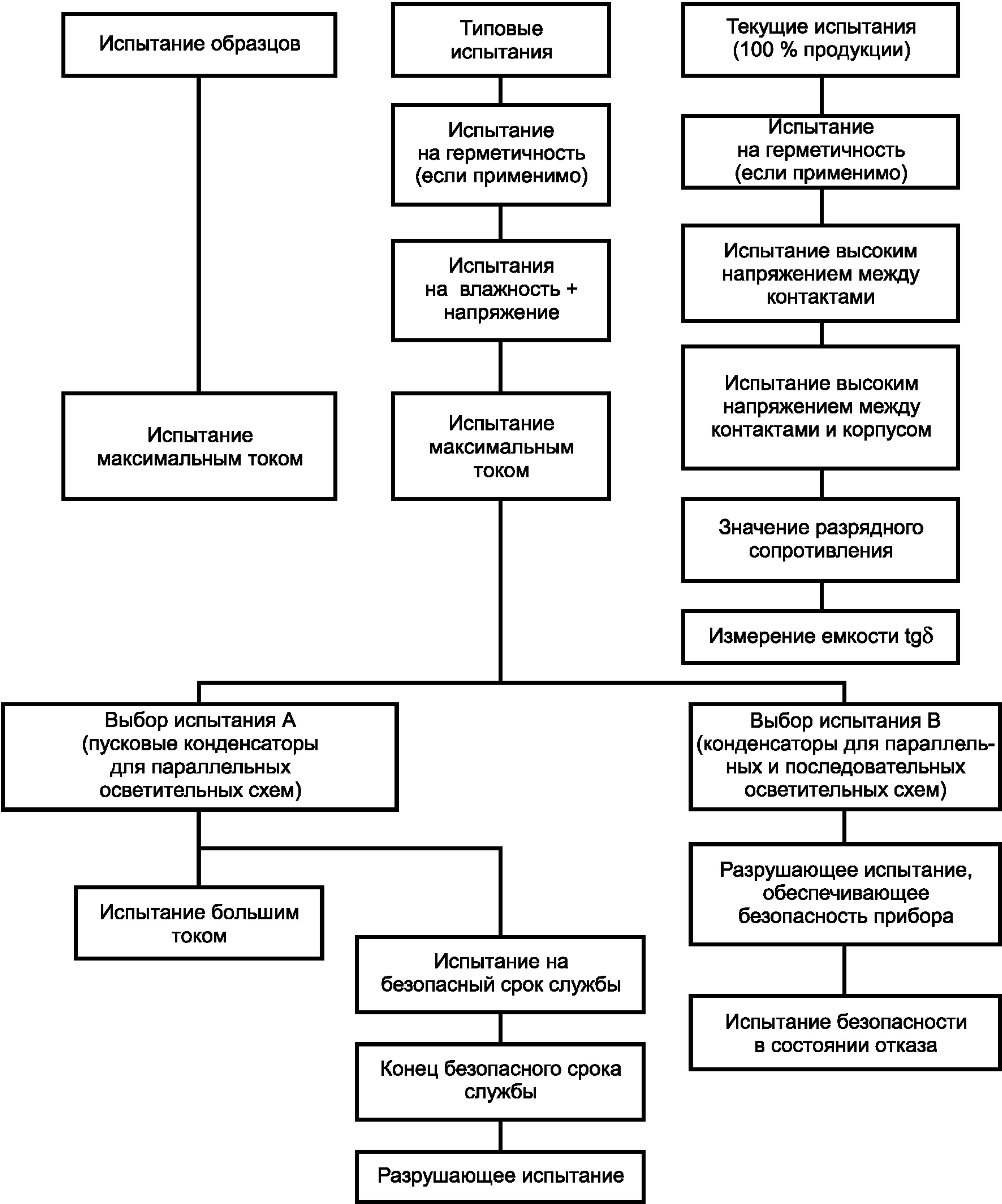
Рисунок 4— Схема процедуры испытаний
