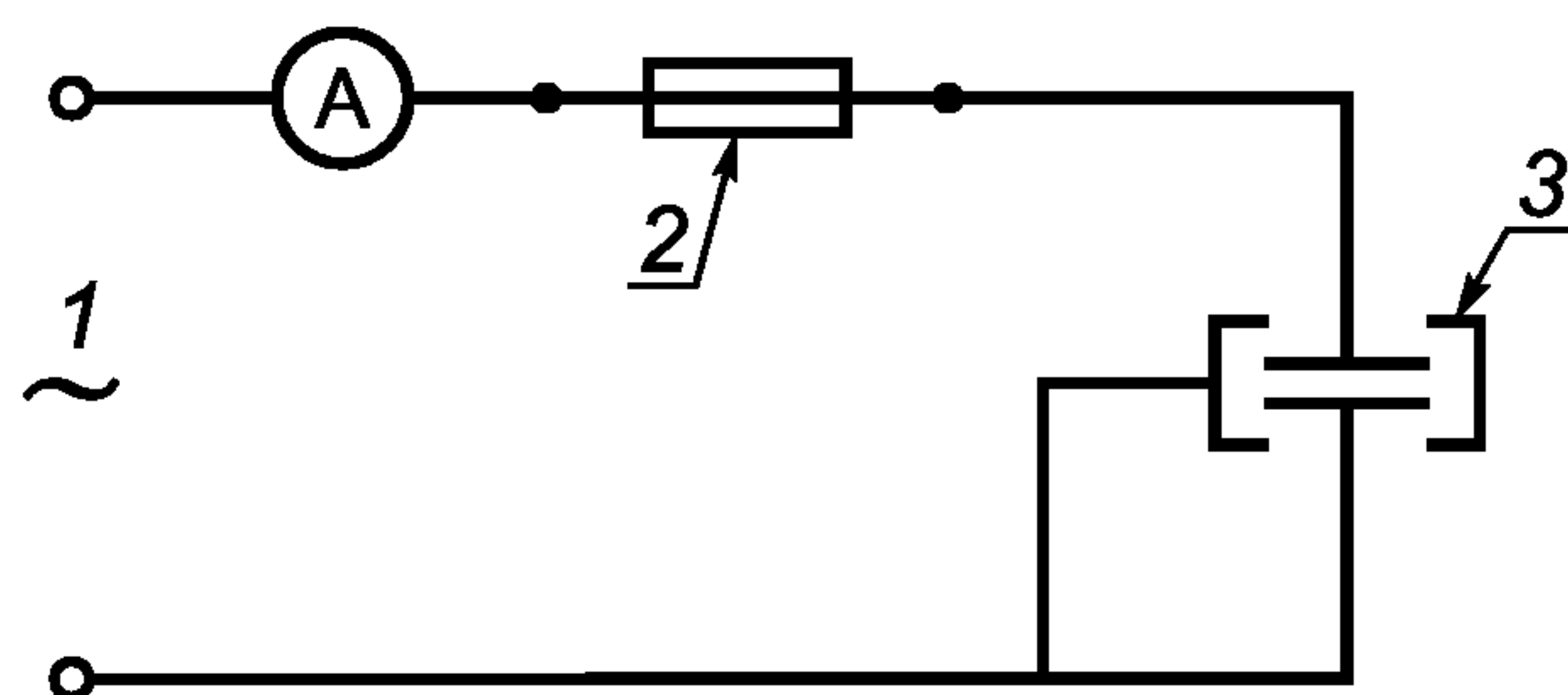
1 — источник переменного напряжения; 2 — плавкий предохранитель; 3 — конденсатор
