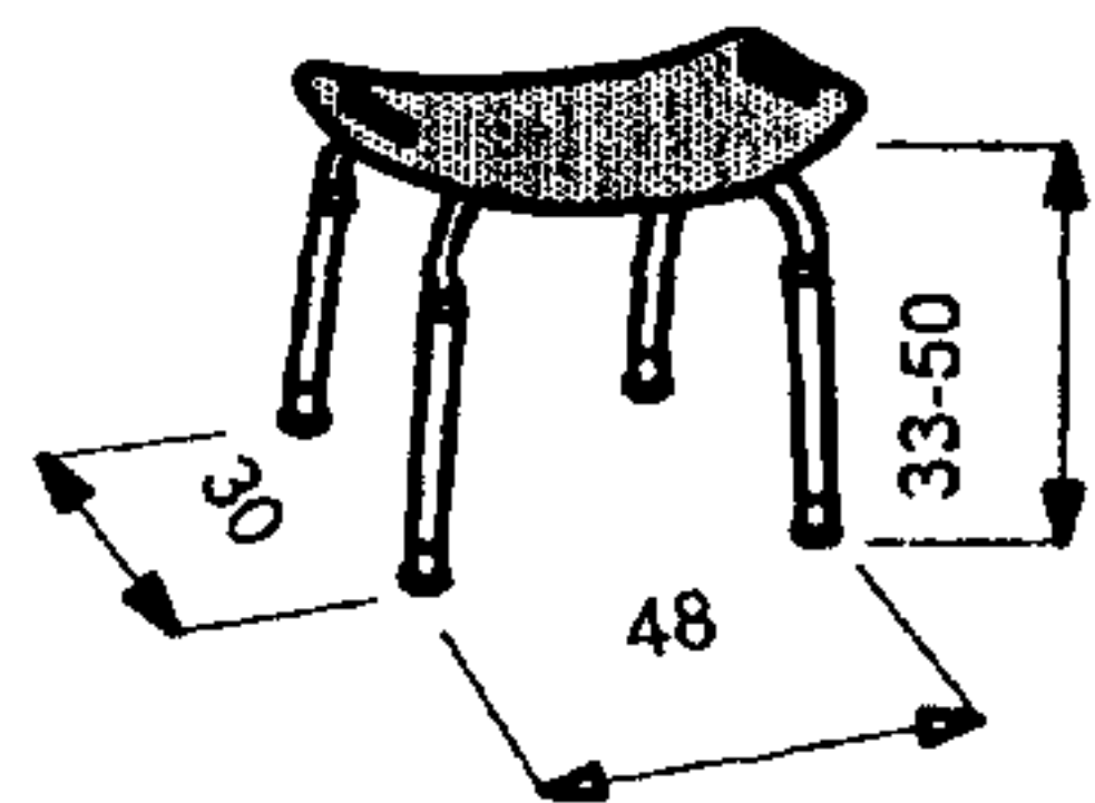
Стульчики для ванны
