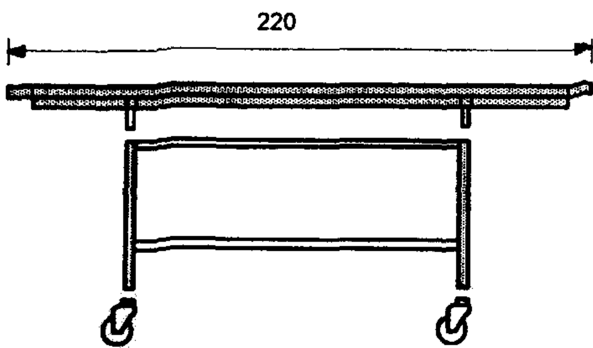
Каталка больничная со съемными носилками
