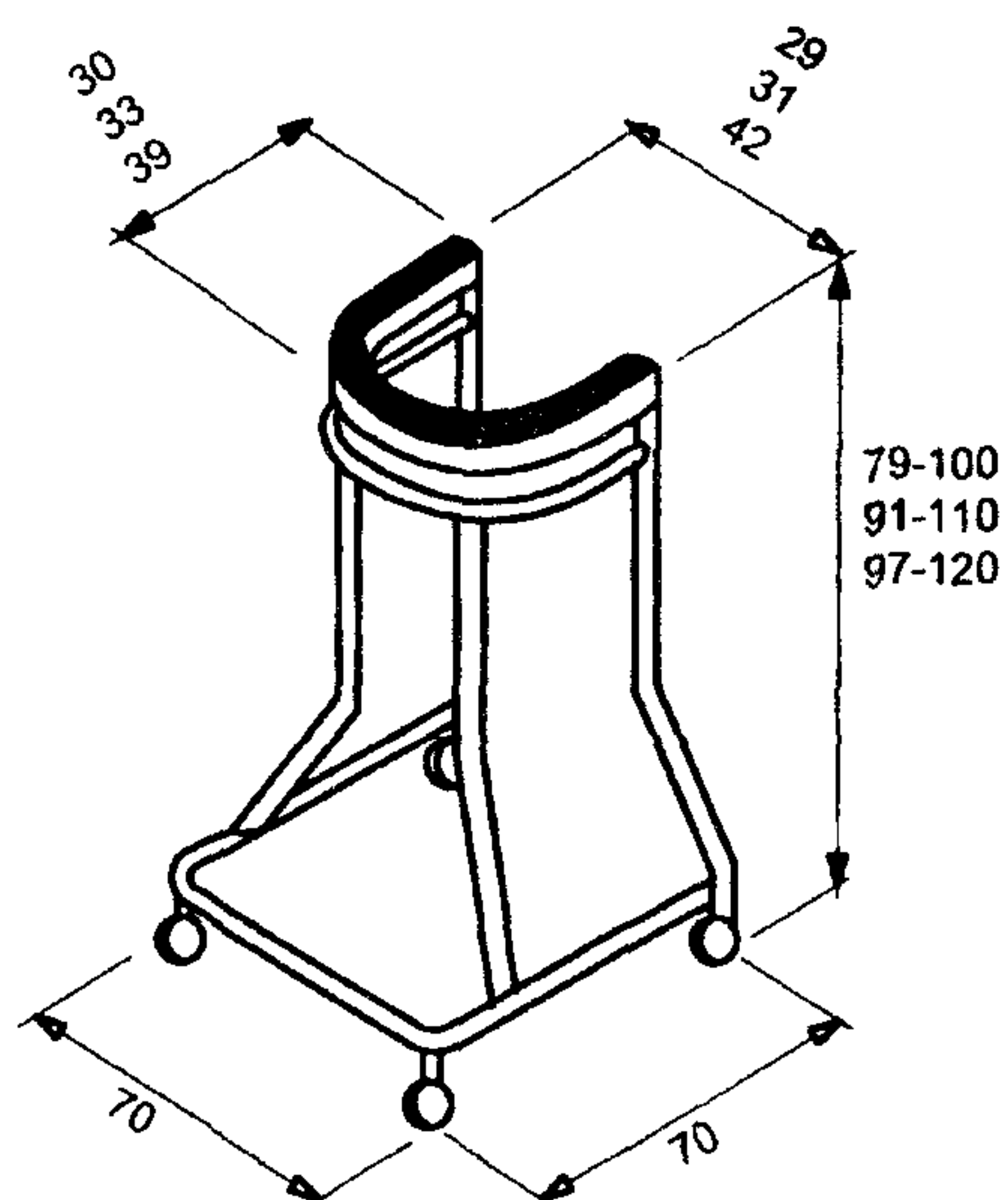
Ходунок на колесиках
