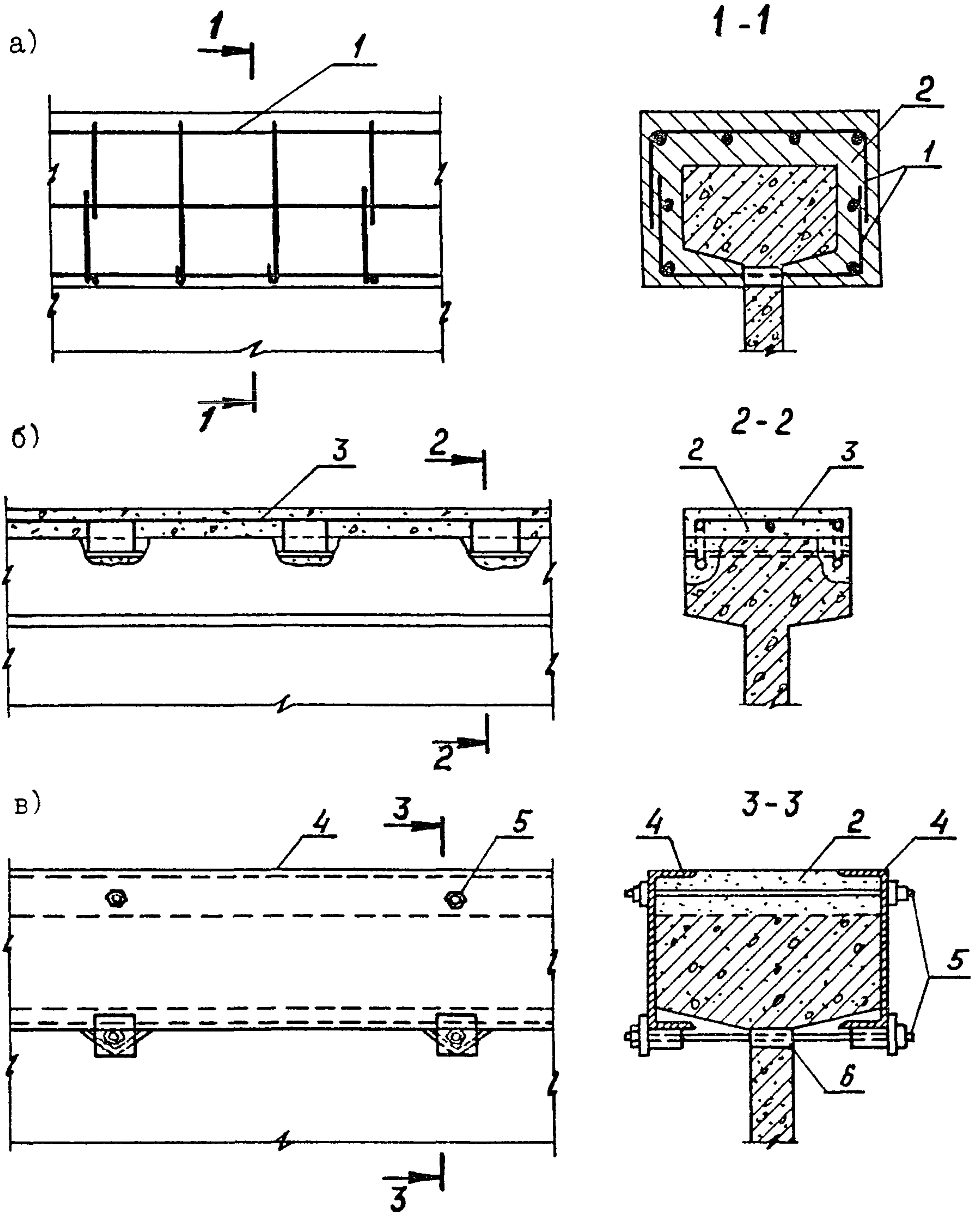
Рис. 4.8. Усиление верхней полки железобетонных балок
