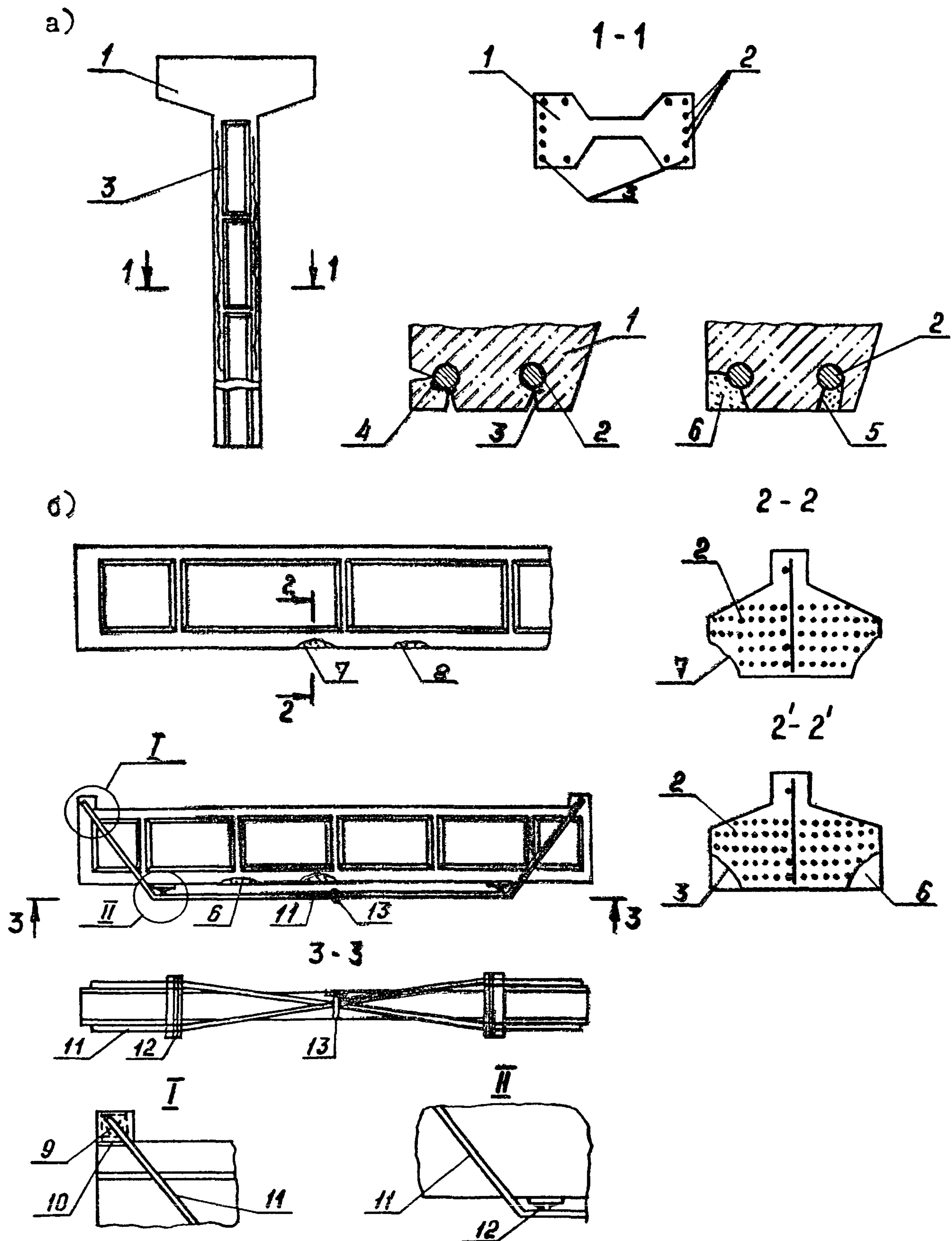
Рис. 5.33. Усиление технологической эстакады под трубопроводы
