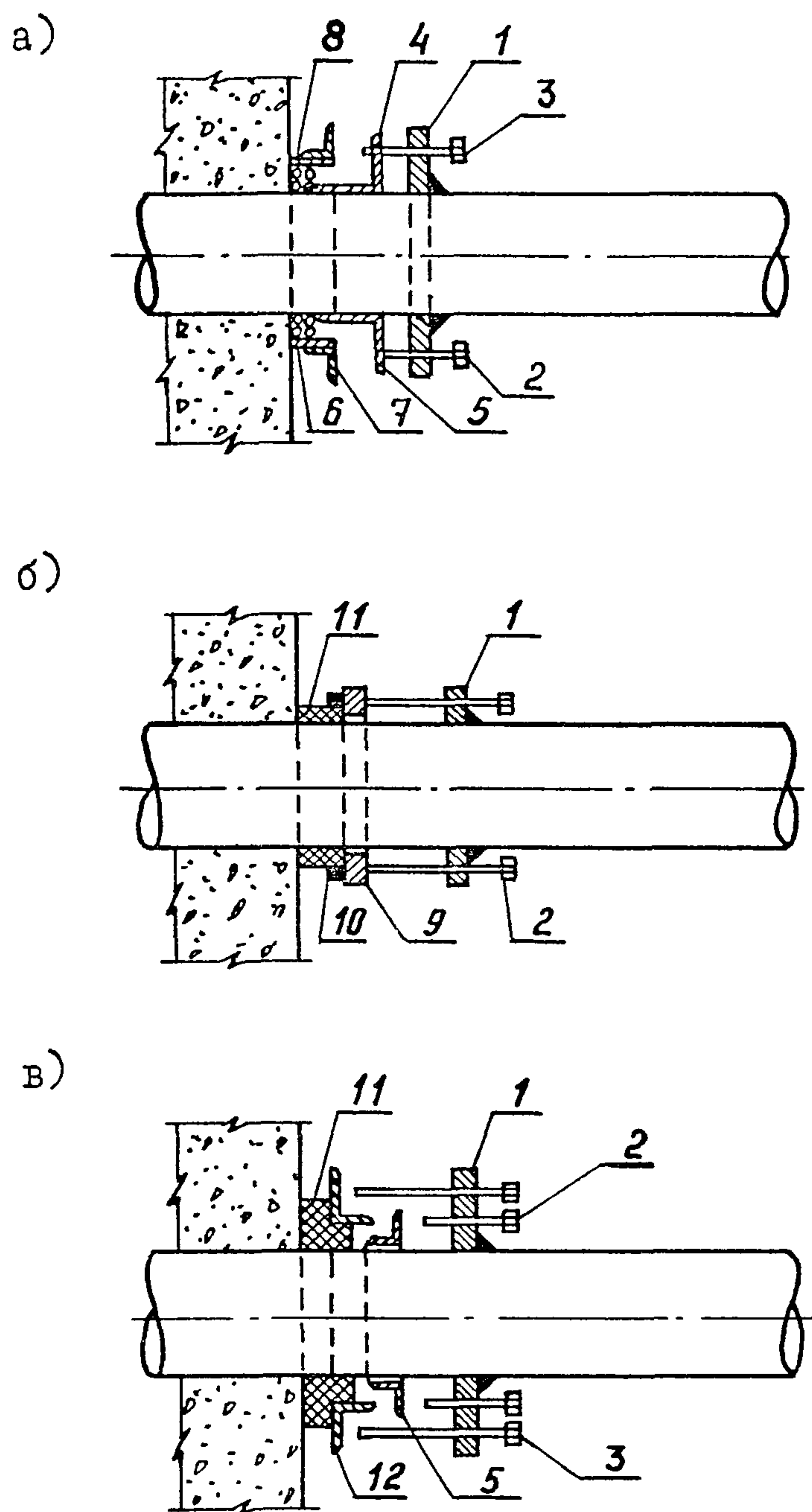
Рис. 5.5. Герметизация места вводов трубопроводов в резервуар с помощью уплотняющих прокладок
