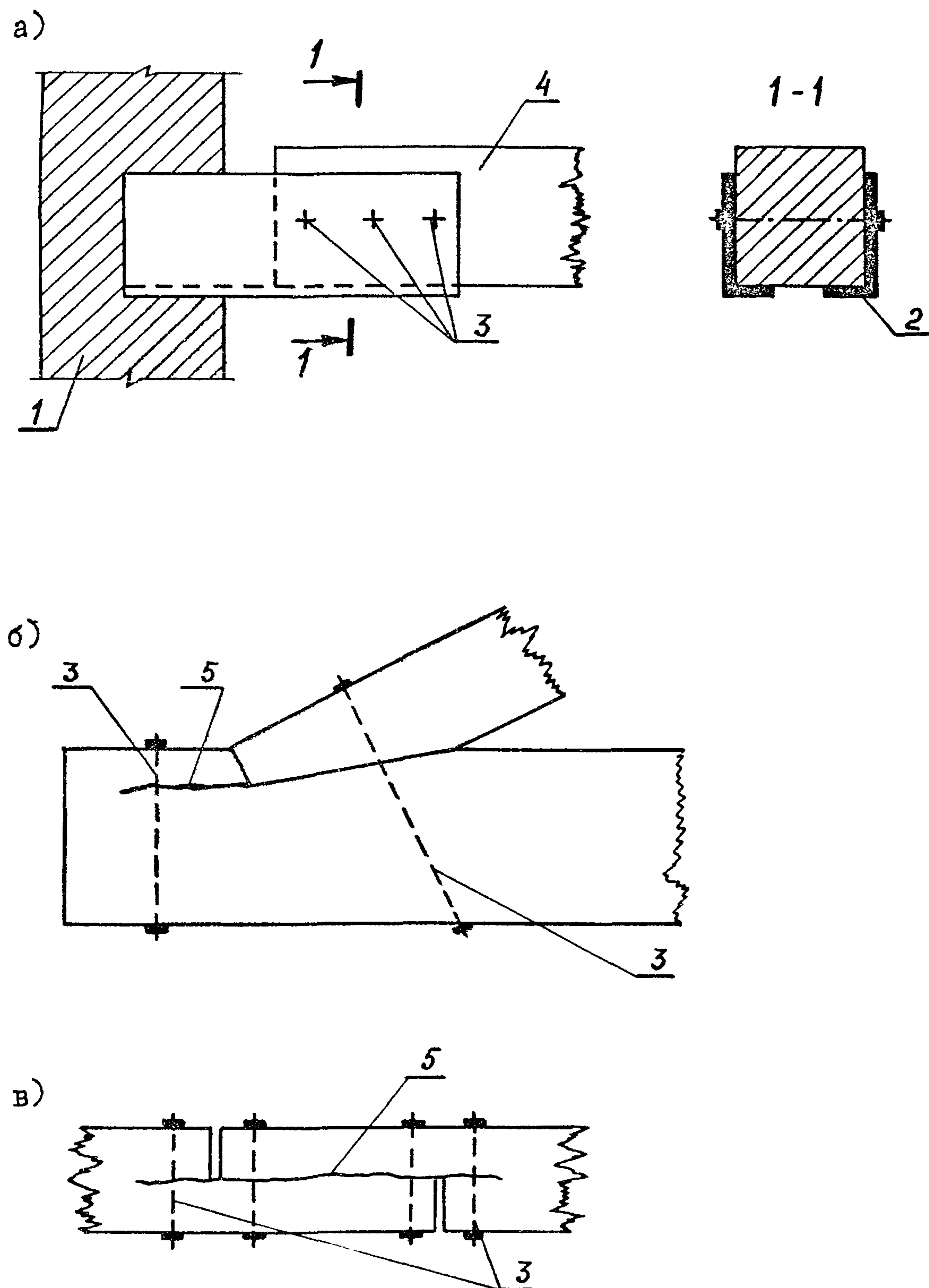
Рис. 4.19. Усиление узлов деревянных конструкций
