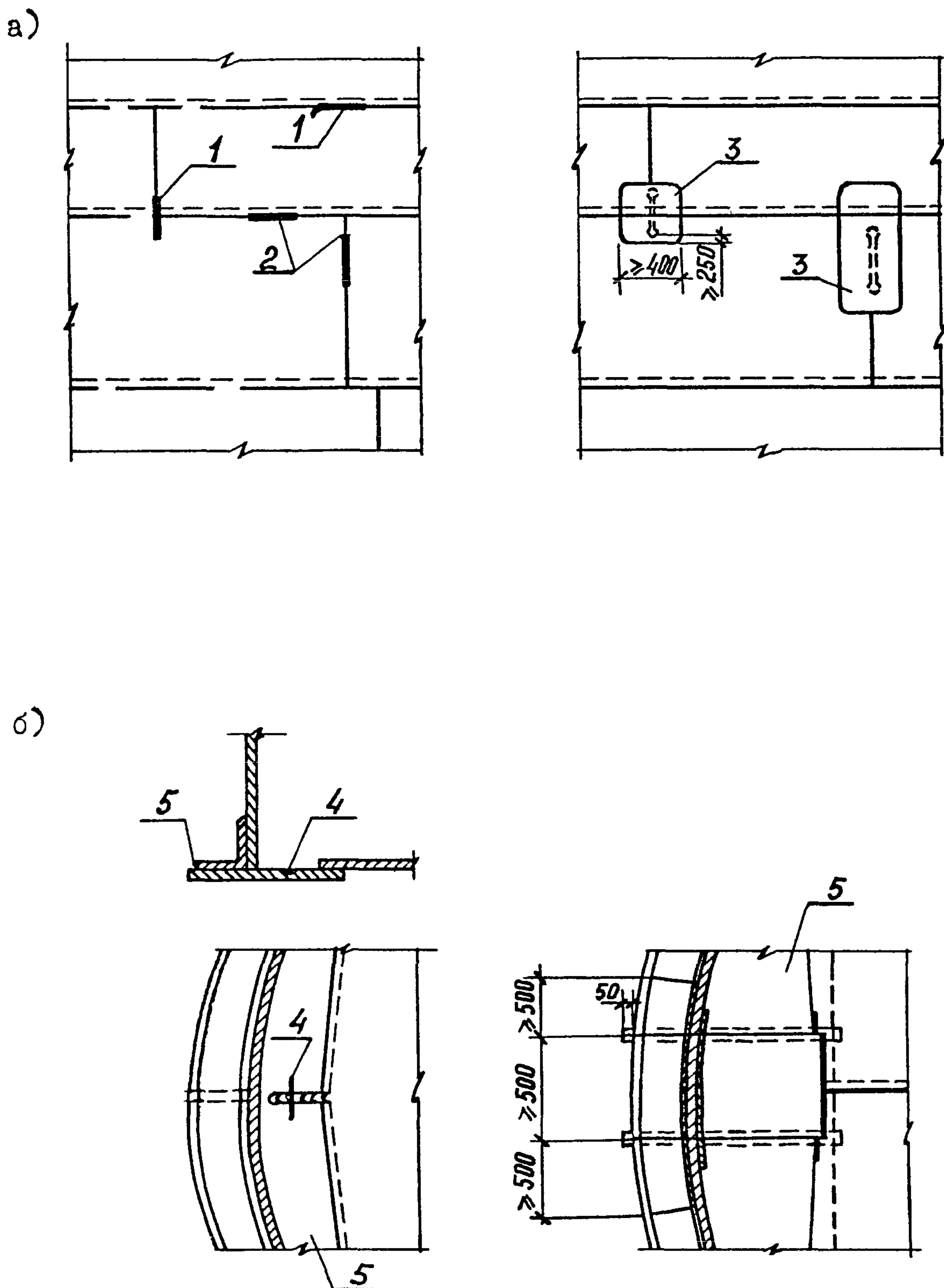
Рис. 5.17. Ремонт дна стального резервуара при трещинах в сварных швах
