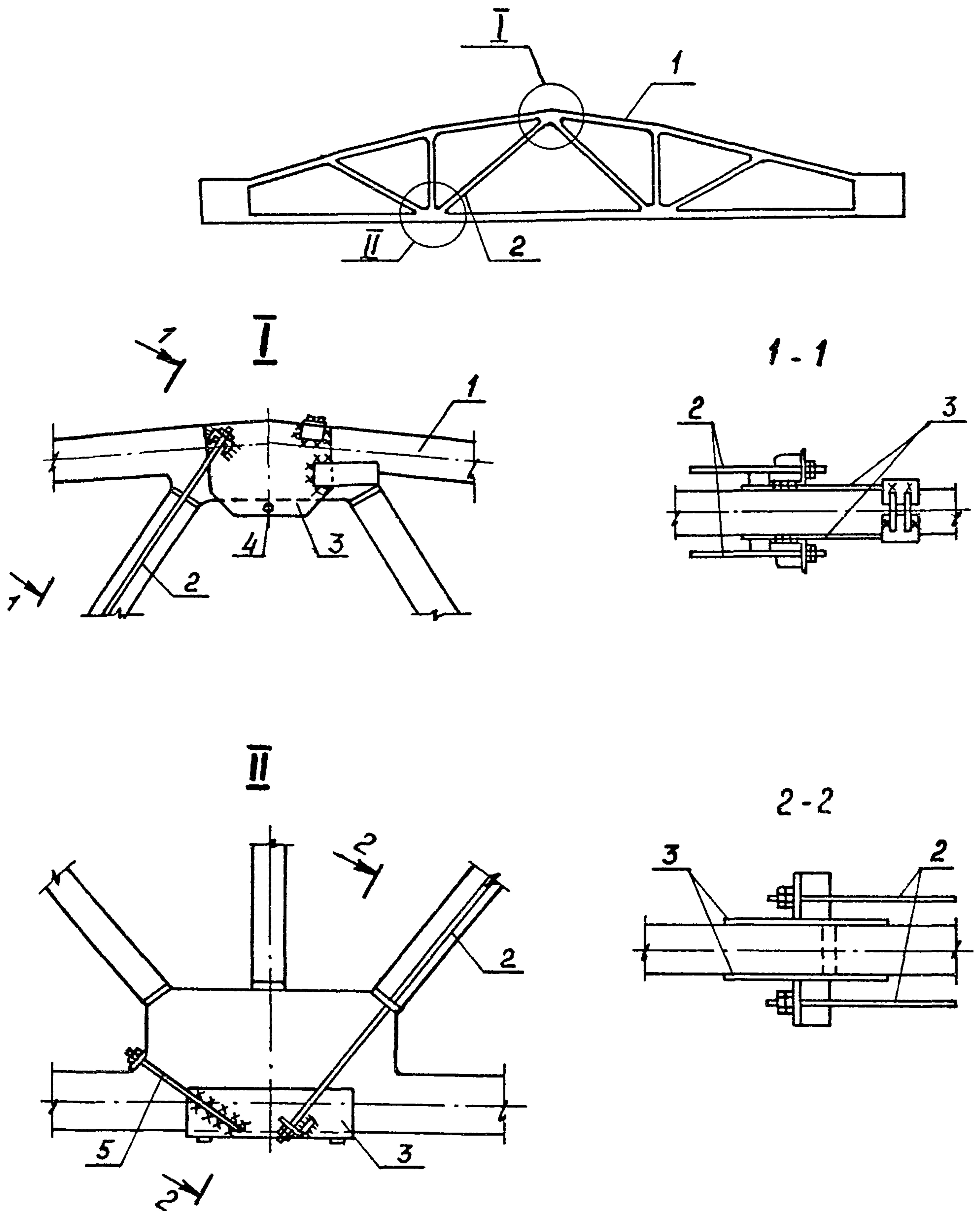
Рис. 4.12. Усиление растянутых элементов решетки ферм
