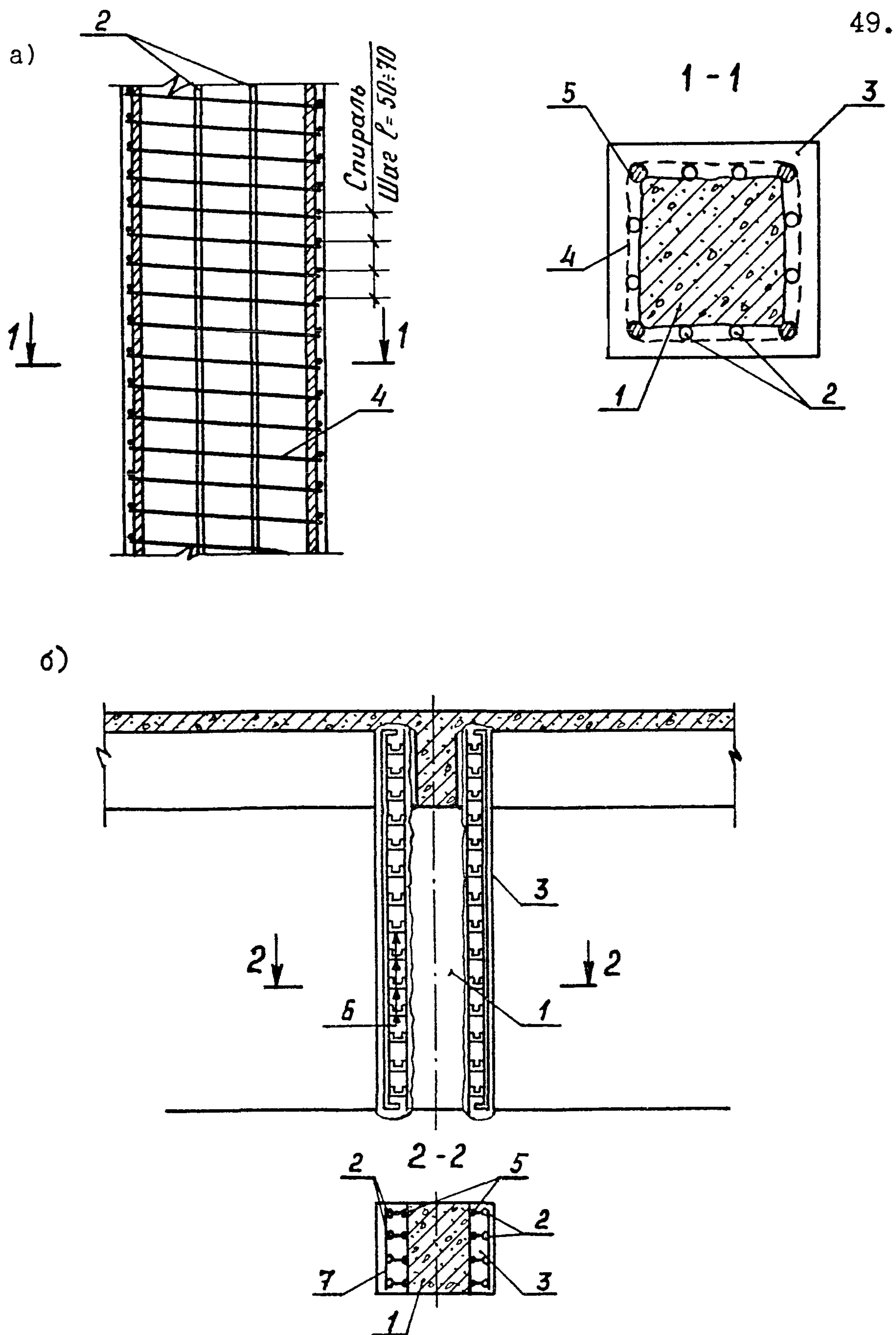
Рис. 4.13. Усиление железобетонных колонн
