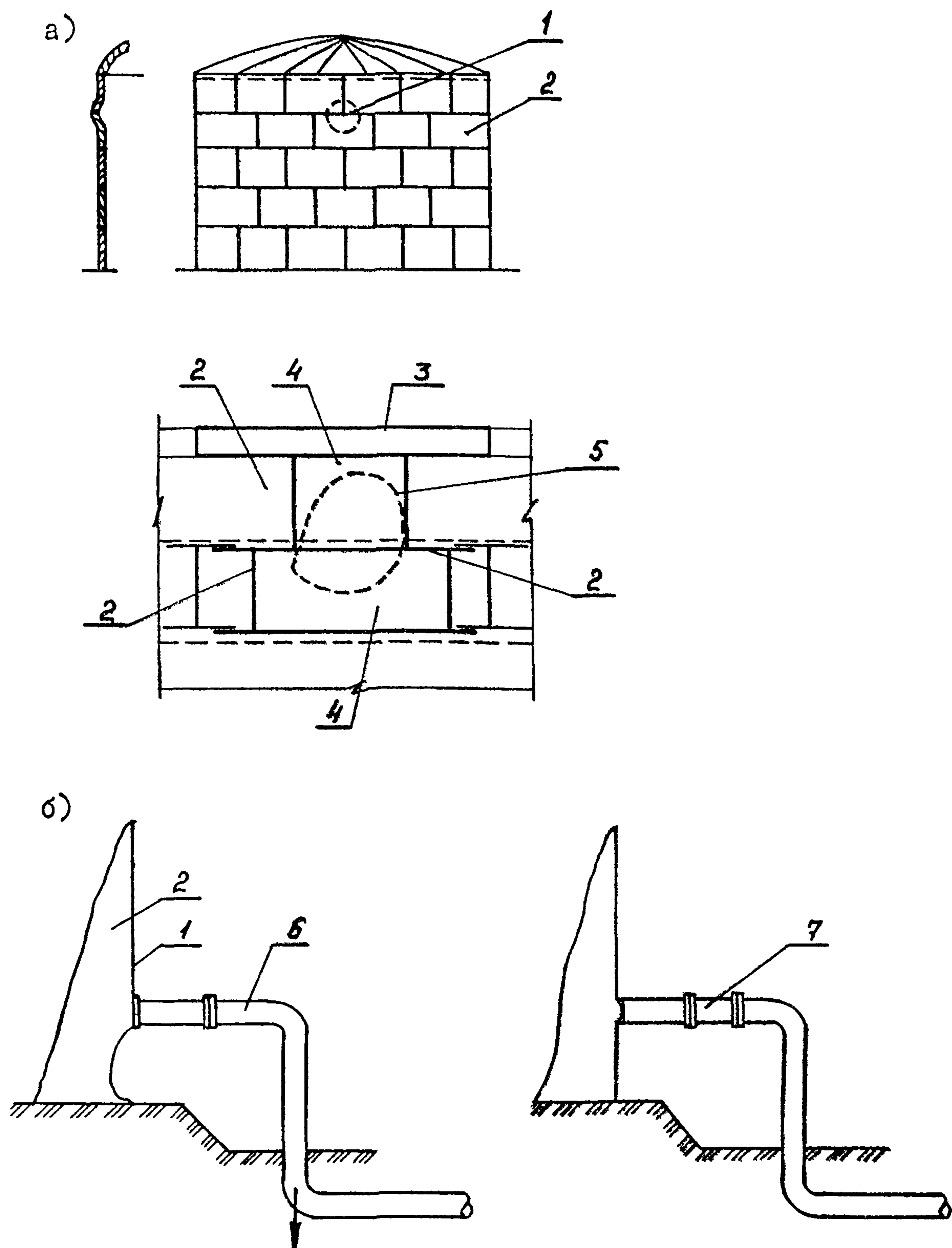
Рис. 5.20. Ремонт деформированных стен стального резервуара
