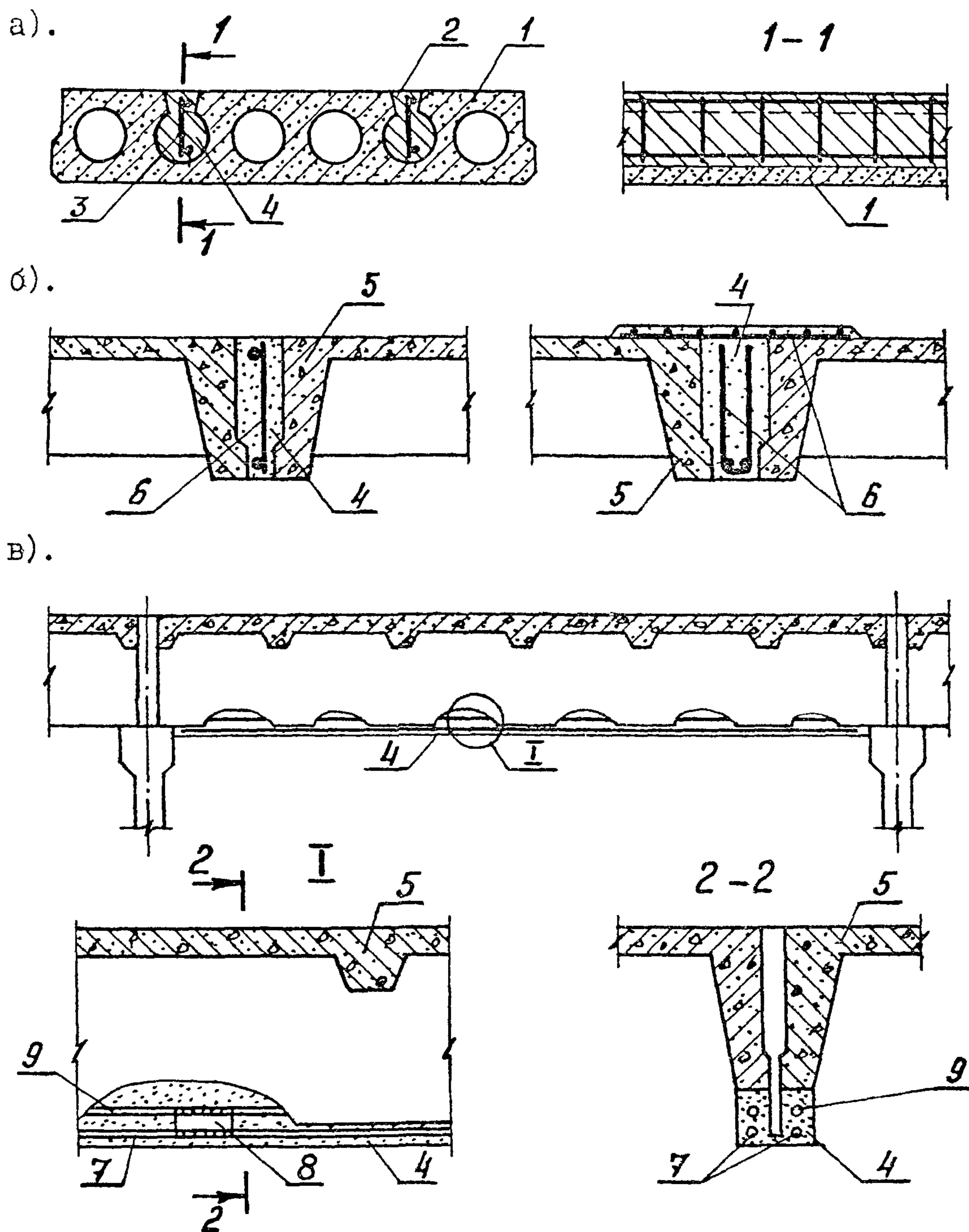
Рис. 4.6. Усиление ребер сборных плит
