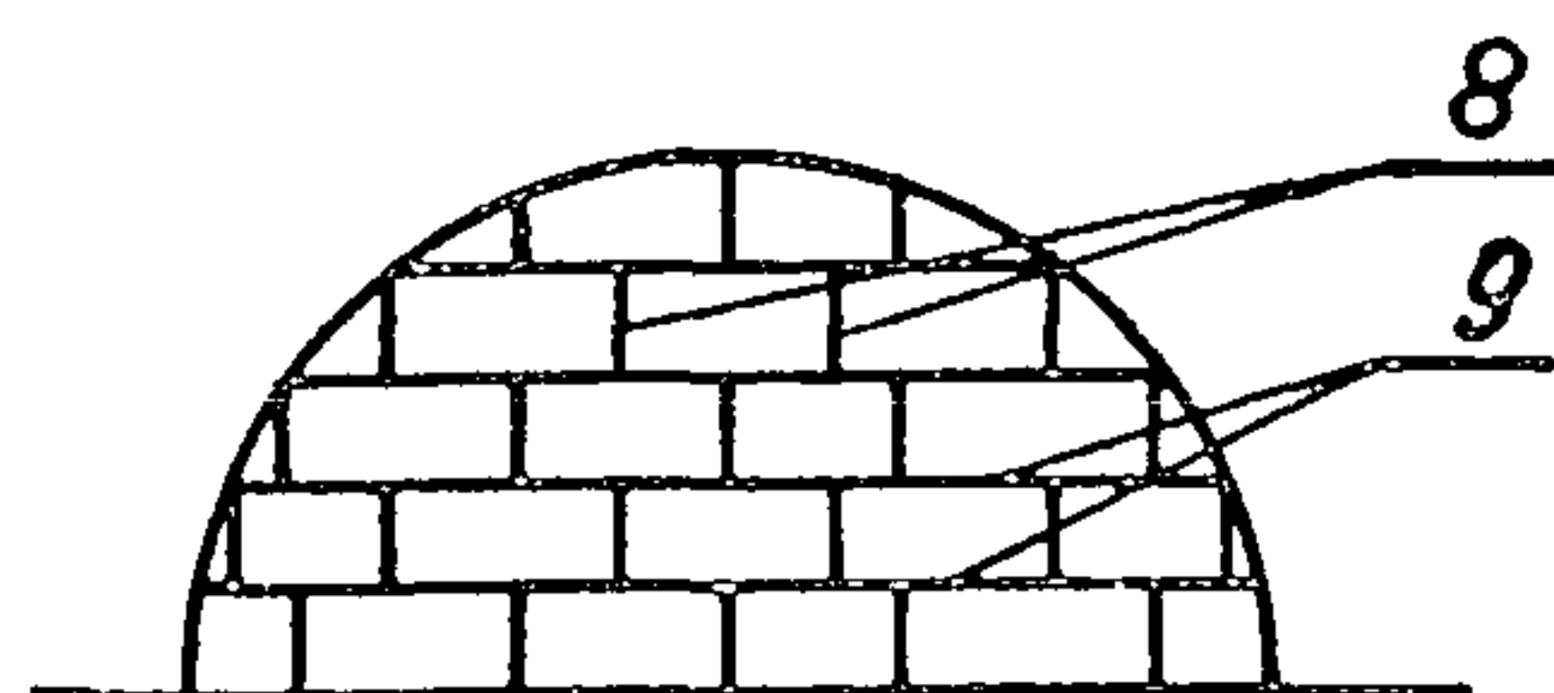
Рис. 5.21. Ремонт покрытия стального резервуара
