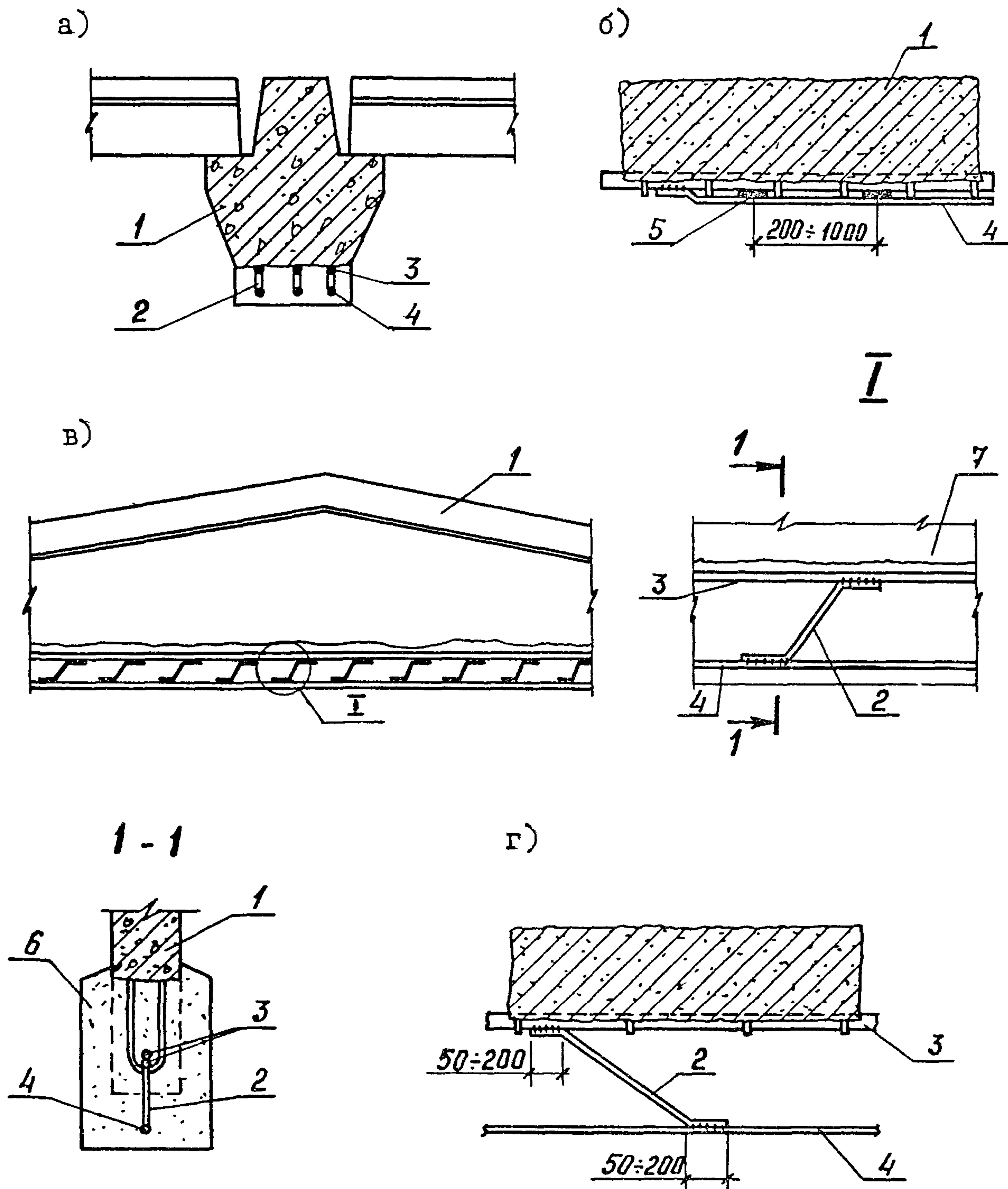
Рис. 4.9. Усиление железобетонных балок
