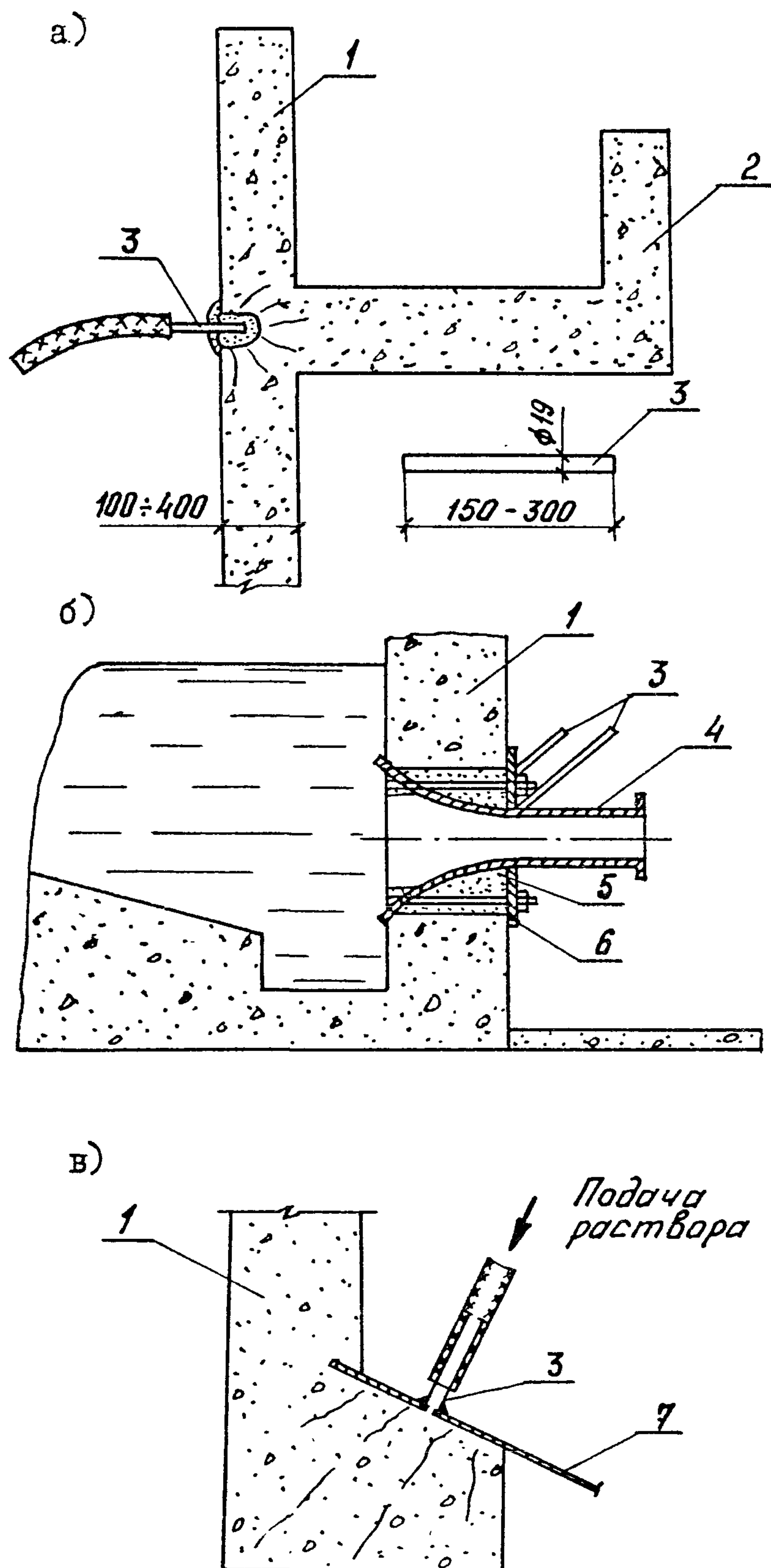
Рис. 5.1. Ремонт железобетонных емкостей при протечках
