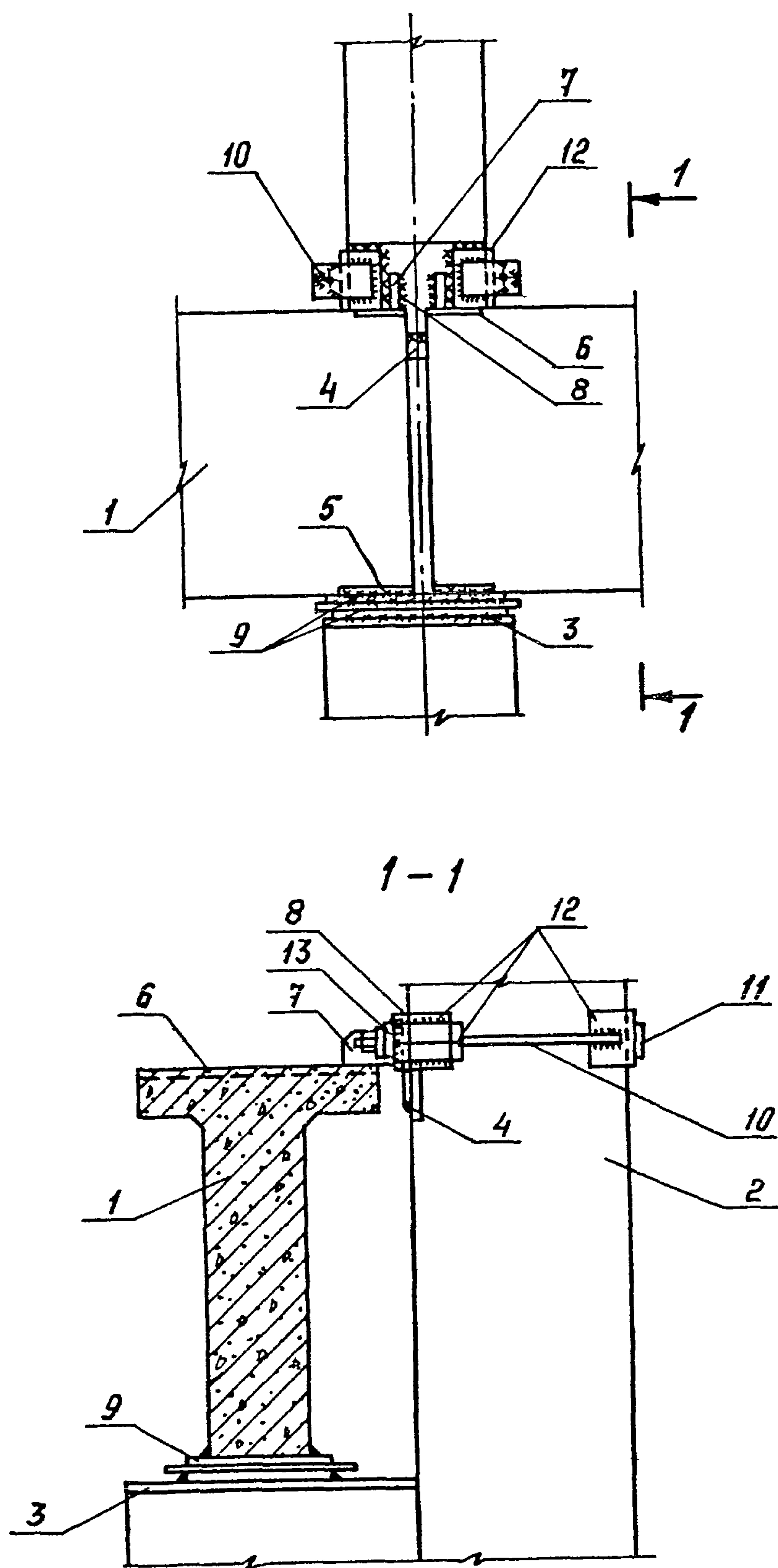
Рис. 5.37. Усиление крепления подкрановой балки к колонне
