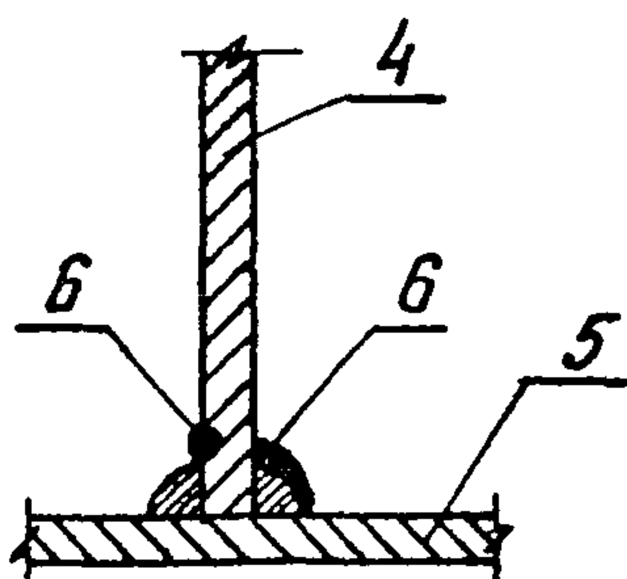
Рис. 5.19. Ремонт нижнего пояса стены стального резервуара
