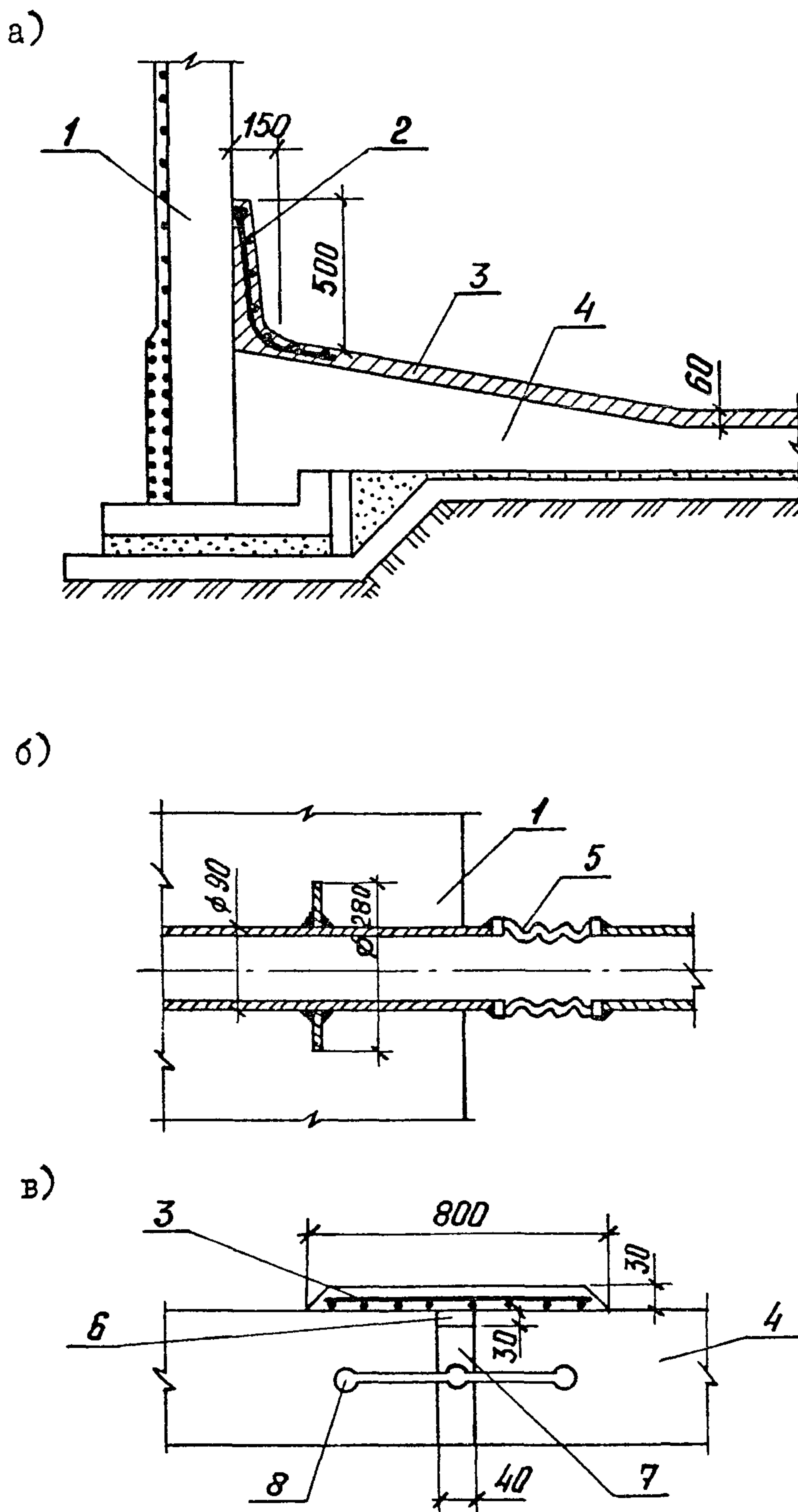
Рис. 5.3. Ремонт железобетонных емкостей
