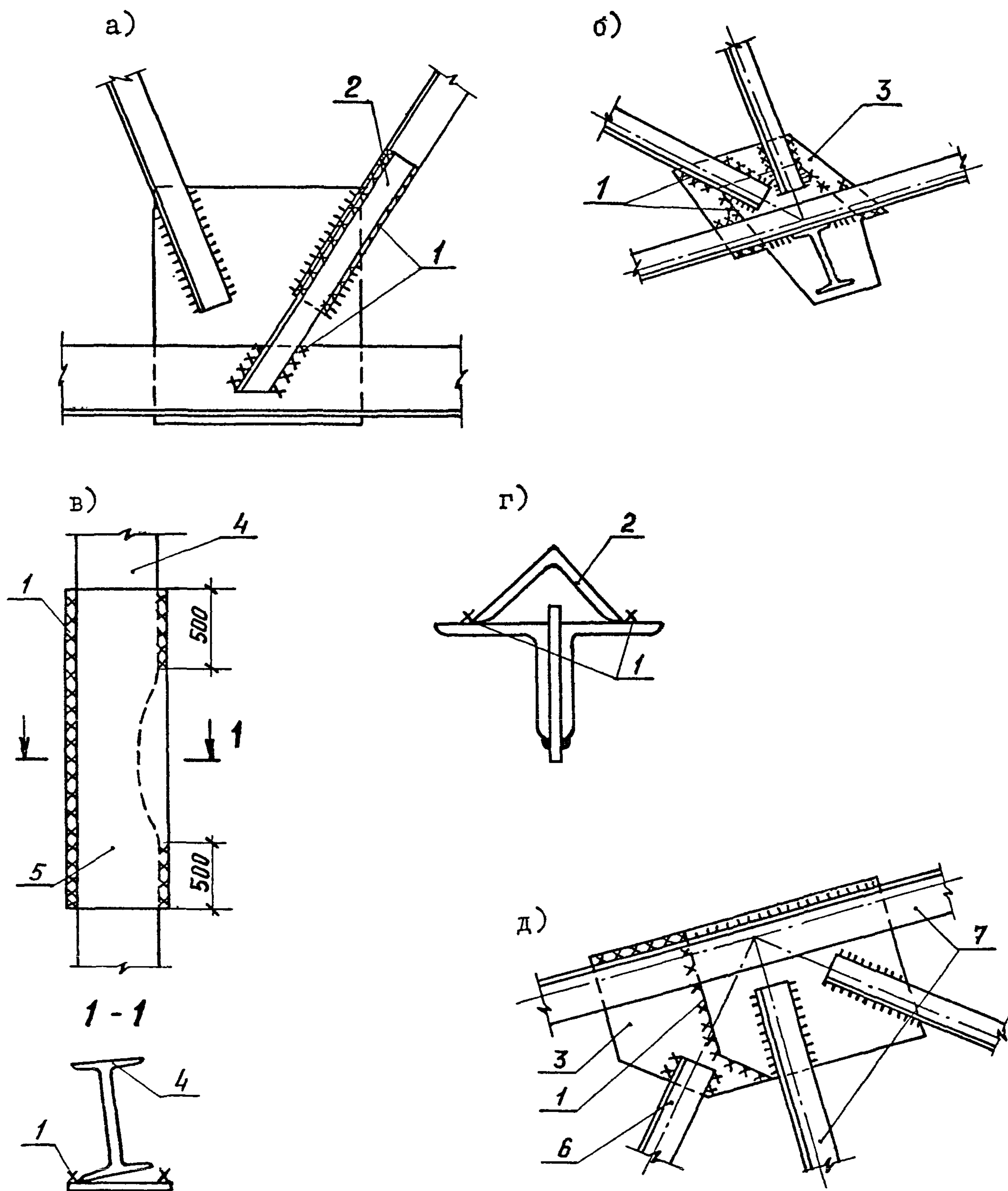
Рис. 5.31. Ремонт стальных конструкций конвейерных галерей а -раскоса при трещинах, коррозии или недостаточной длине свар- ных швов прикрепления; б -нижнего узла наваркой дополнительной фасонки; в -погнутой ветви опоры; г -раскосов фермы; е -верхне- го пояса фермы; 1 -монтажные сварные швы; 2 -усиливающий уголок 3 -дополнительная фасонка; 4 -ветвь опоры; 5 -усиливающая на- кладка; 6 -дополнительный стержень усиления фермы; 7 -существу- ющие стержни фермы.
