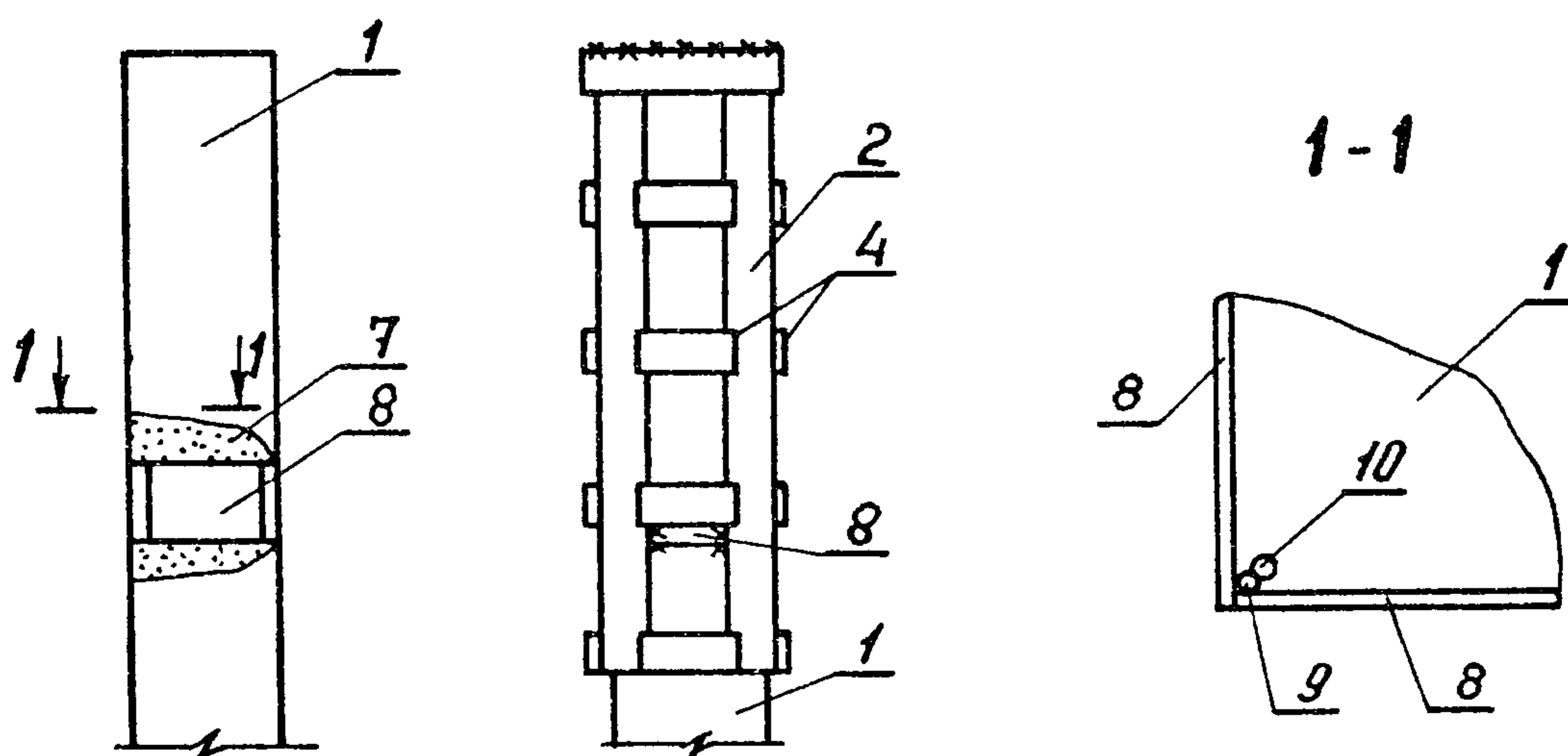
Рис. 4.14. Усиление железобетонных колонн стальной обоймой
