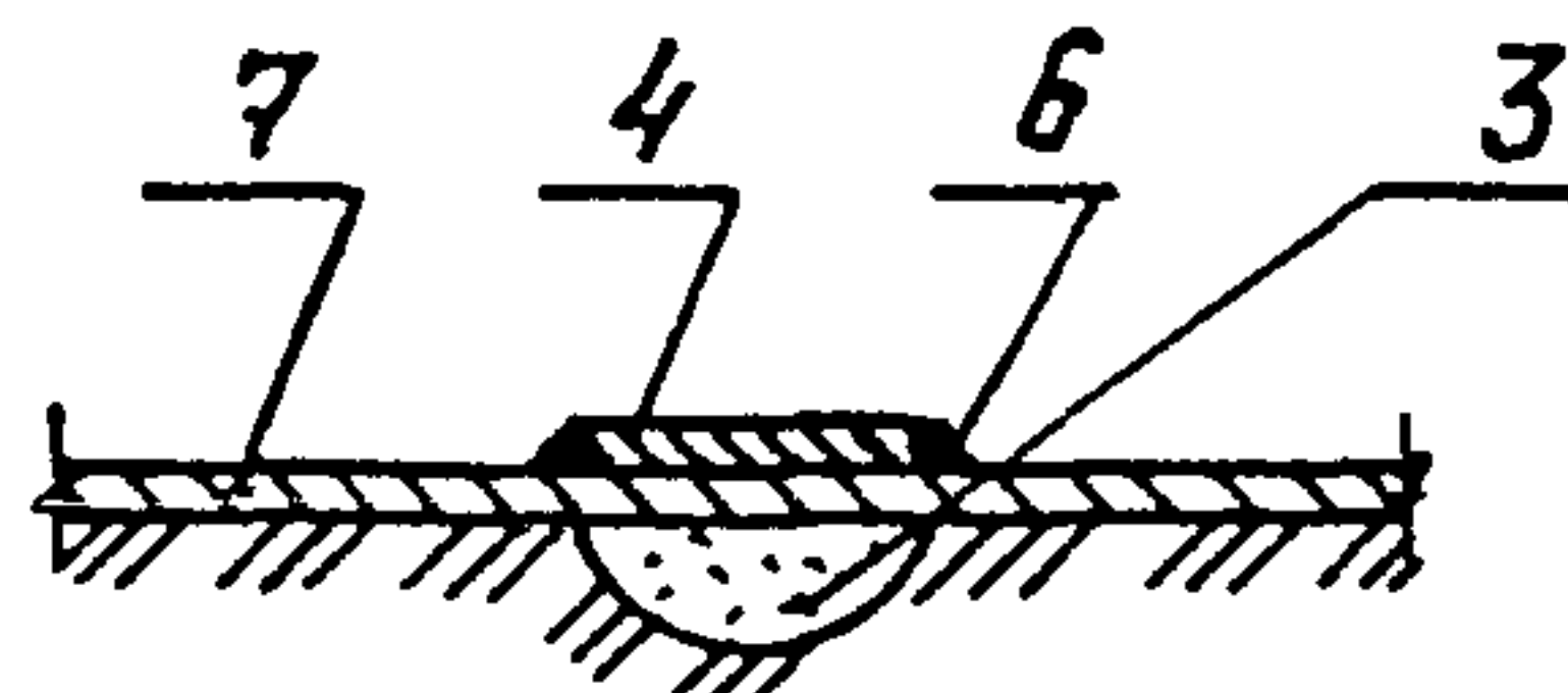
Рис. 5.14. Местный ремонт дна стального резервуара
