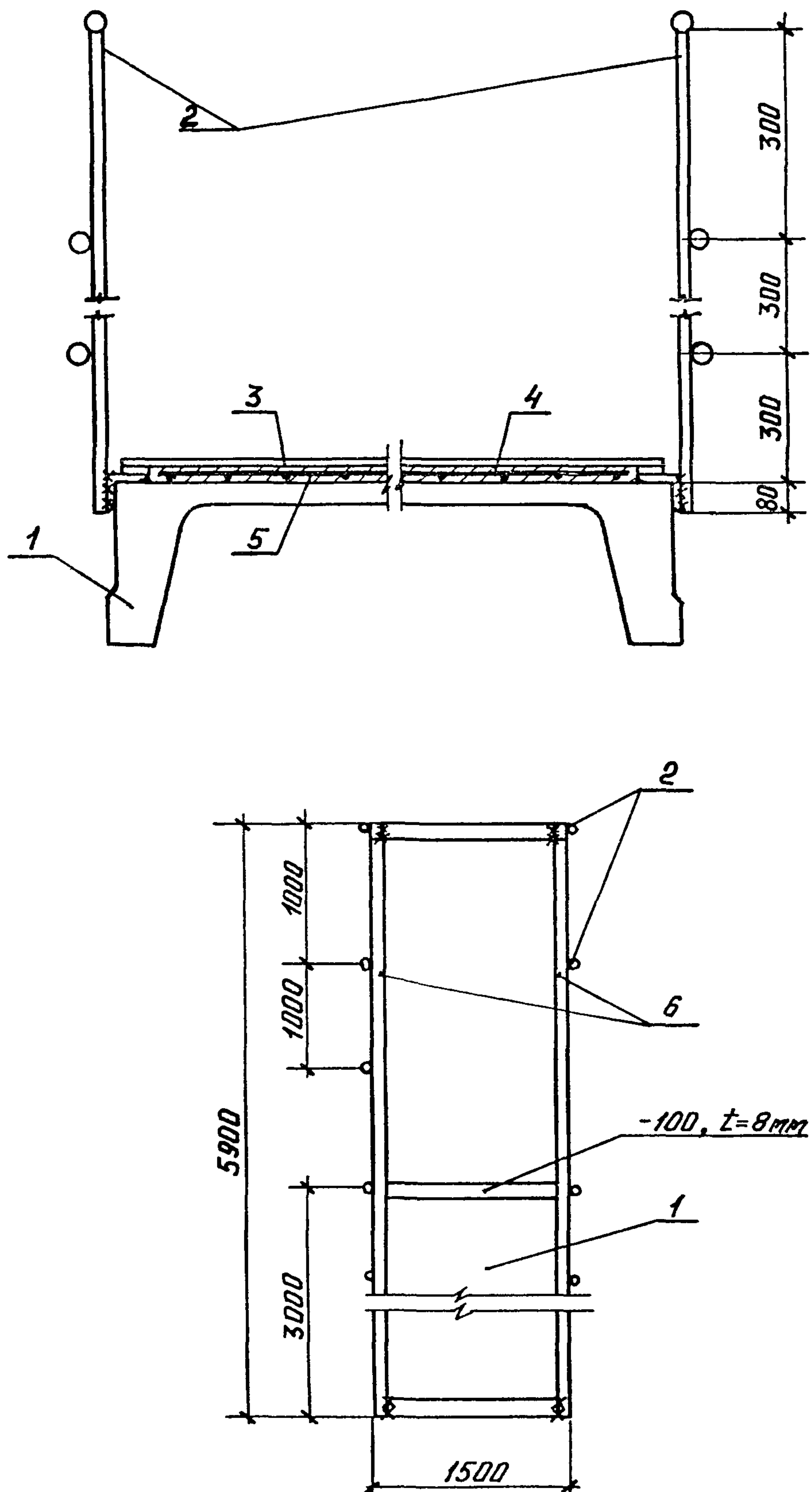
Рис. 5.11. Усиление конструкций сборных мостиков
