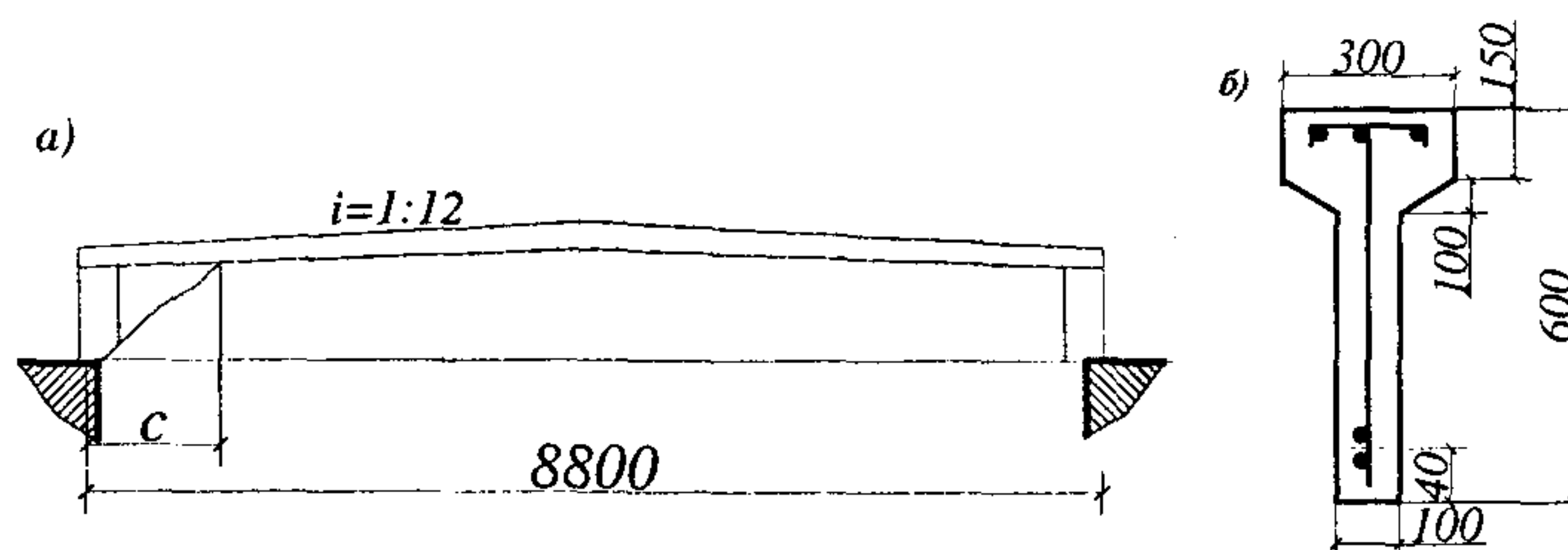
Черт.3.23. К примеру расчета 16
