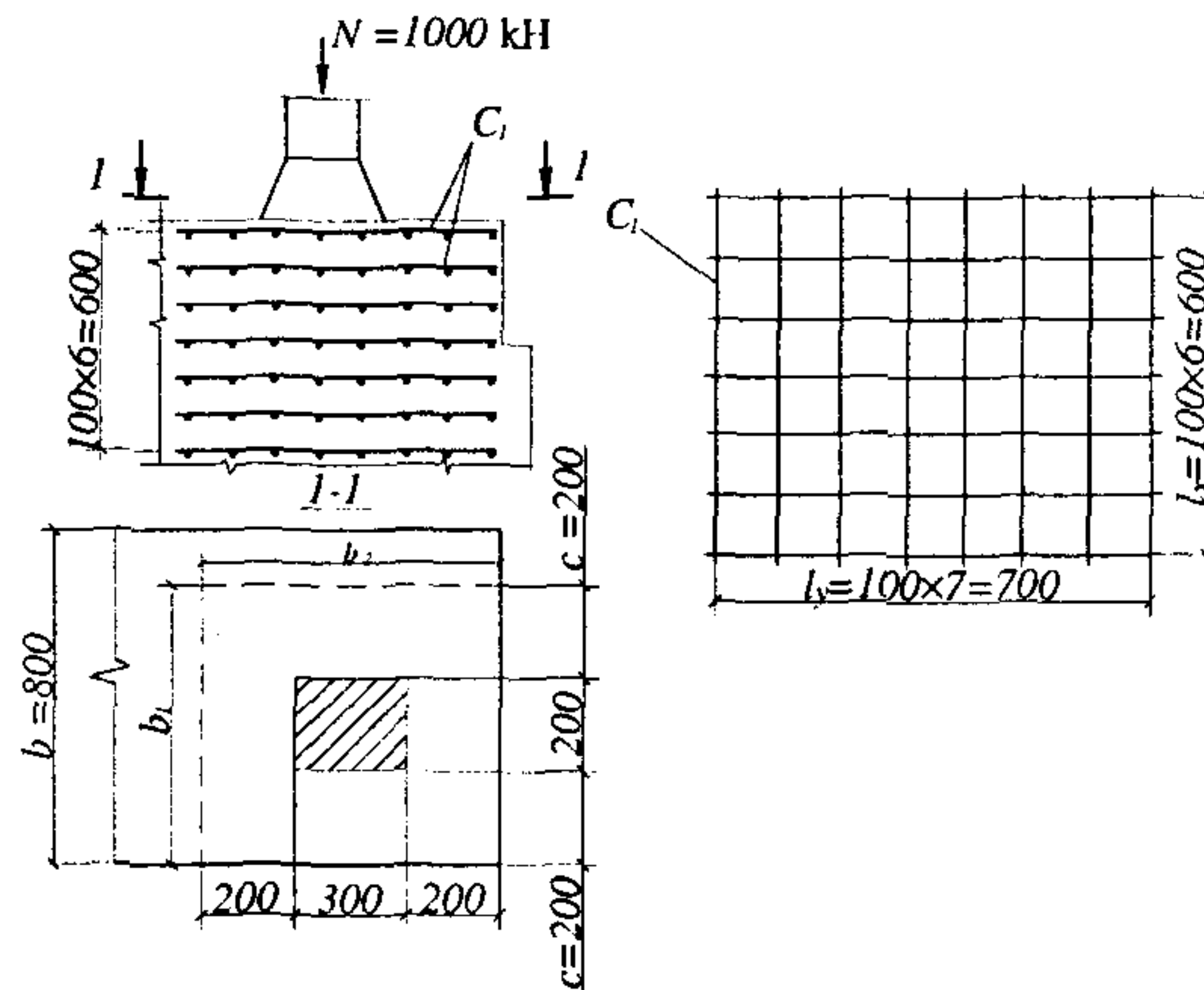
Черт.3.45.К примеру расчета 39
