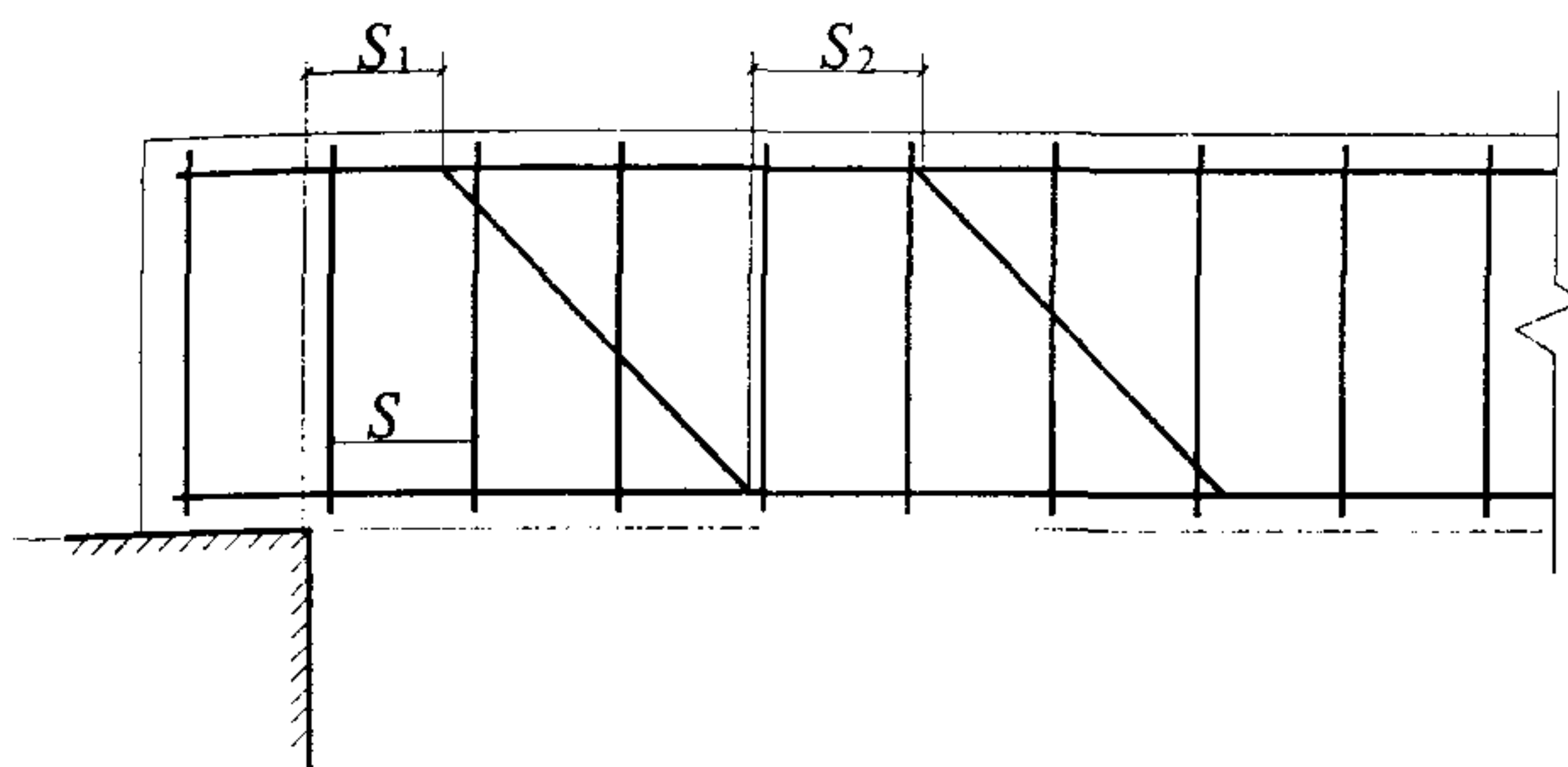
Черт.3.16. Расстояния между хомутами, опорой и отгибами
