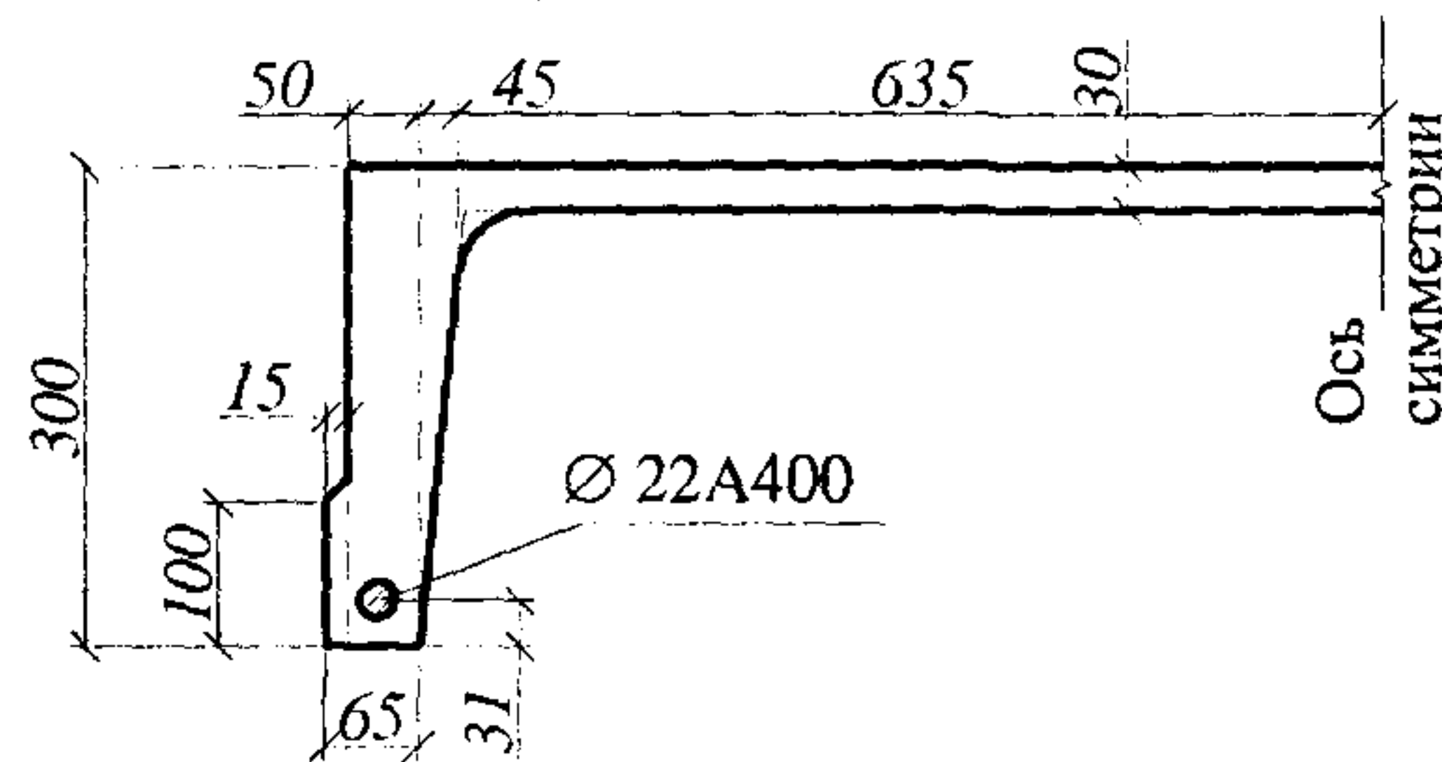
Черт.4.9. К примеру расчета 46
