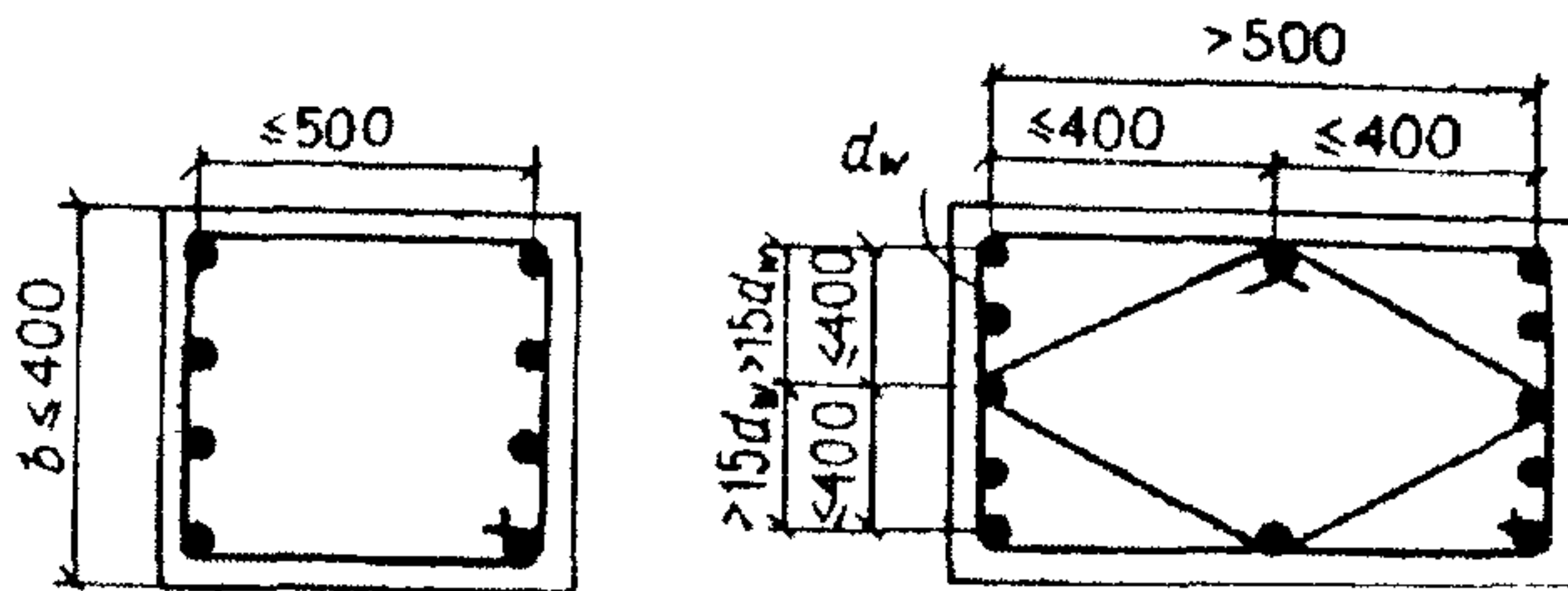
Черт.5.3. Конструкция пространственных арматурных каркасов в сжатых элементах
