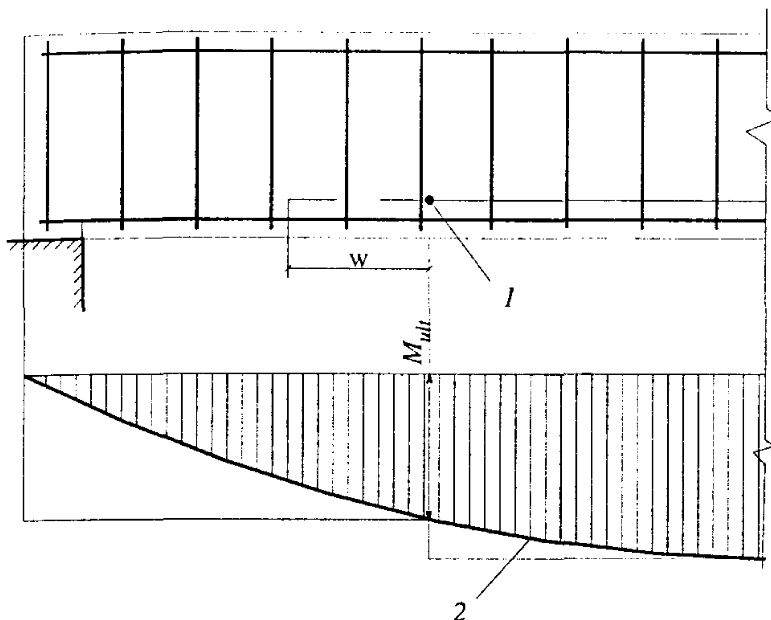
Черт.3.20. Обрыв растянутых стержней в пролете 1- точка теоретического обрыва; 2- эпюра M
