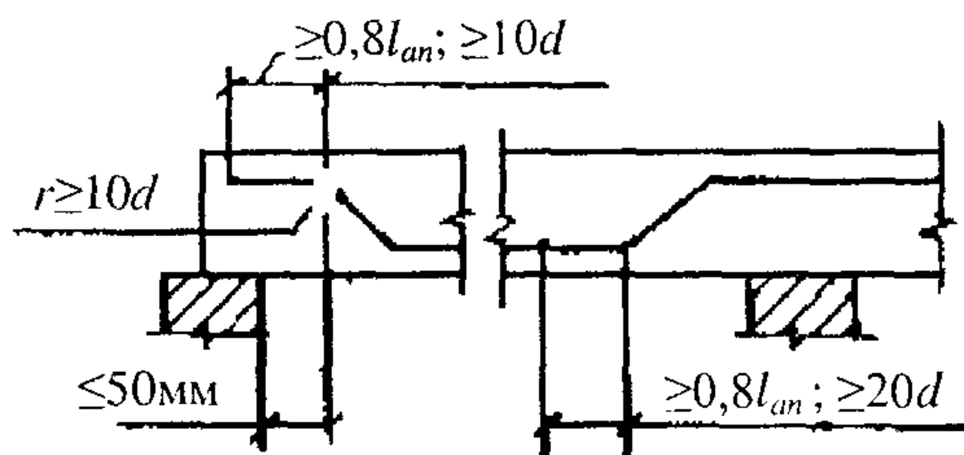
Черт.5.2. Конструкция отгибов арматуры
