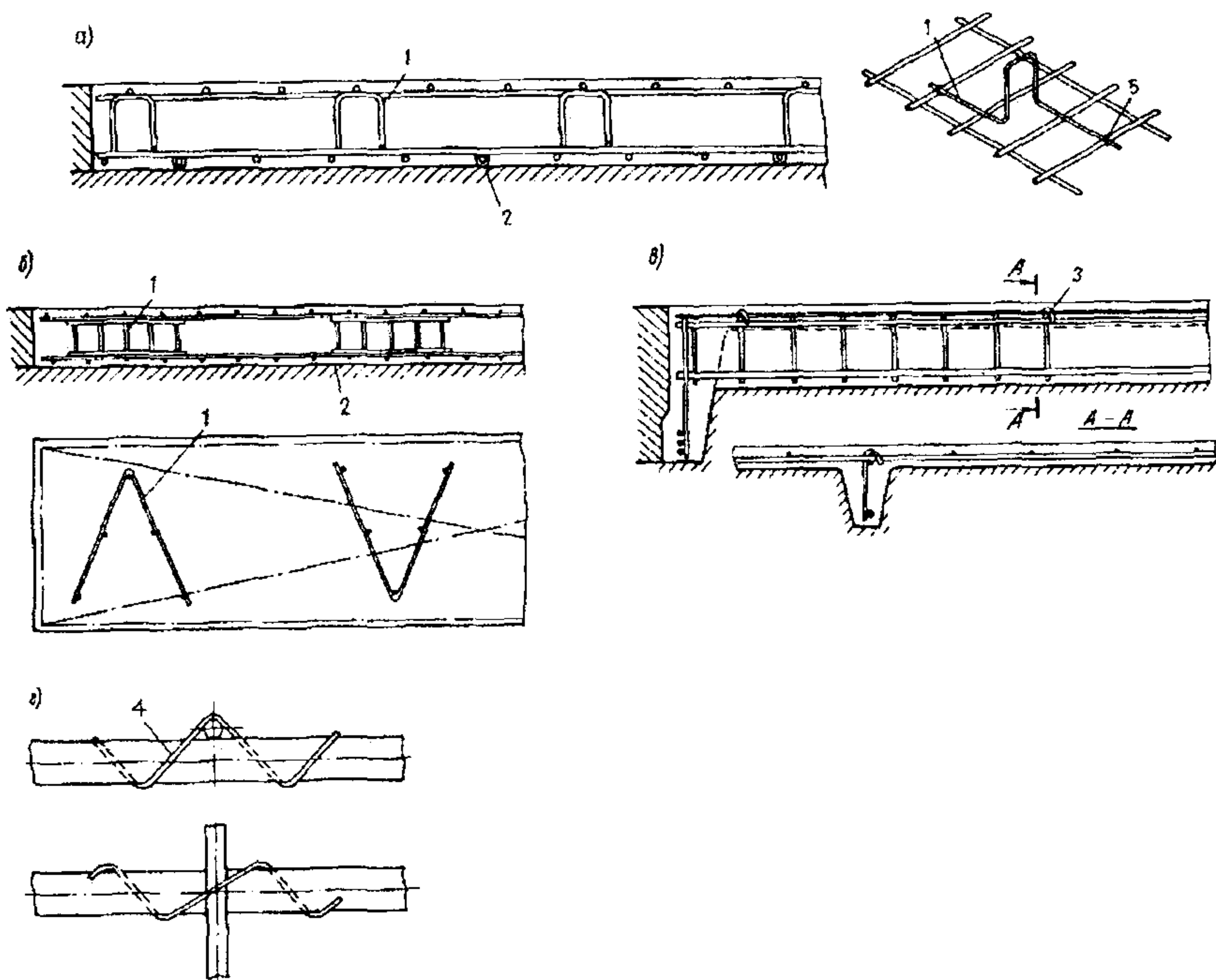
Черт.5.13. Фиксаторы однократного использования, обеспечивающие требуемое расстояние
