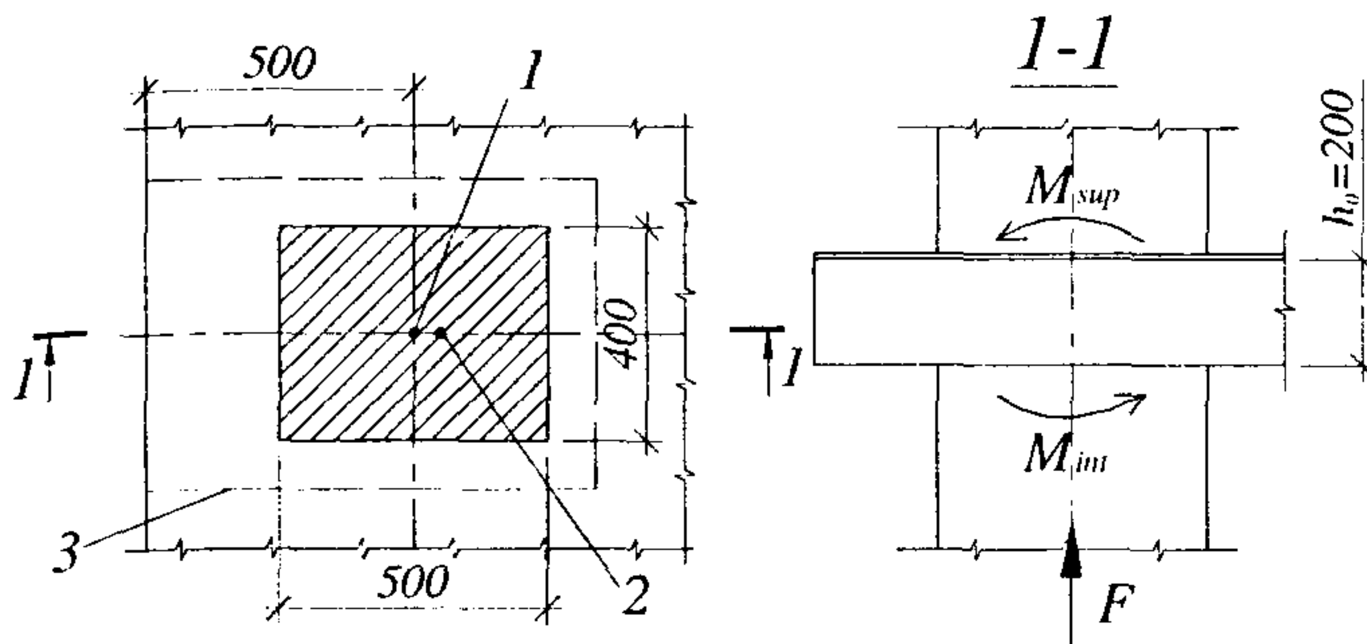
Черт.3.51. К примеру расчета 41
