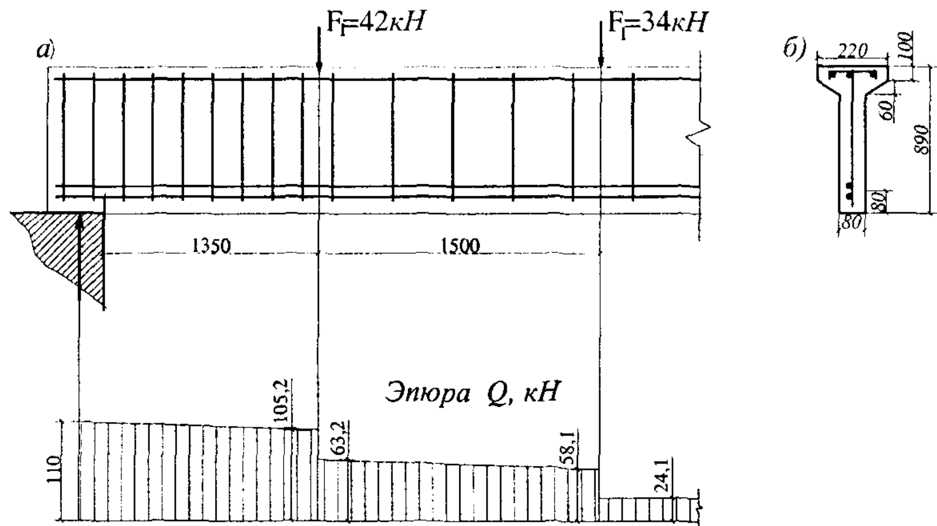
Черт.3.22. К примеру расчета 15
