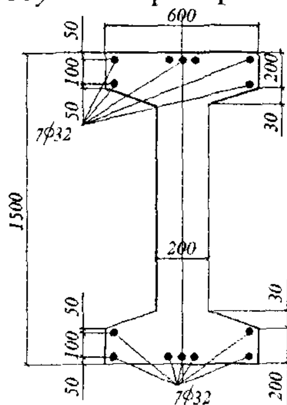
Черт.3.34. К примерам расчета 28 и 29
