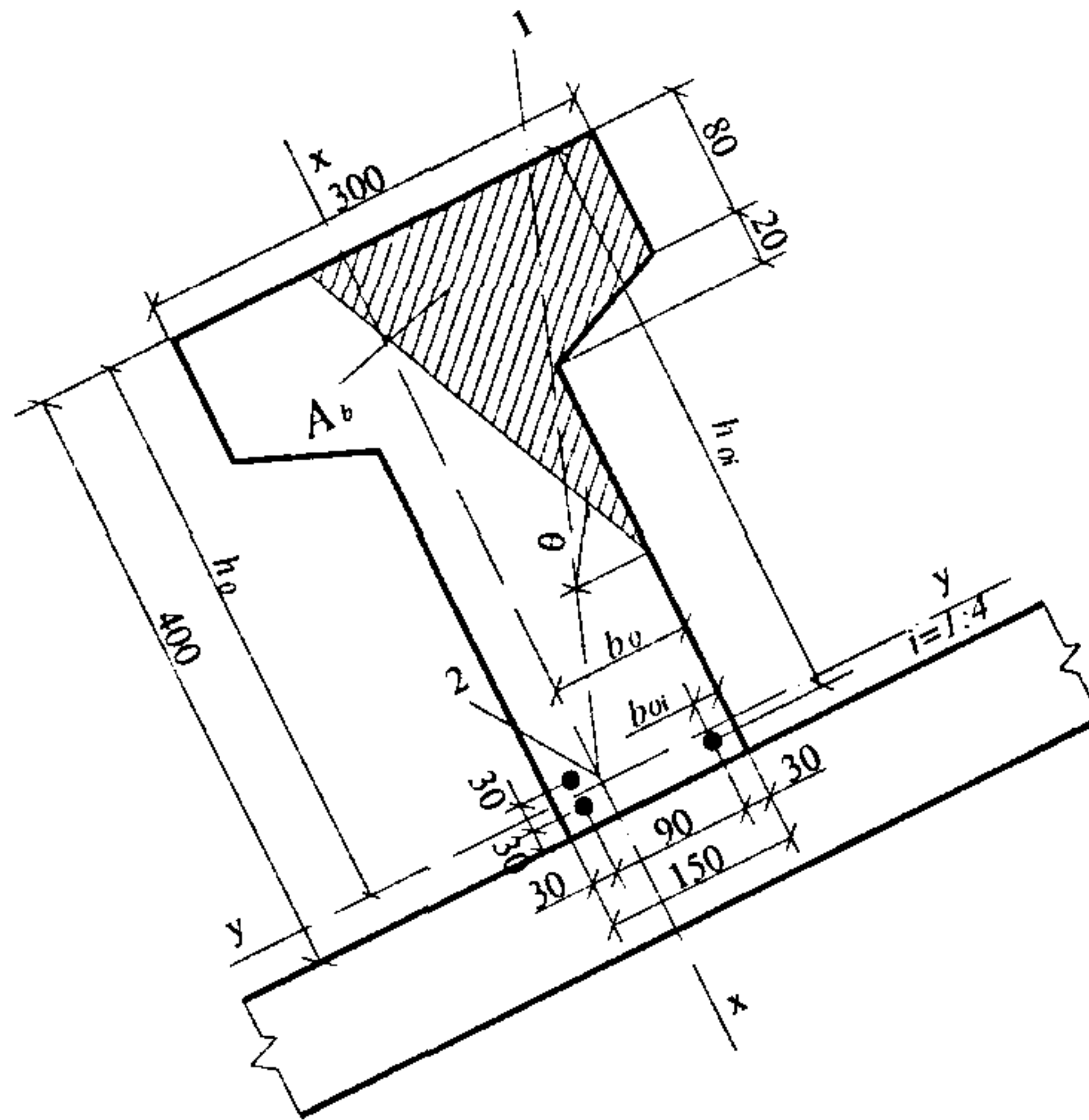
Черт.3.8 К примеру расчета 10
