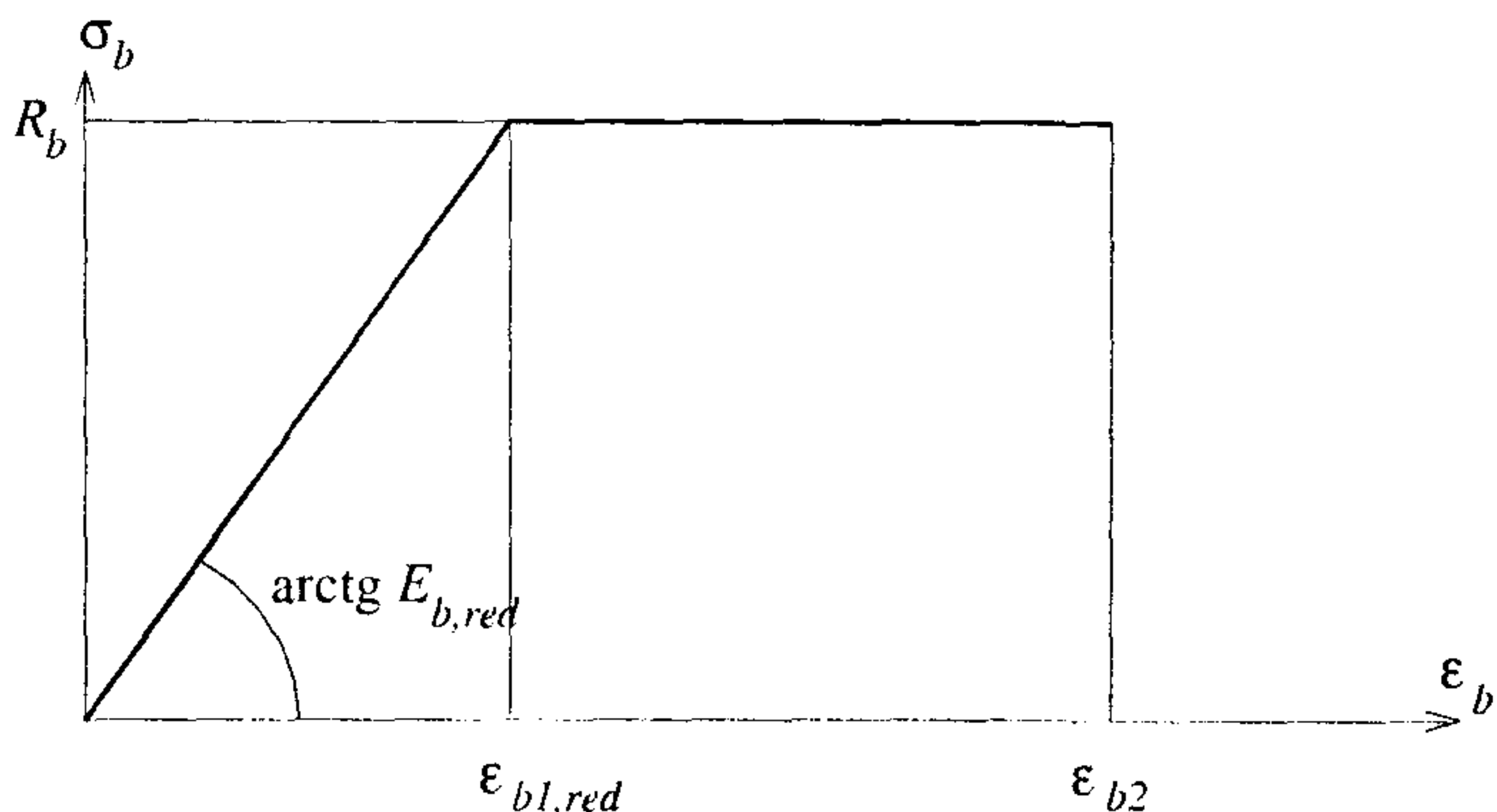
Черт.3.37. Двухлинейная диаграмма состояния сжатого бетона
