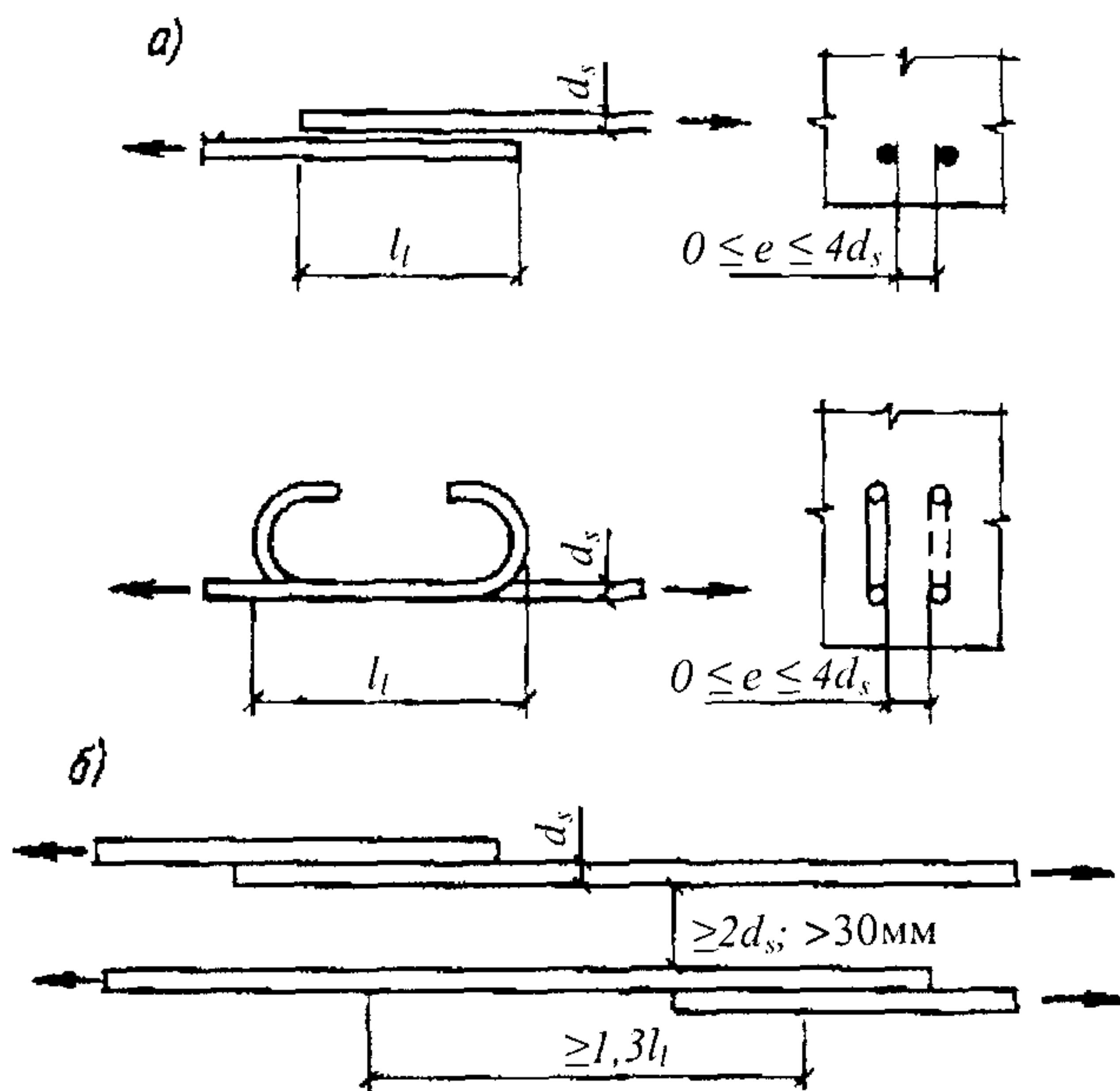
Черт.5.6 Расположение стержней, стыкуемых внахлестку, и самих стыков а – расположение стержней в стыке; б – расположение стыков
