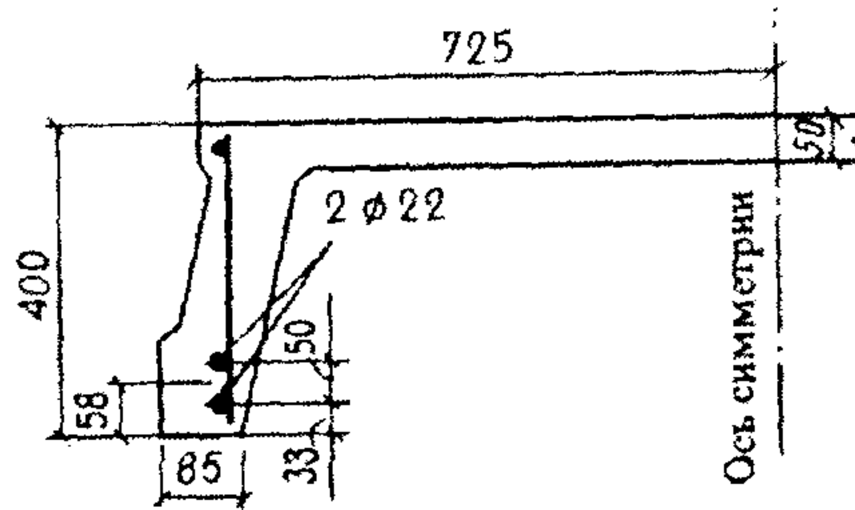
Черт.4.4. К примеру расчета 42
