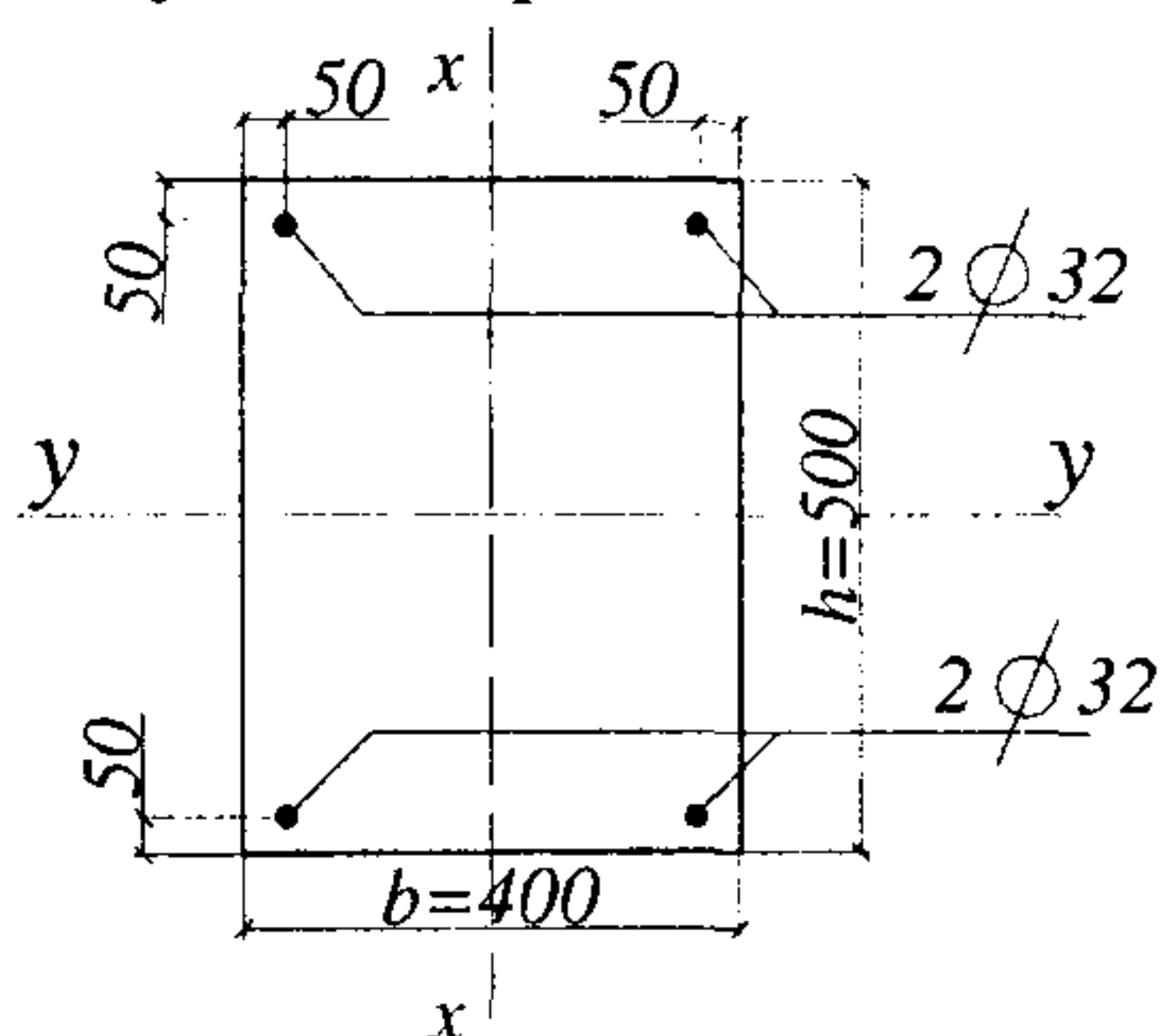
Черт.3.35. К примеру расчета 33
