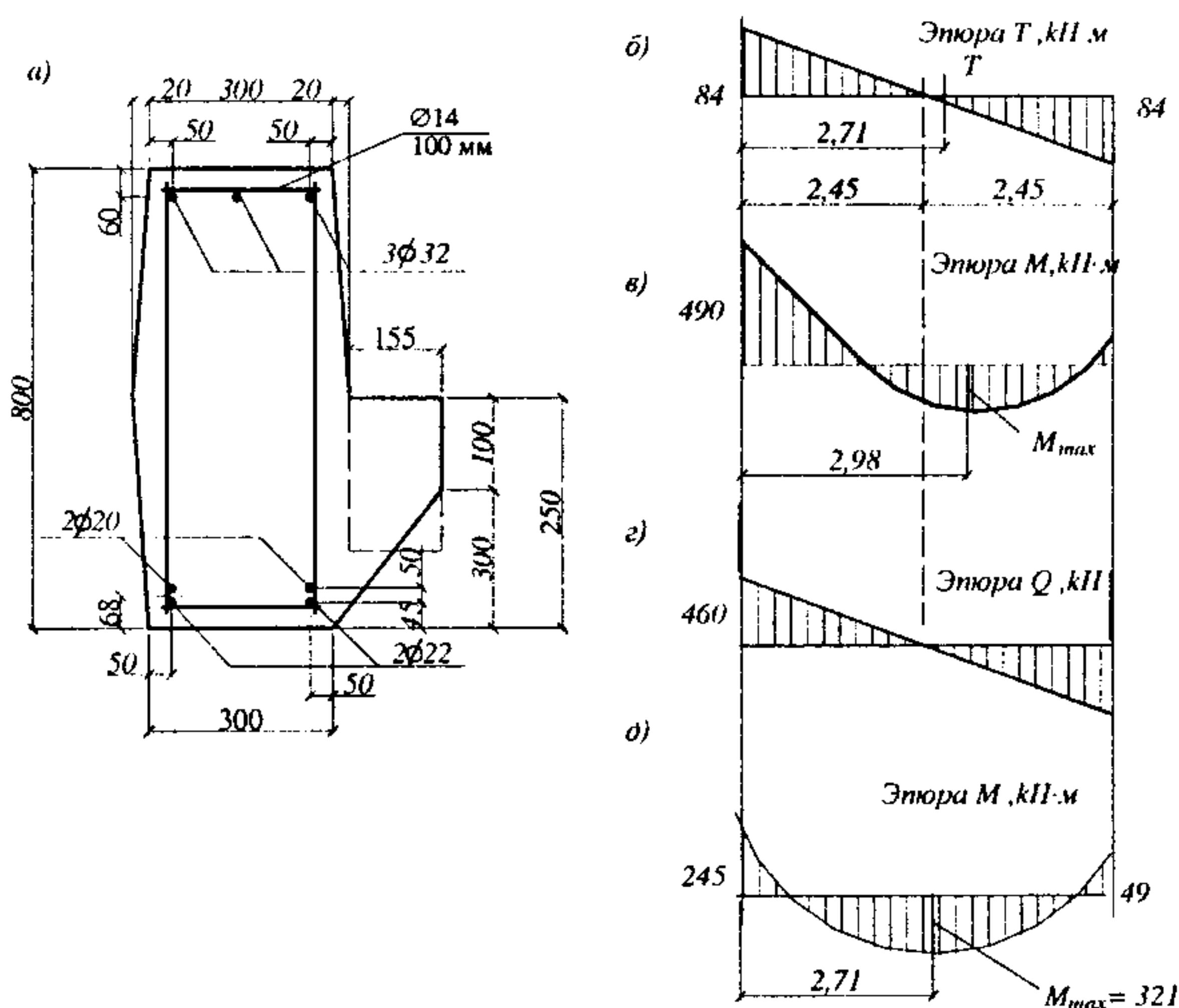
Черт.3.43. К примеру расчета 38
