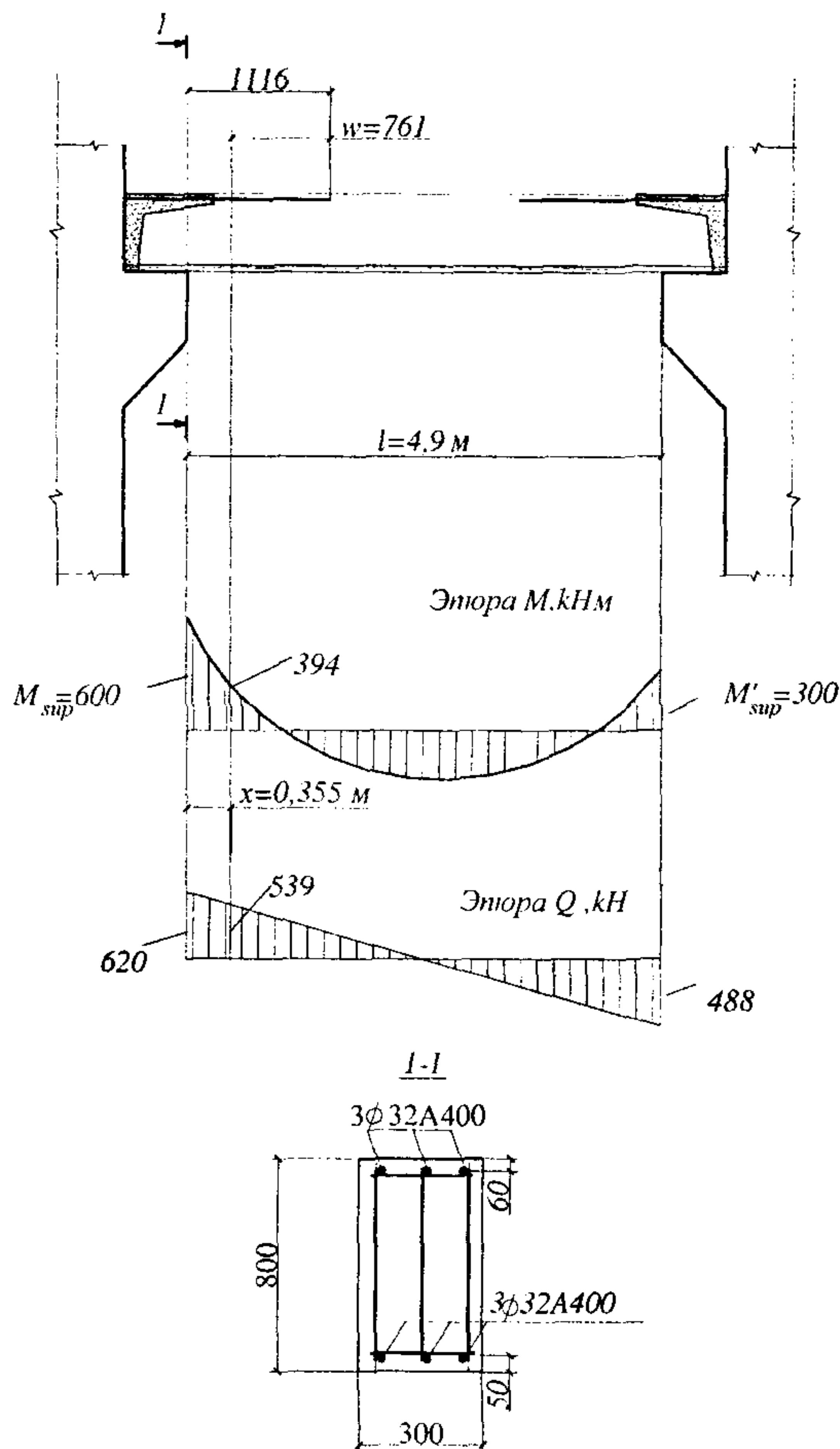
Черт.3.26. К примеру расчета 21
