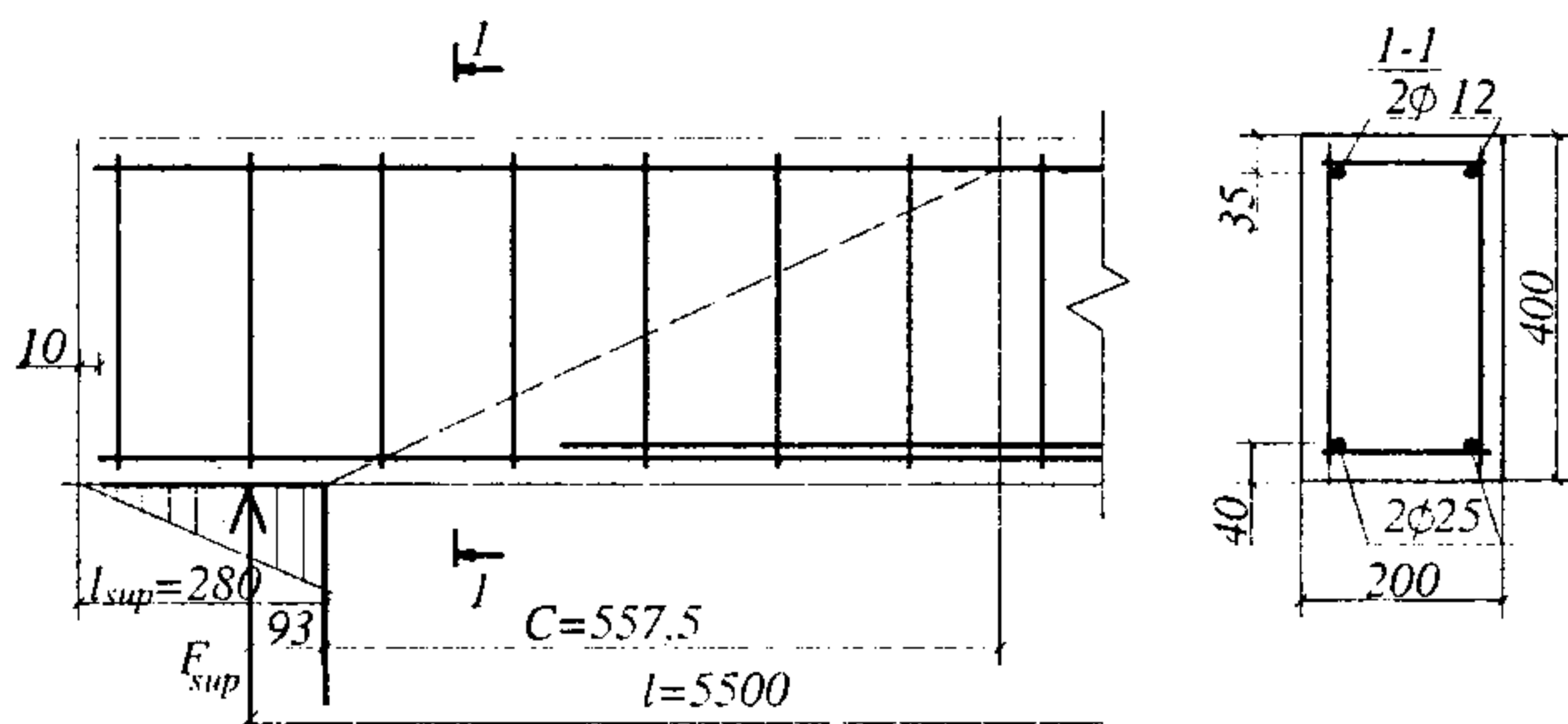
Черт.3.25. К примеру расчета 20
