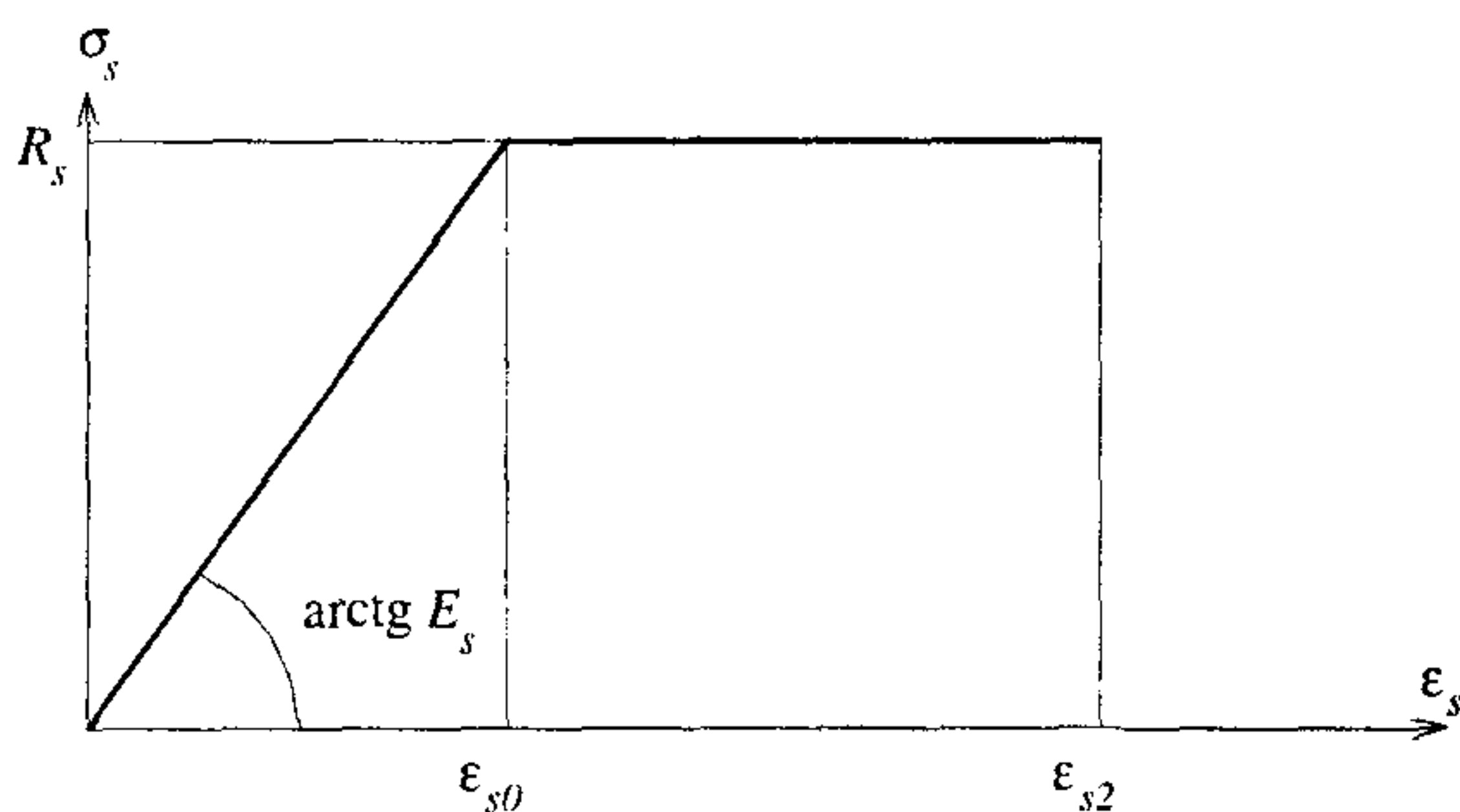
Черт.3.38. Диаграмма состояния растянутой арматуры
