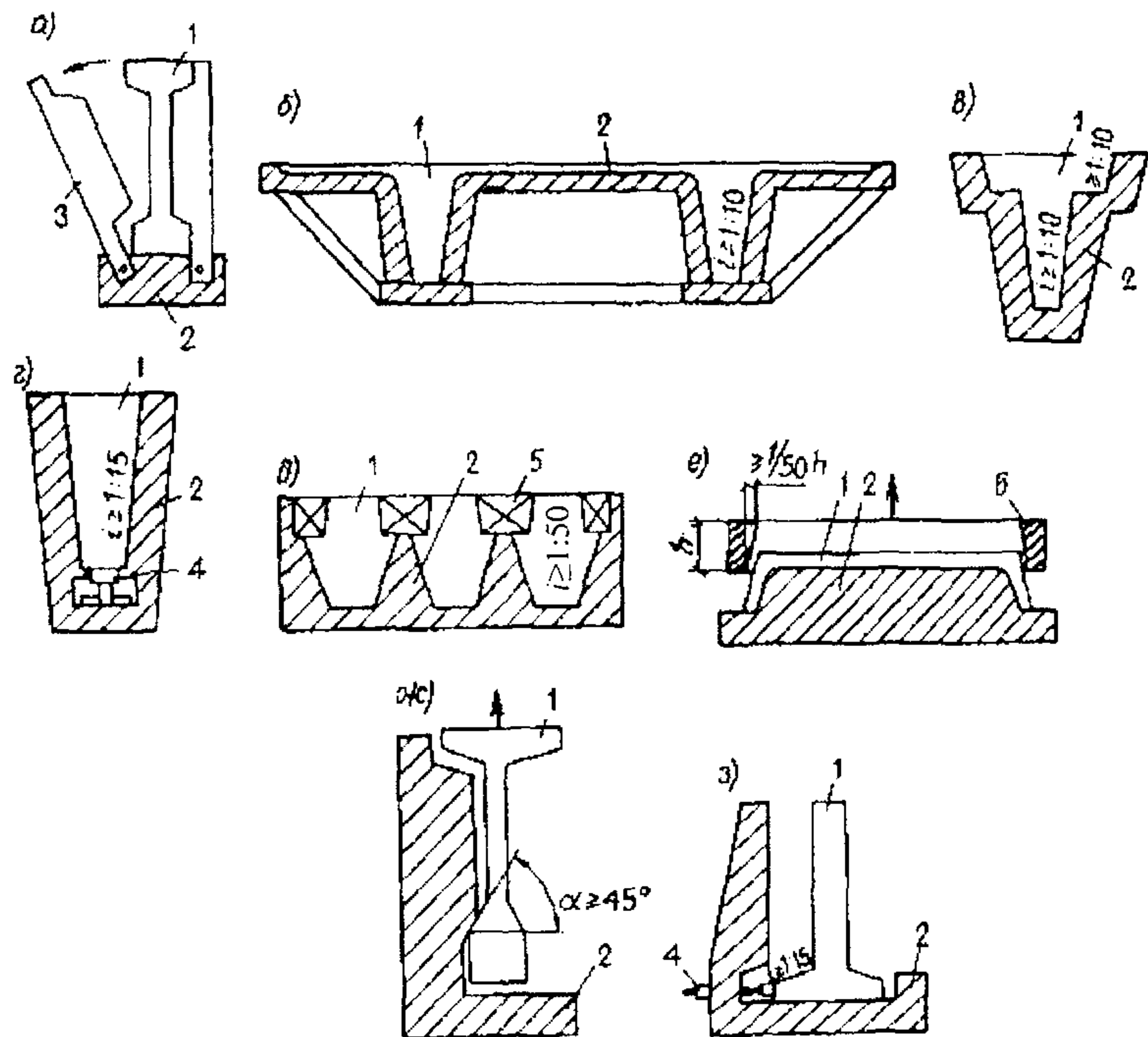
Черт.5.8. Технологические уклоны
