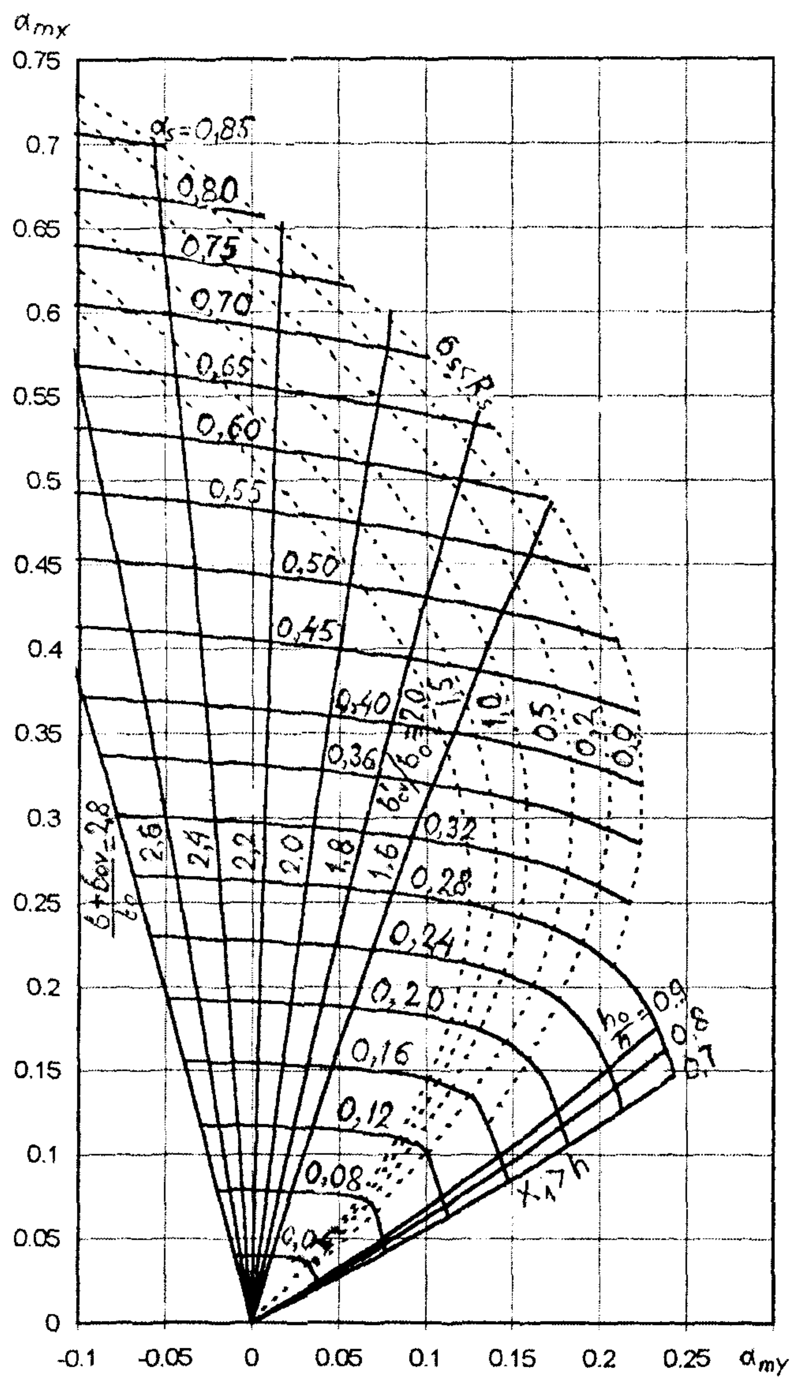
Черт.3.7. График несущей способности прямоугольного, таврового и Г-образного сечений для элементов, работающих на кривой изгиб
