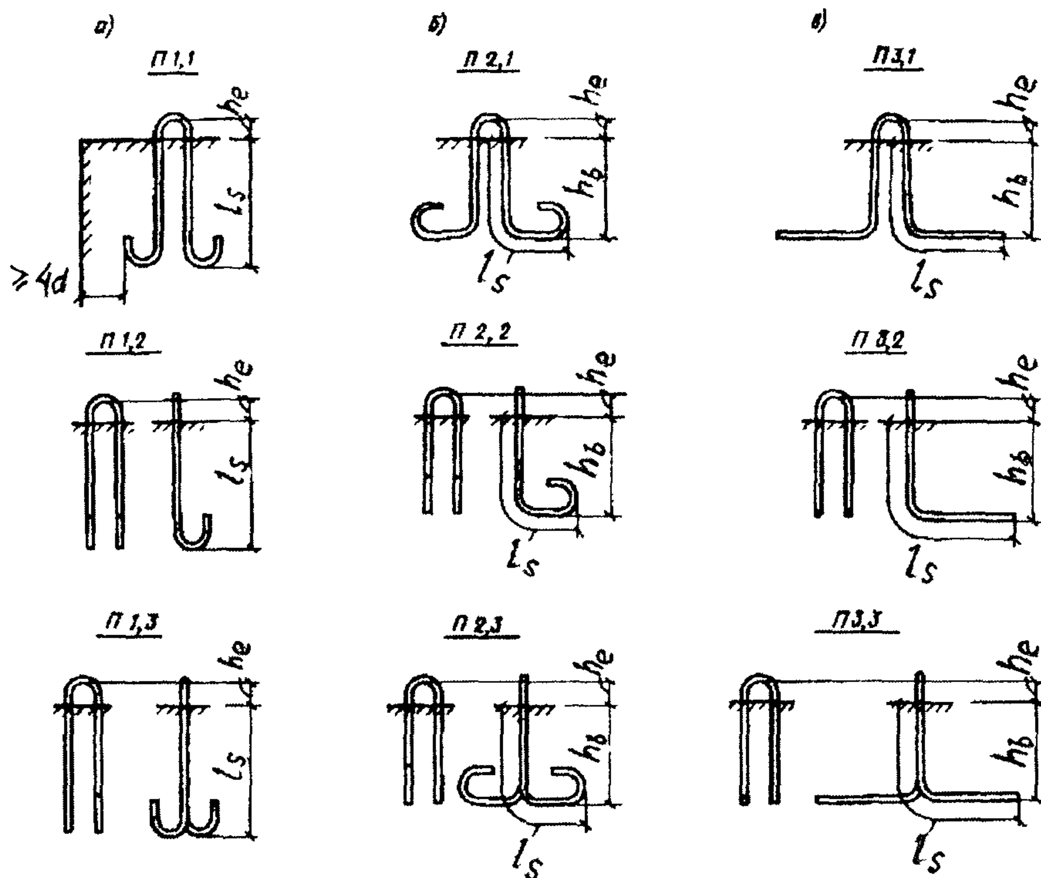
Черт.5.10. Типы строповочных петель
