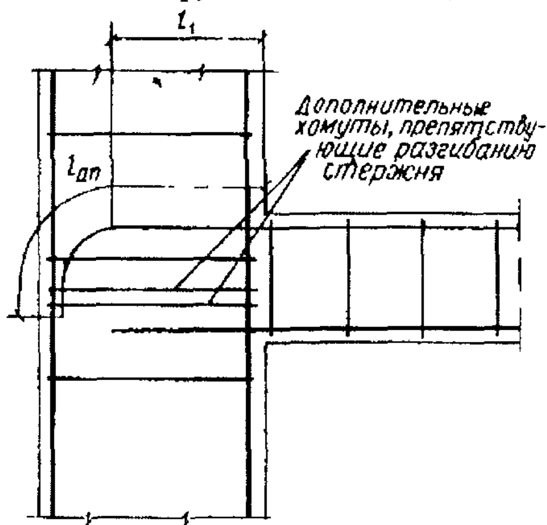
Черт.5.5. Анкеровка арматуры путем отгиба
