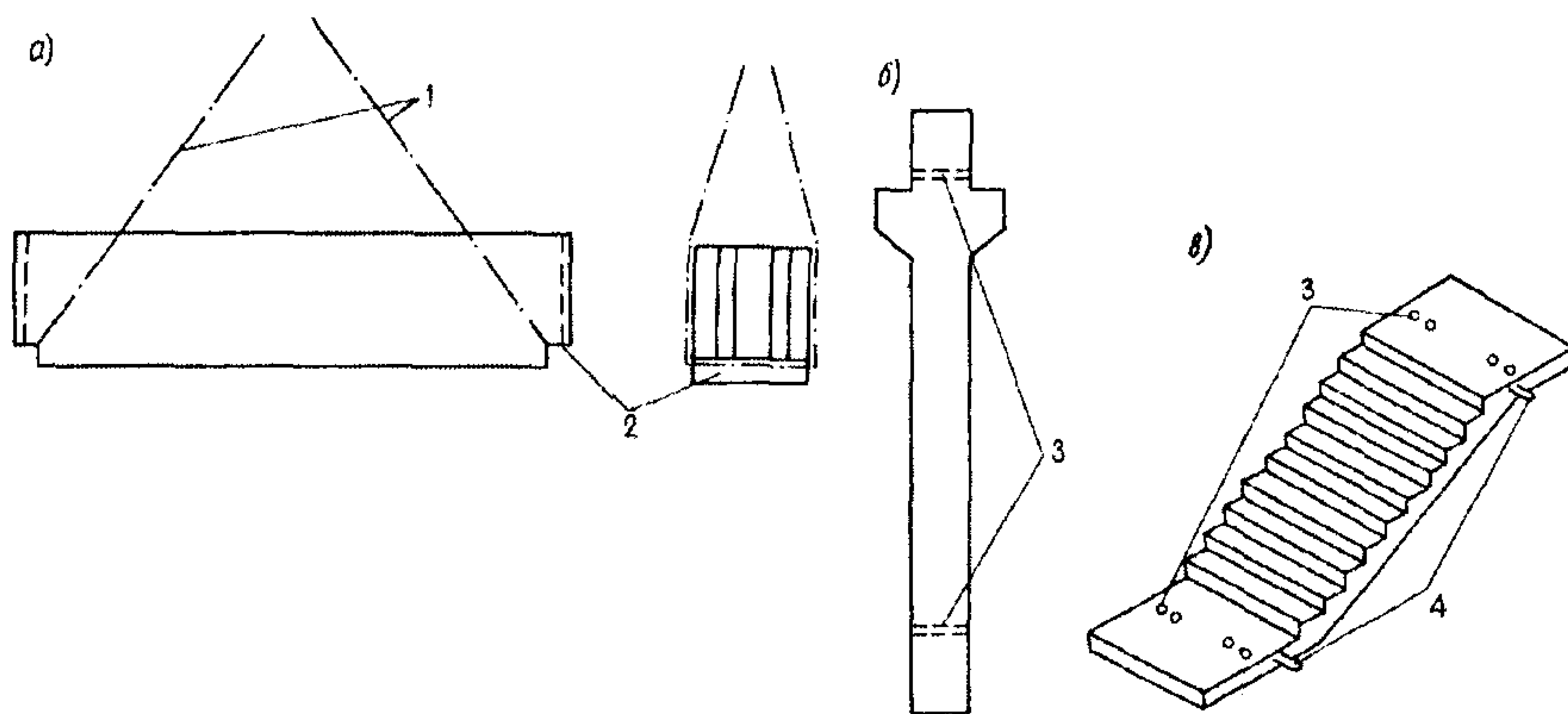
Черт.5.9. Примеры строповочных устройств без петель
