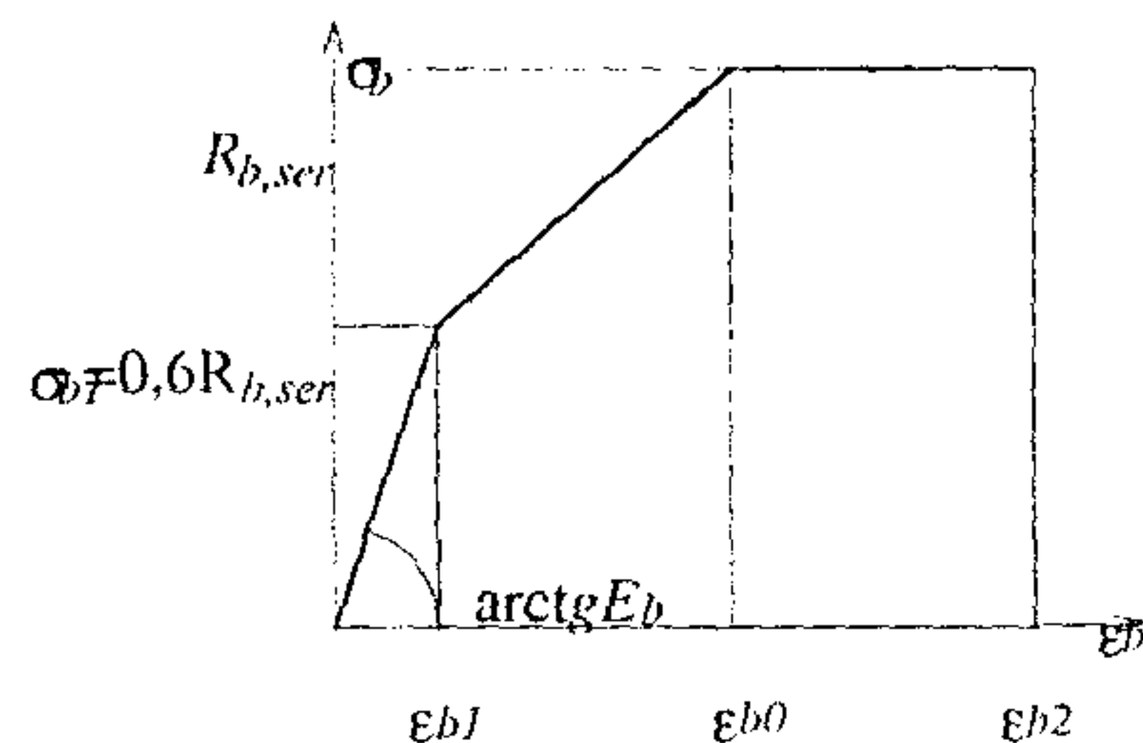
Черт.4.8.Трехлинейная диаграмма состояния сжатого бетона
