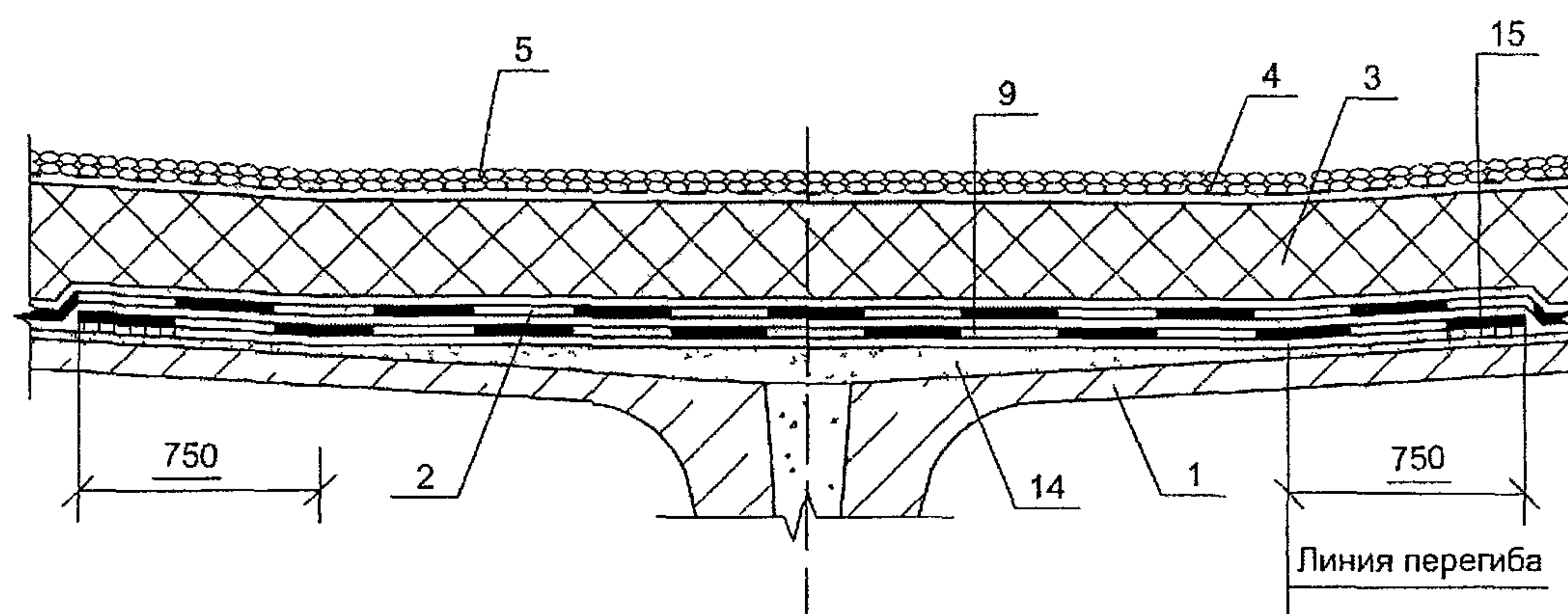
Рис. 1 14 Инверсионная кровля
