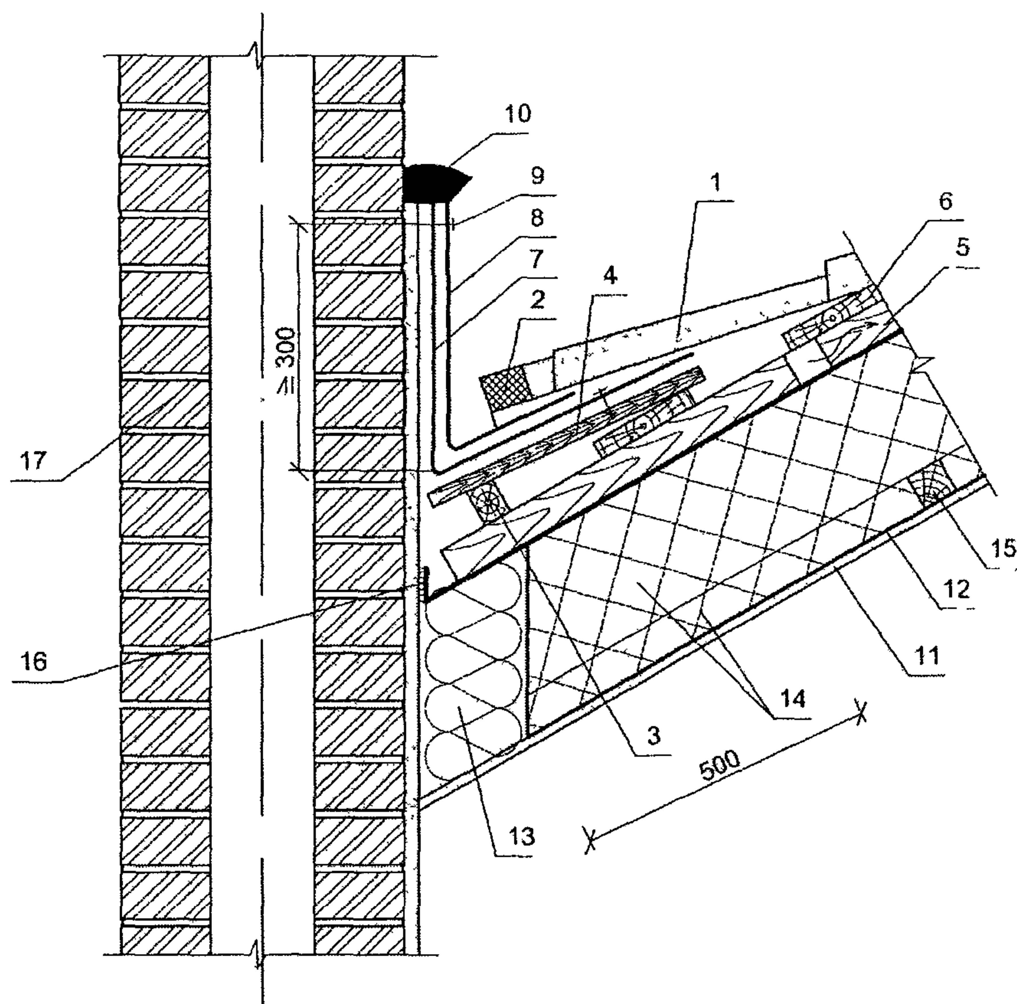
Рис. 1.43. Примыкание кровли к кирпичной трубе
