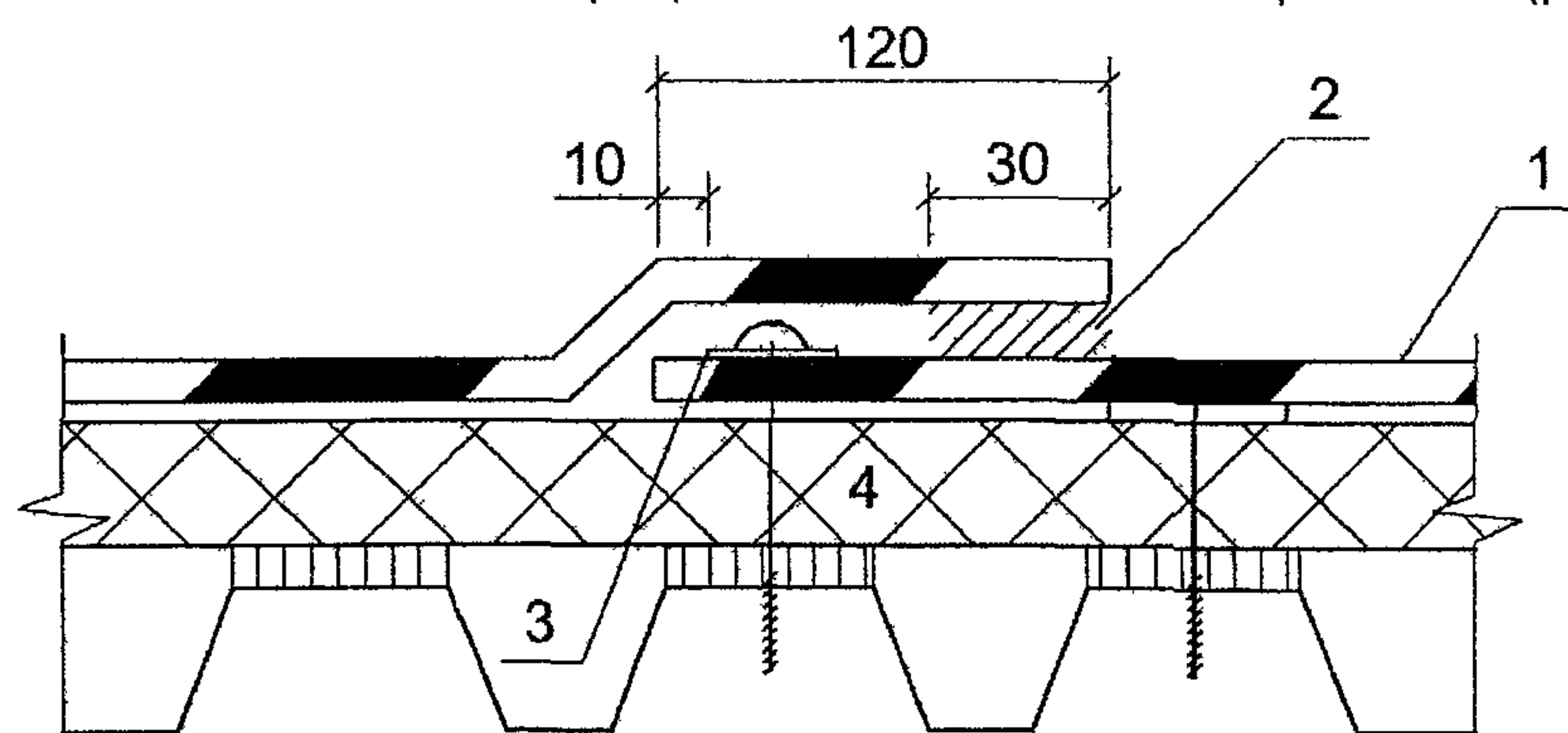
Рис. 2.11. Стык смежных полотнищ термопластичной пленки
