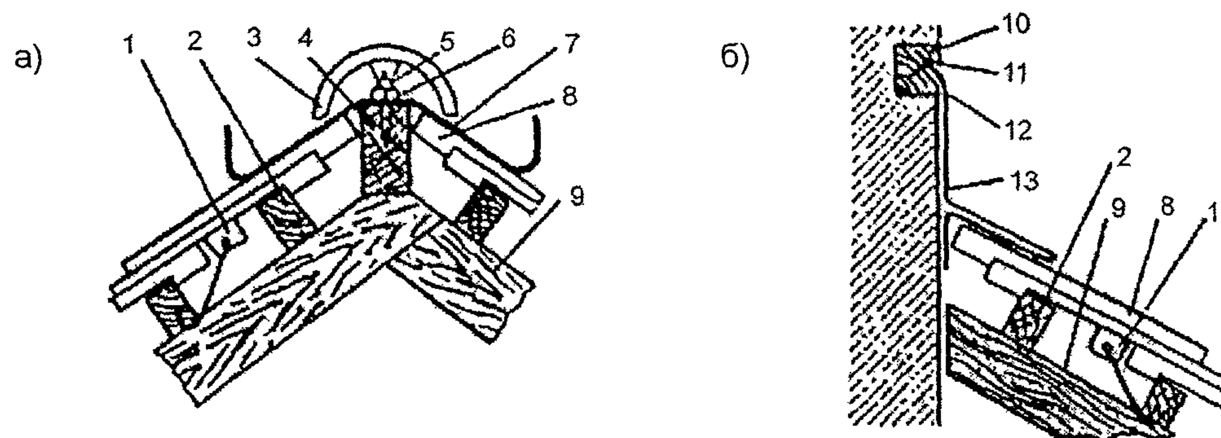
Рис. 2.34. Кровля из ленточной черепицы
