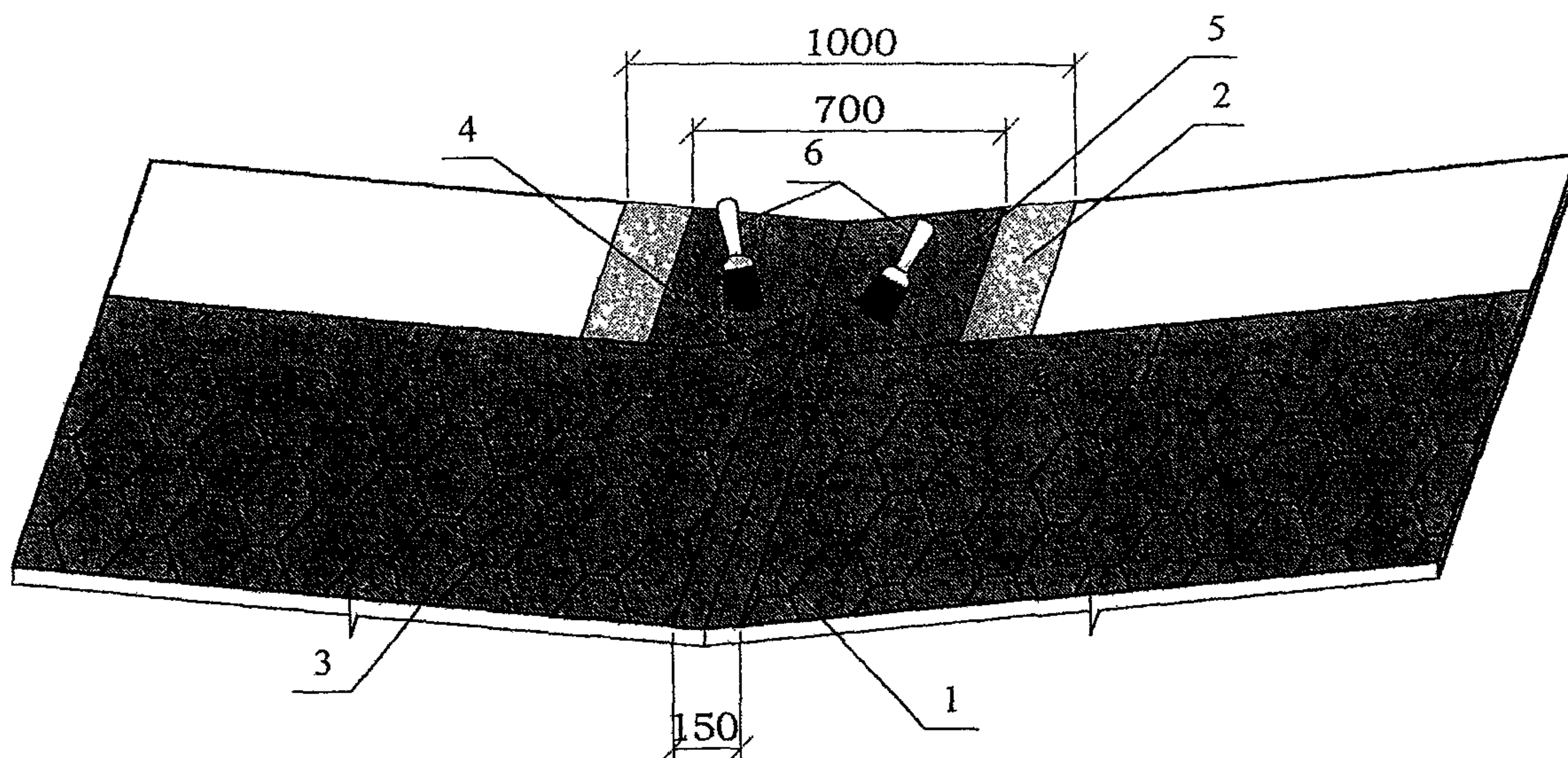
Рис. 2.40. Укладка гибкой черепицы в ендове 1 – специальный (ендовый) материал; 2 – подкладочный слой; 3 – рядовая черепица; 4 – линия обрезки черепицы; 5 – гвозди с шагом 100 мм; 6 – нанесение мастики.
