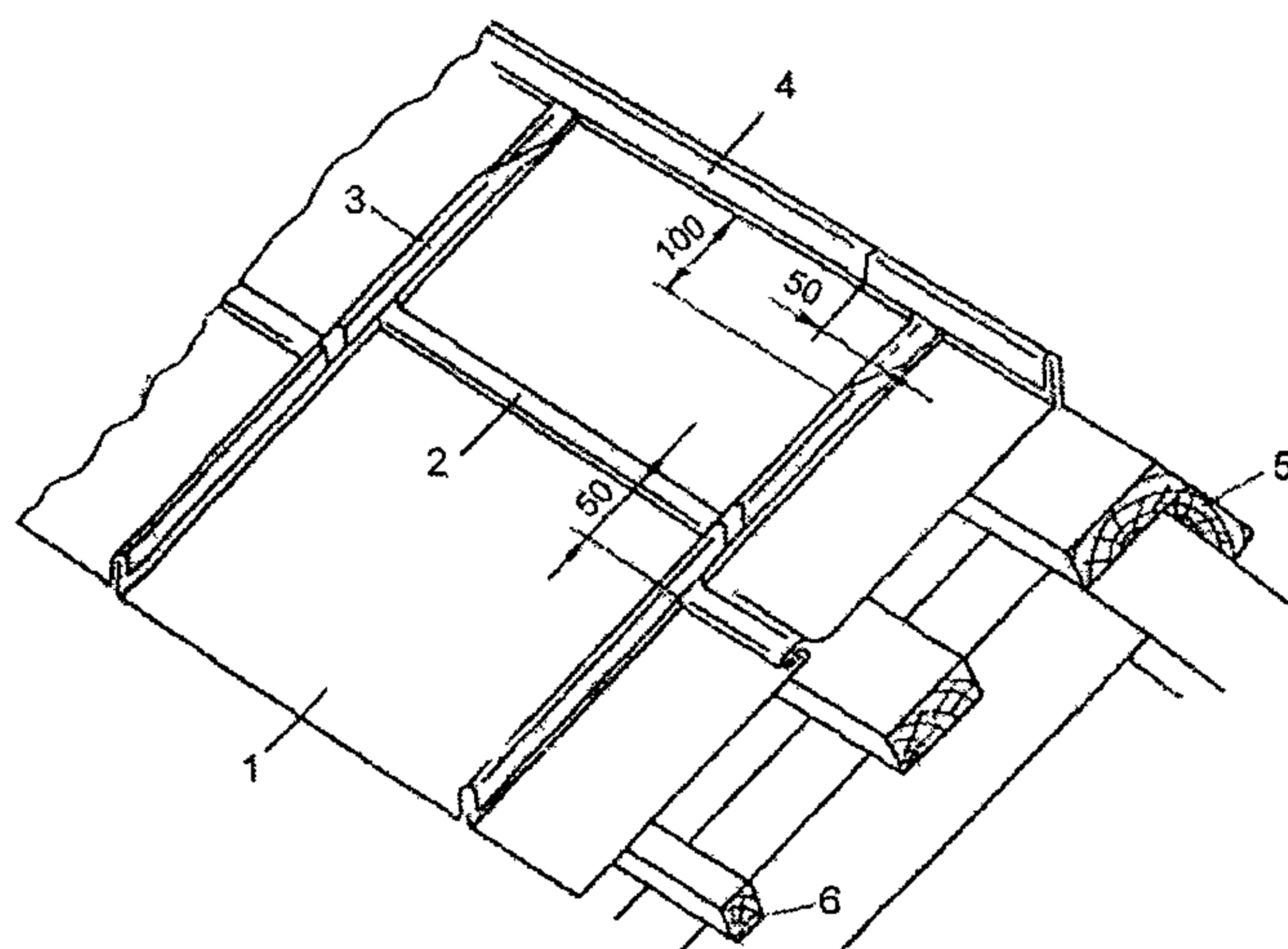
Рис. 2.49 Рядовое покрытие ската листовой сталью (медью) 1 — картина в рядовой полосе, 2 — одинарный лежащий фальц, 3 — одинарный стоячий фальц, 4 — коньковый стоячий фальц, 5 — доска, 6 — брус обрешетки
