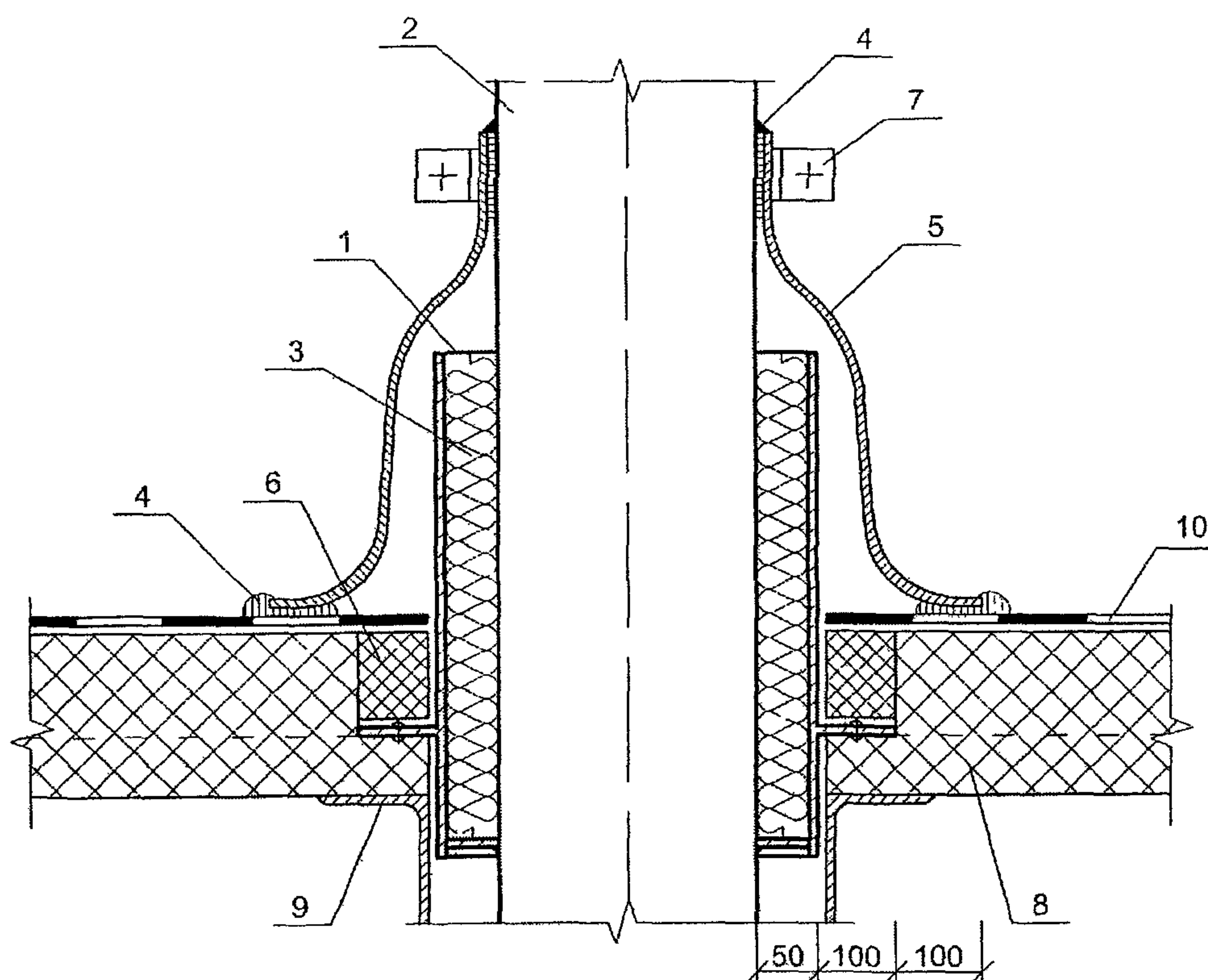
Рис. 1.8 Примыкание кровли к трубе
