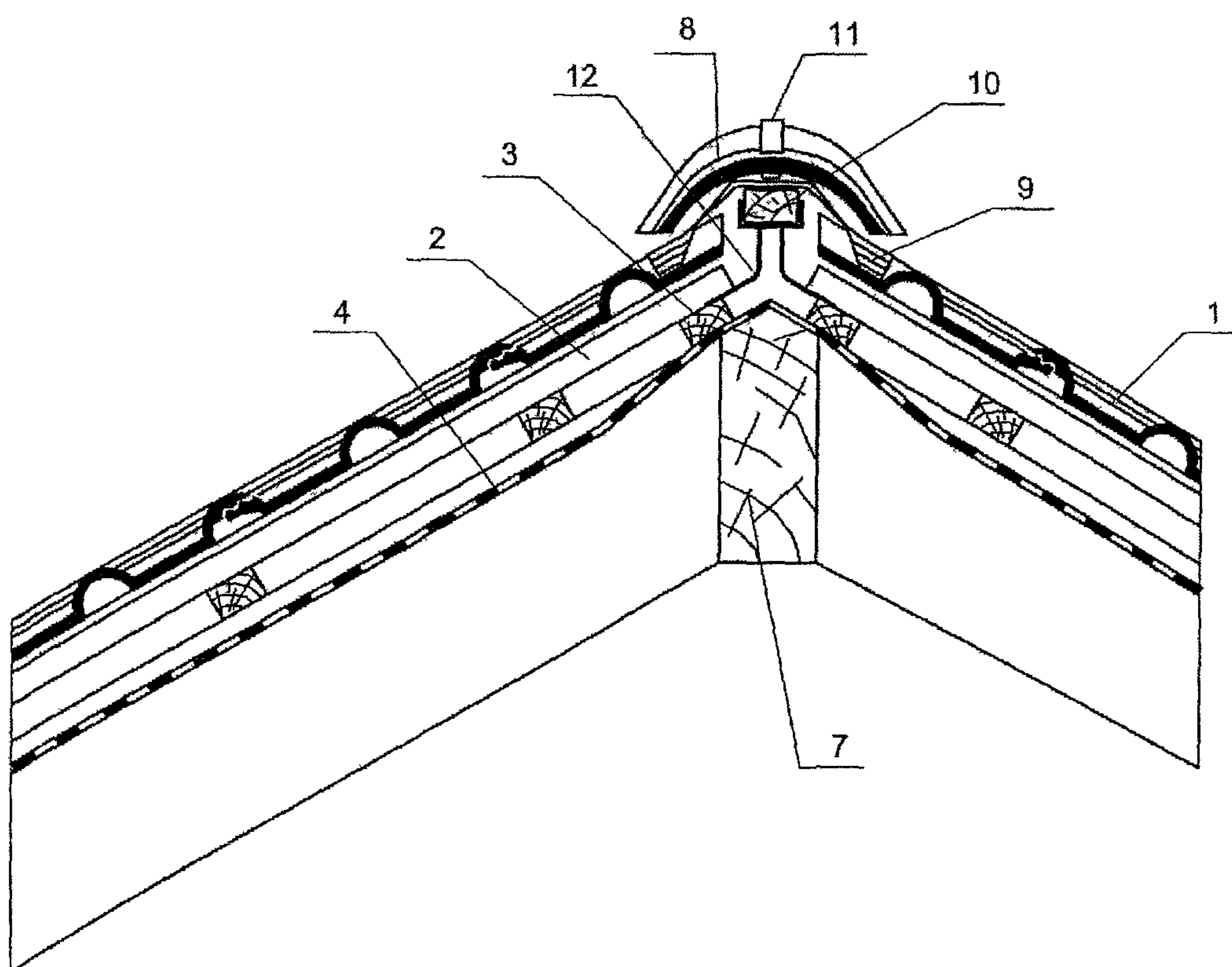
Рис. 1.28. Хребет крыши (а) и чердачной кровли (б)
