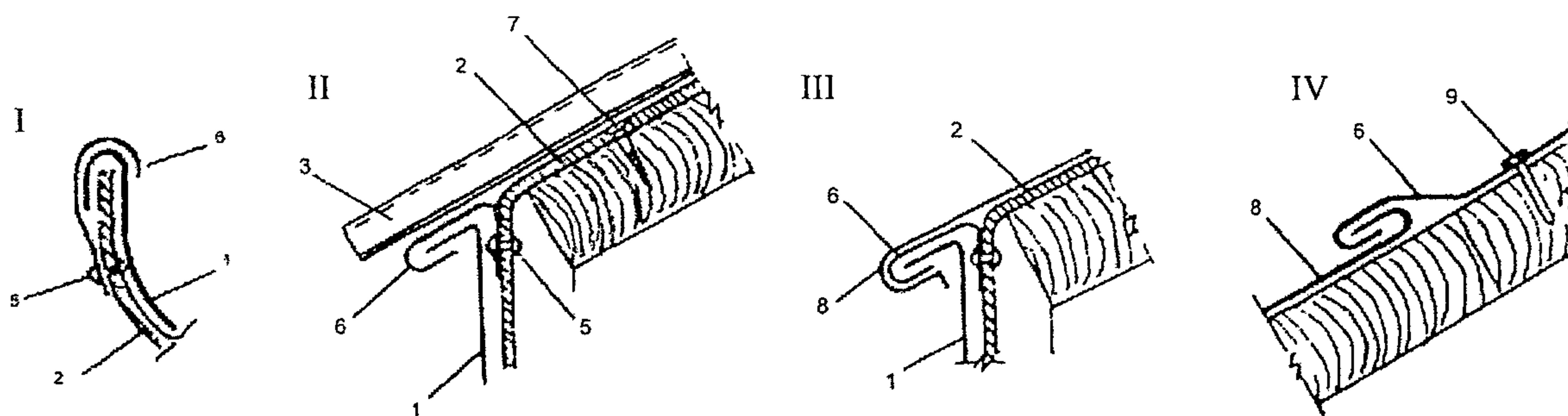
Рис. 1.63. Подвесной желоб (лоток)
