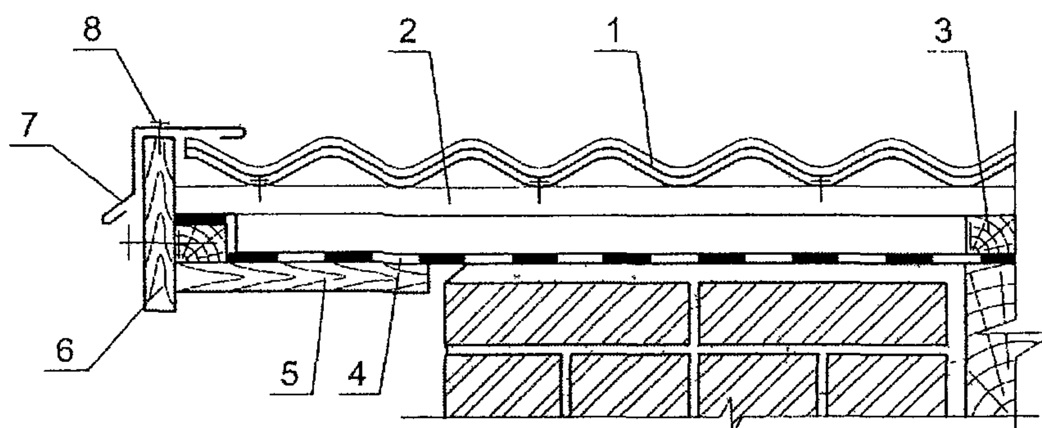
Рис. 1.41. Фронтонный свес кровли
