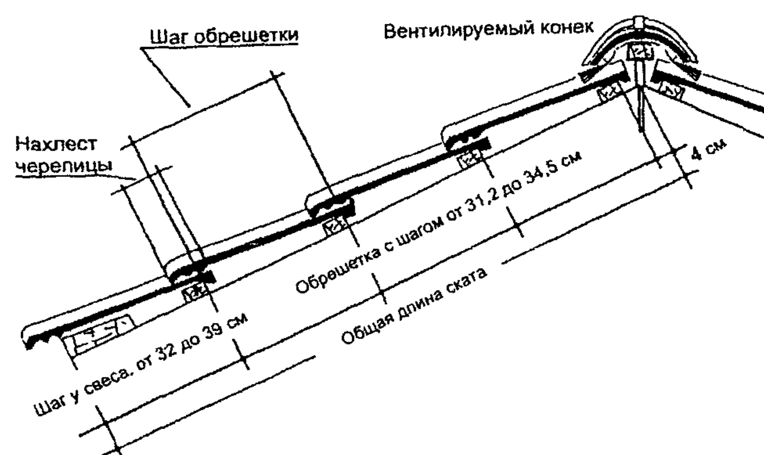
Рис. 1.15. Поперечный разрез черепичной кровли
