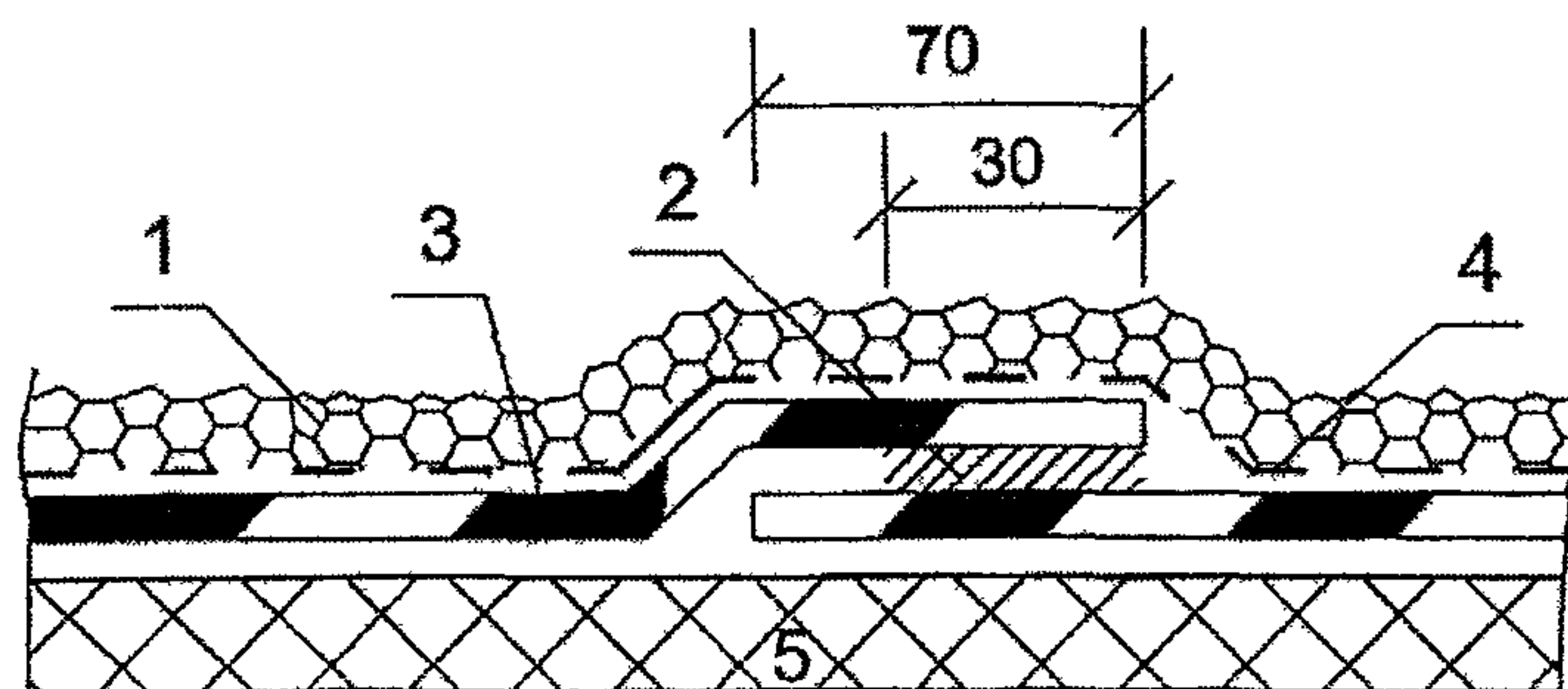
Рис. 2.10. Стык смежных полотенц термопластичной пленки
