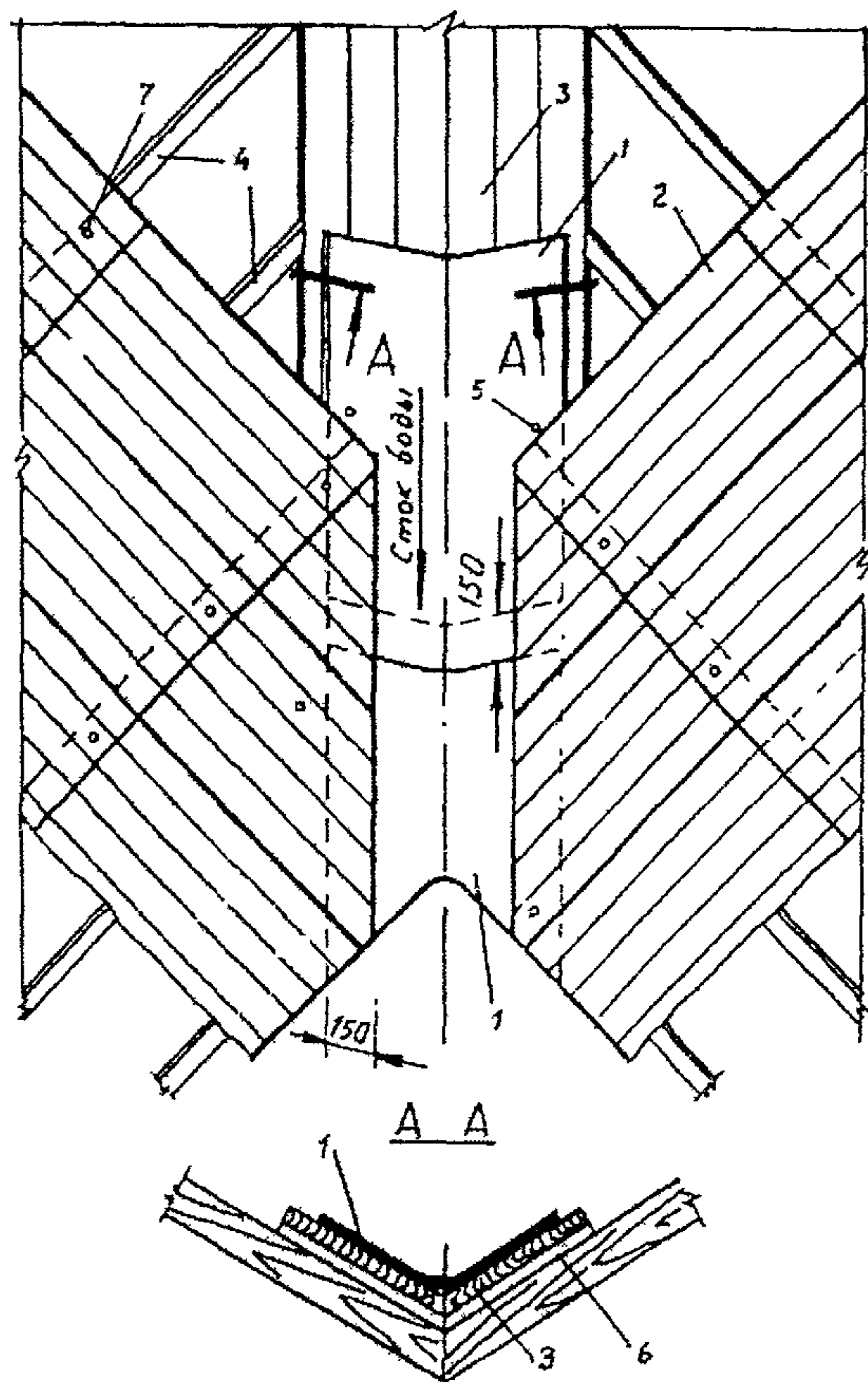
Рис. 1.45. Ендова (разжелобок)
