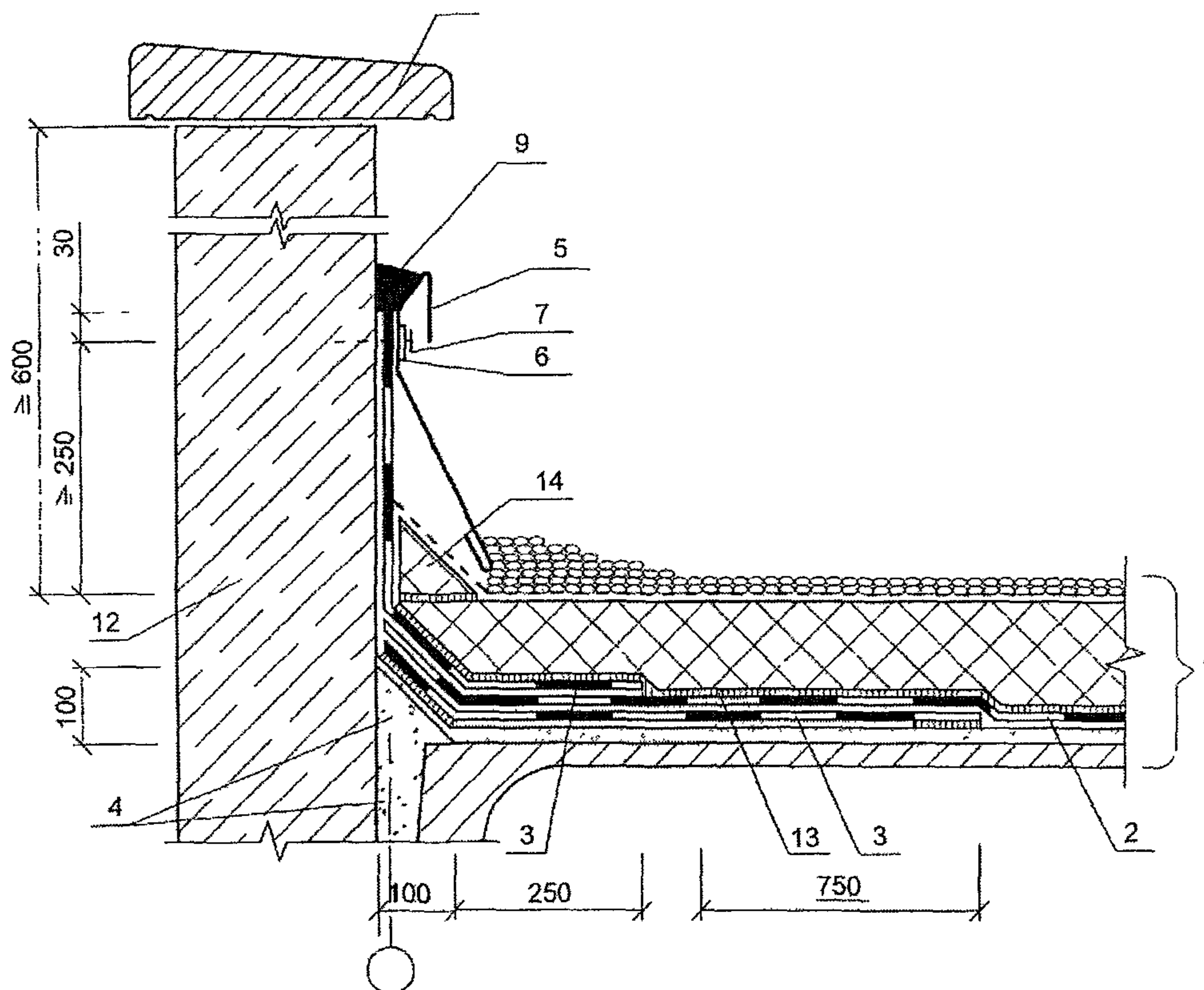
Рис 1 13 Примыкание инверсионной кровли к парапету
