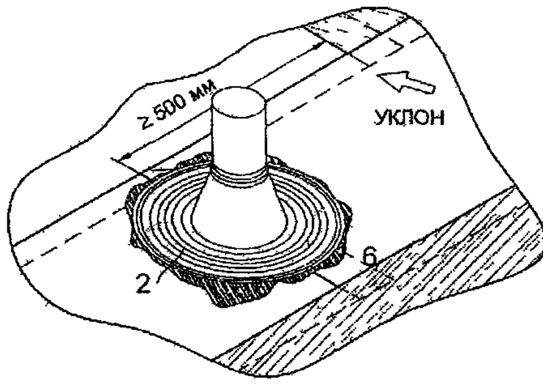
Рис 2 24 Приклейка фасонного элемента к поверхности нижнего слоя основного водоизоляционного ковра
