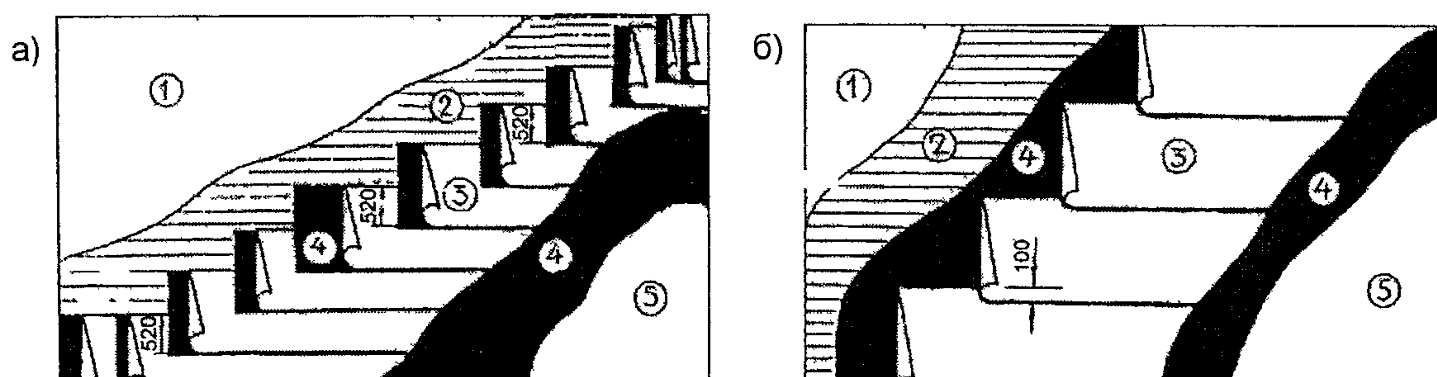
Рис 2 13 Схема расположения слоев мастичного кровельного ковра
