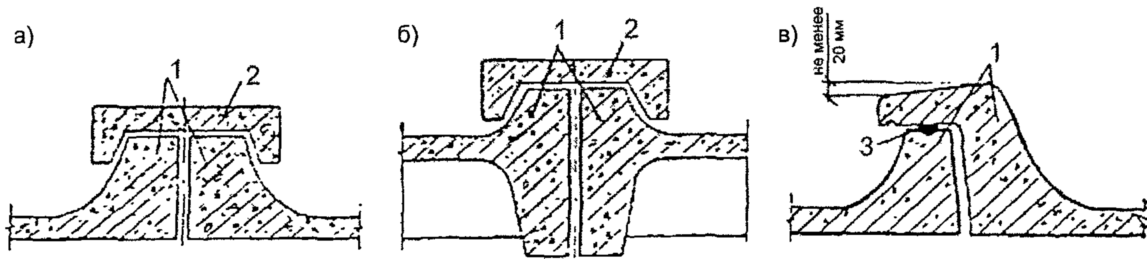
Рис. 1.66. Конструкции стыков кровельных панелей
