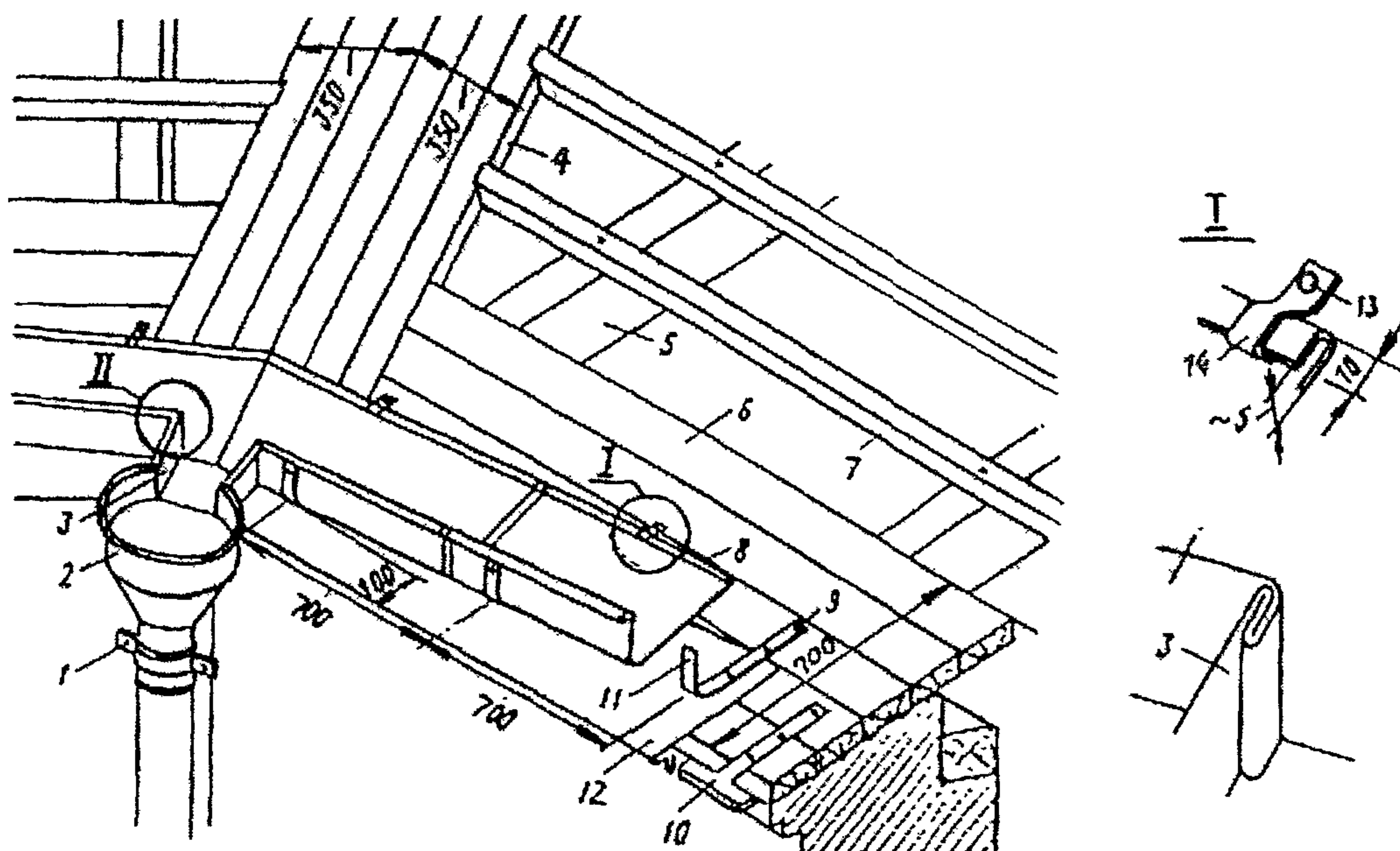
Рис. 2.51. Устройство настенного желоба
