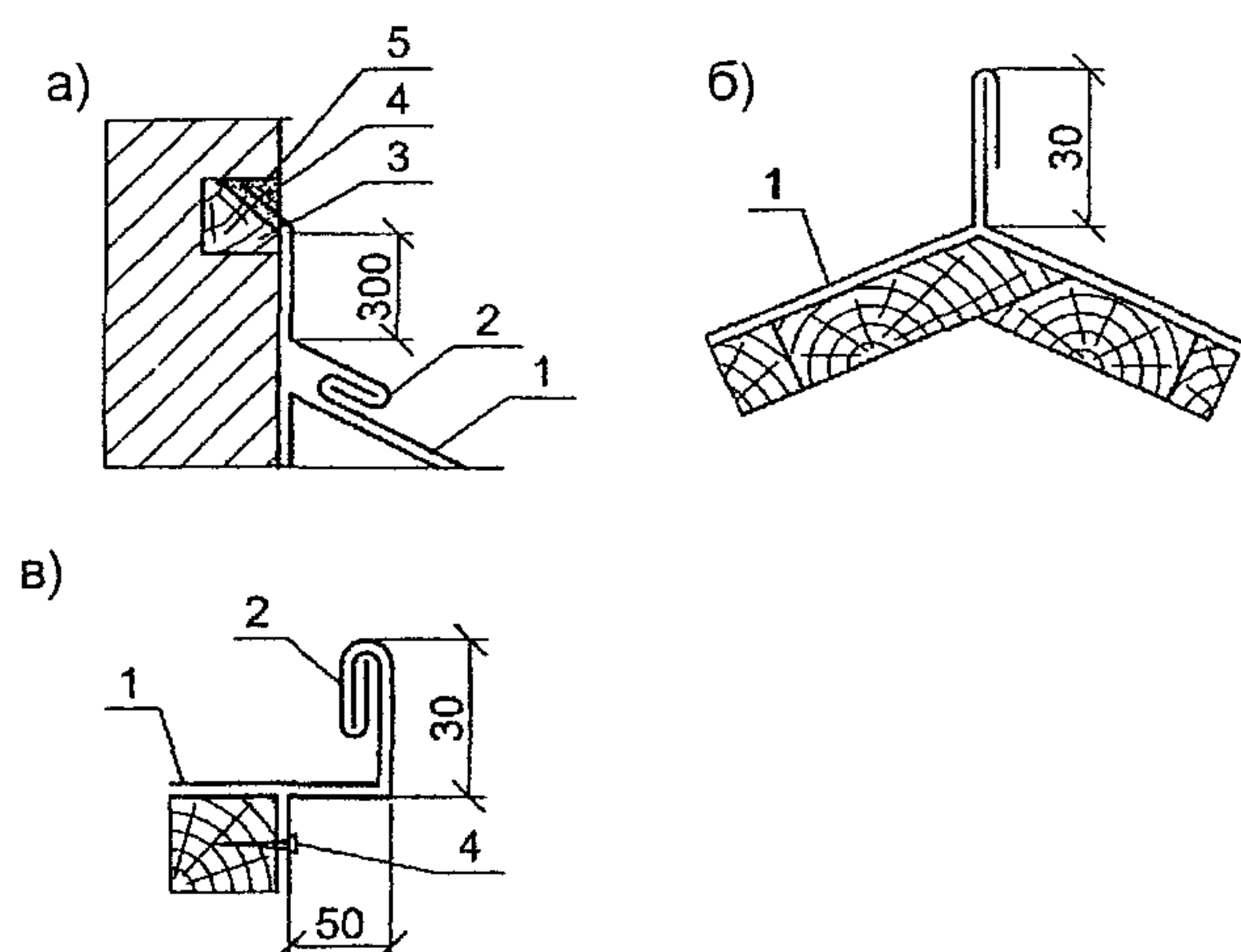
Рис. 1.61 Примыкание кровли из листовой стали к стене (а), коньковый стоячий фальц (б) и крепление фронтового края рядовой полосы (в) 1 – картина в рядовой полосе кровли; 2 – фартук из оцинкованной кровельной стали; 3 – деревянный брусок; 4 – кровельный гвоздь; 5 – герметик.
