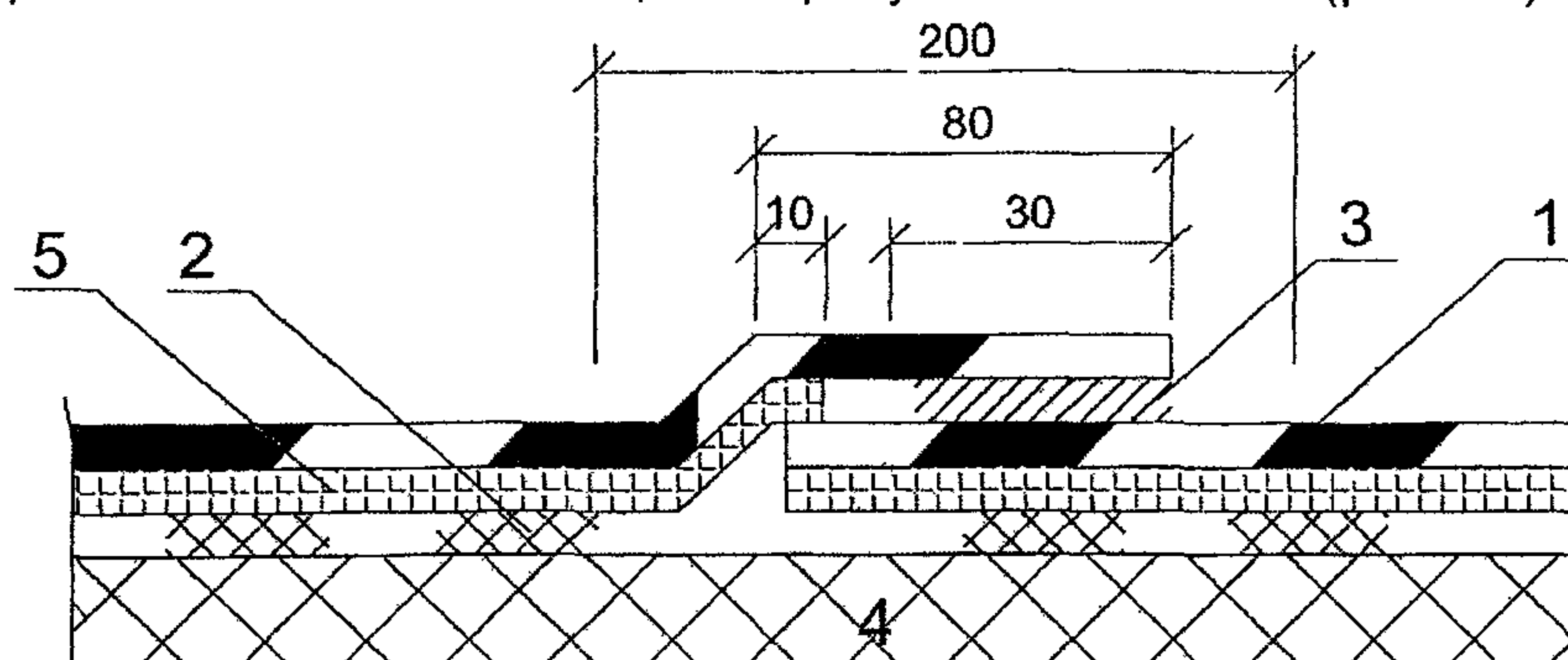
Рис. 2.9. Стык смежных полотенц термопластичной пленки
