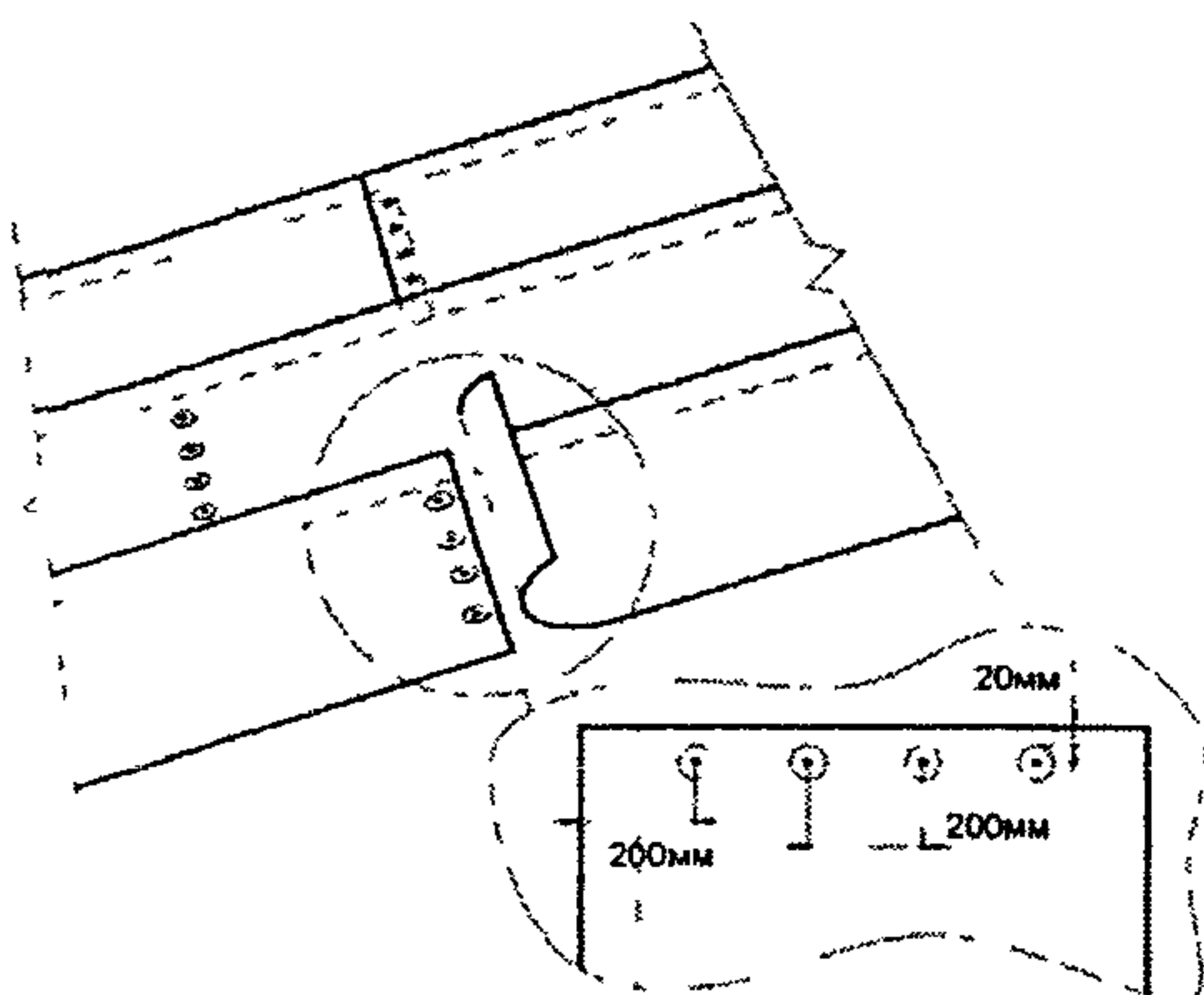
Рис. 27. Схема закрепления полотенц наплавляемых рулонных материалов на уклонах более 15 %
