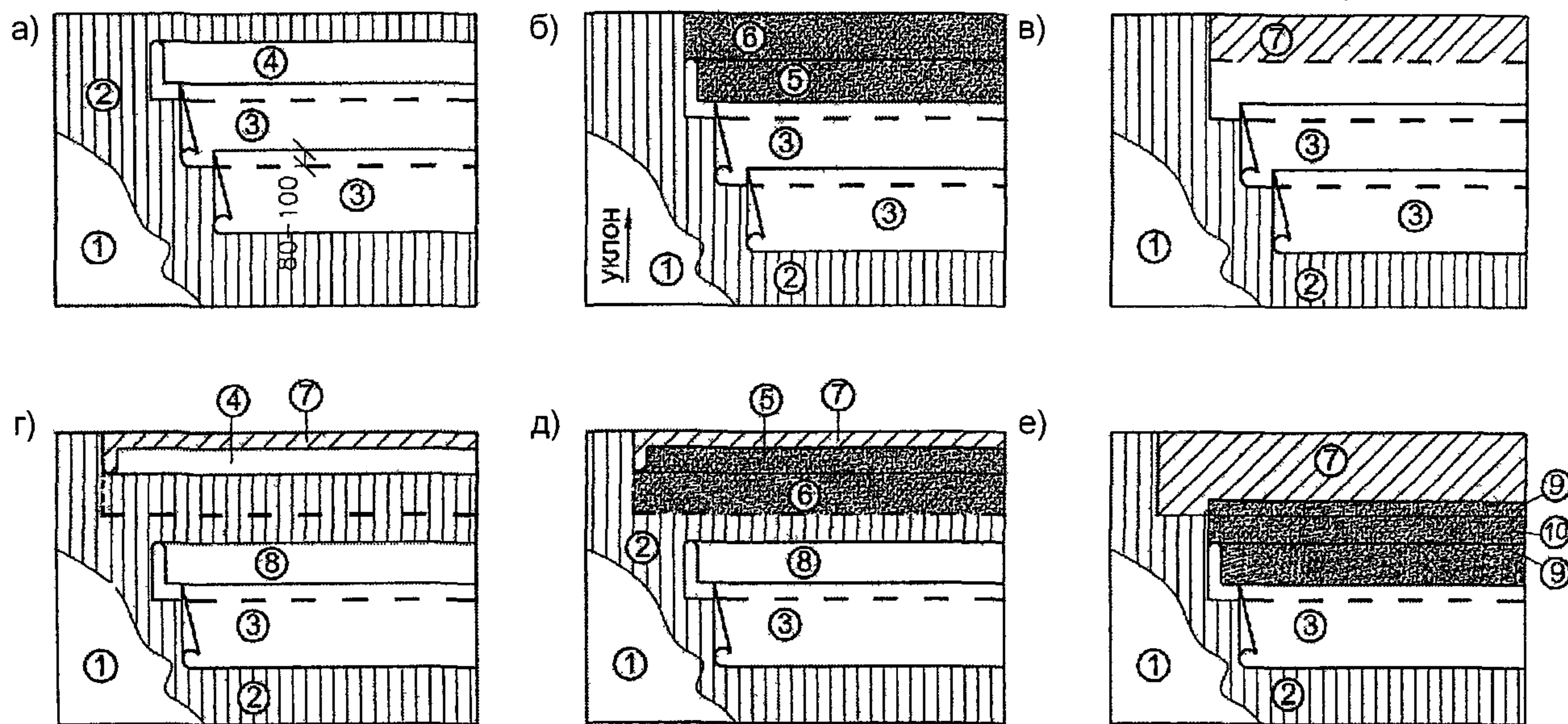
Рис. 2.8. Последовательность наклейки эластомерной пленки
