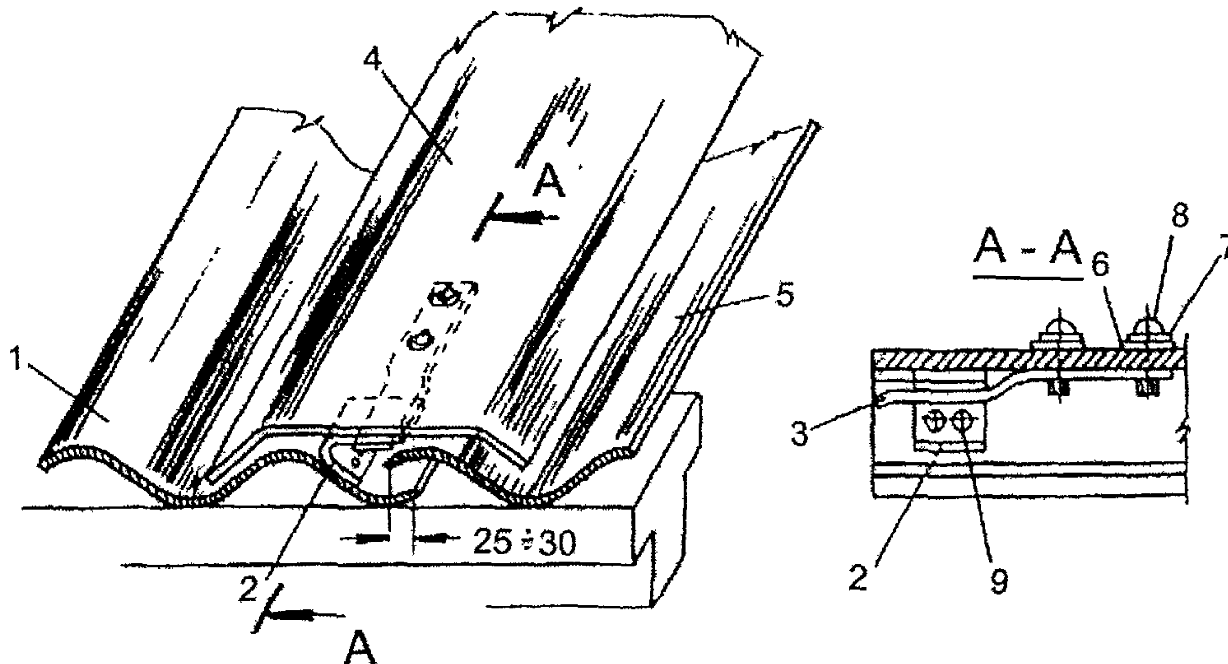
Рис 1.47 Компенсационный шов
