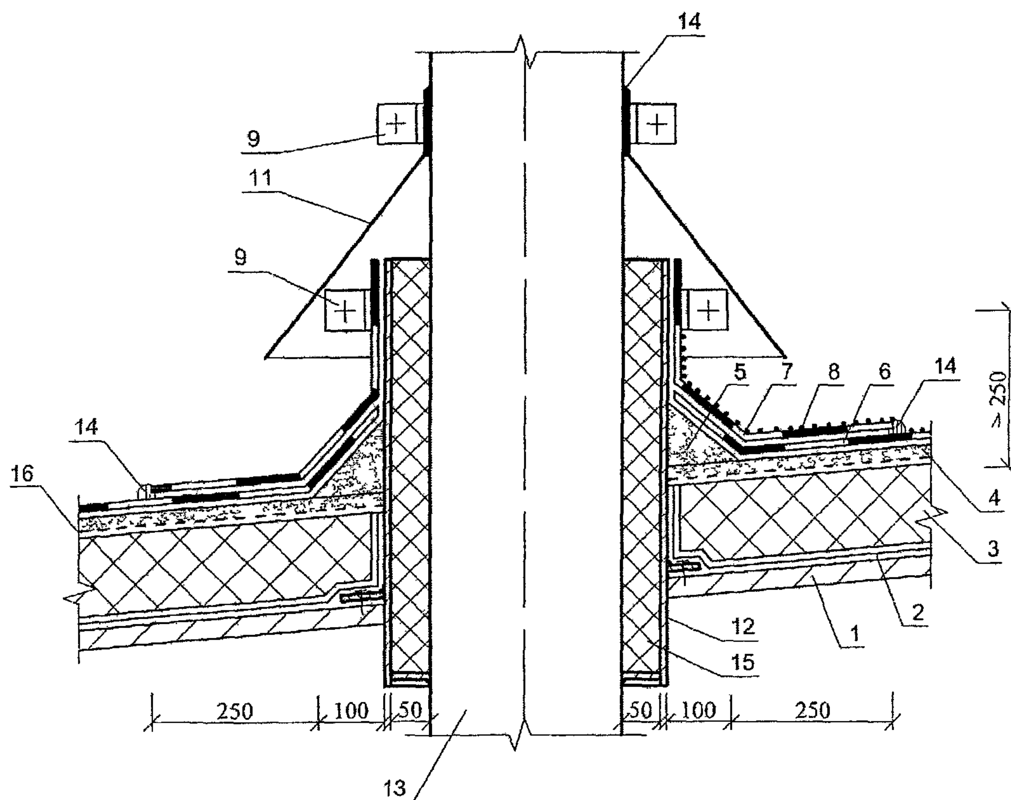
Рис 1 7 Пропуск трубы через покрытие с традиционной кровлей а) с герметизацией мастикой, б) с устройством бортиков из раствора, 1 – сборная железобетонная панель, 2 – пароизоляция, 3 – теплоизоляция, 4 и 5 – выравнивающая стяжка и бортик из цементно-песчаного раствора, 6 – основной водоизоляционный ковер, 7 – дополнительные слои водоизоляционного ковра, 8 – защитный слой (крупнозернистая посыпка), 9 – хомут, 10 – рамка из стального уголка, 11 – зонт из оцинкованной стали, 12 – патрубок с фланцем, 13 – труба, 14 – герметизирующая мастика, 15 – стекловата, 16 – разделительный слой
