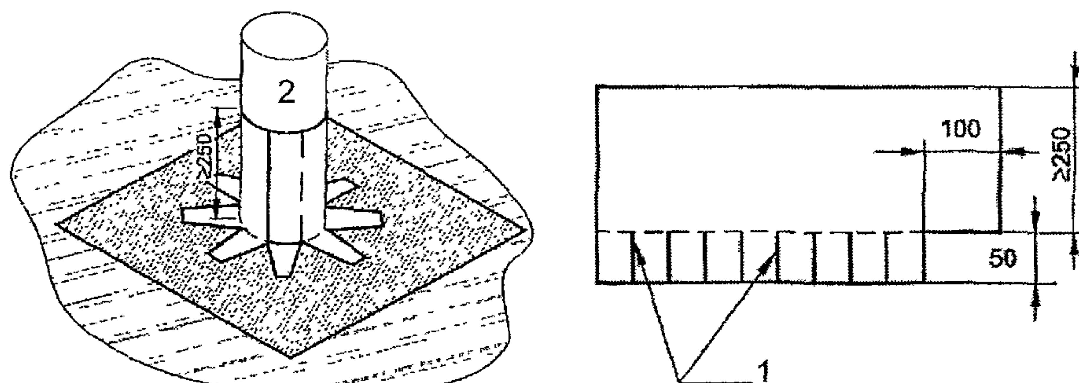
Рис. 2.19. Обклейка трубы нижним слоем дополнительного водоизоляционного ковра 1 – надрезы; 2 – труба.
