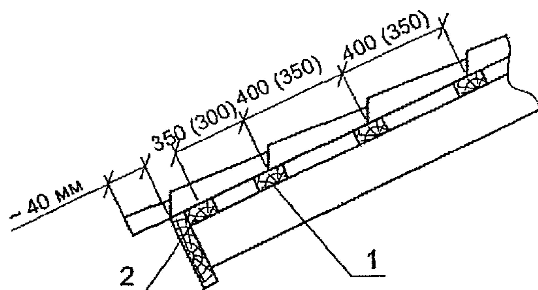
Рис. 1.37. обрешетка под металлочерепицу
