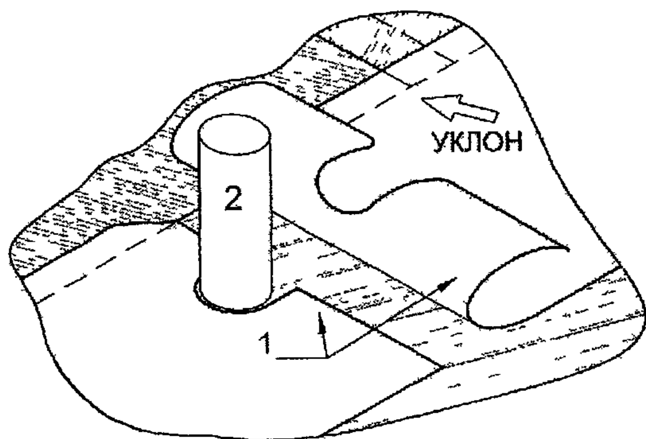
Рис 2 23 Обклейка трубы нижним слоем основного водоизоляционного ковра
