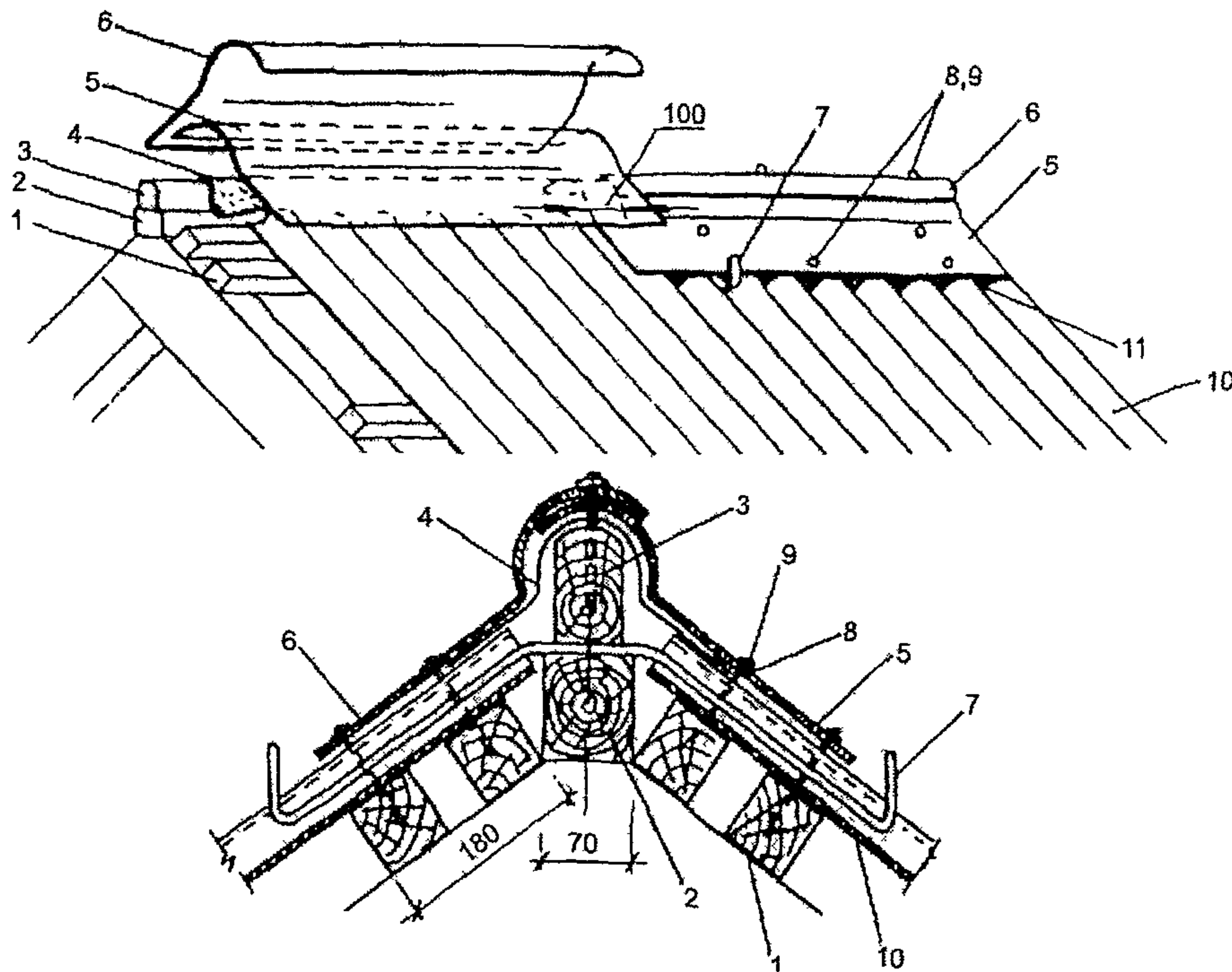
Рис. 1 48. Конек (ребро) кровли по деревянным брускам
