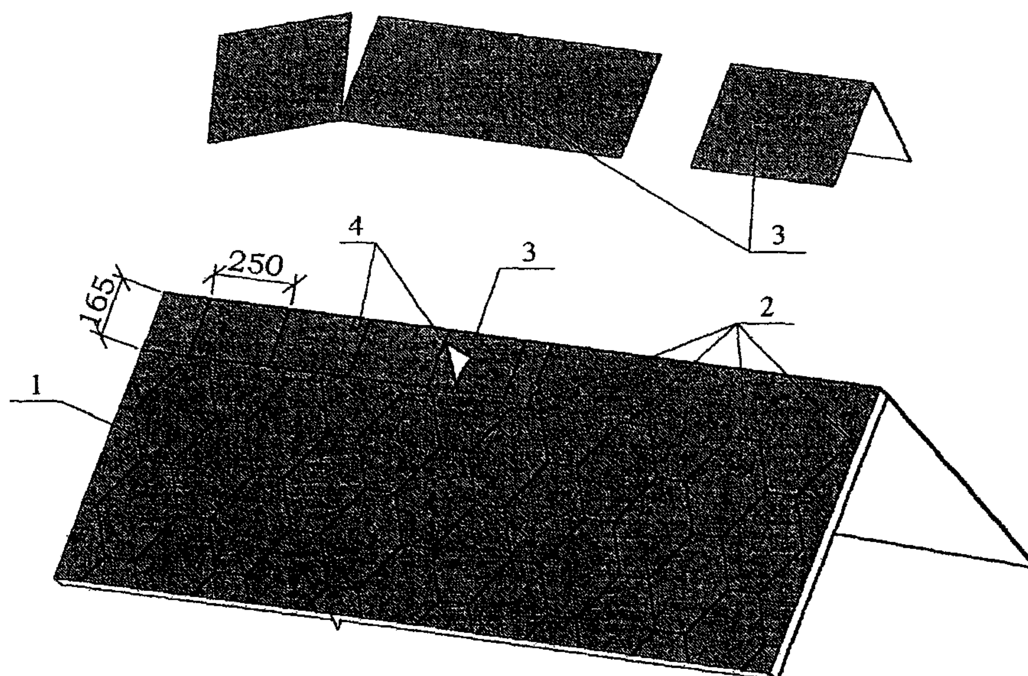
Рис. 2.41. Укладка коньковой черепицы
