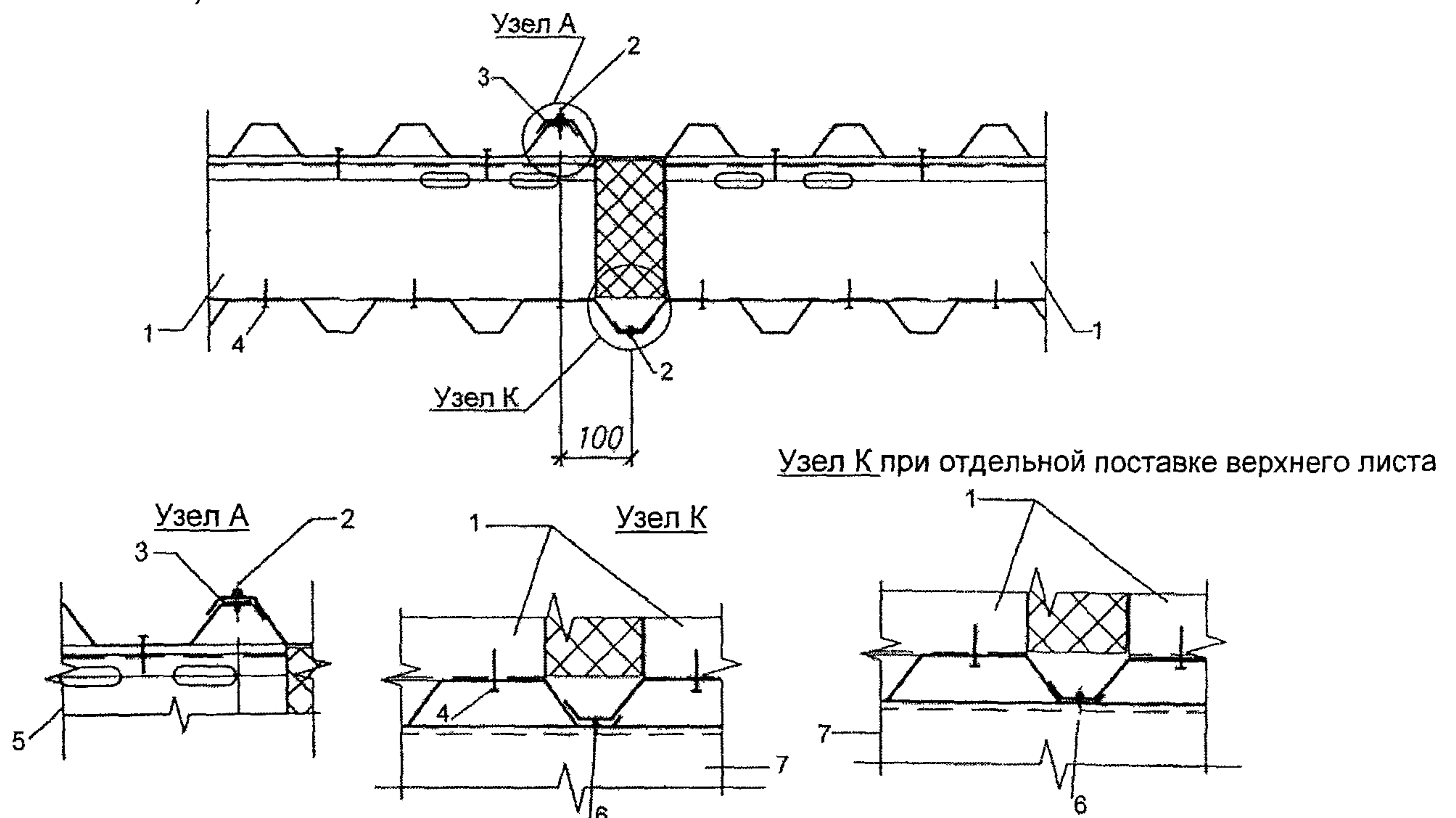
Рис. 2.48. Крепление металлического профлиста в составе кровельной панели 1 – панель; 2 – комбинированная заклепка; 3 – прокладка из EPDM; 4 – крепление профлиста к каркасу панели; 5 – каркас панели; 6 – винт; 7 – прогон (опора панели).
