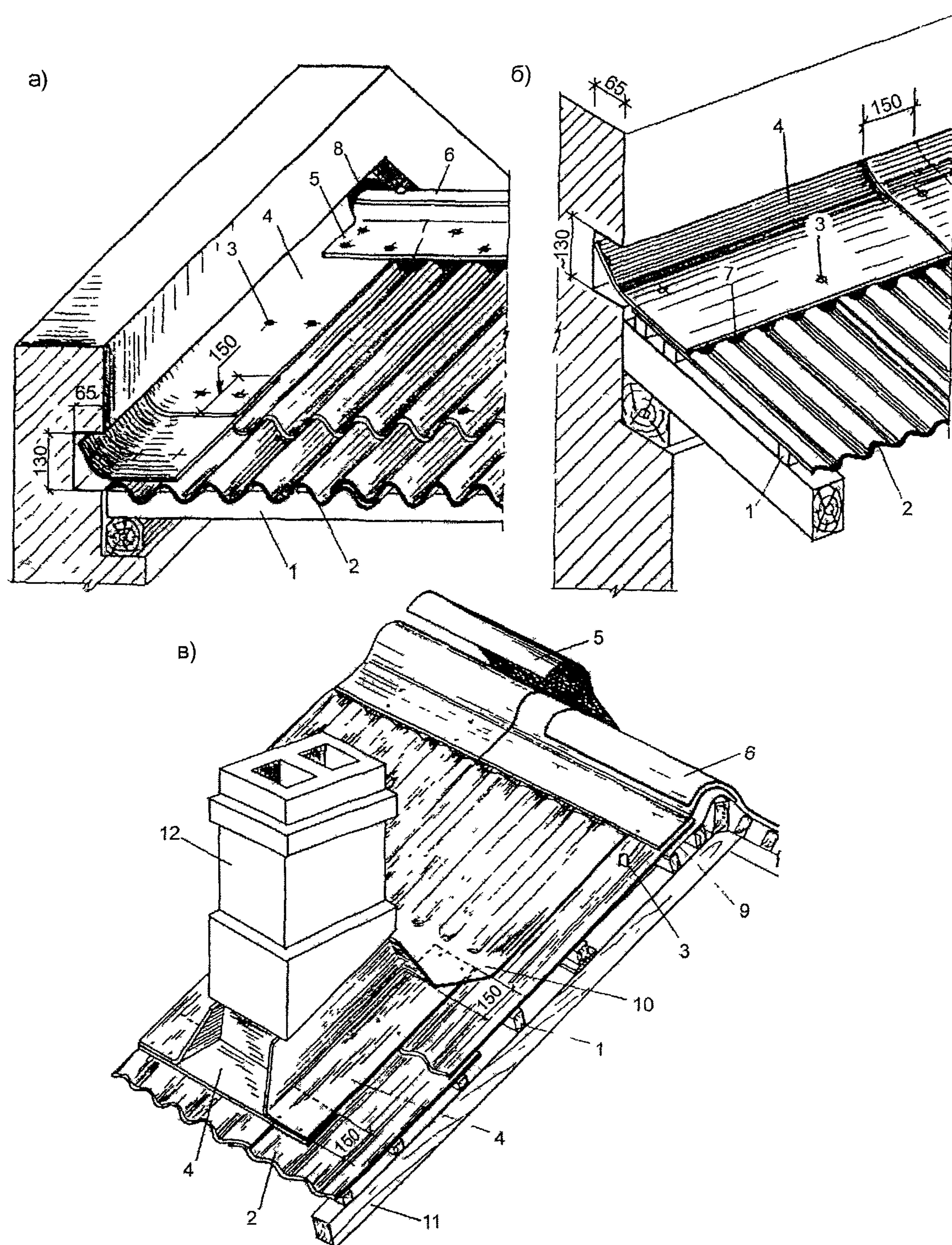
Рис 1 46 Примыкание кровли из асбестоцементных волнистых листов к поперечной (а) и продольной (б) стенам и к дымовой трубе (в)
