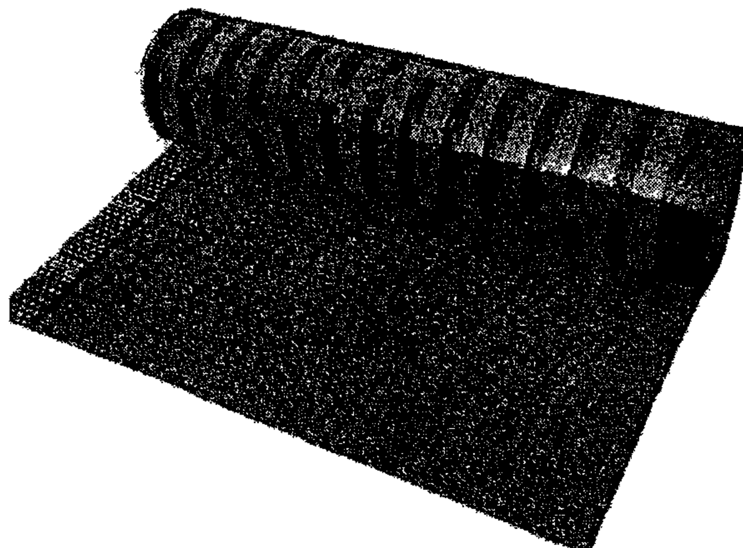
Рис 2 27 Рулонный материал с полосами приклеивающего состава (ТУ 5774-016-05766480-01)
