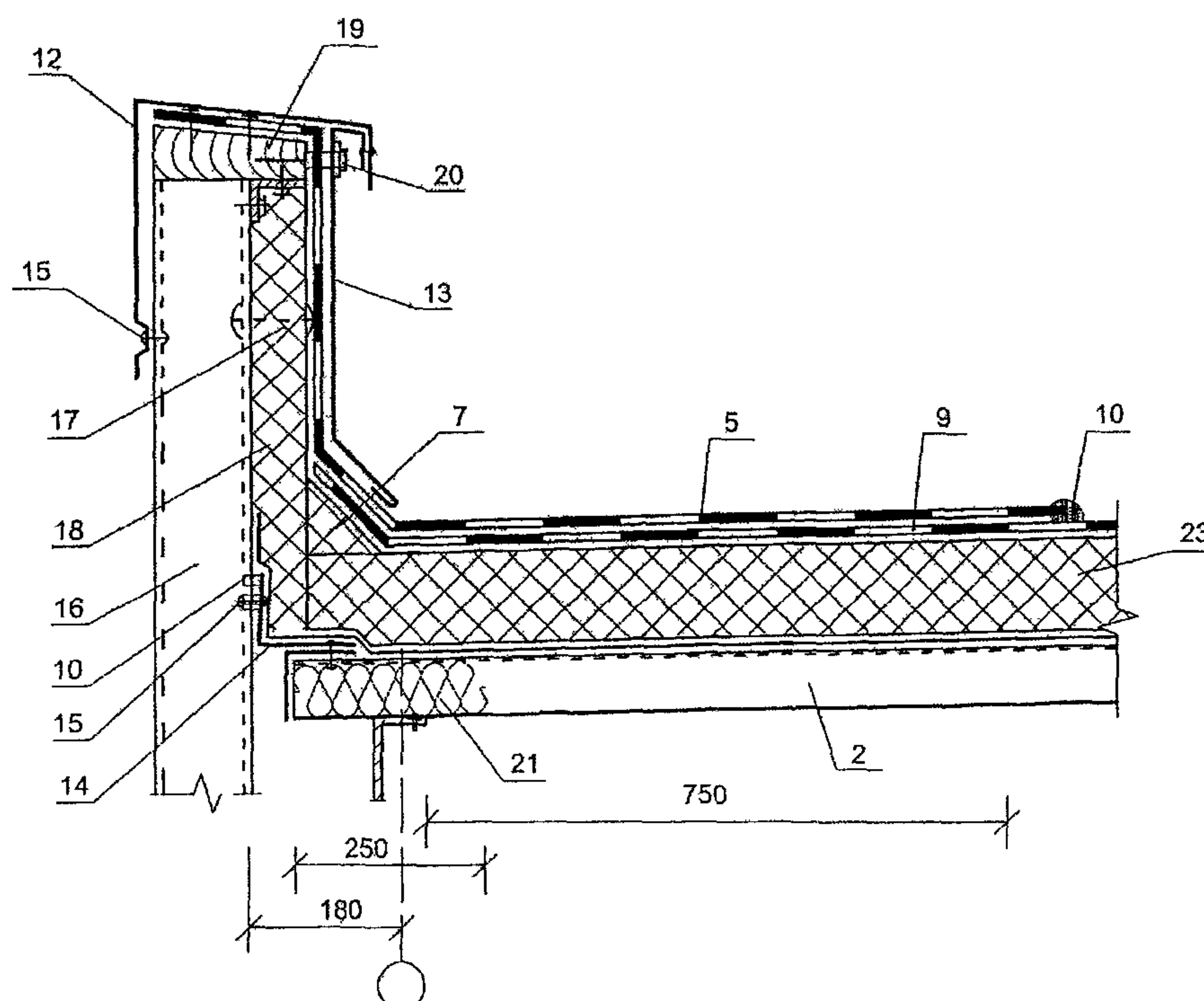
Рис 1 5 Примыкание к парапету
