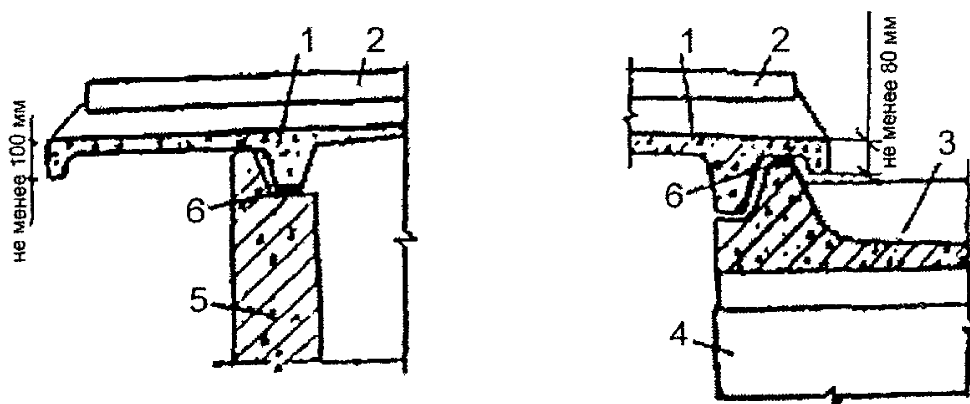
Рис. 1.67. Конструкции свесов
