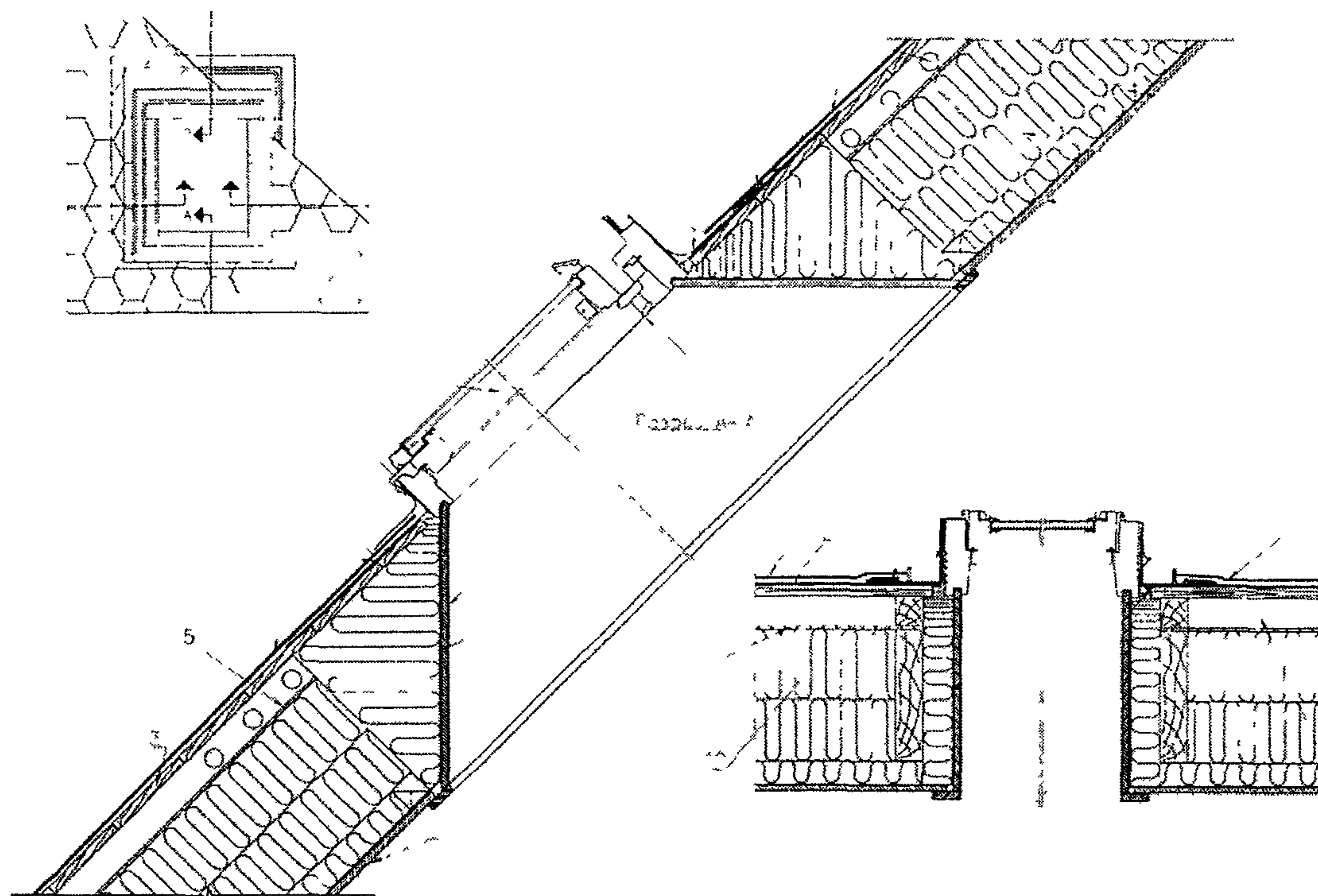
Рис. 1.35. Узел установки мансардного окна "Velux"
