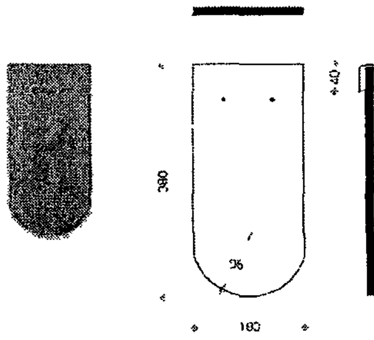
Рис. 1.17. План черепицы, поперечный и продольный разрезы.
