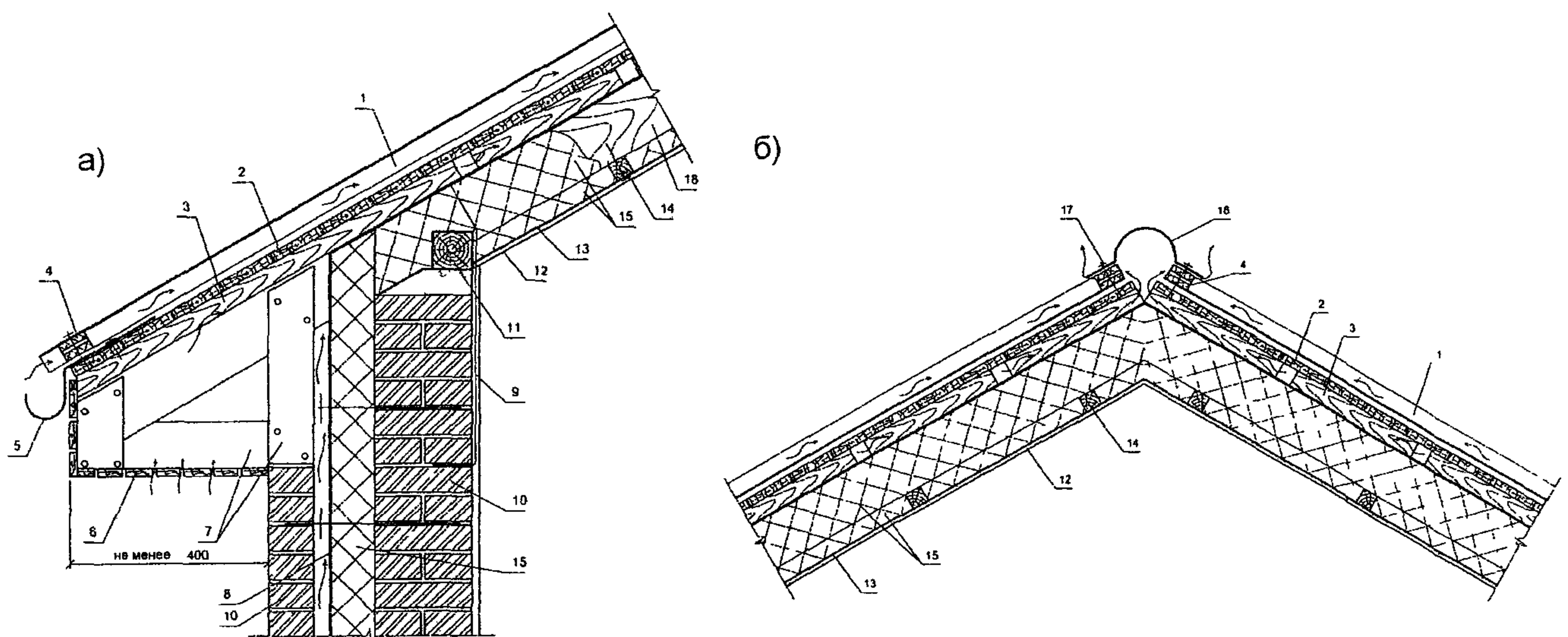
Рис. 1 50 Карнизный (а) и коньковый (б) узлы кровли
