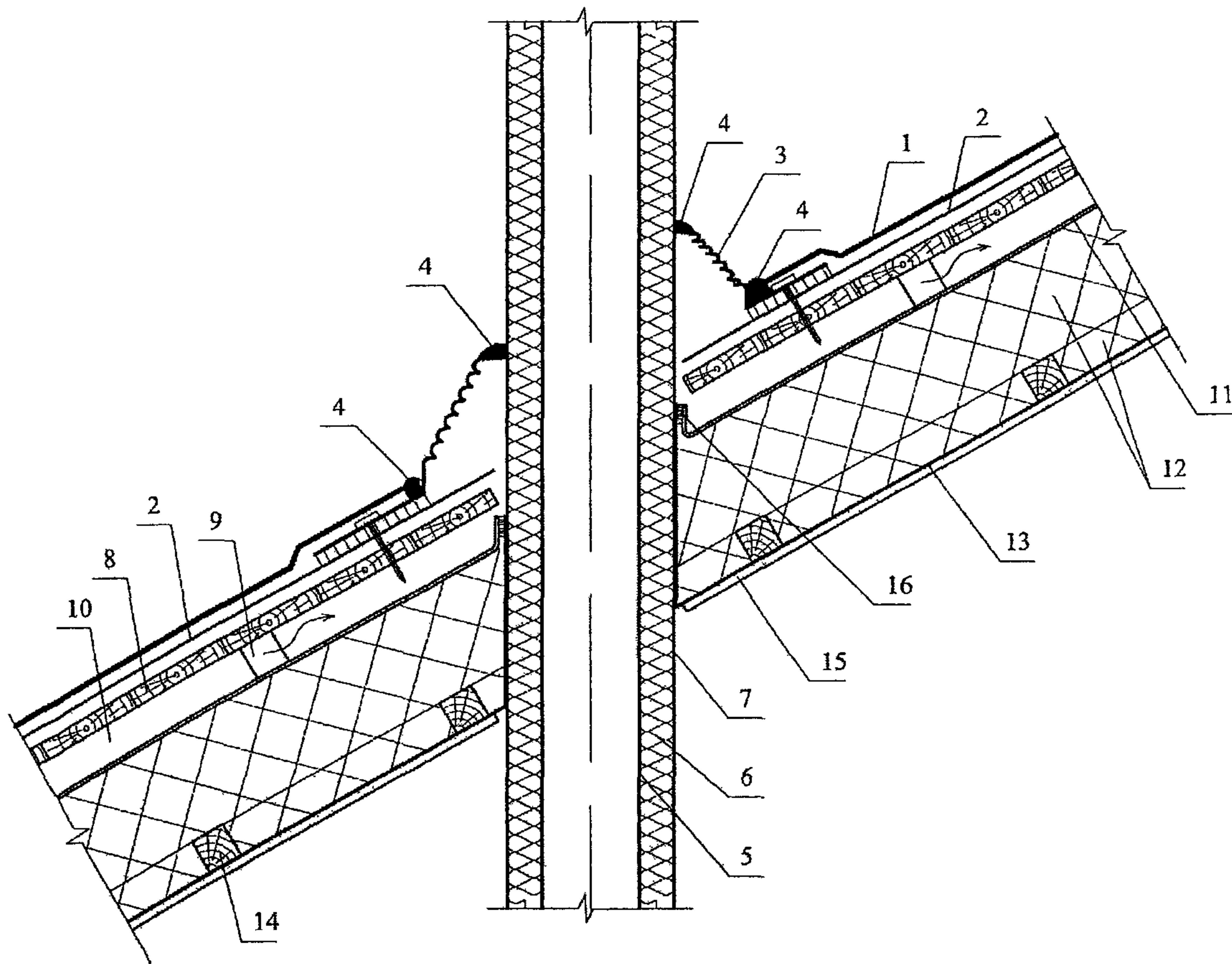
Рис. 1.33. Примыкание кровли к дымовой металлической трубе
