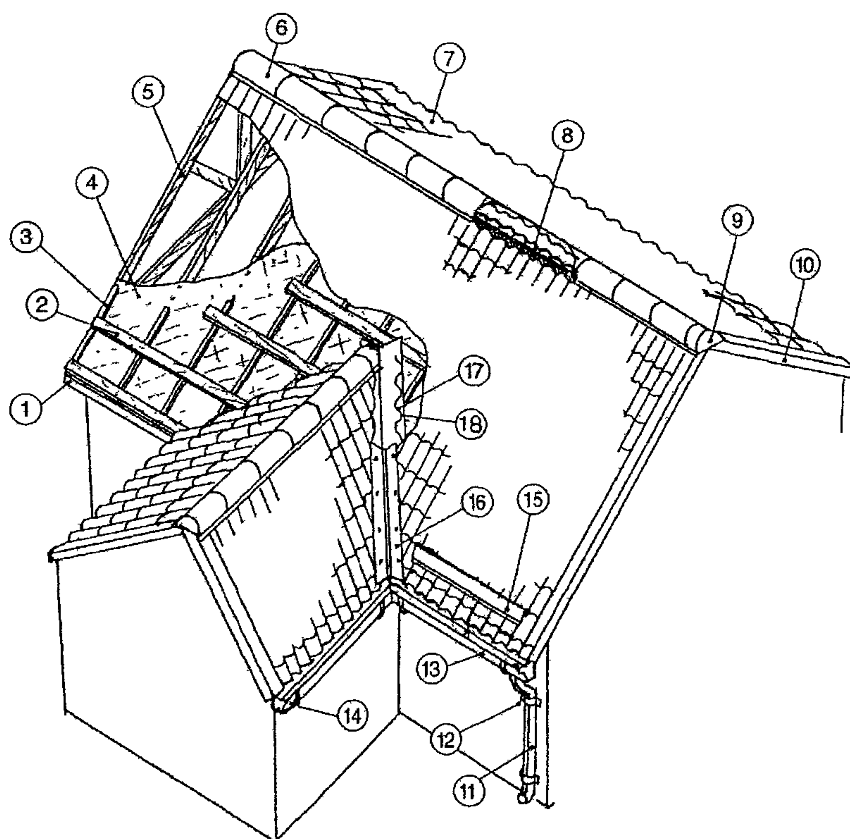
Рис. 1.38. Схема кровли из металлочерепицы
