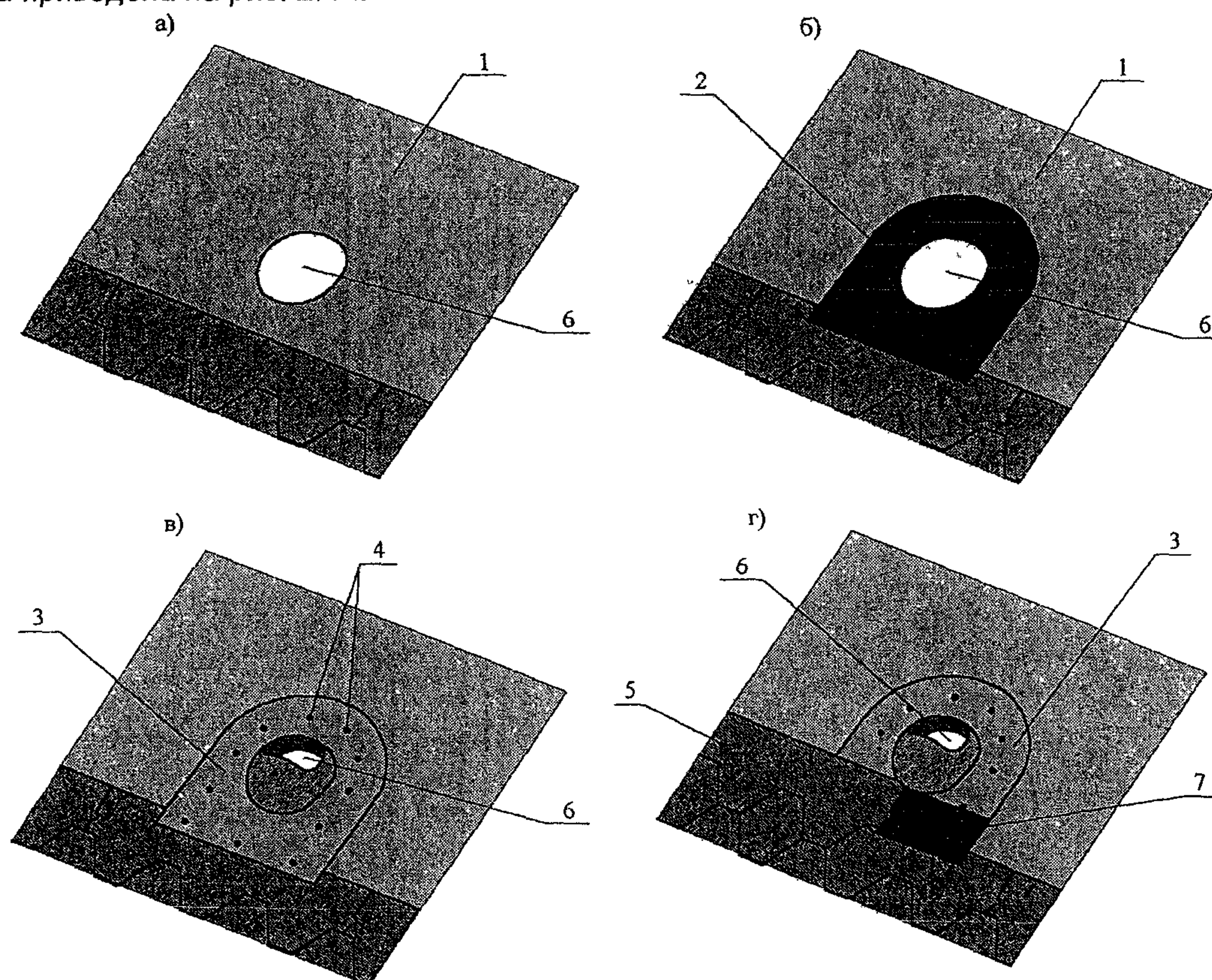
Рис. 2.42. Установка фланца для вентилятора
