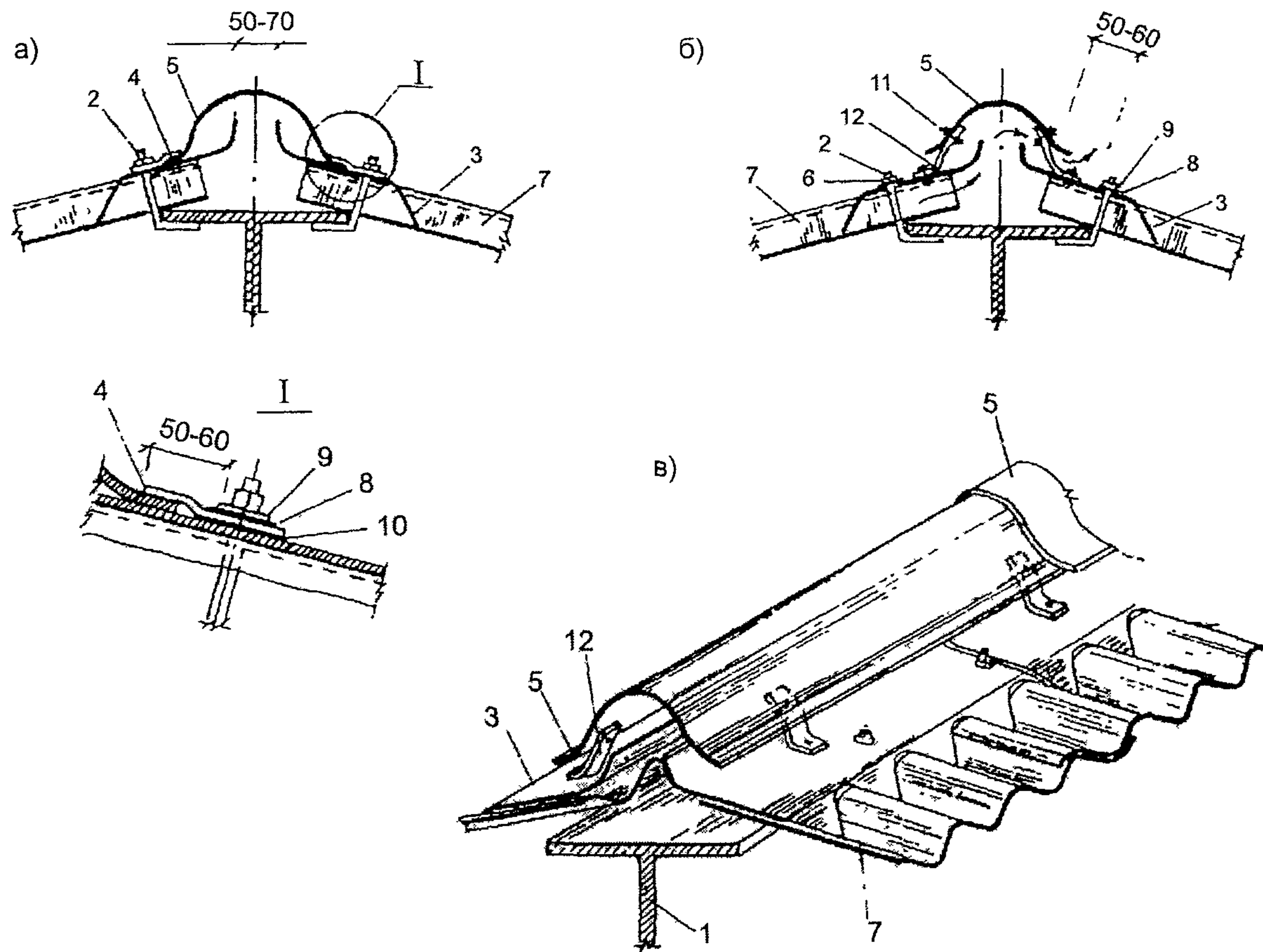
Рис 1 49. Коньковые узлы по металлическим прогонам
