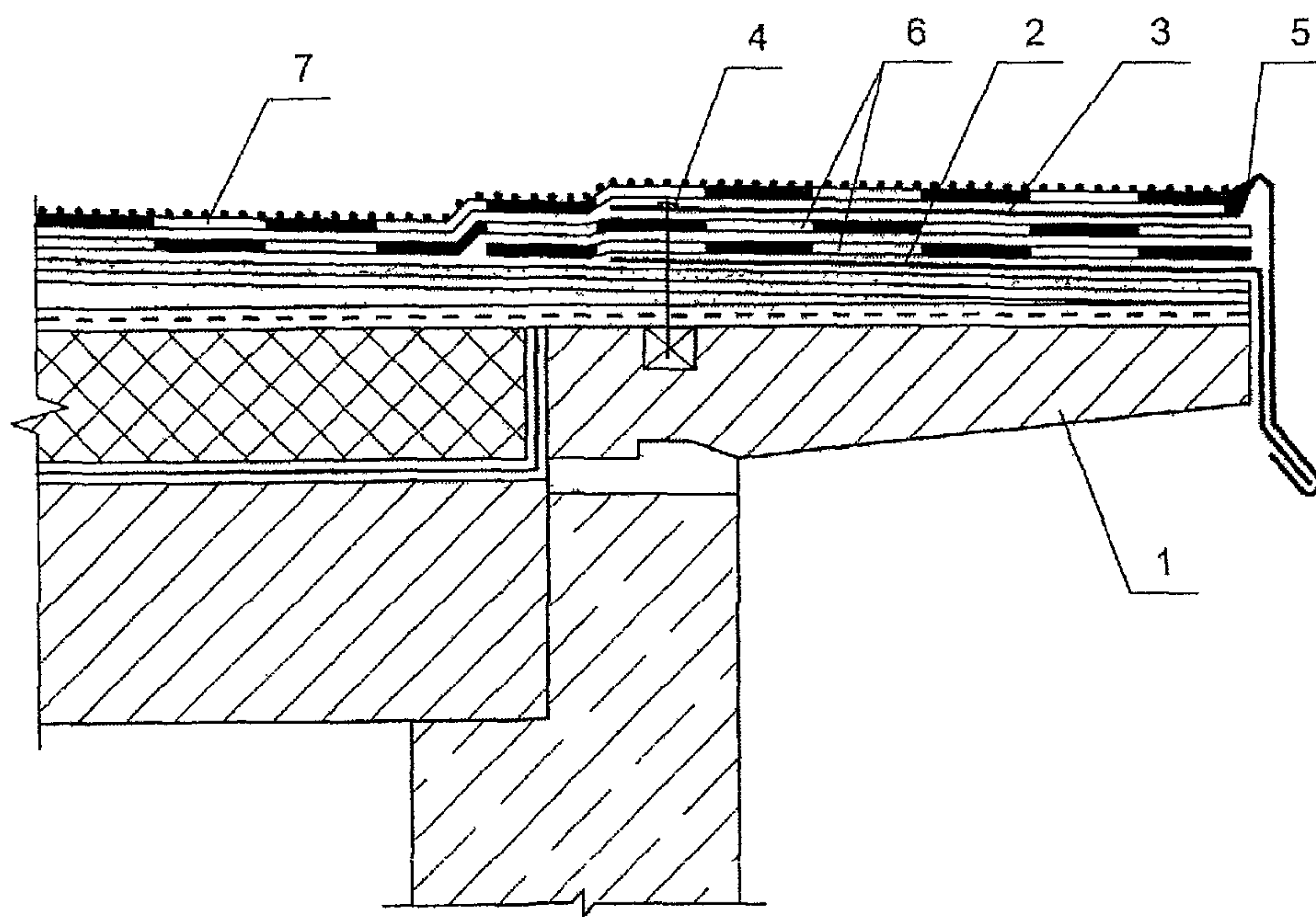
Рис. 1.9 Карниз кровли
