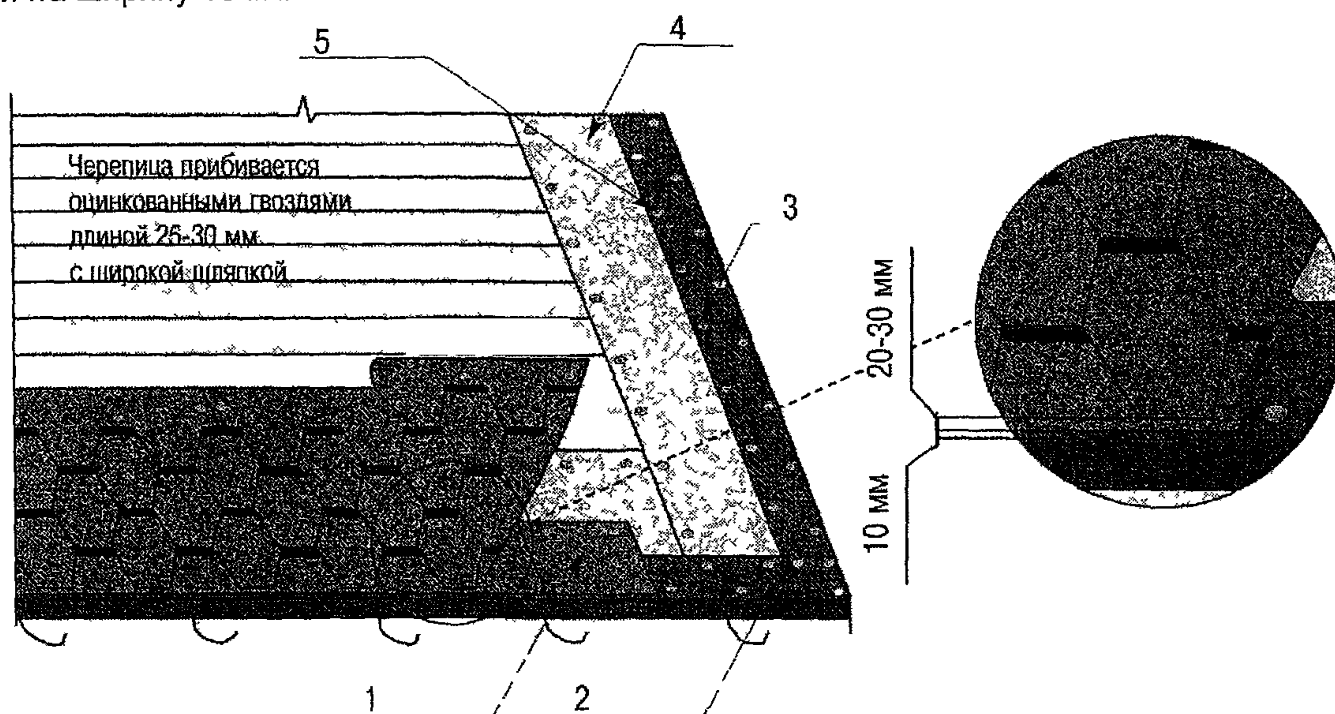
Рис 2 38 Схема укладки гибкой черепицы 1 – карнизная черепица, 2 – металлическая карнизная планка, 3 – металлическая (фронто- нная) планка, 4 – подкладочный слой, 5 – кровельные гвозди
