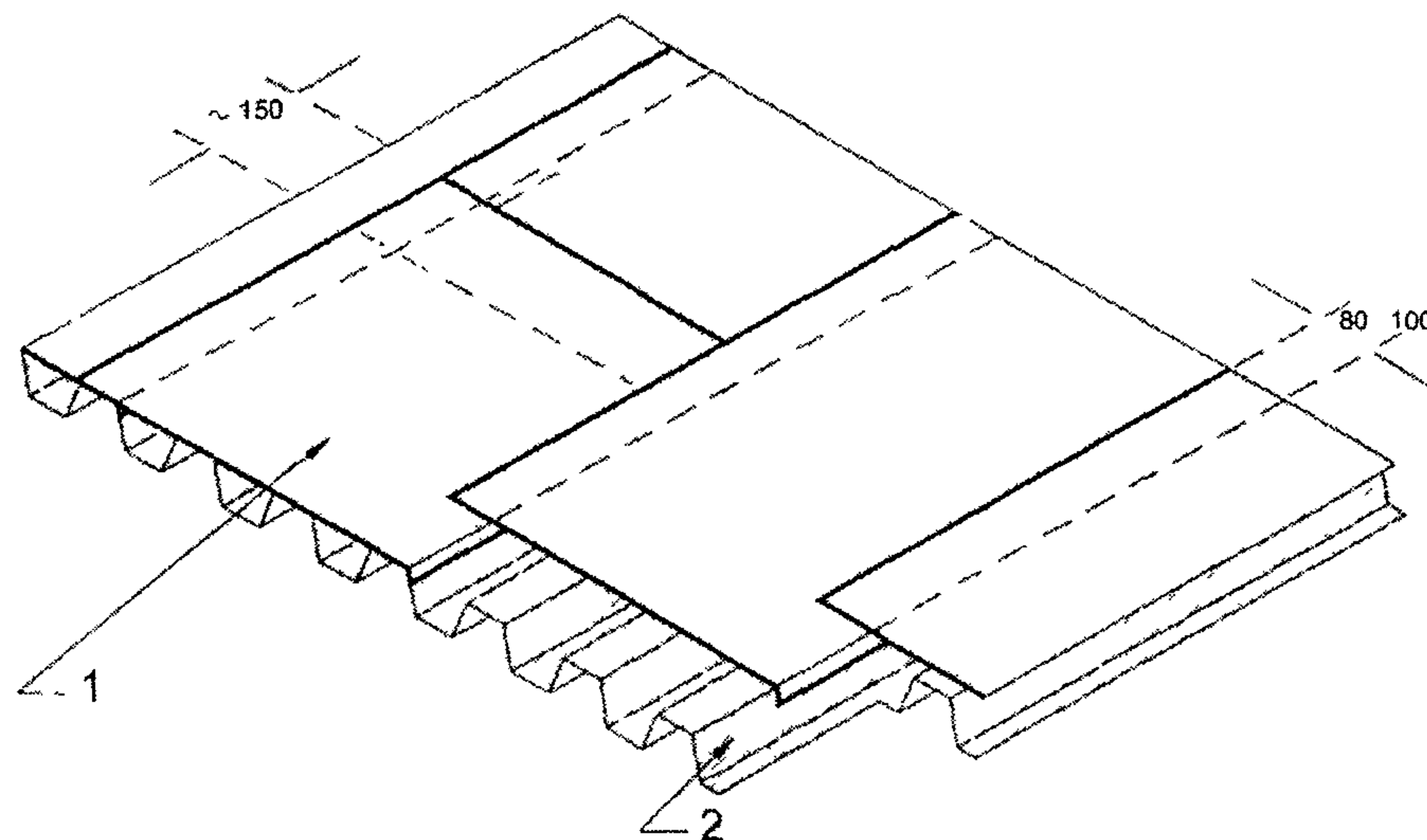
Рис. 2.1. Укладка пароизоляционного материала на профнастил 1 – пароизоляция; 2 – профнастил
