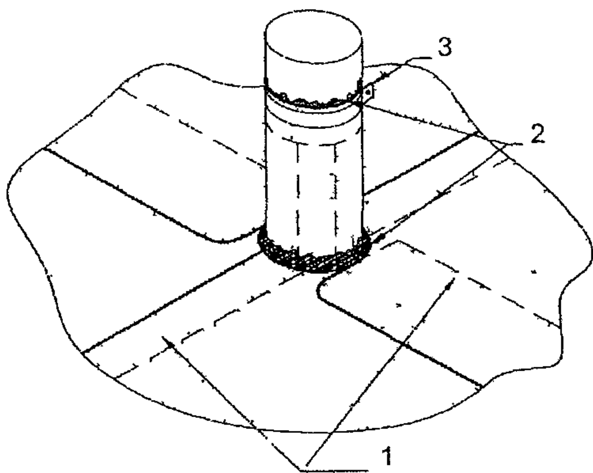
Рис 2 22 Обклейка трубы верхним слоем основного водоизоляционного ковра
