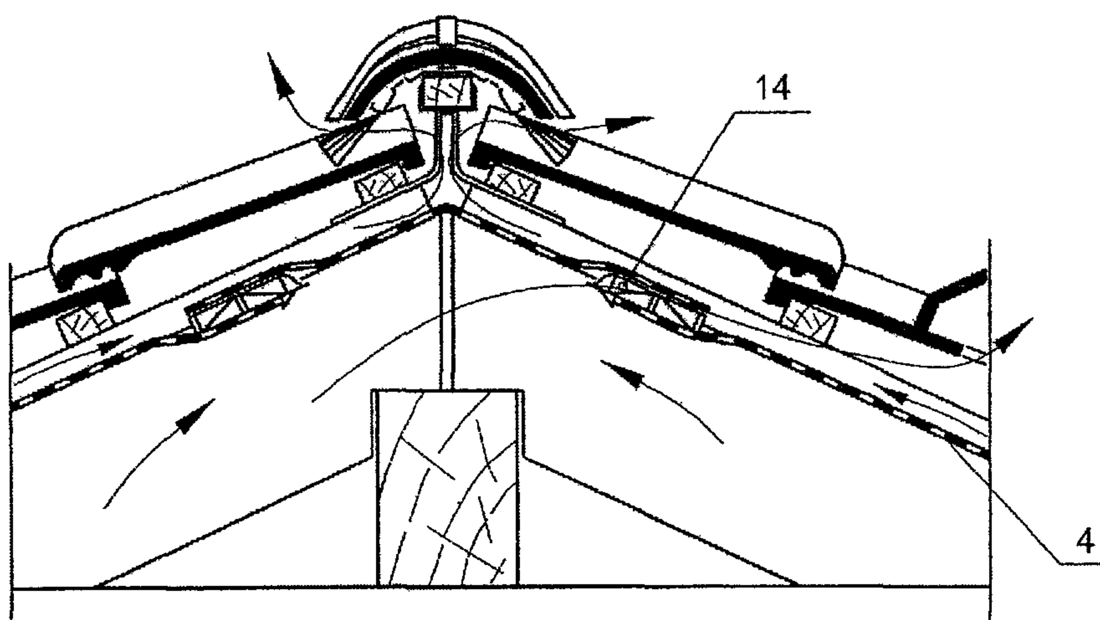
Рис 1 26 Конек крыши с одним вентиляционным зазором (а) и чердачной кровли с вентиляционным элементом в диффузионно-гидроизоляционной пленке (б)
