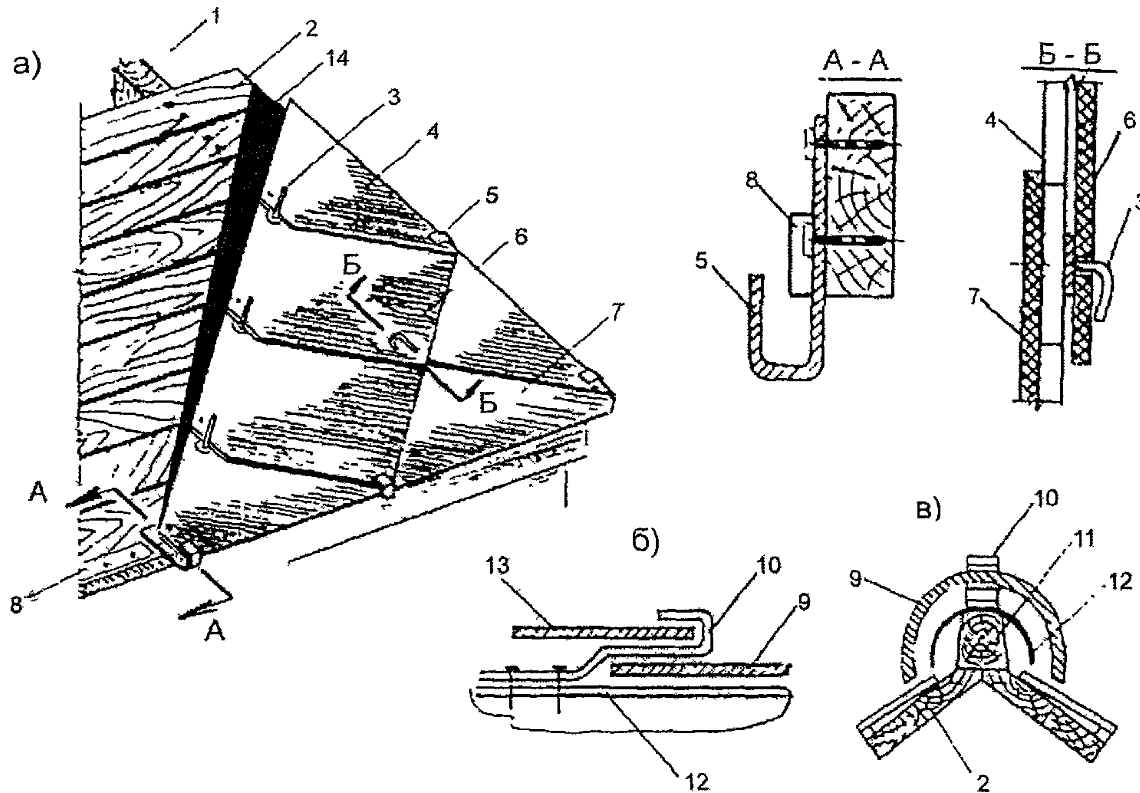
Рис. 1.52. Кровля из асбестоцементных плоских плиток а – общий вид; б – продольный разрез конька; в – поперечный разрез конька; 1 – стропильная нога; 2 – обрешетка; 3 – противоветровая кнопка; 4 – половина плитки, 5 – противоветровая скоба 2×25 мм; 6 – рядовая плитка; 7 – краевая плитка; 8 – уравнивательная деревянная рейка с сечением 8×50 мм; 9 – желобчатый конек; 10 – скоба сечением 2×25 мм, 11 – брус сечением 50×80 мм; 12 – лента гидроизоляционного материала; 13 – накрывающий конец желобчатого конька, 14 – водоизоляционный слой.
