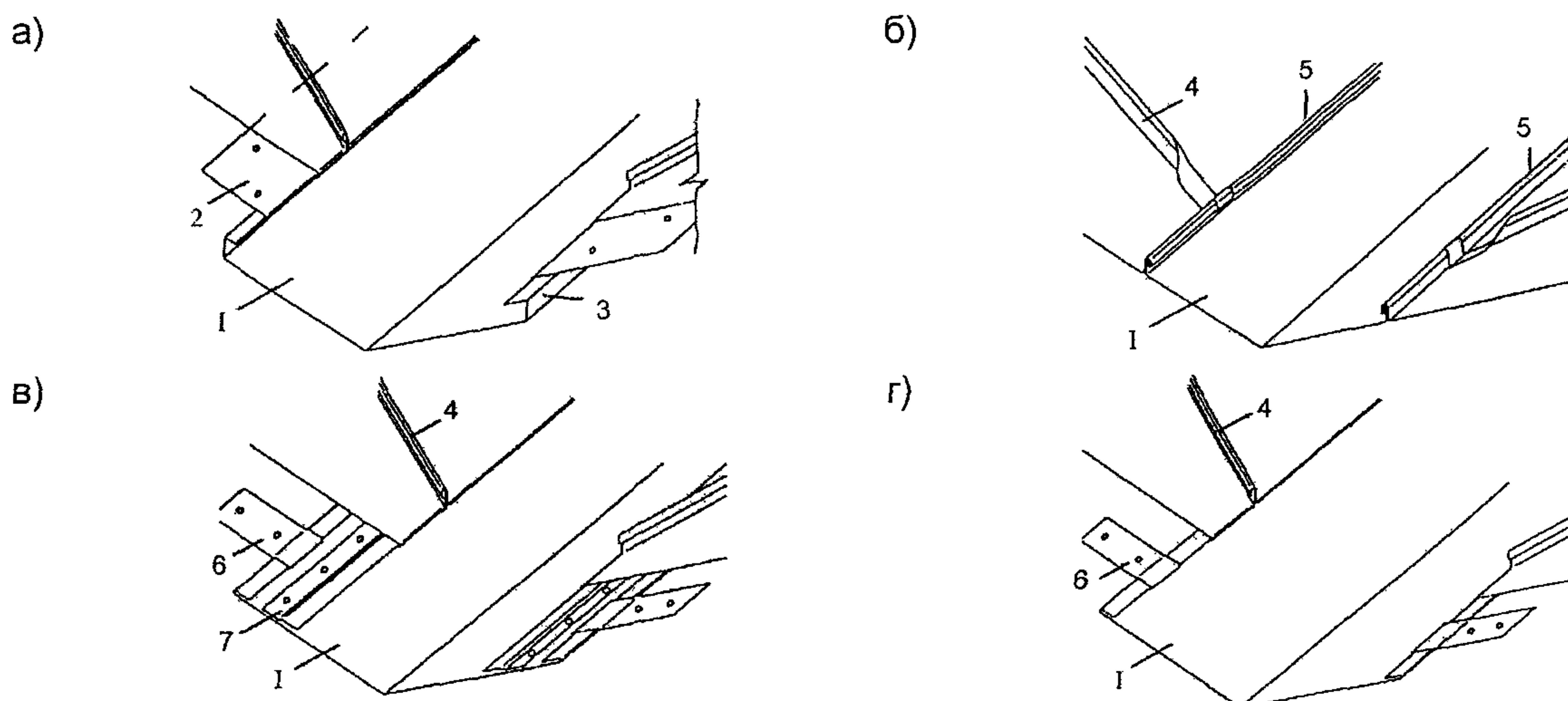
Рис. 1.64. Ендова кровли
