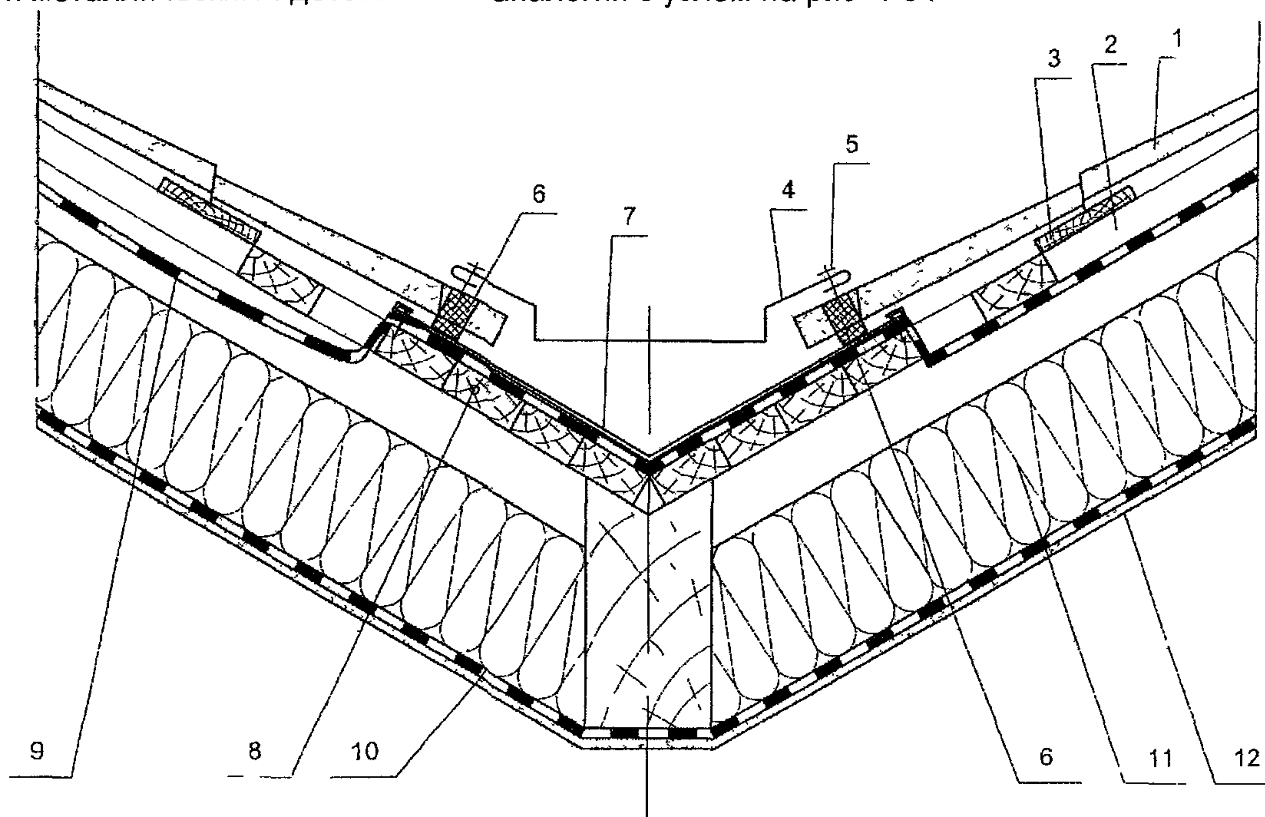
Рис. 1 42. Ендова кровли
