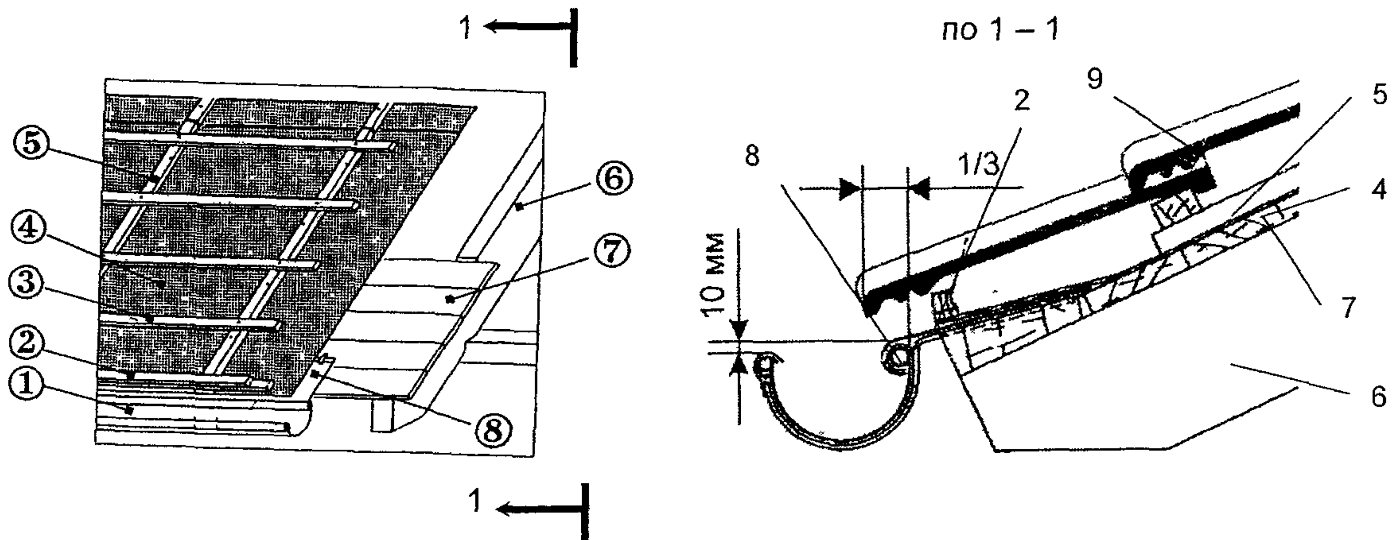
Рис. 2.30. Карнизный свес кровли.
