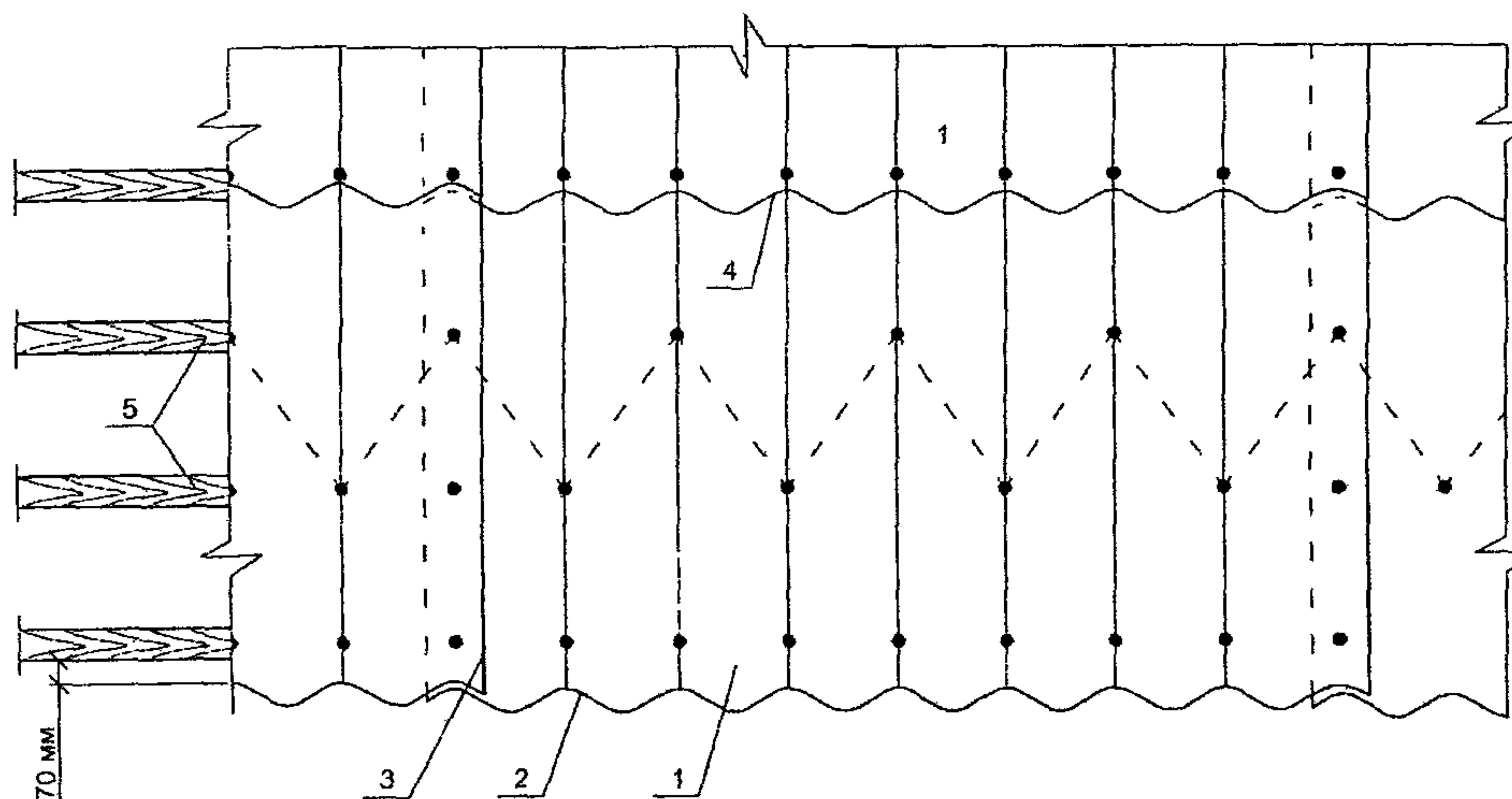
Рис. 2.47. Крепление битумного волнистого листа
