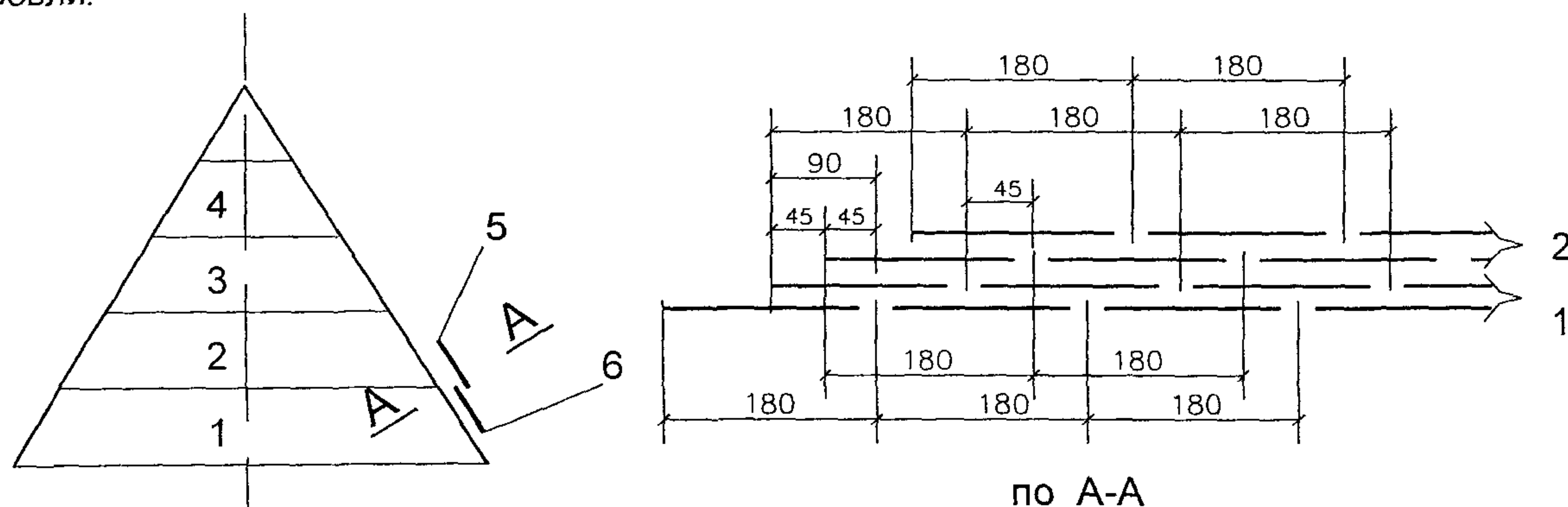
Рис. 2.32. Неравномерная укладка черепицы.
