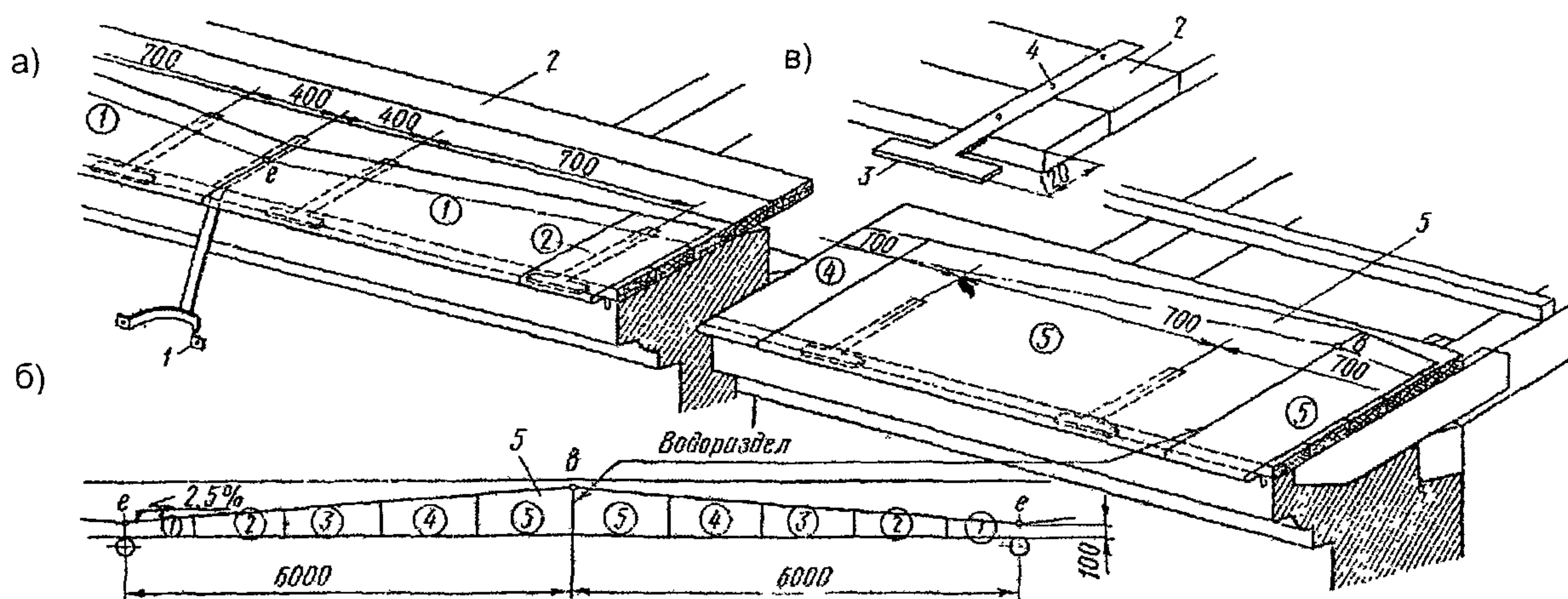
Рис. 2.50. Устройство карнизного свеса
