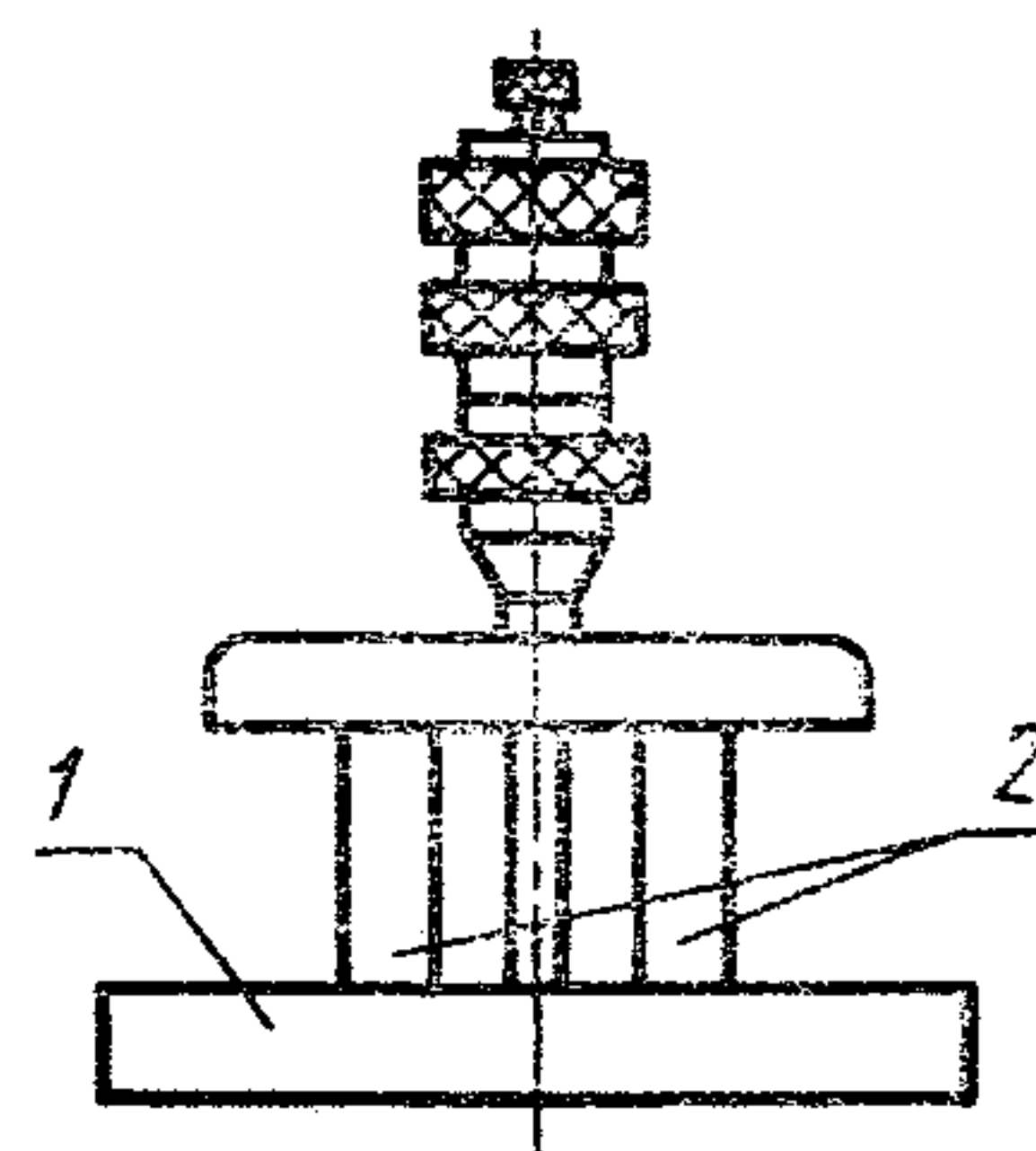
1—стеклянная пластина или плита; 2—концевые меры
