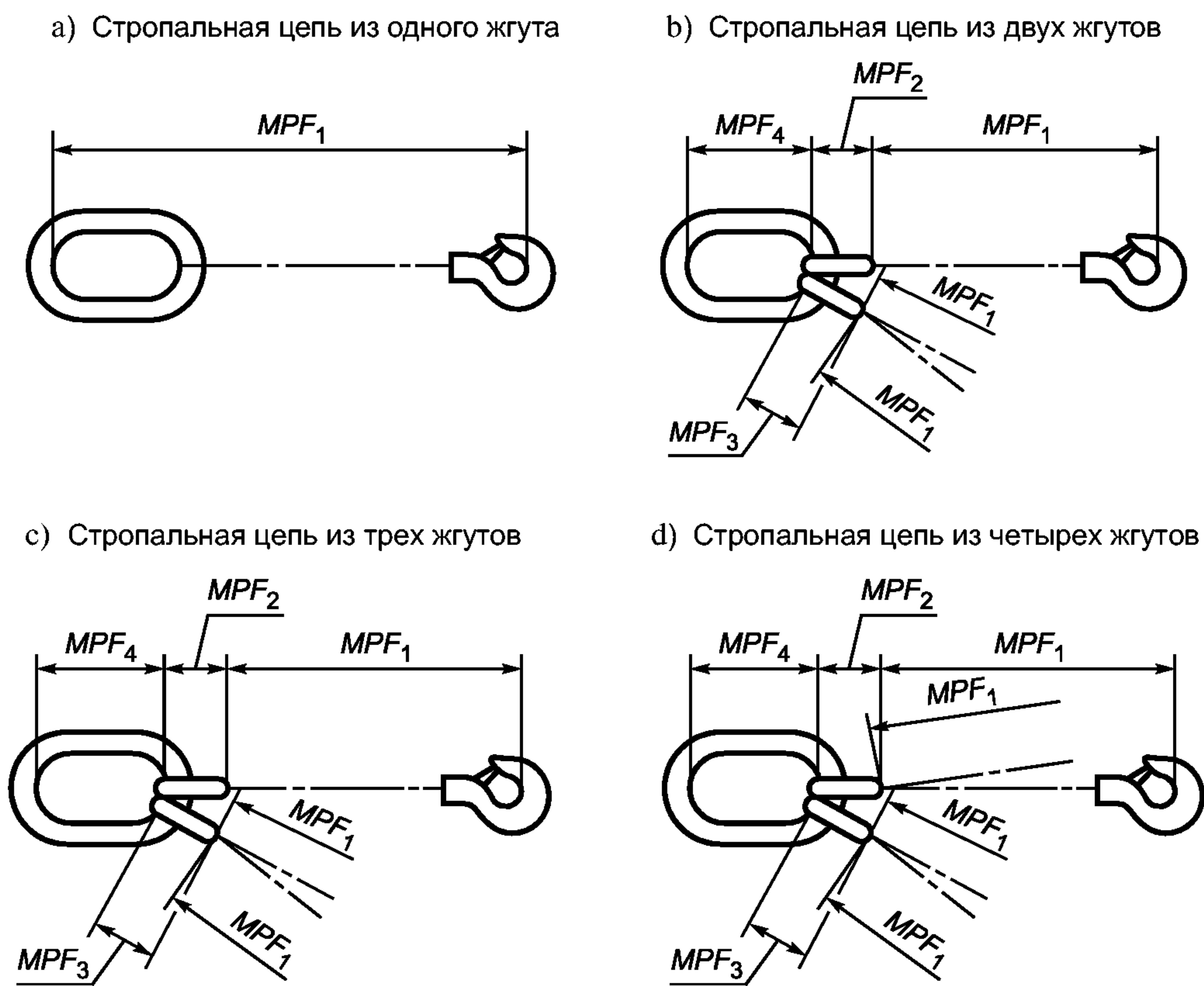
Рисунок 6 — Испытательные участки стропальных цепей
