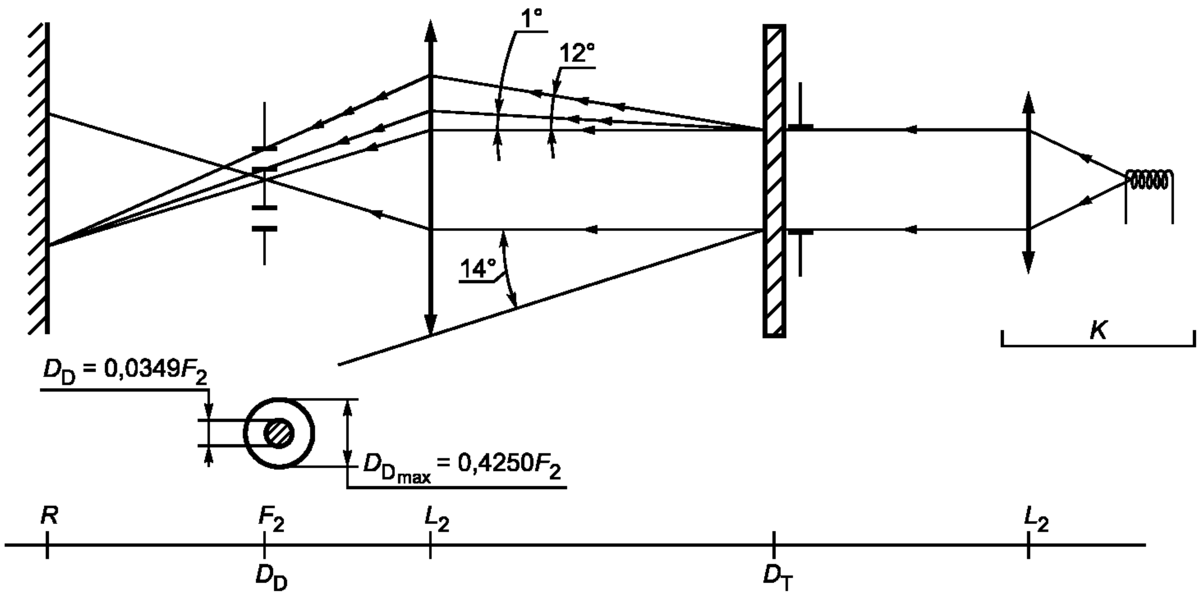
Рисунок 1 — Схема измерения коэффициента рассеивания и пропускания света
