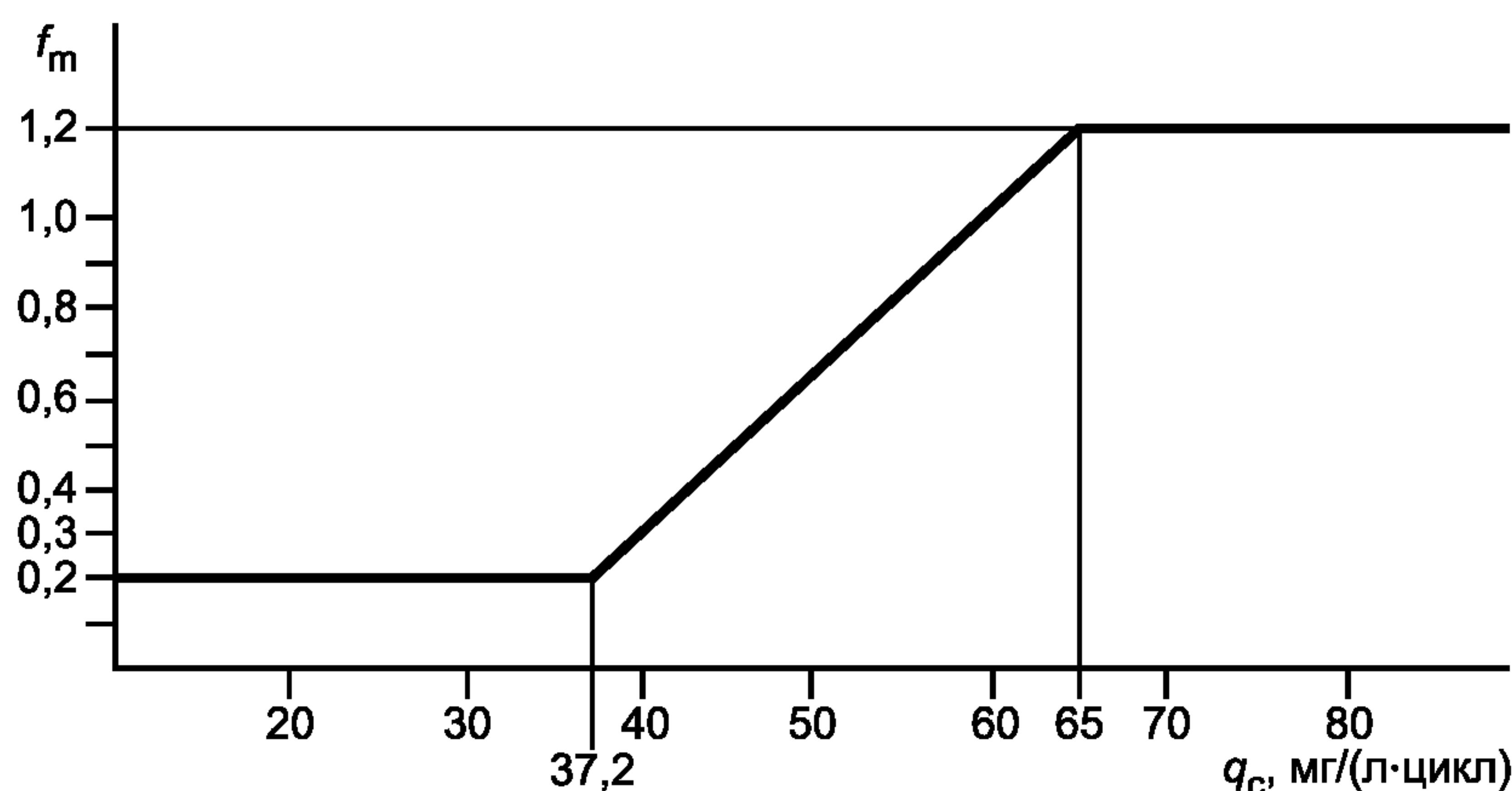
Рисунок 4 — Коэффициент двигателя f_m как функция корректированной удельной цикловой подачи топлива q_c
