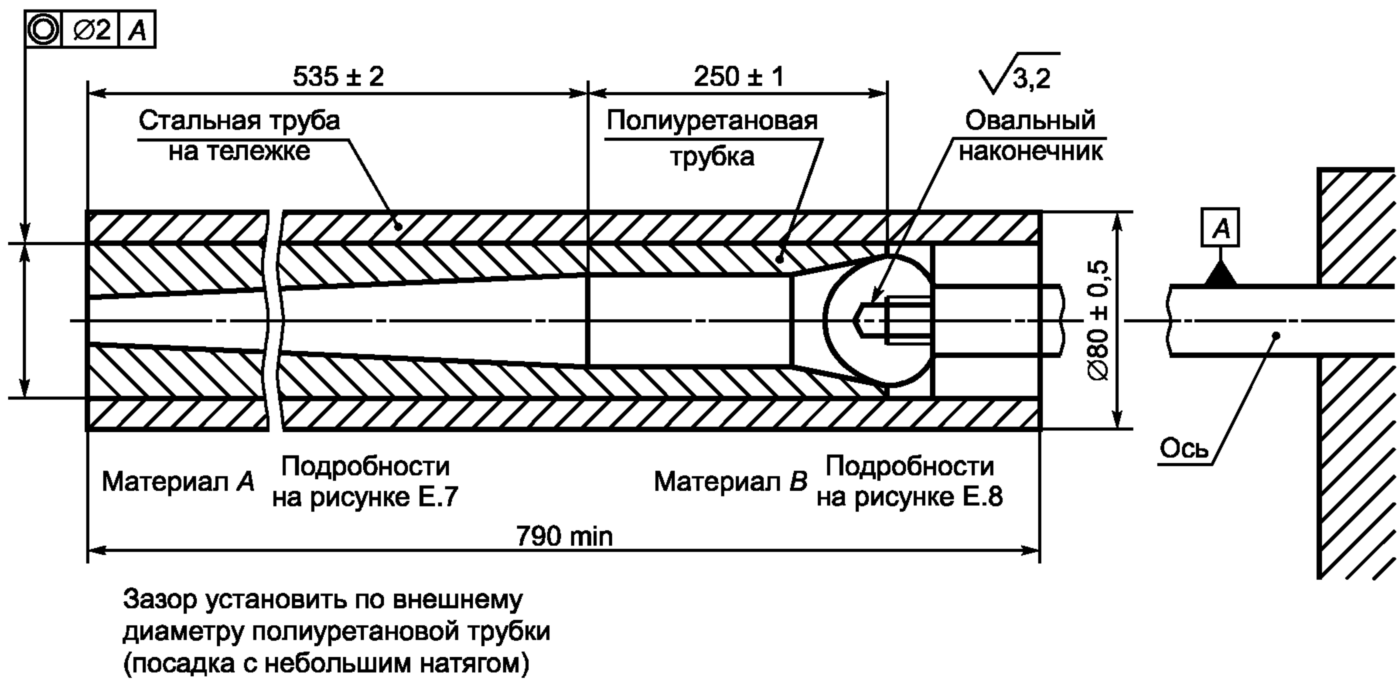
Рисунок Е.6 — Размеры стопорного устройства
