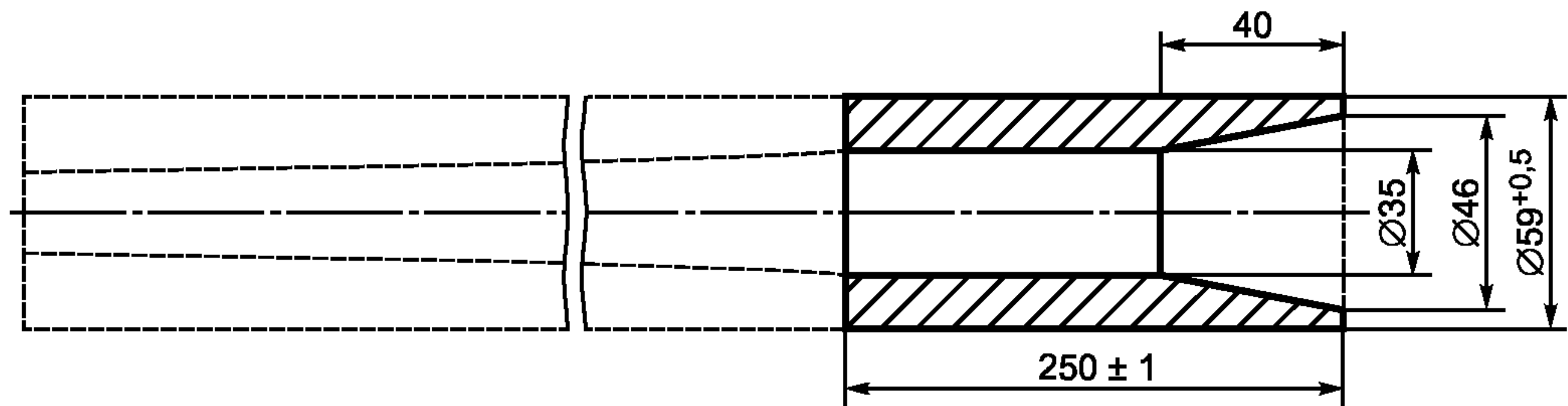
Рисунок Е.8 — Полиуретановая трубка из материала В
