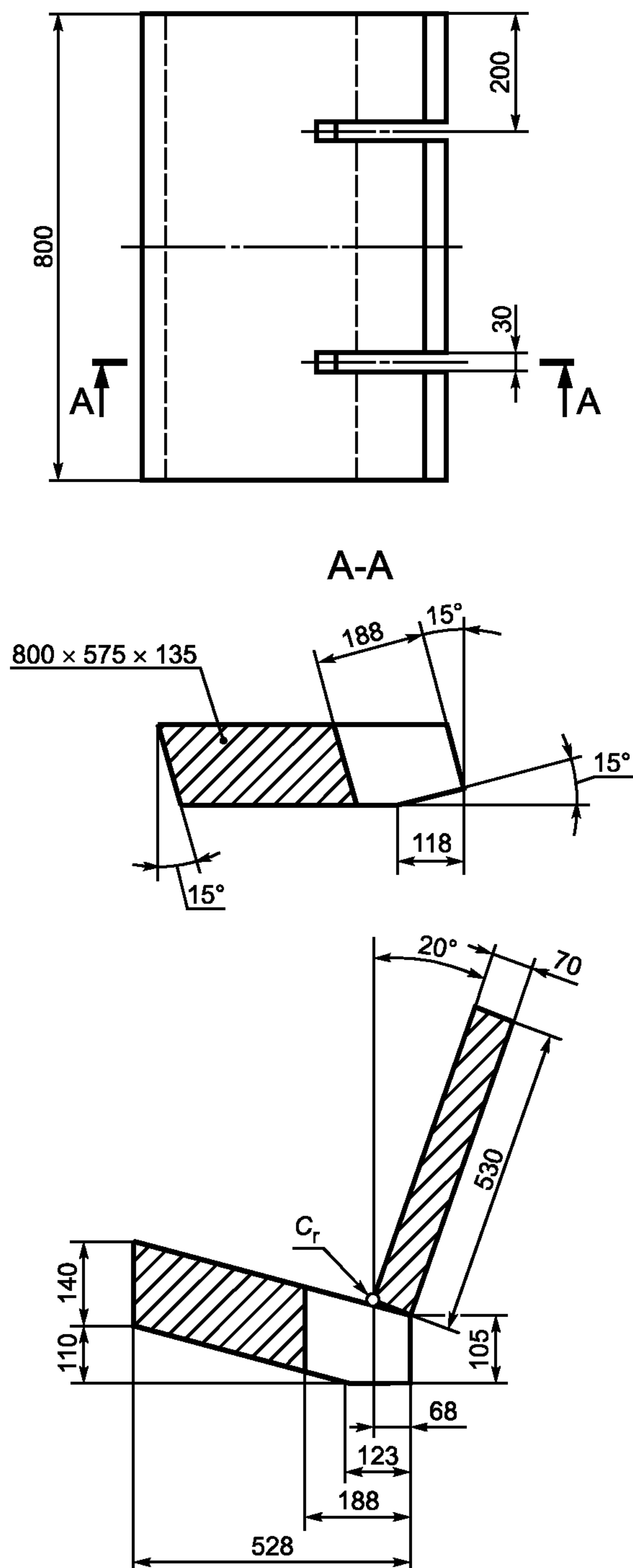
Рисунок Е.2 — Размеры сиденья и подушек сиденья
