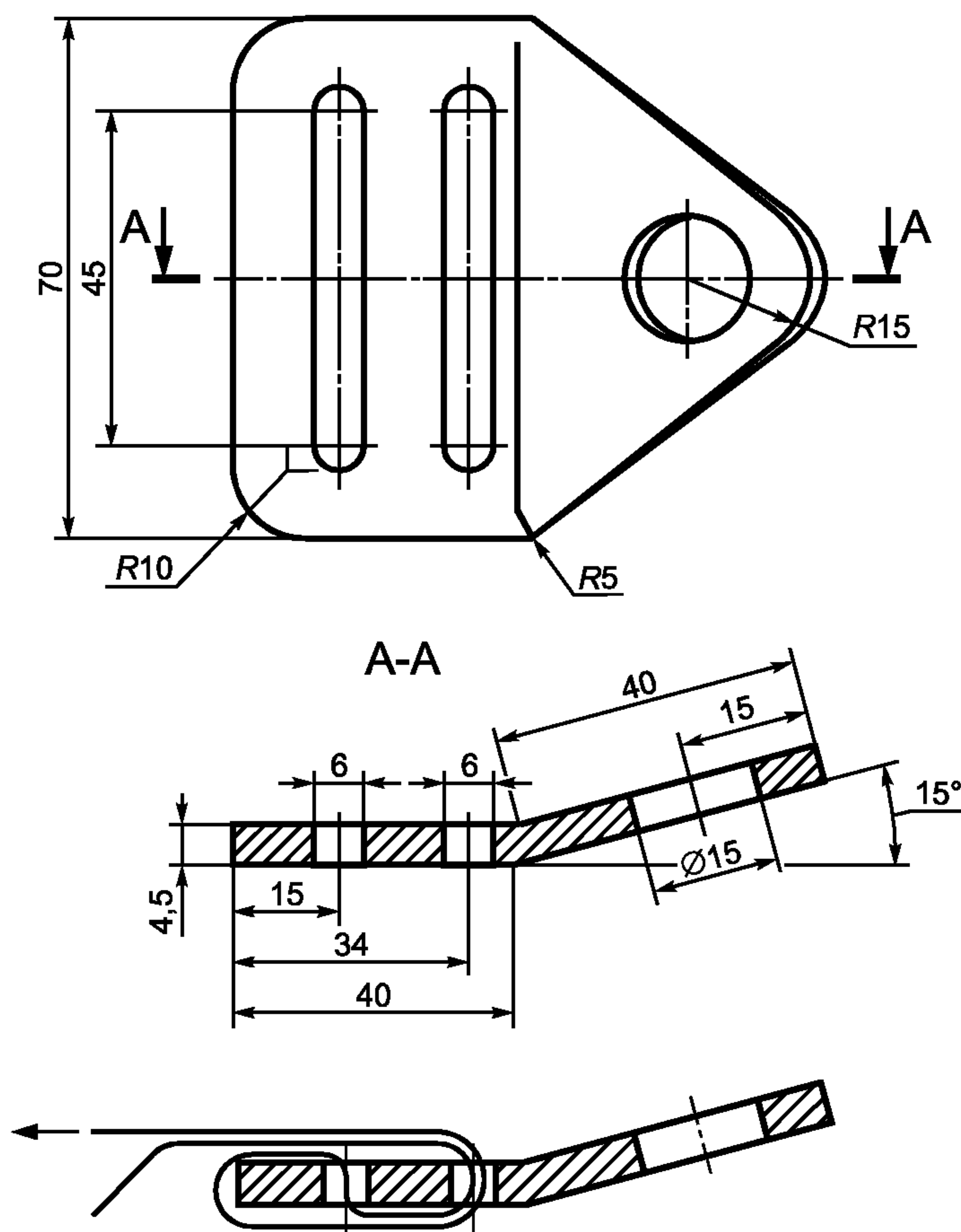
Рисунок П.2 — Стандартная пластина для крепления
