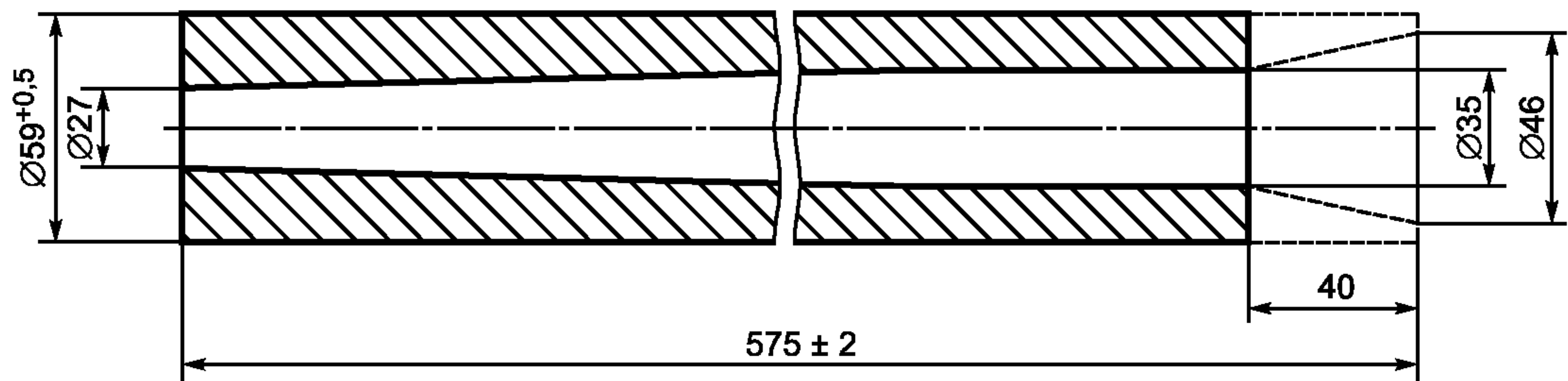
Рисунок Е.7 — Полиуретановая трубка из материала А
