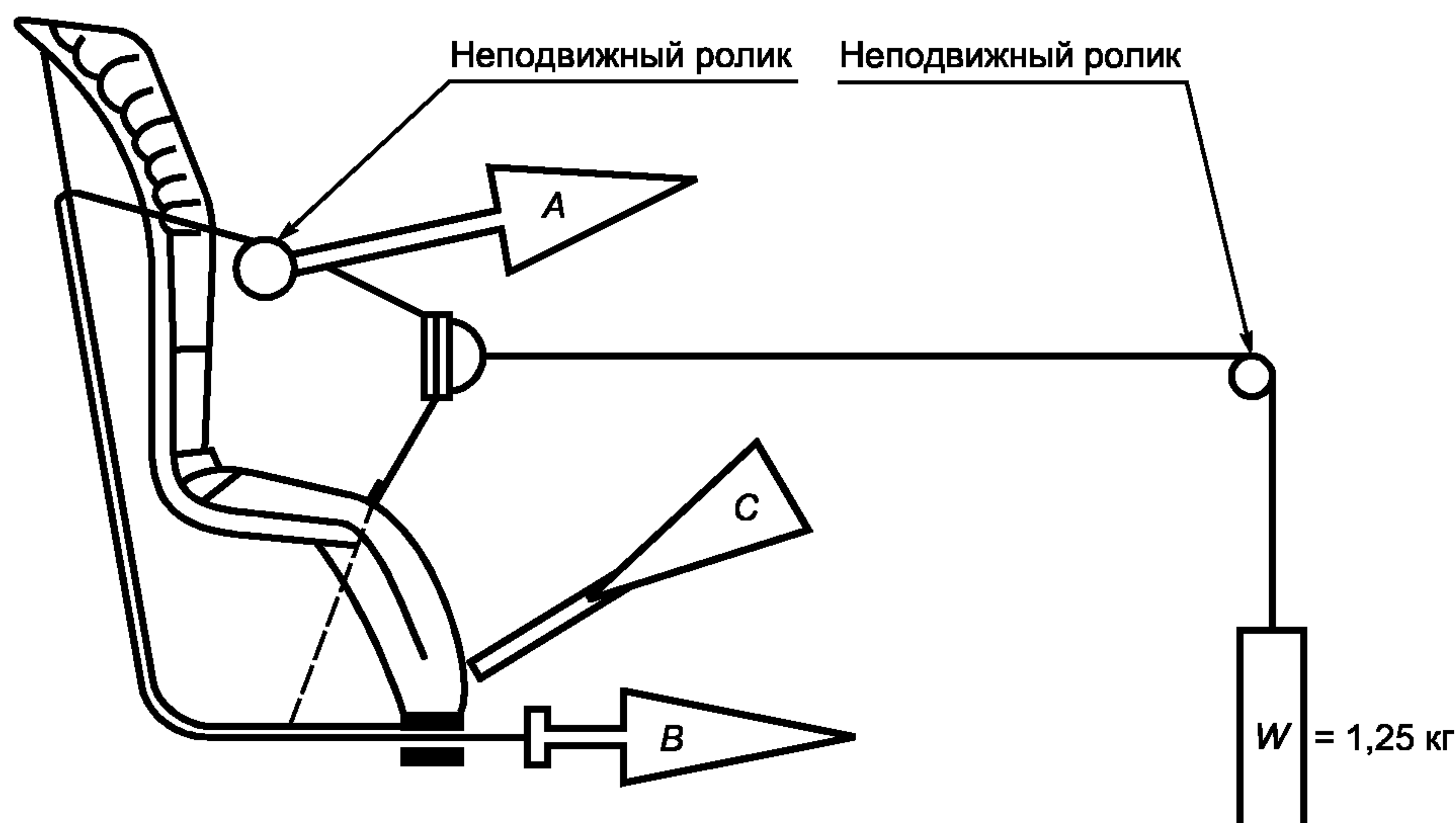
Рисунок X.1 — Схема испытательного устройства
