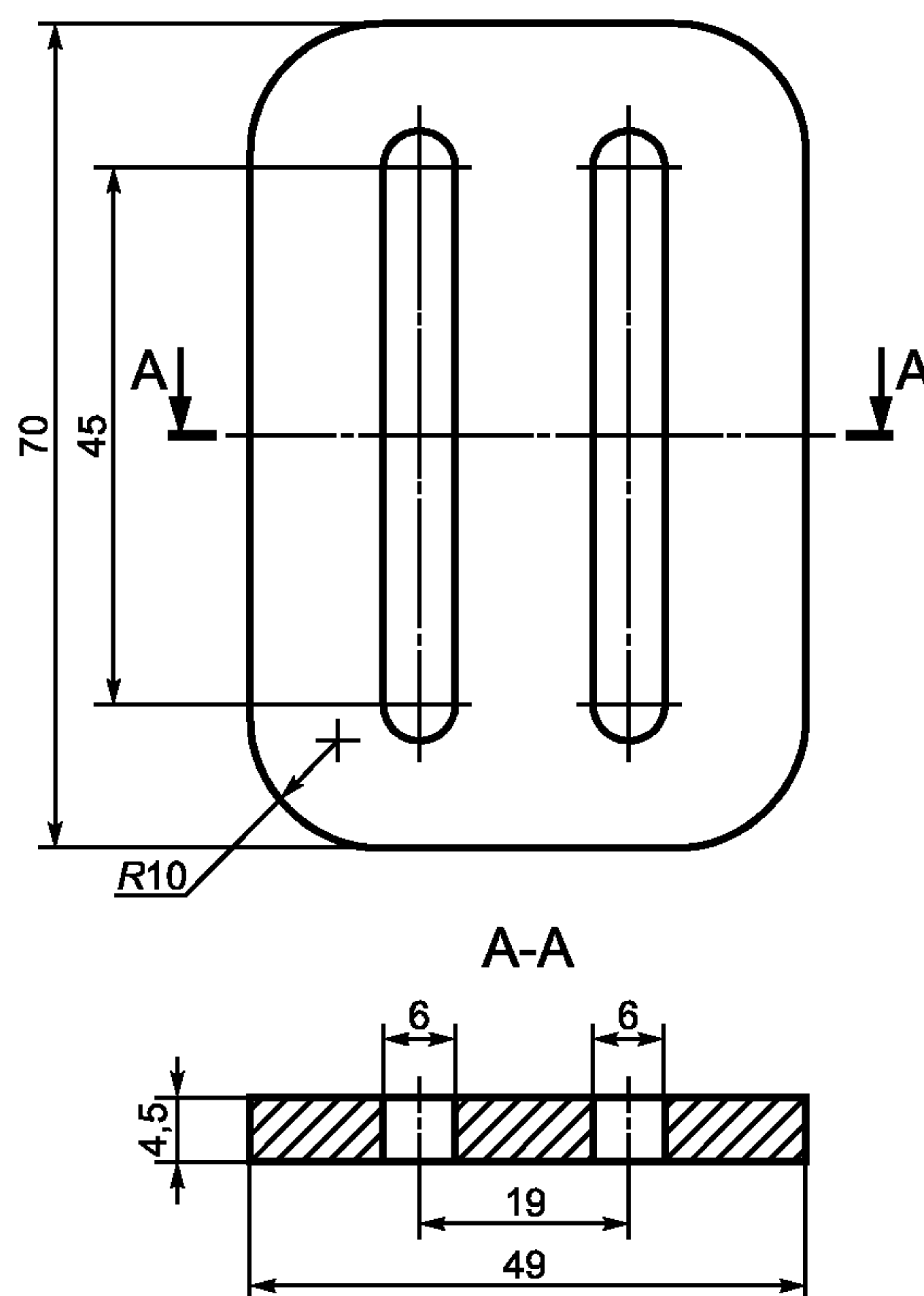
Рисунок П.3 — Центральная деталь стандартного ремня безопасности
