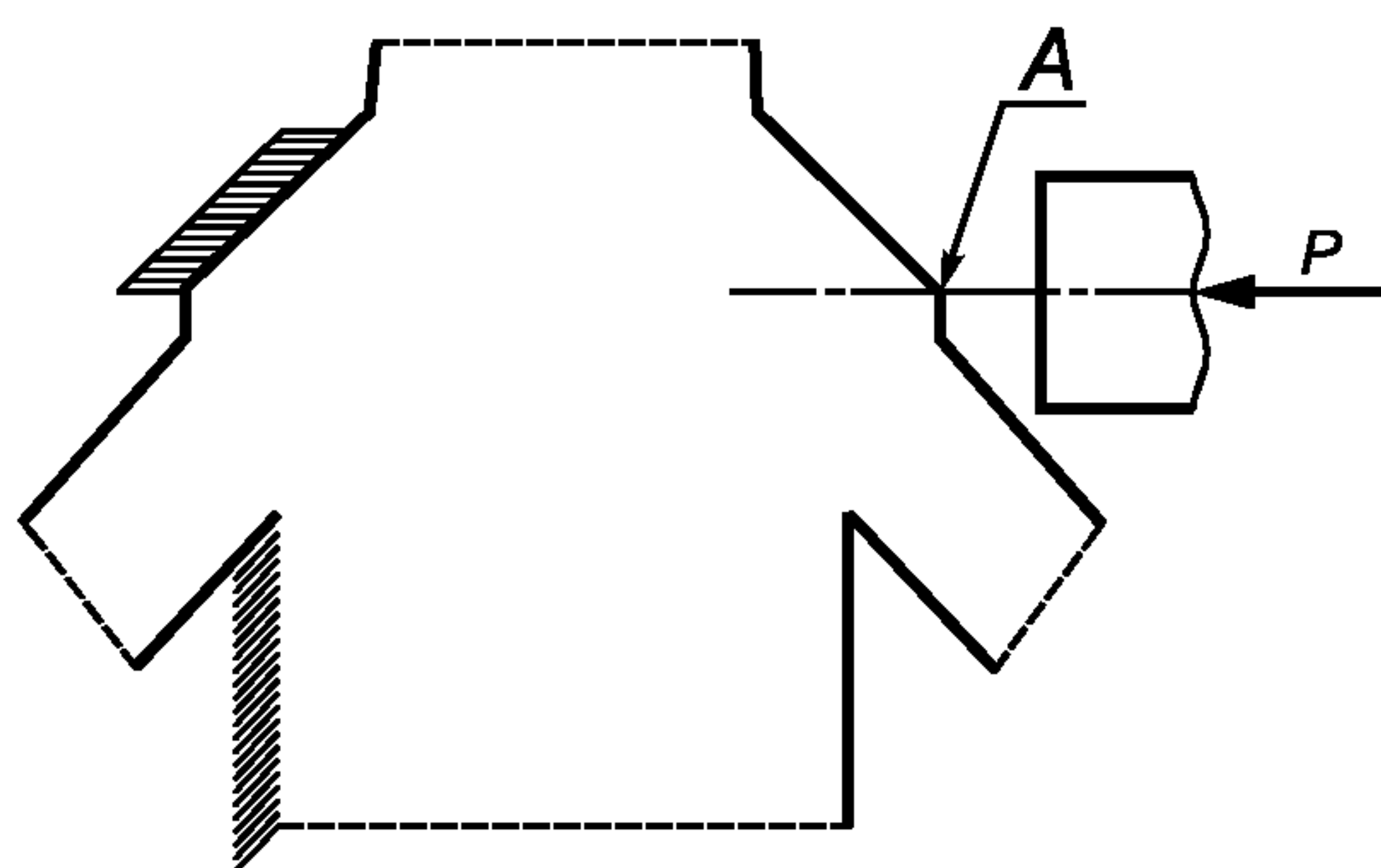
Рисунок И.11 — Калибровка жесткости плечевого сустава
