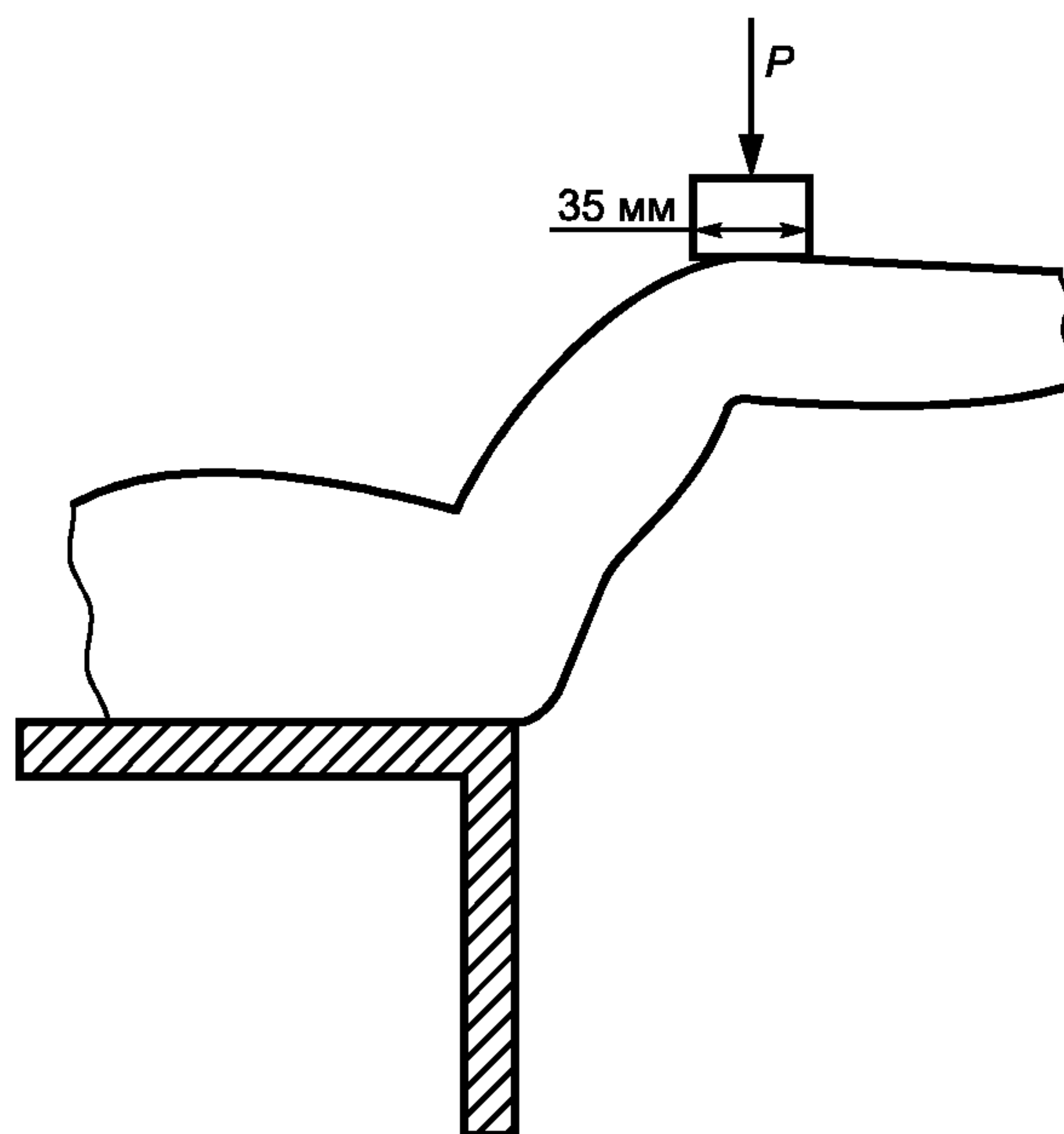
Рисунок И.12 — Калибровка жесткости сочленения ноги
