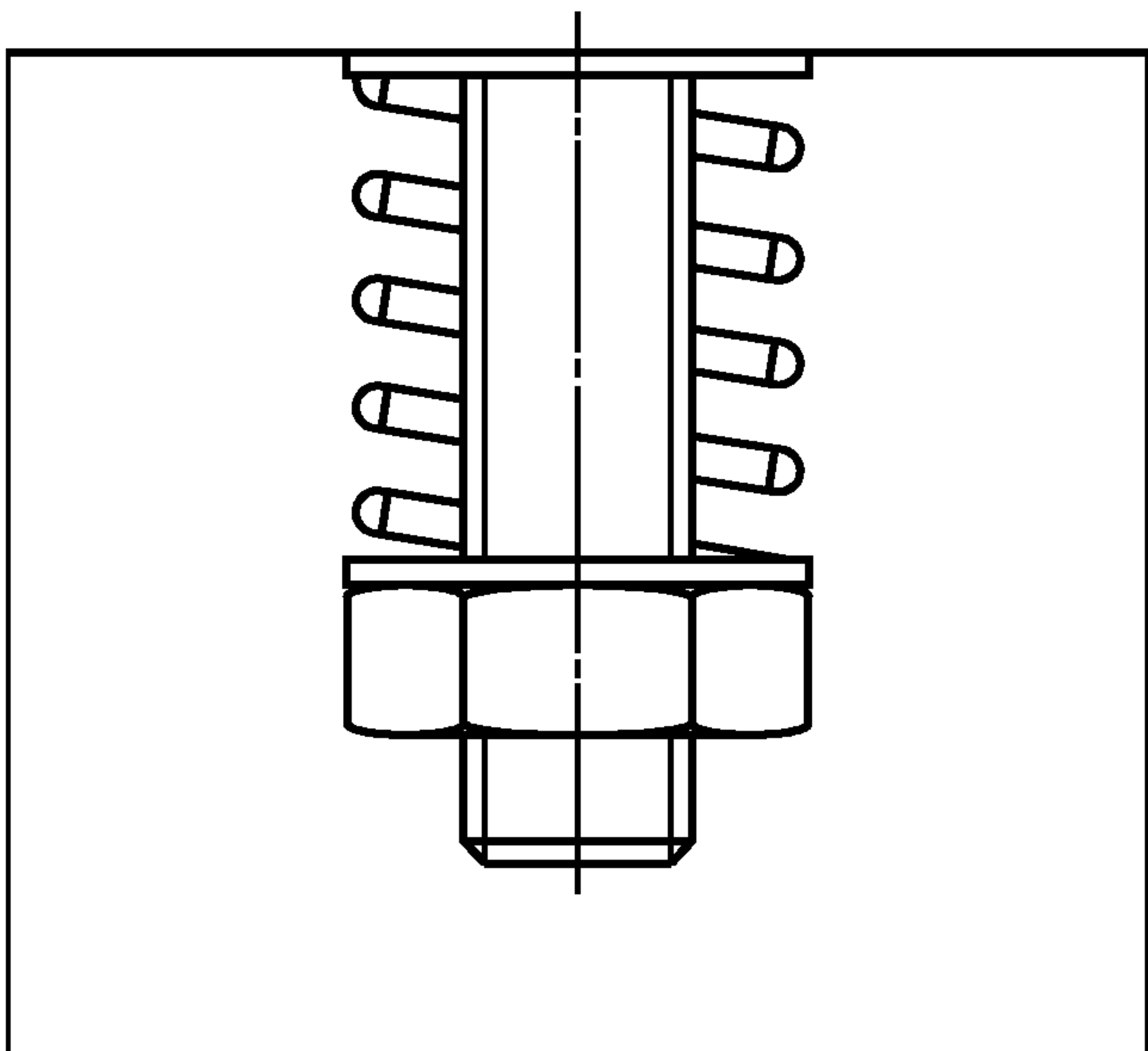
Рисунок И.8 — Регулирование поясничного троса
