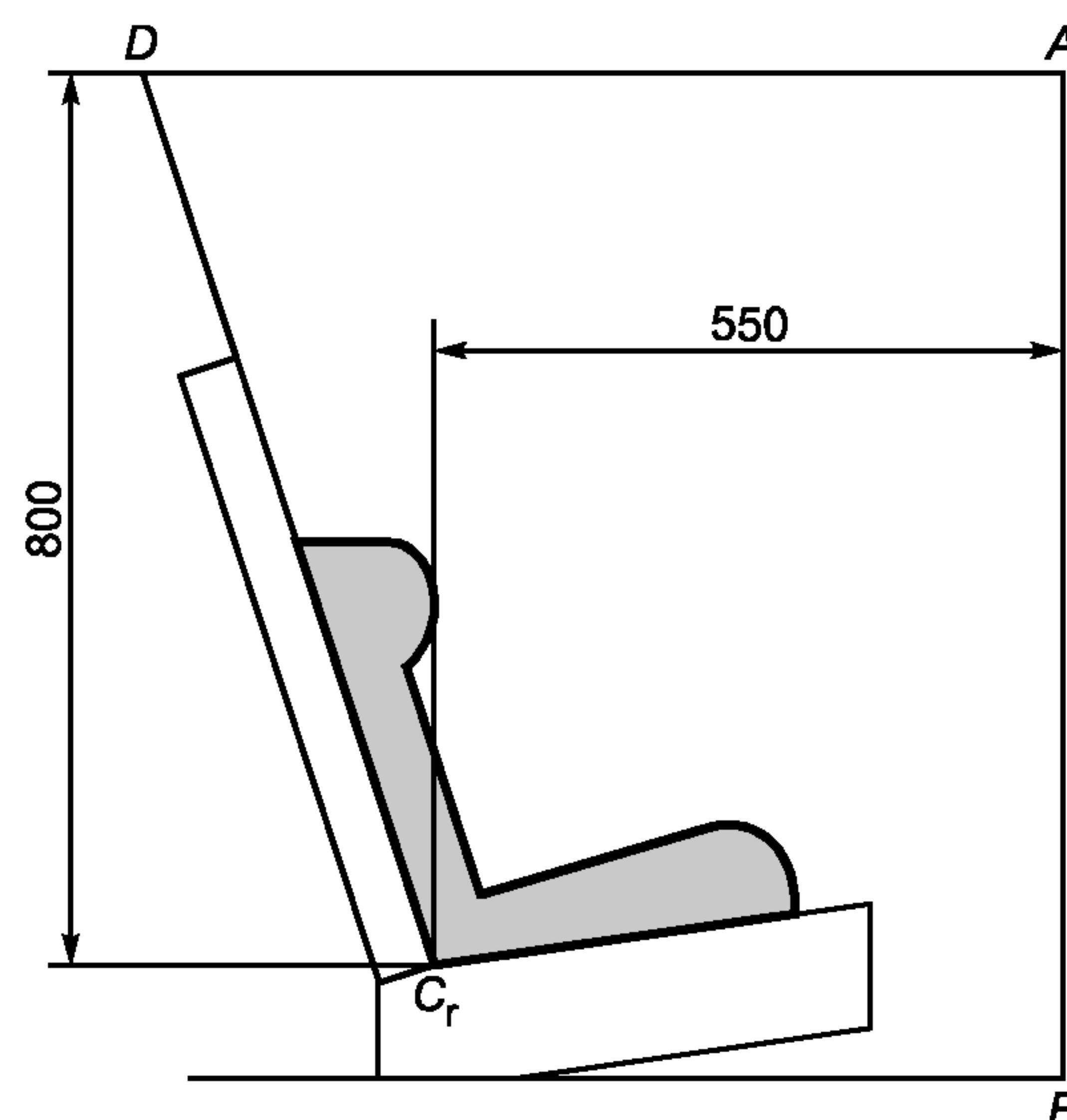
Рисунок 1 — Схема испытания детского удерживающего устройства, обращенного вперед
