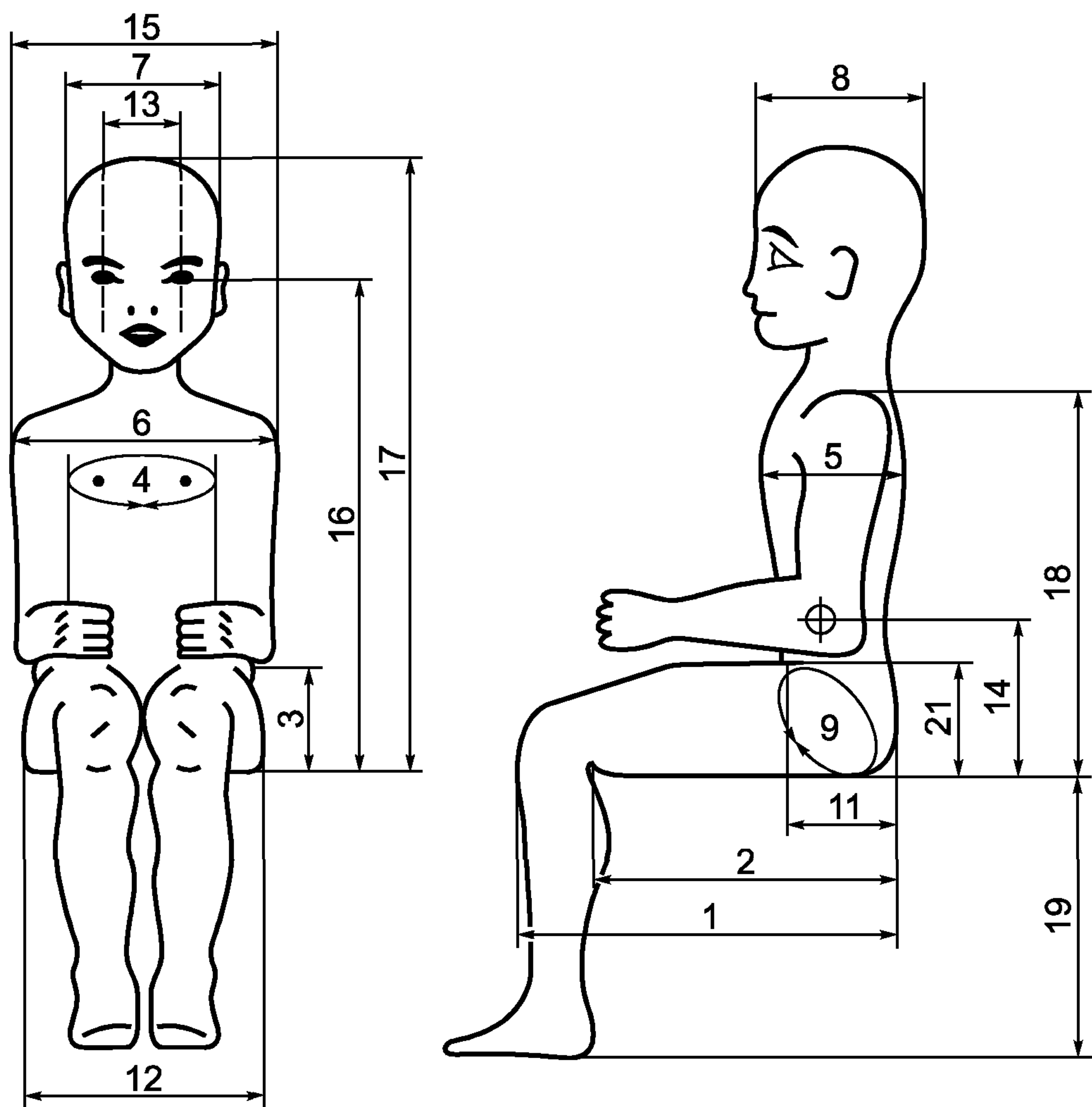
Рисунок И.13 — Основные размеры манекена 18-месячного ребенка
