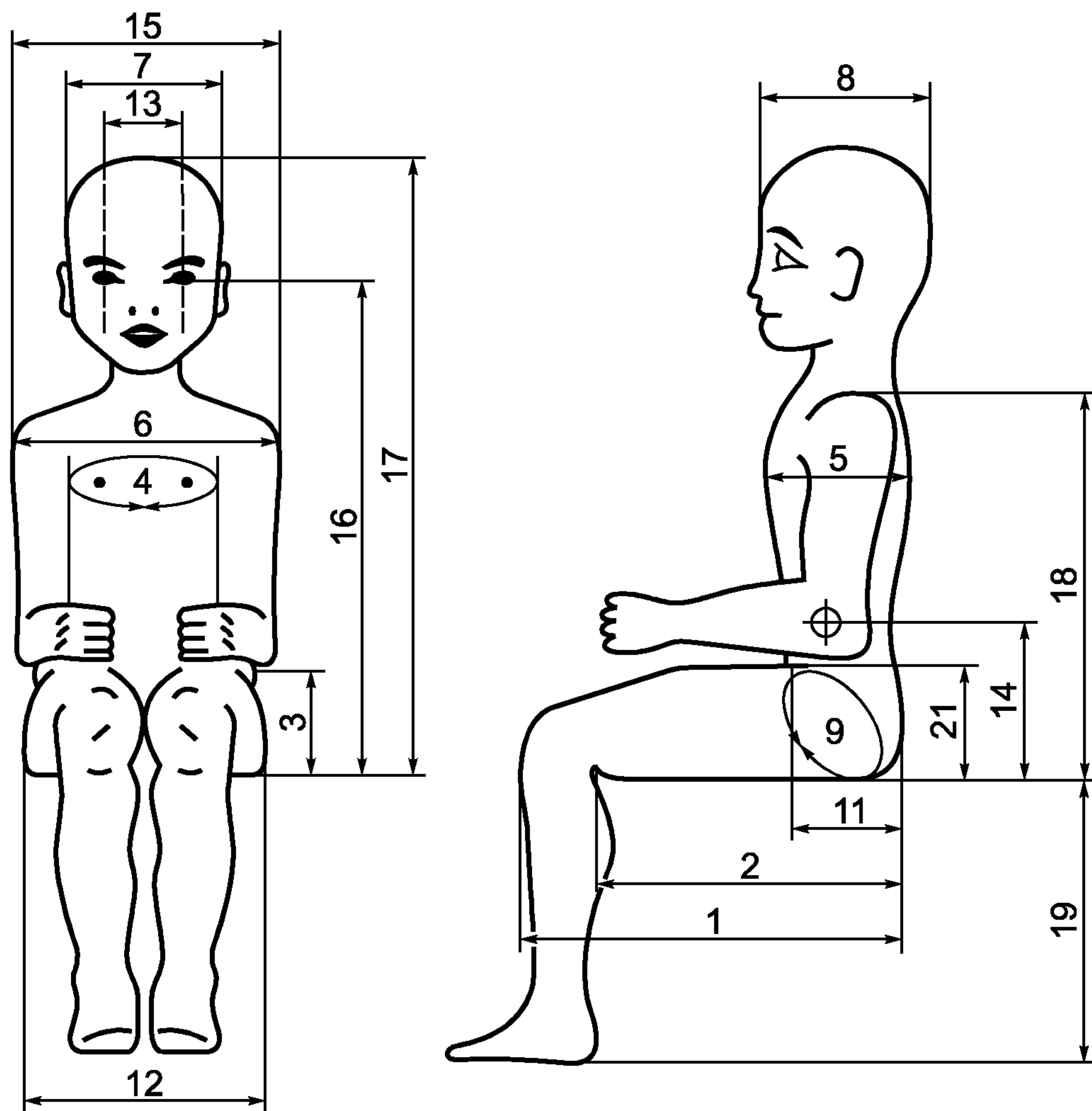
Рисунок И.1 — Основные размеры манекенов
