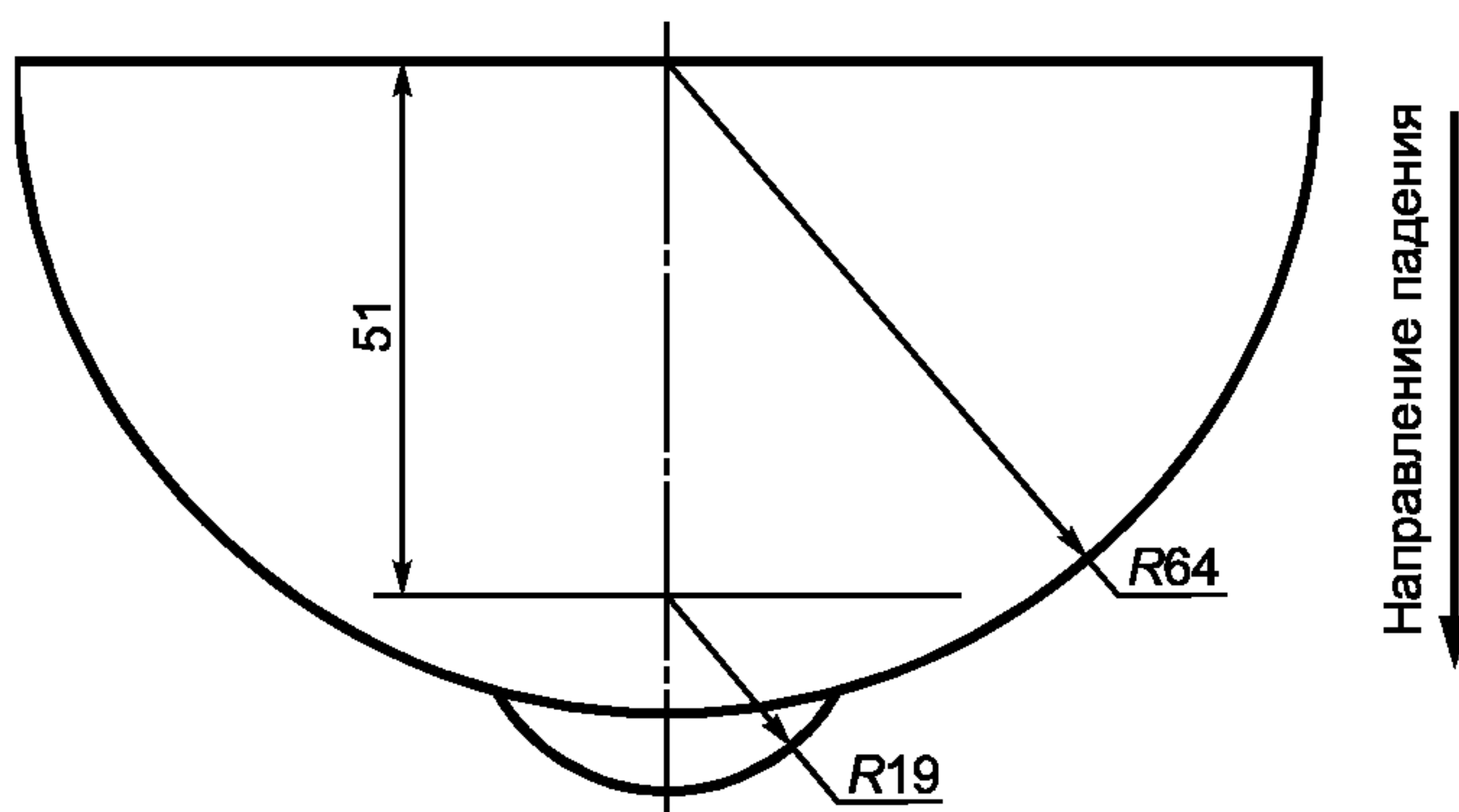
Рисунок Т.1 — Модель головы
