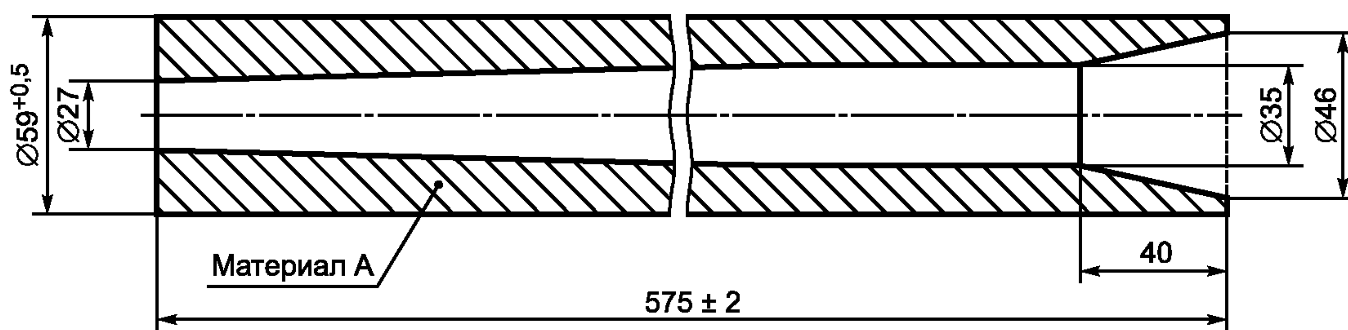
Рисунок Е.12 — Полиуретановая трубка
