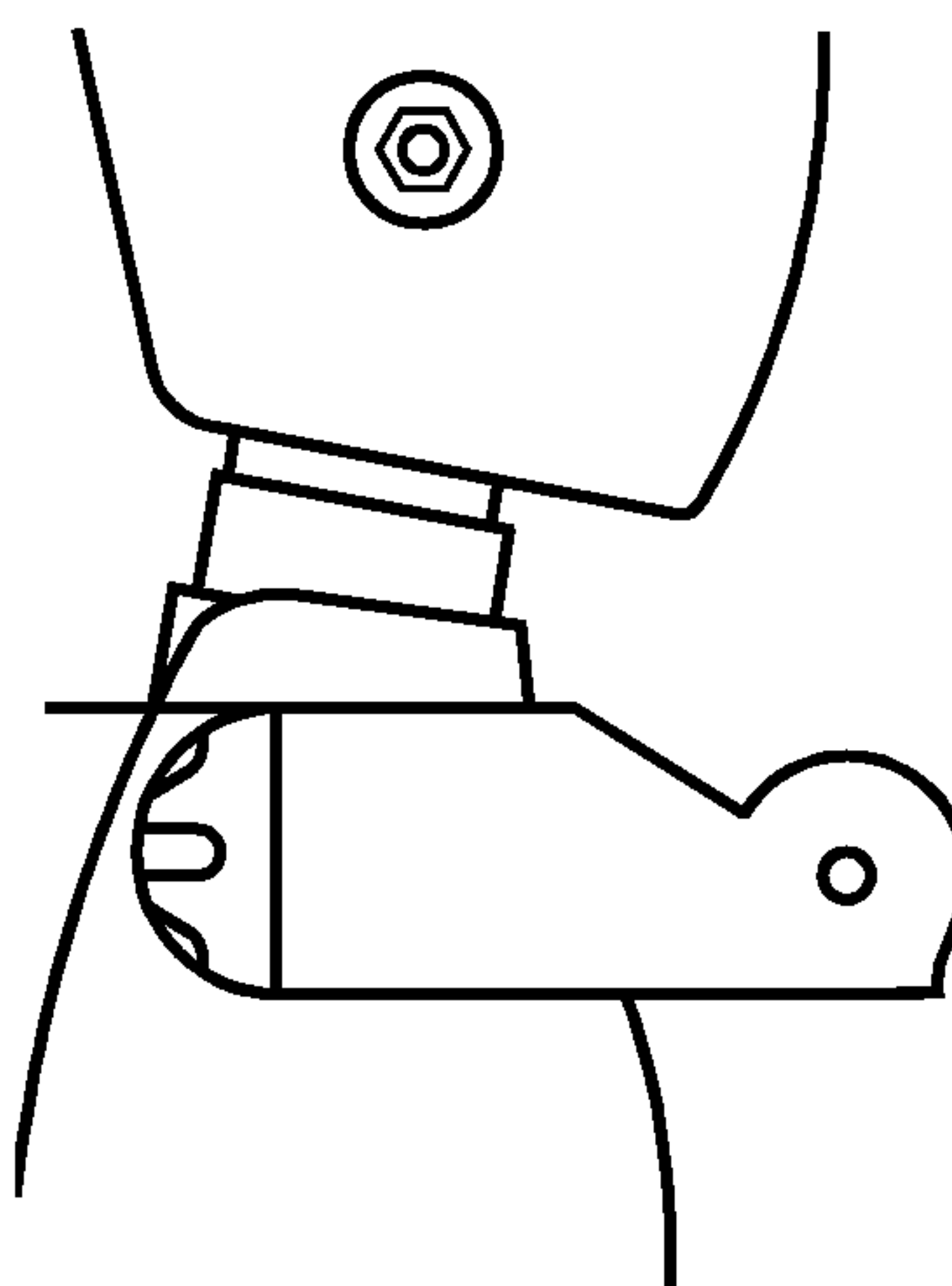
Рисунок И.6 — Регулирование плечевых сочленений
