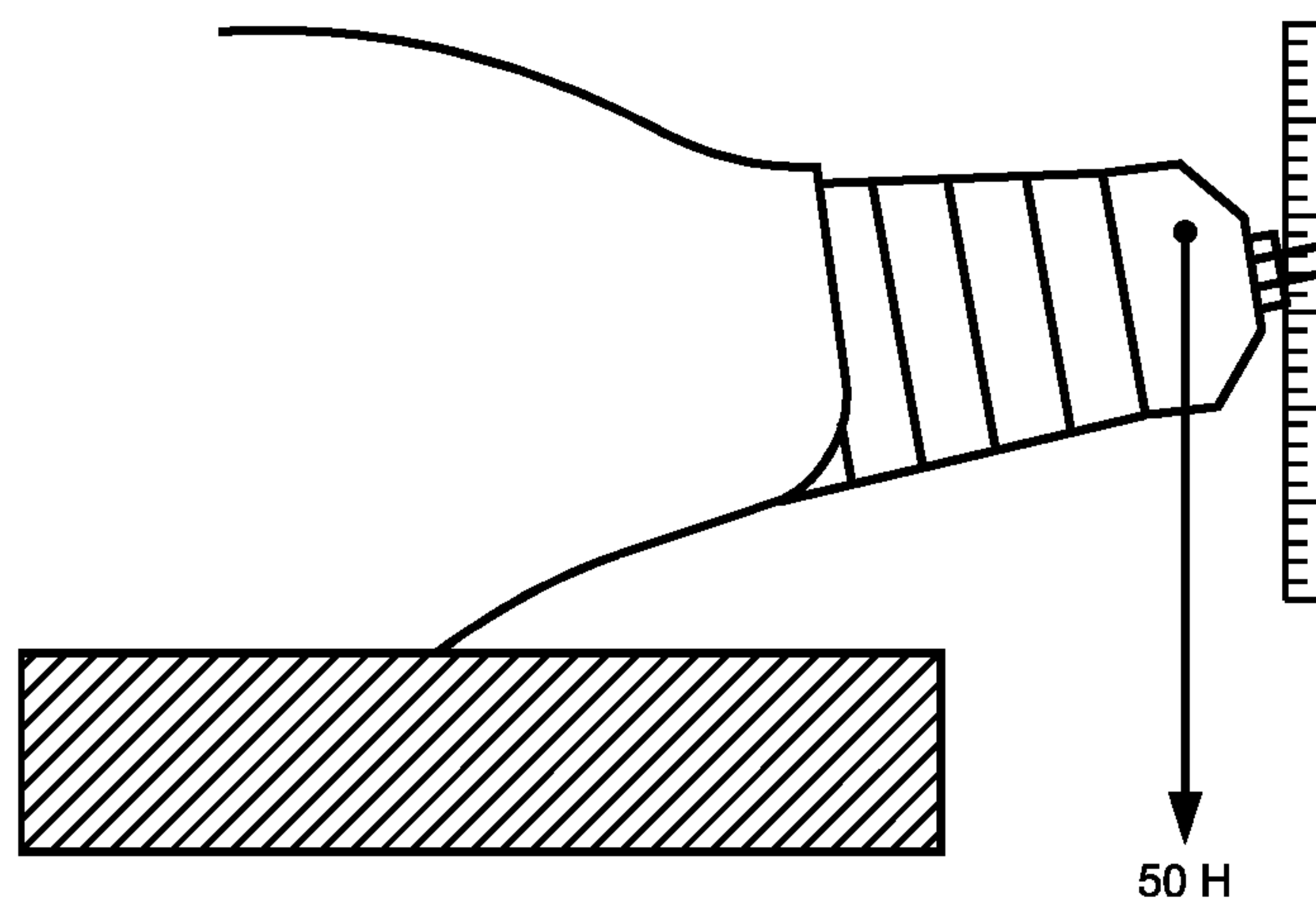
Рисунок И.2 — Регулирование троса шеи
