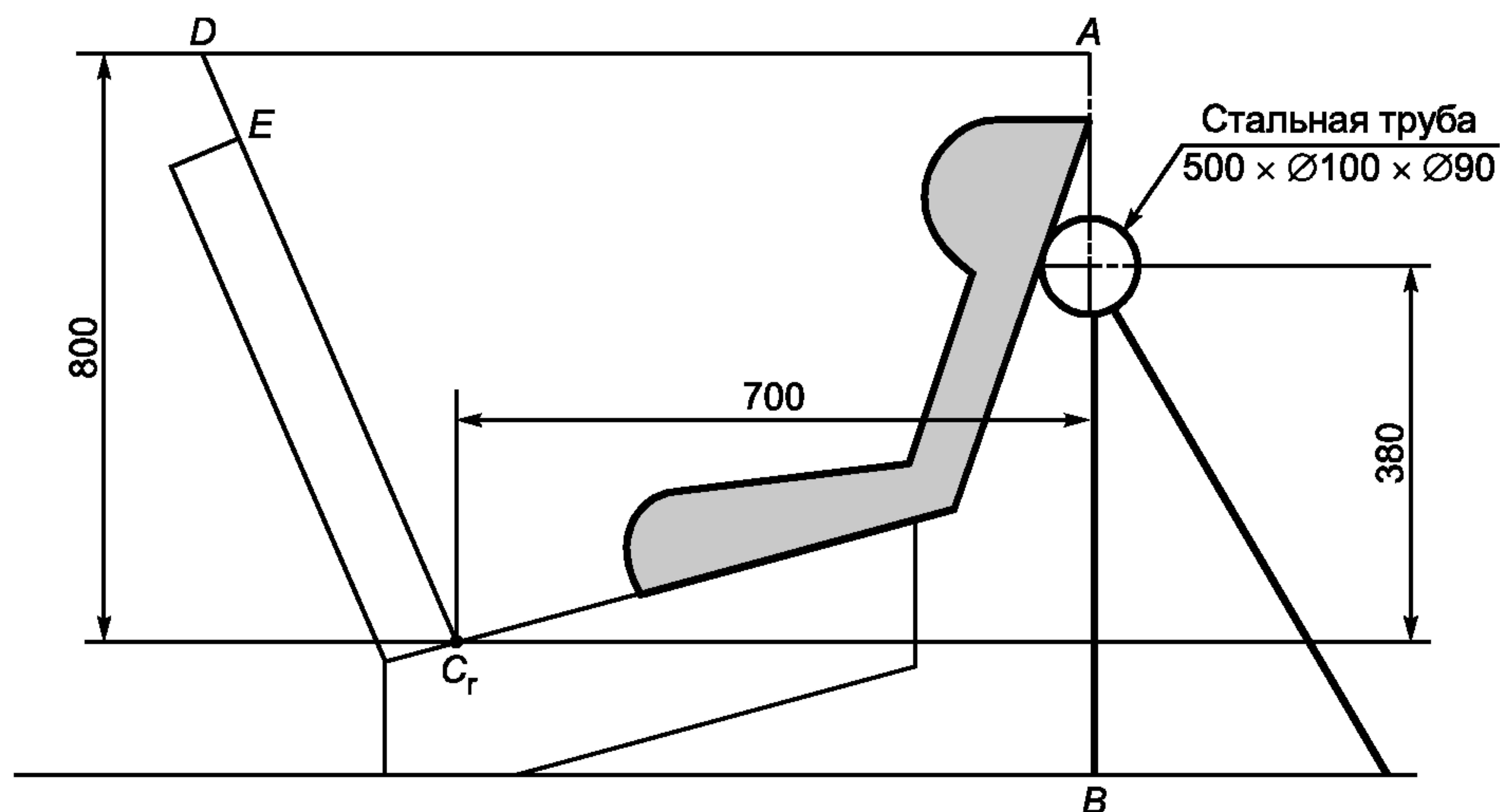
Рисунок 2 — Схема испытания детского удерживающего устройства, обращенного назад
