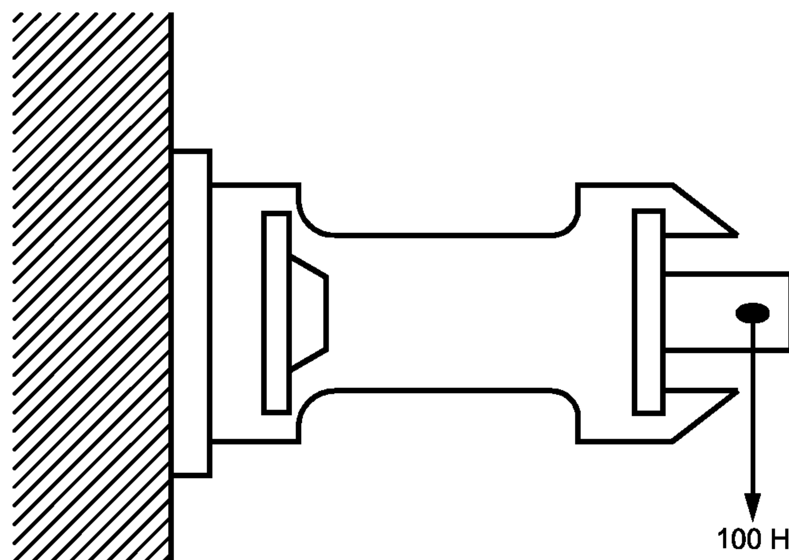
Рисунок И.16 — Монтаж элемента шеи в комплекте
