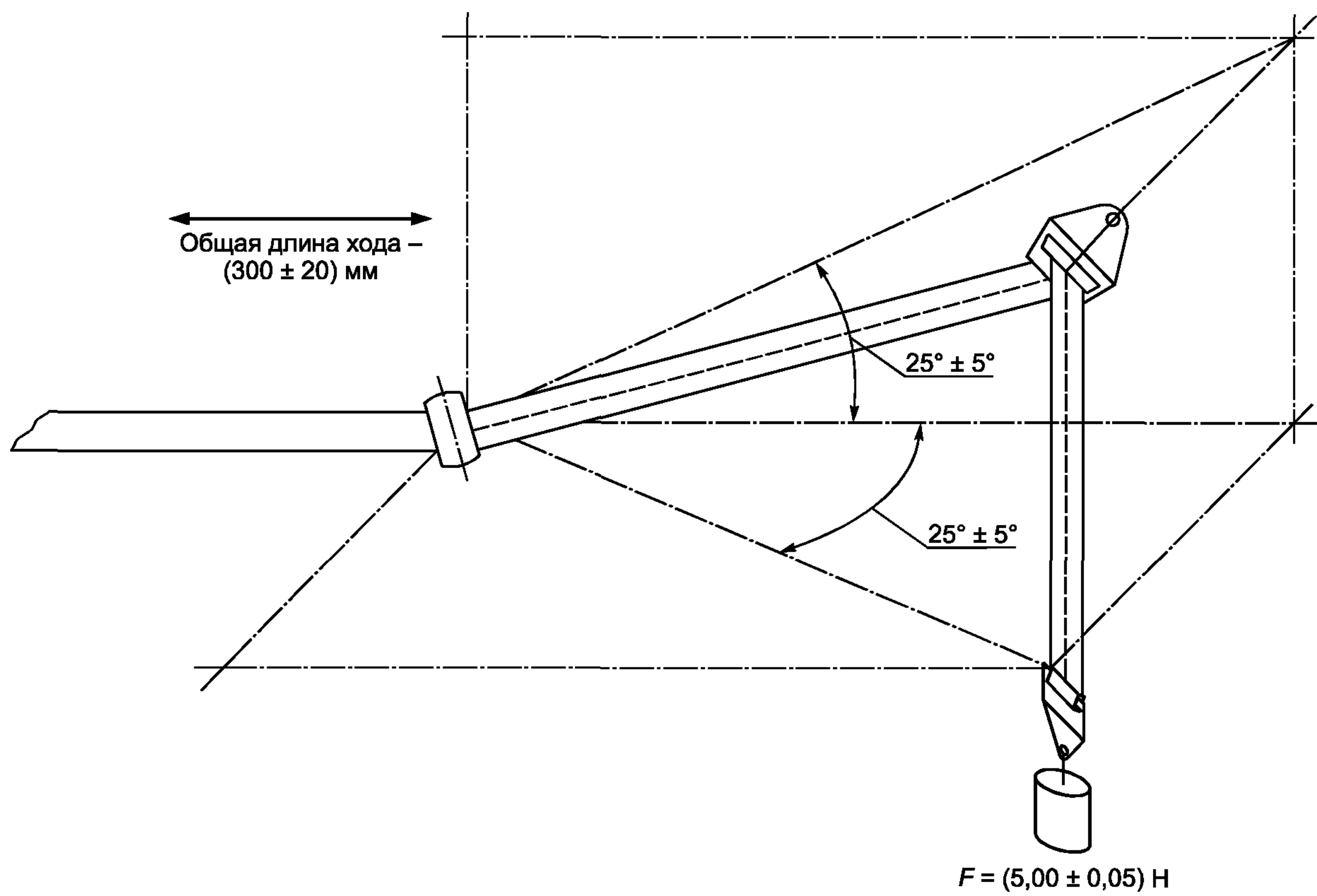
Рисунок Д.4 — Испытание с направляющим устройством
