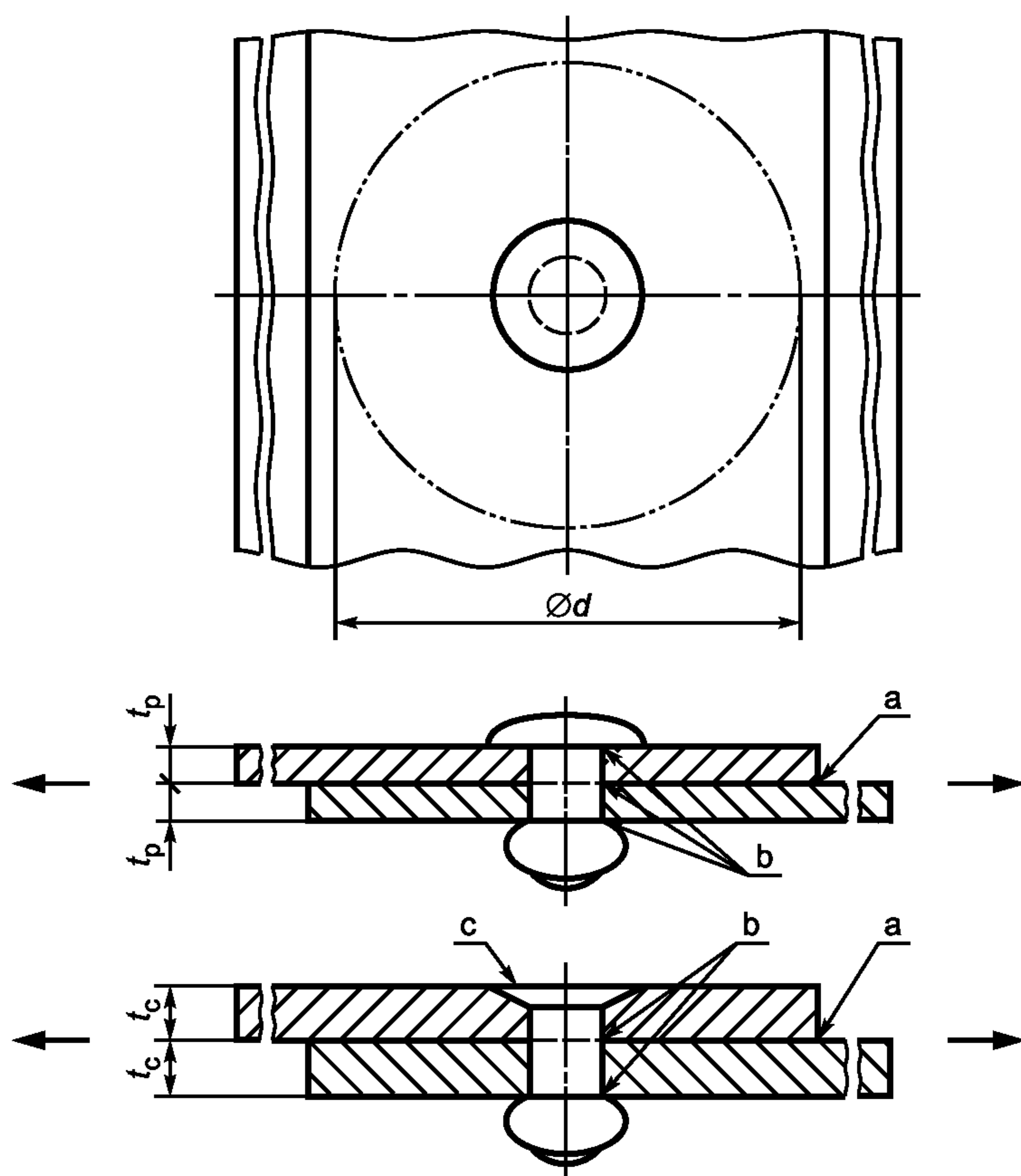
Рисунок 1 — Приспособление для обычных испытаний на срез
