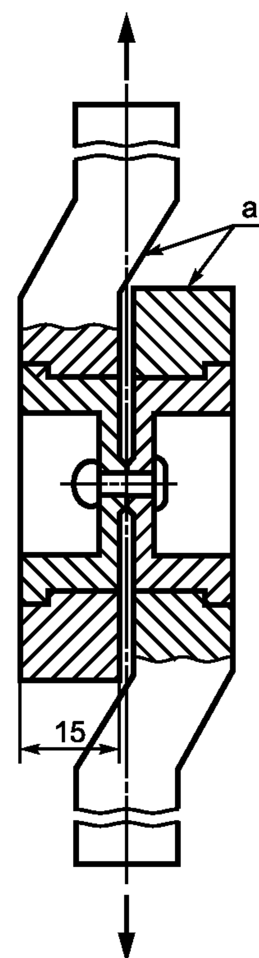
Рисунок 1 — Приспособление для обычных испытаний на срез
