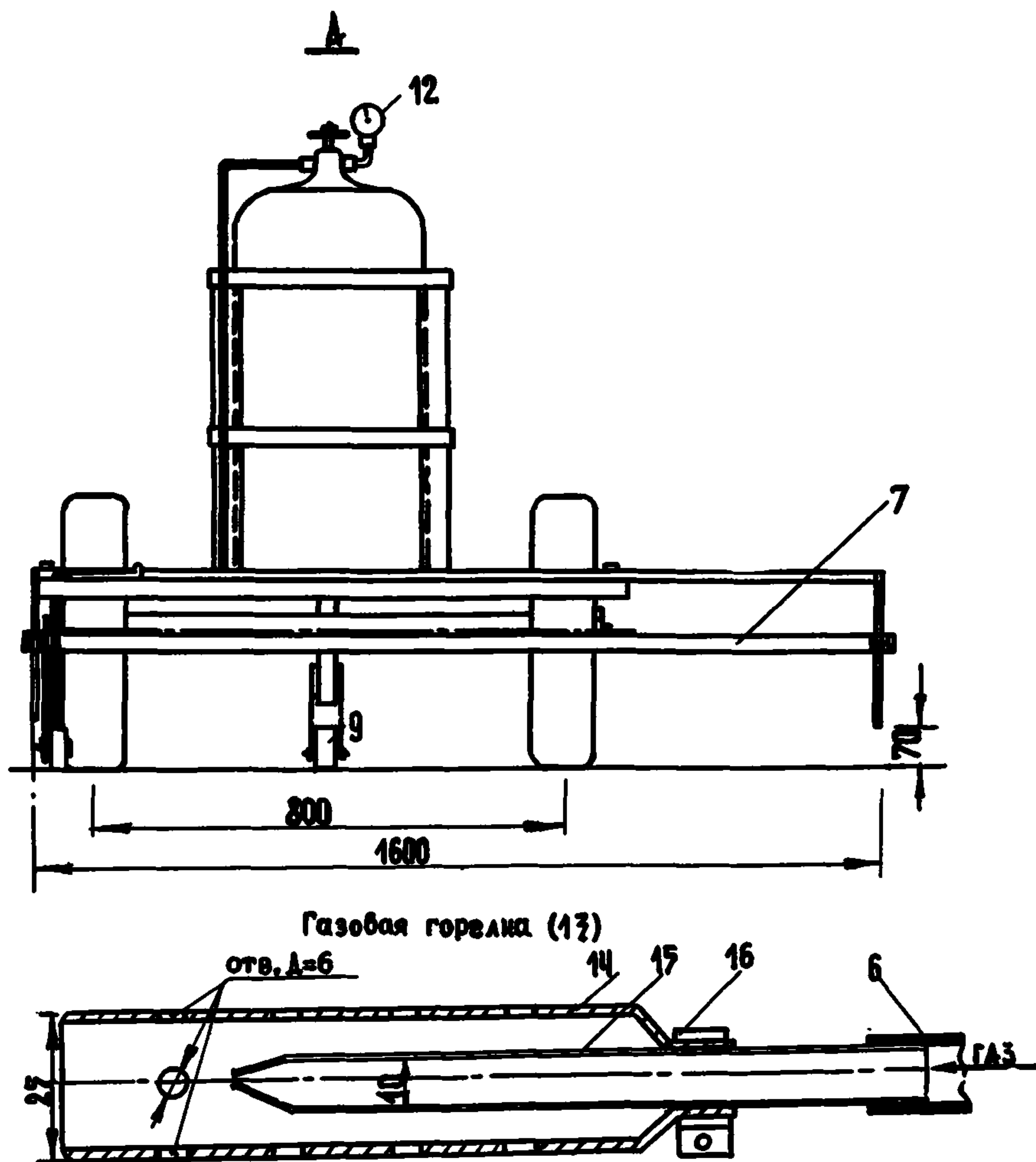
Рис. I2. Схема установки для соединения полотен синтетических материалов:
