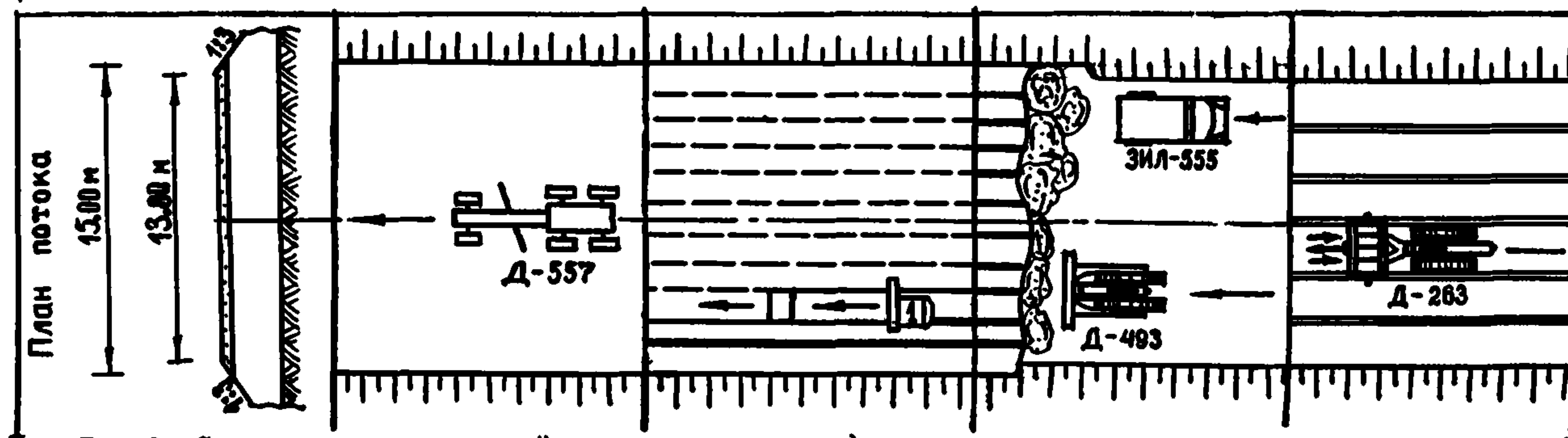
Рис.2. Схема потока по устройству земляного полотна с армированием его верха синтетическим материалом
