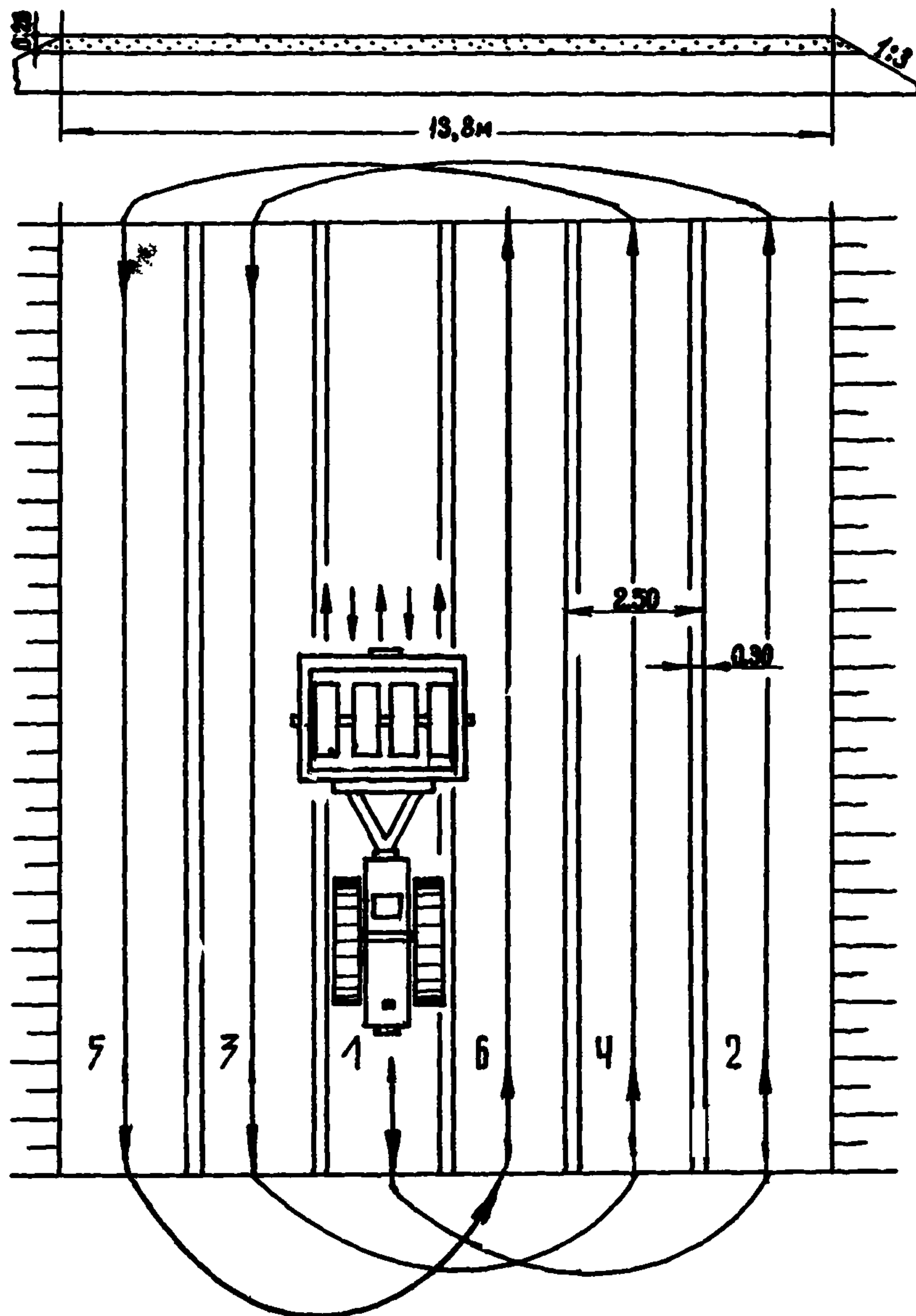
Рис.6. Схема работы катка по уплотнению: I-6 - номера проходов катка
