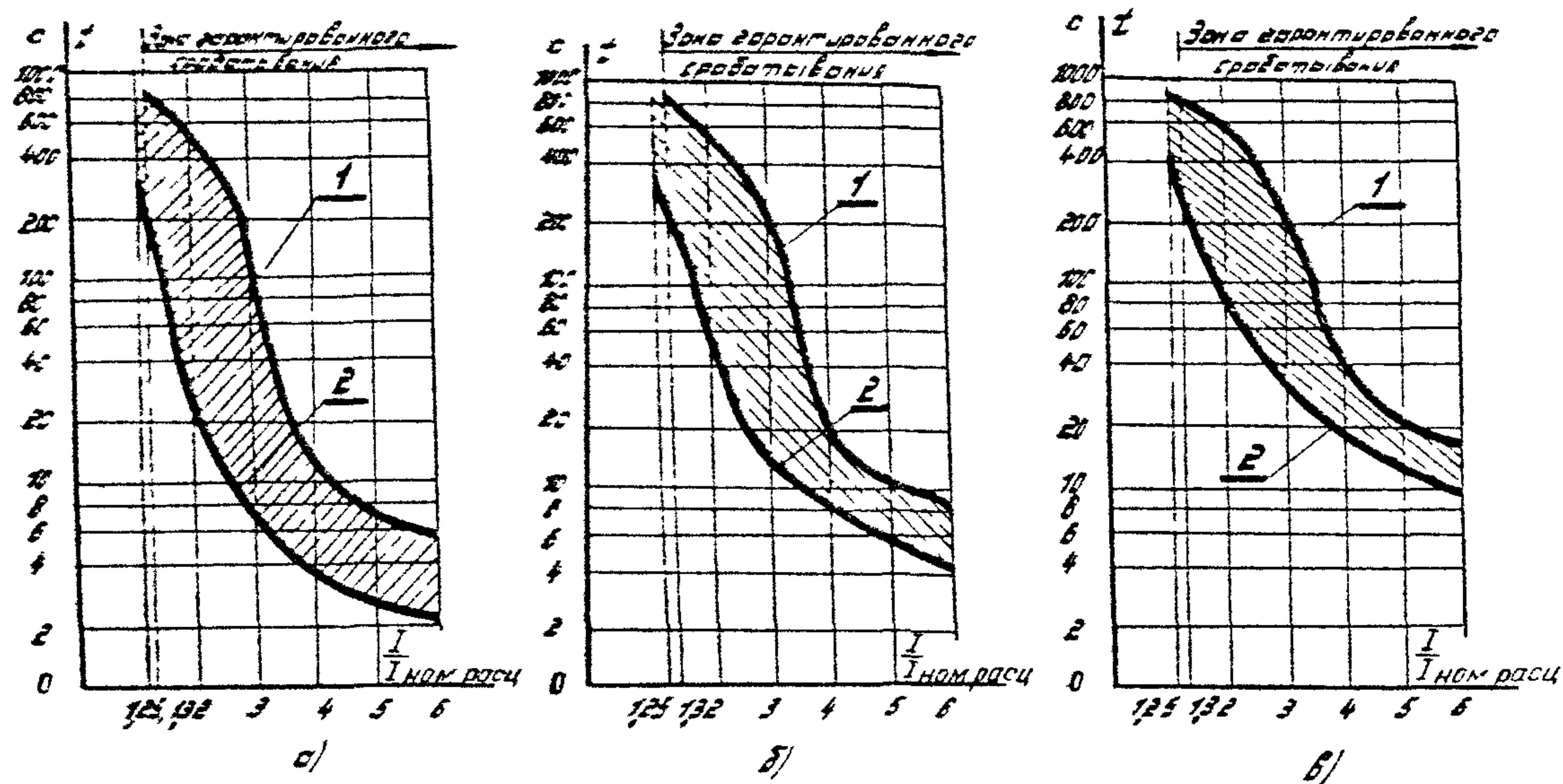
Рис.10. Защитные характеристики полупроводникового распелителя постоянного тока при уставке времени срабатывания:
