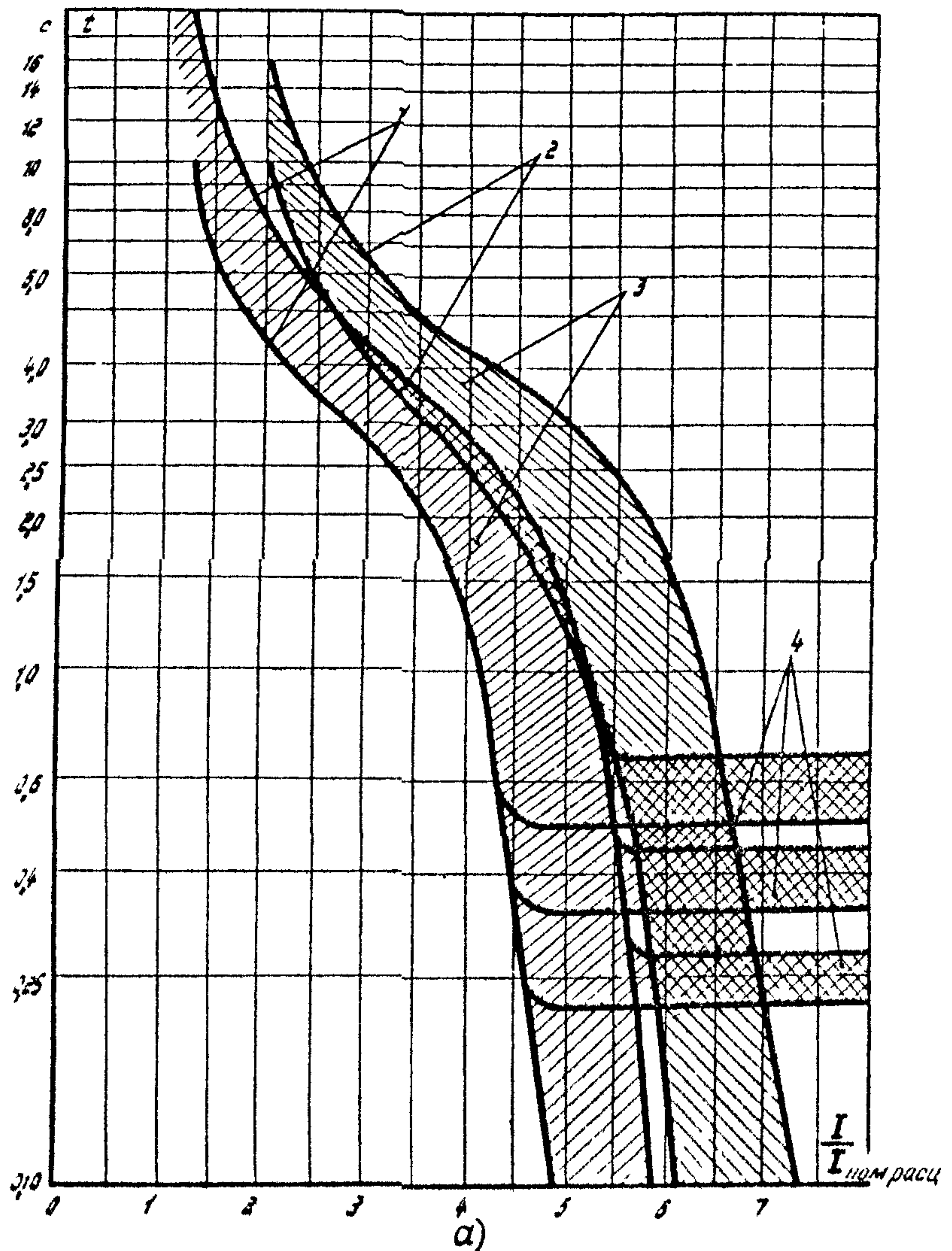
Рис.6. Защитные характеристики выключателей: а - АВМ 16Н и АВМ 16С, АВМ 20Н и АВМ 20С с номинальным током срабатывания МТЗ 1500 А; б - АВМ 20Н и АВМ 20С с номинальным током срабатывания МТЗ 1800 А I - при минимальных уставках на шкалах замедленного и мгновенного срабатывания электромагнитного максимального расцепителя тока;
