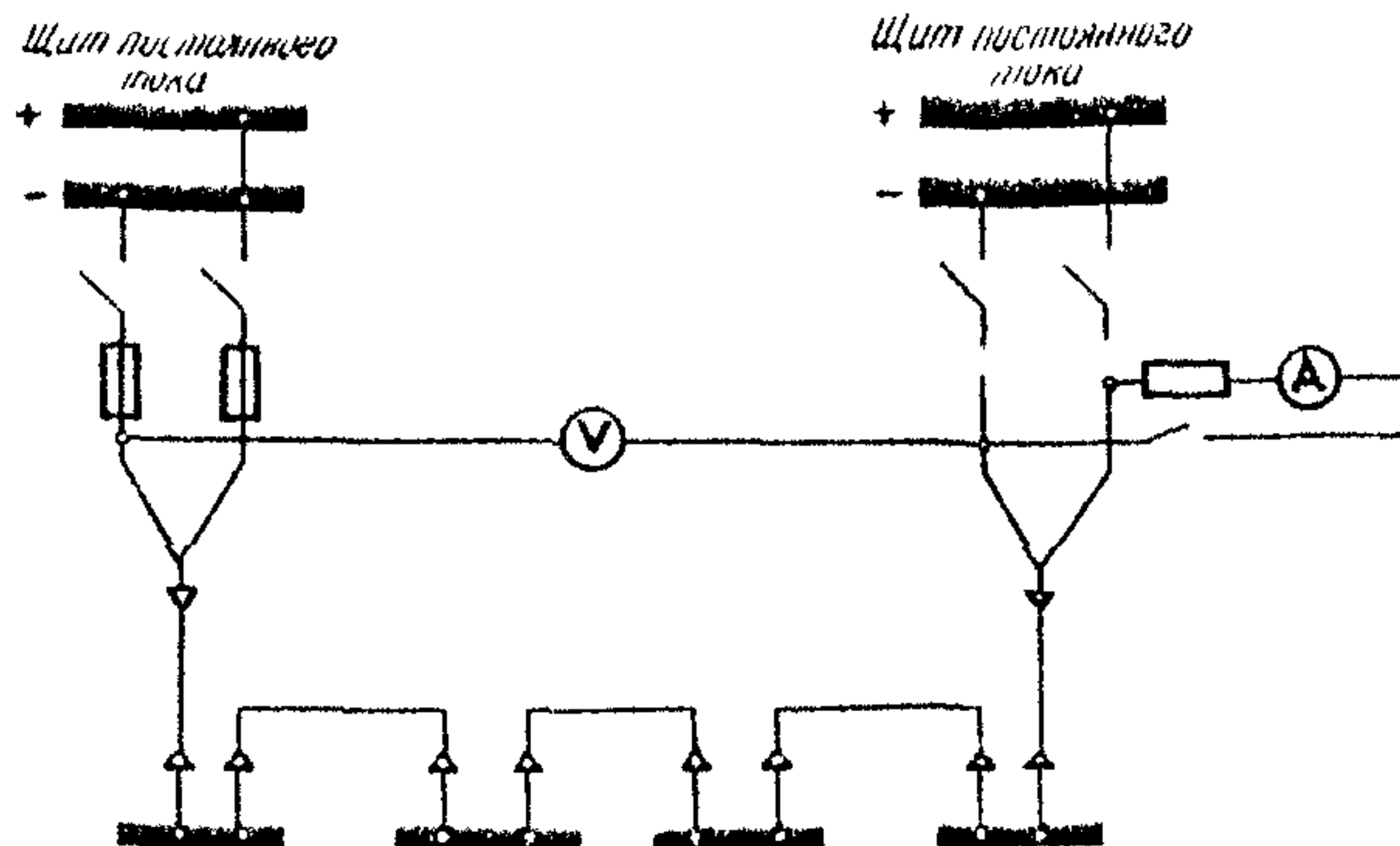
Рис.3. Принципиальная схема измерения сопротивлений "кольца" постоянного тока
