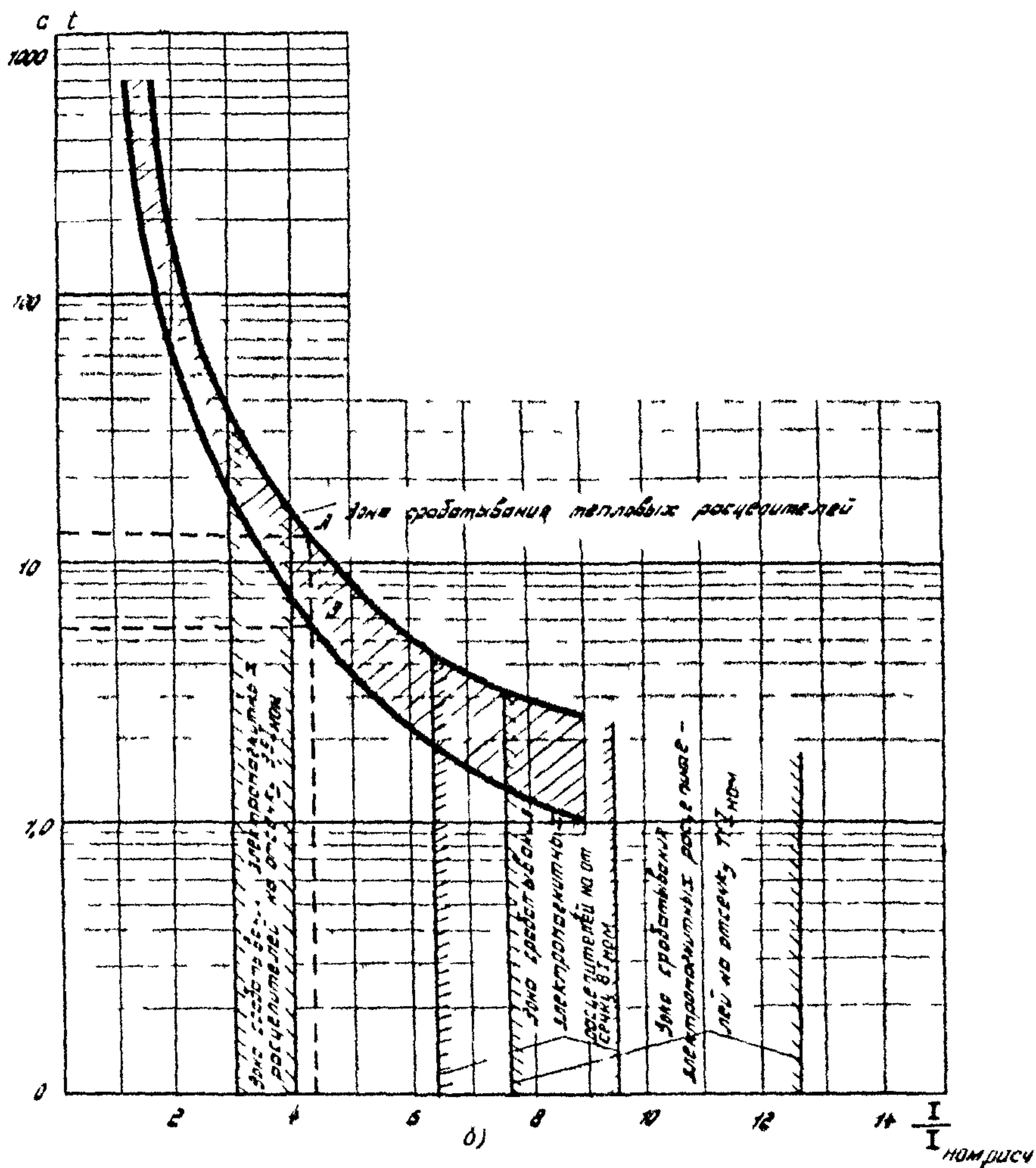
Рис.14. Время-токовые характеристики выключателя серии АП-50 на номинальный ток: \alpha - 10 А; \delta - 16 А
