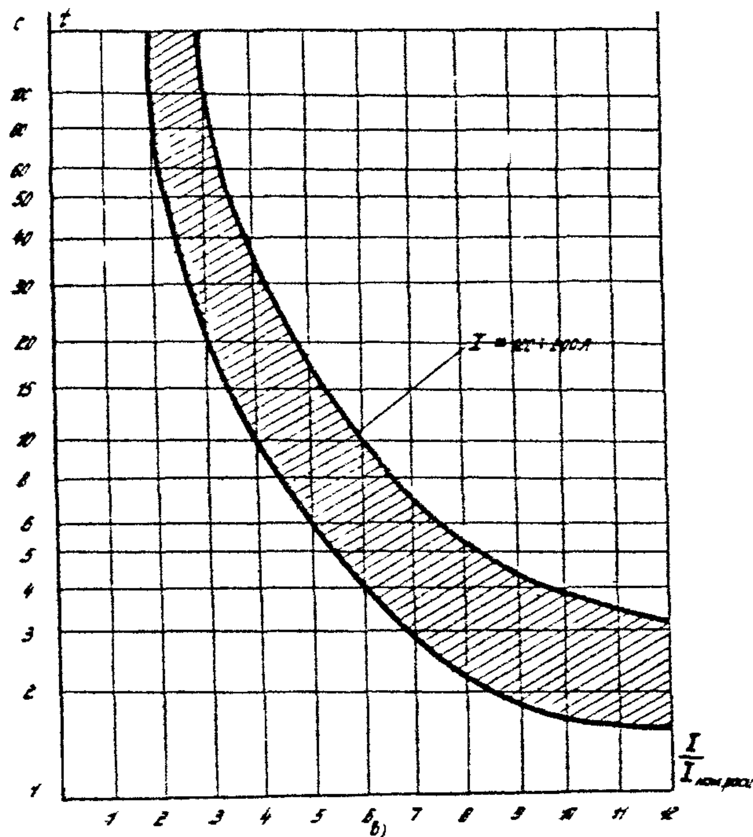
Рис. II. Время-токовая характеристика срабатывания выключателей: а - АЗИ10; б - АЗИ20; в - АЗИ30; г - АЗИ40
