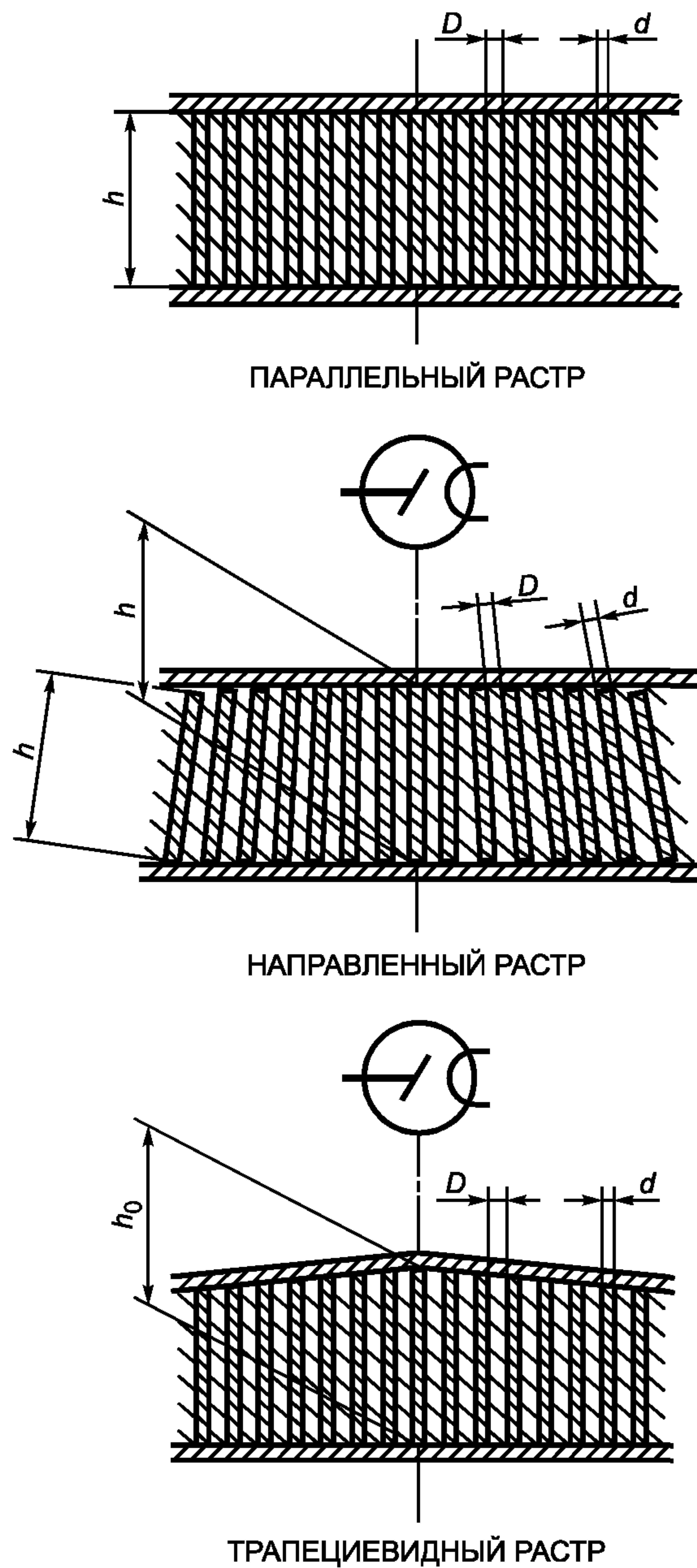
Рисунок 1 — Конструкция ОТСЕИВАЮЩИХ РАСТРОВ
