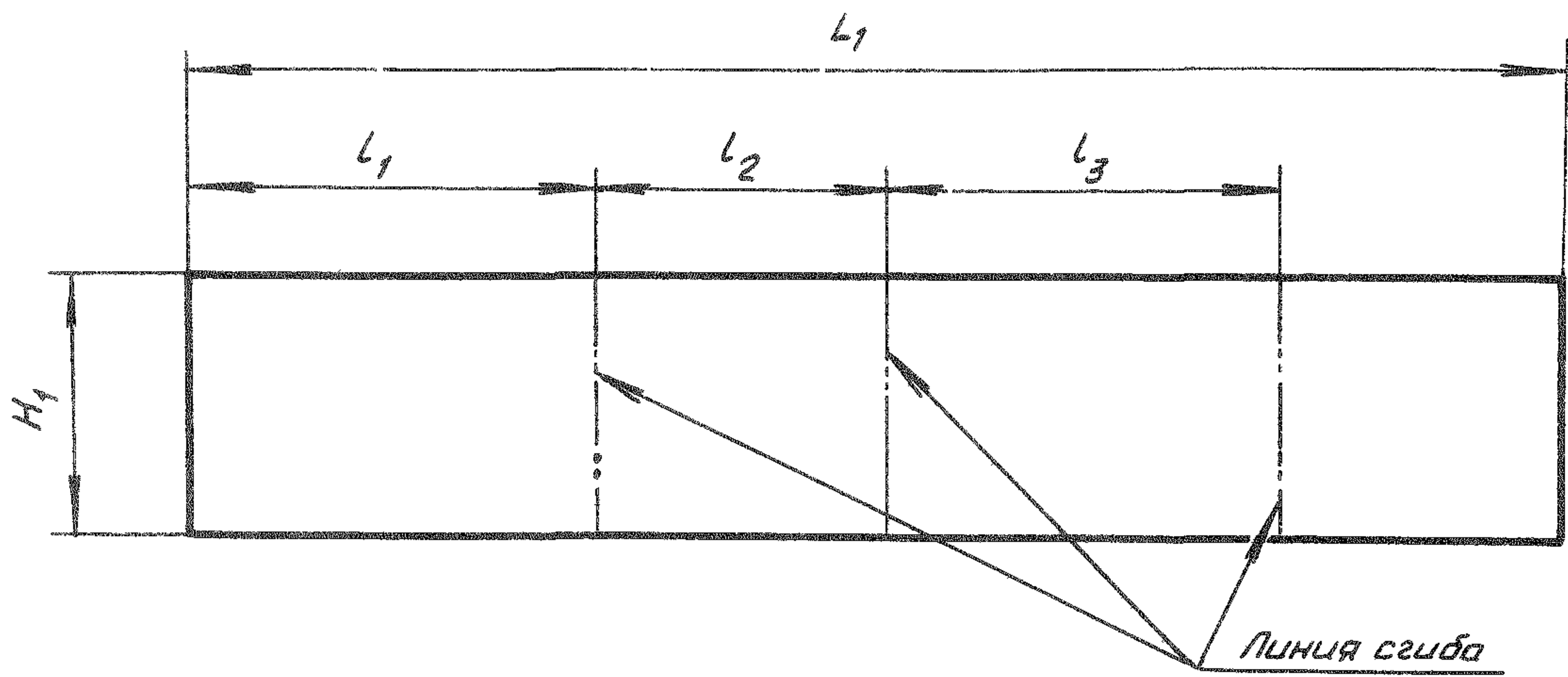
Развертка
