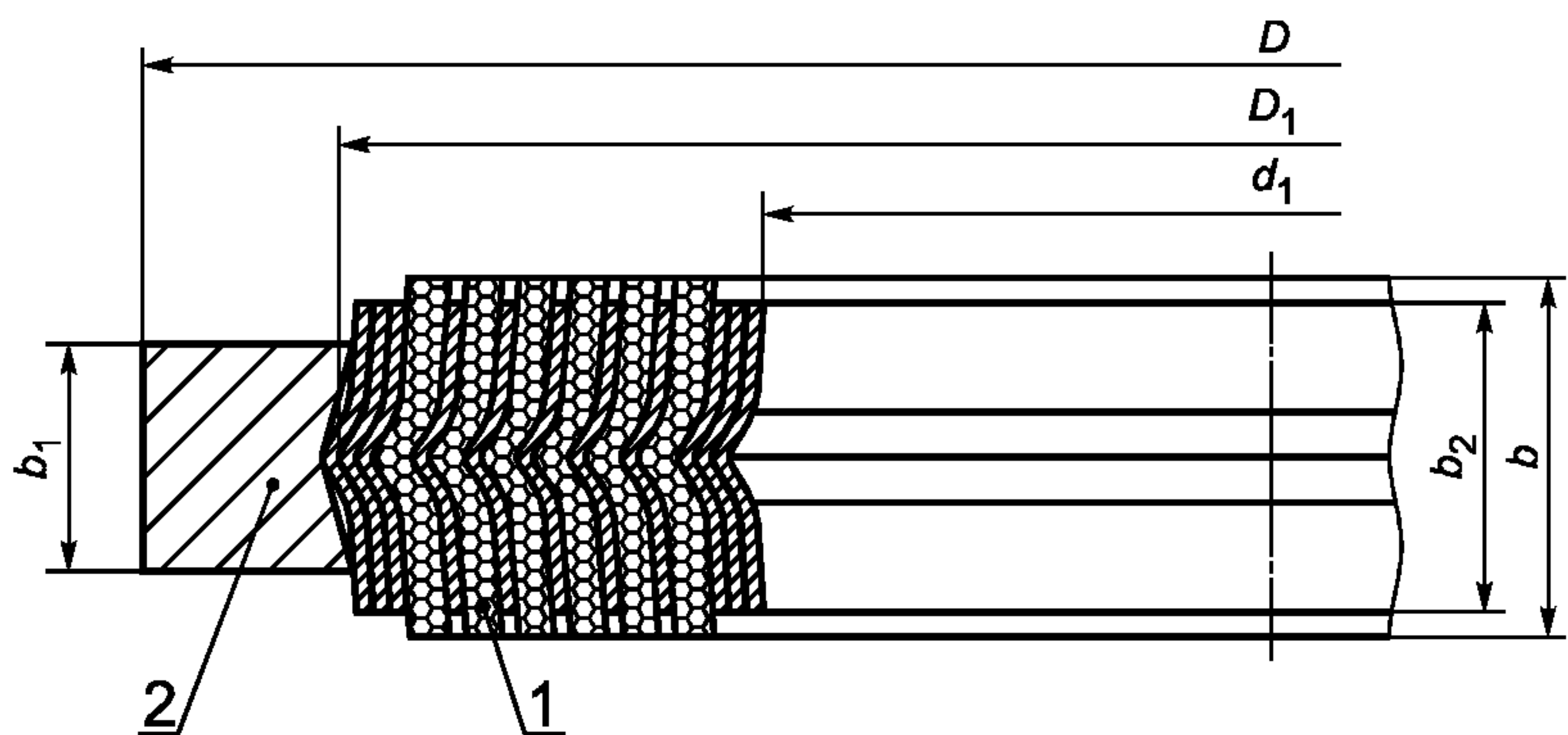
1 — уплотнительное кольцо (см. сноску к рисунку 1); 2 — наружное ограничительное кольцо из углеродистой стали марок 20, 35, 40 или коррозионно-стойкой стали марок 08Х18Н10Т, 08Х18Н9 и других марок, свойства которых не ниже перечисленных
