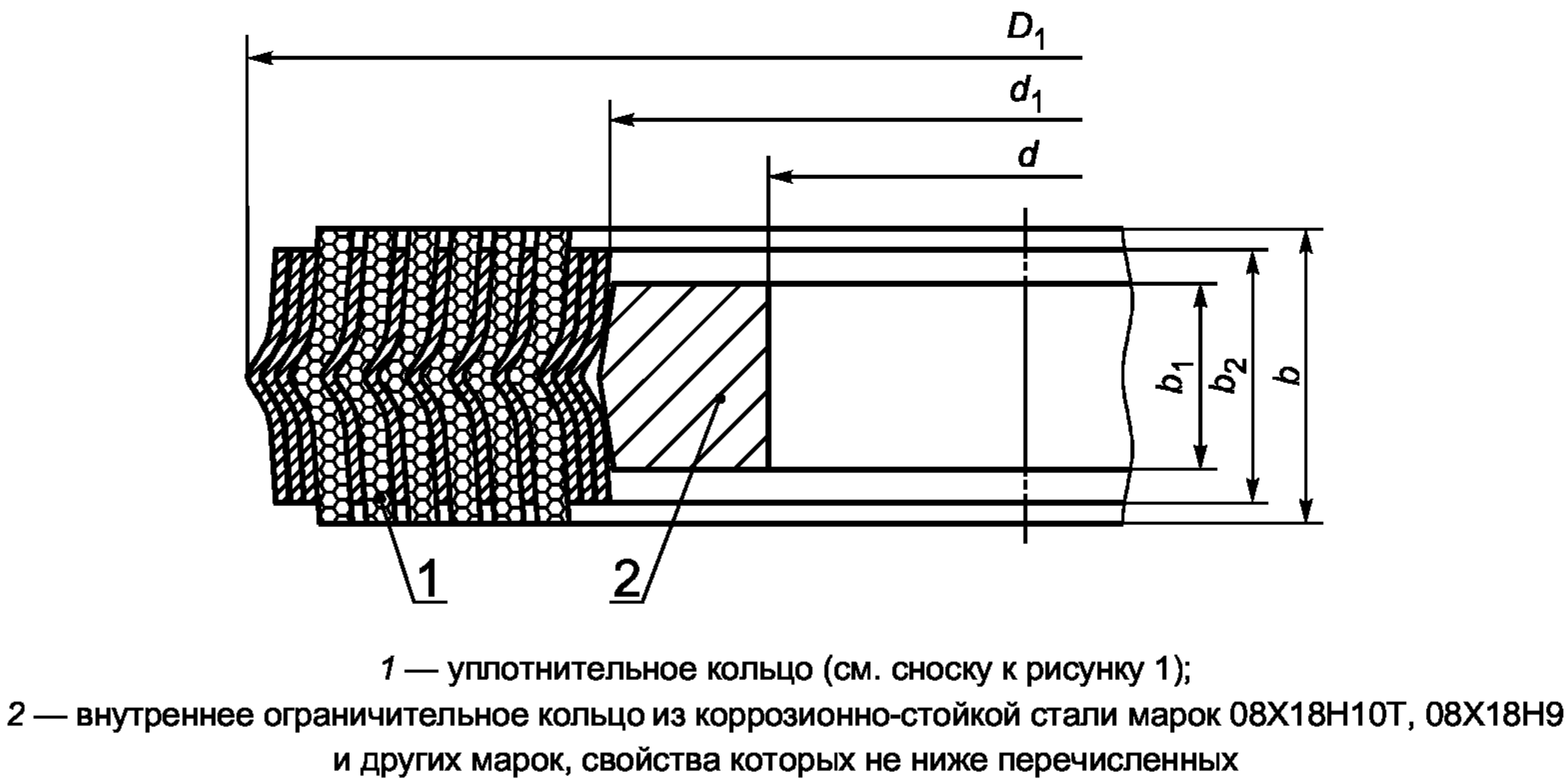
Рисунок 2 — СНП типа В
