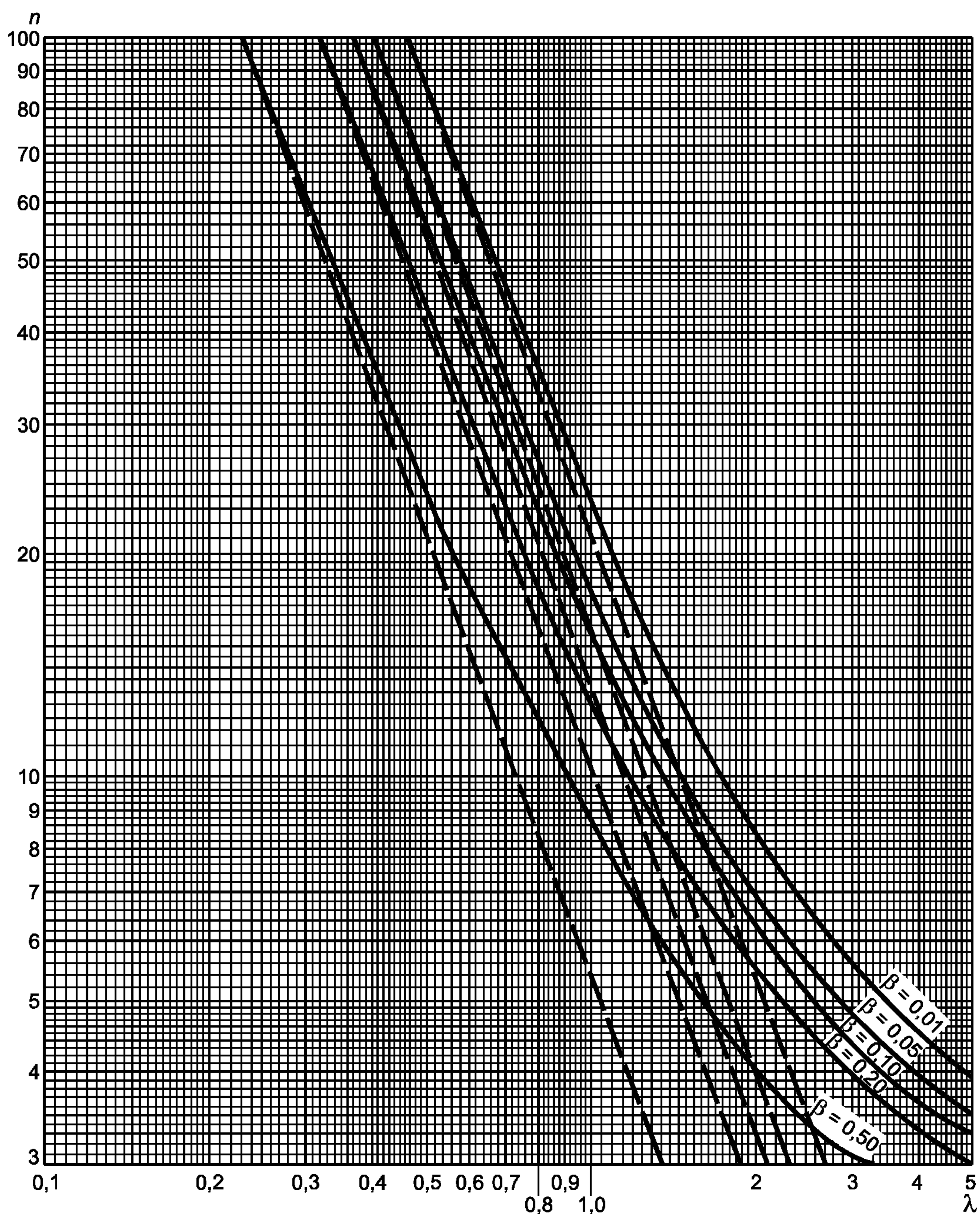
Рисунок 4.2 — Односторонний критерий сравнения средних (риск первого рода \alpha = 0,01 )
