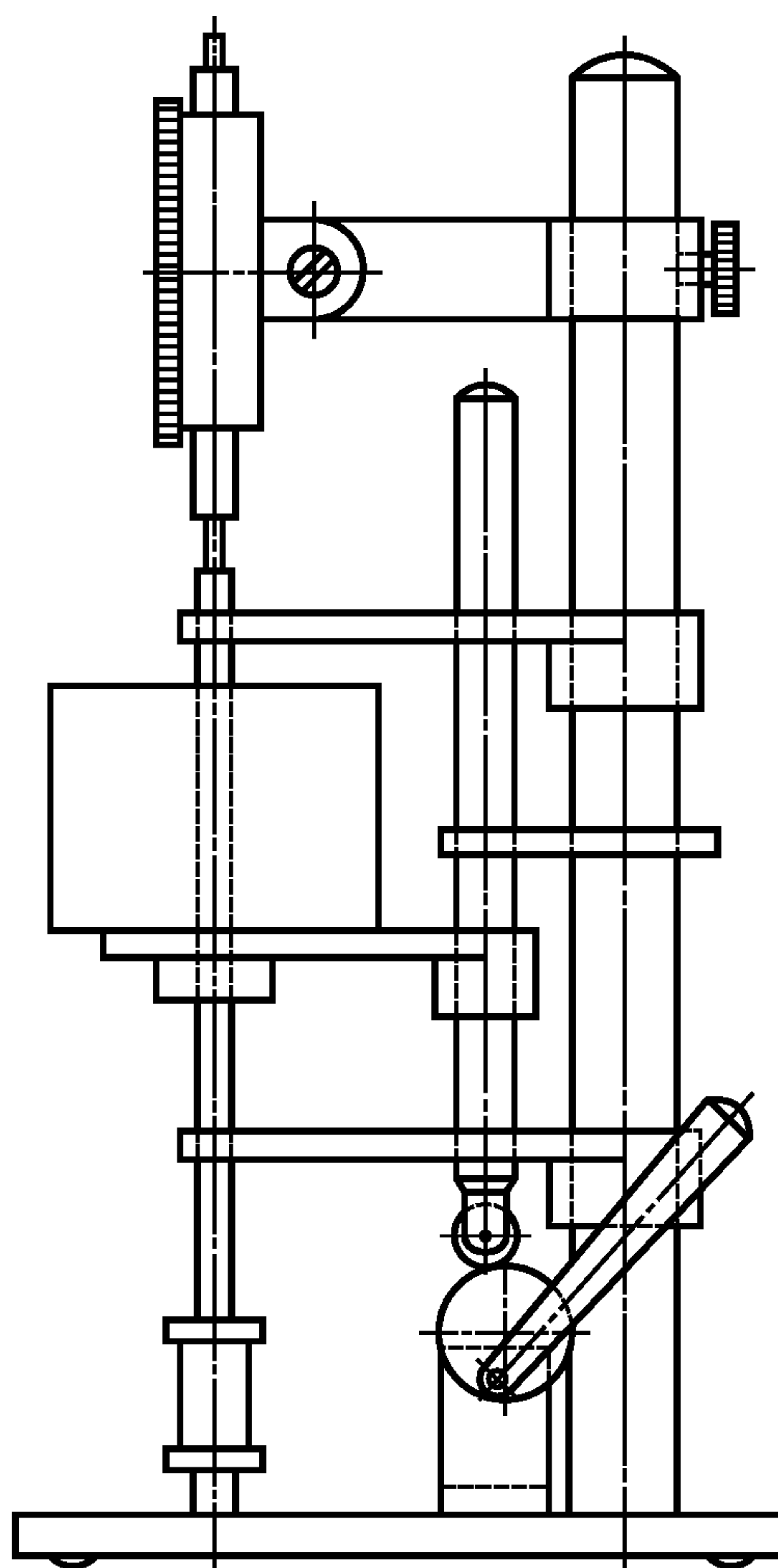
Рисунок 6 — Устройство для испытания на деформацию сжатия
