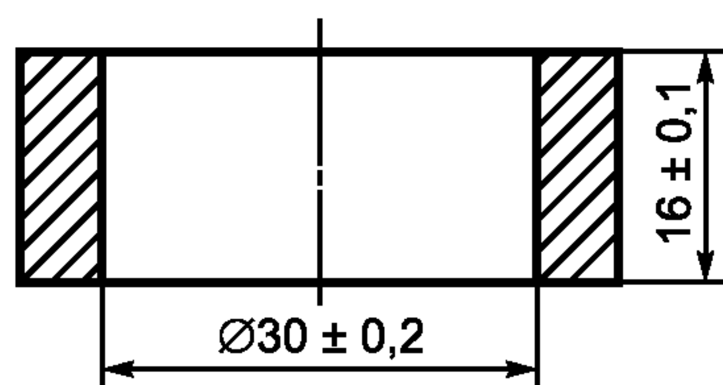
Рисунок 2 — Кольцевая форма
