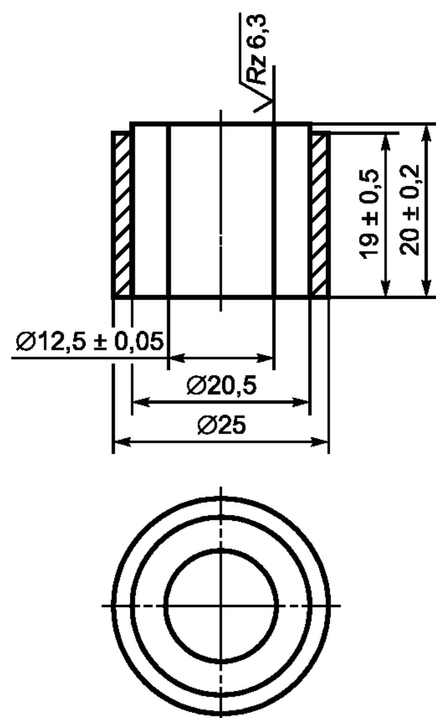
Рисунок 5 — Разъемная форма с фиксирующим кольцом
