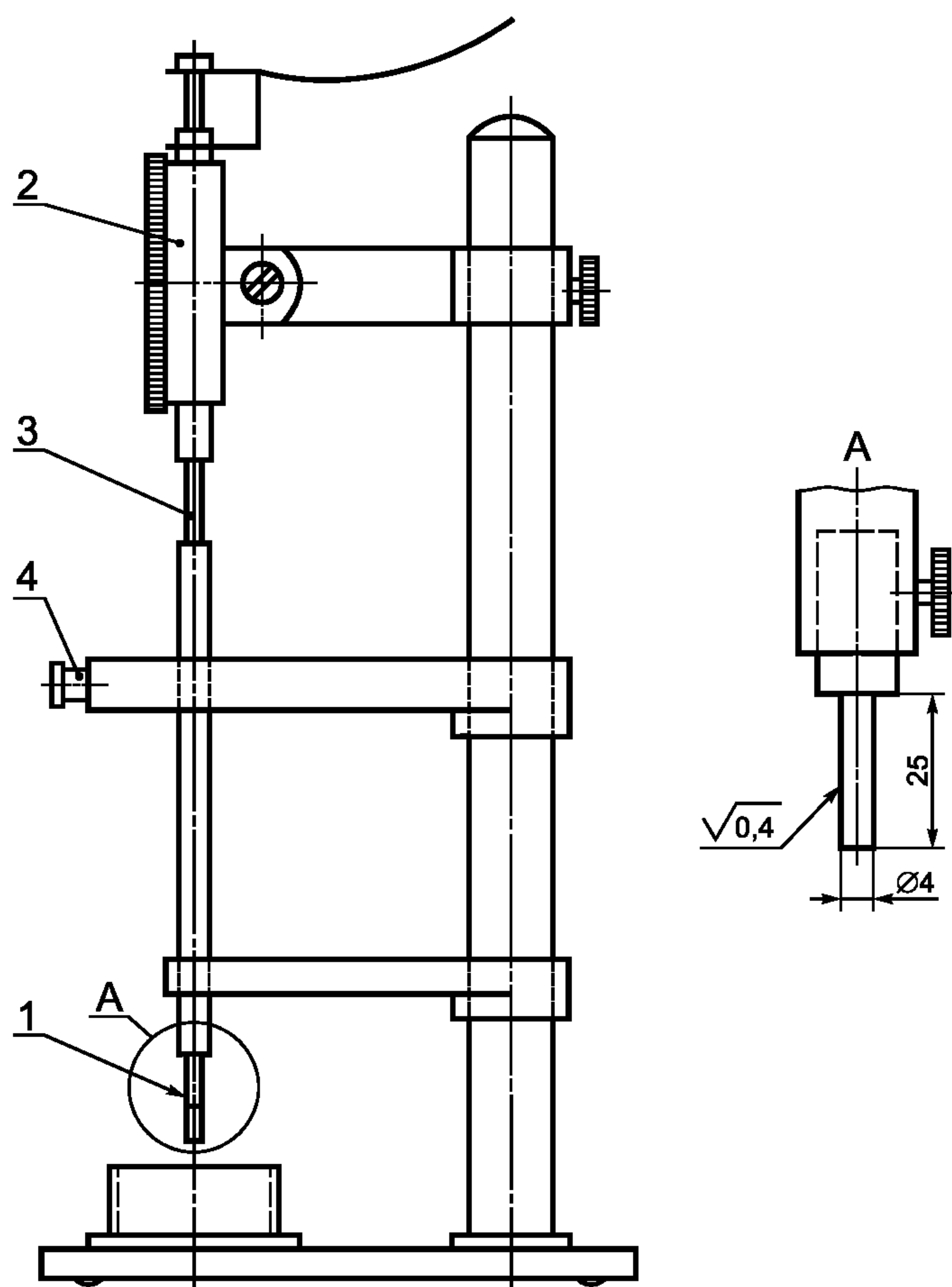
1 — индентер с иглой; 2 — цифровой индикатор; 3 — шпindel; 4 — блокировочное устройство
