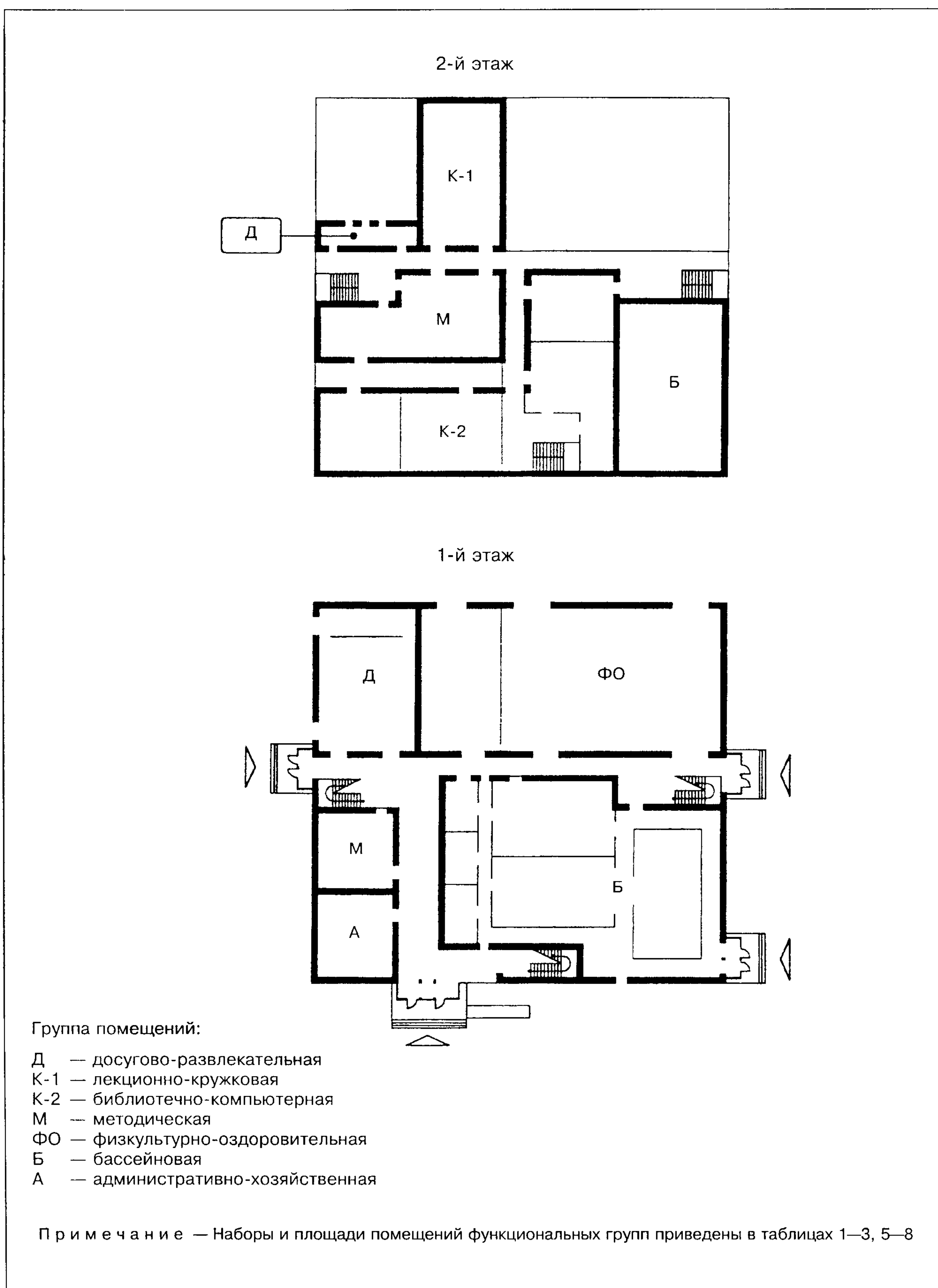
Рисунок Б.2 — Проектное решение досугово-оздоровительного центра
