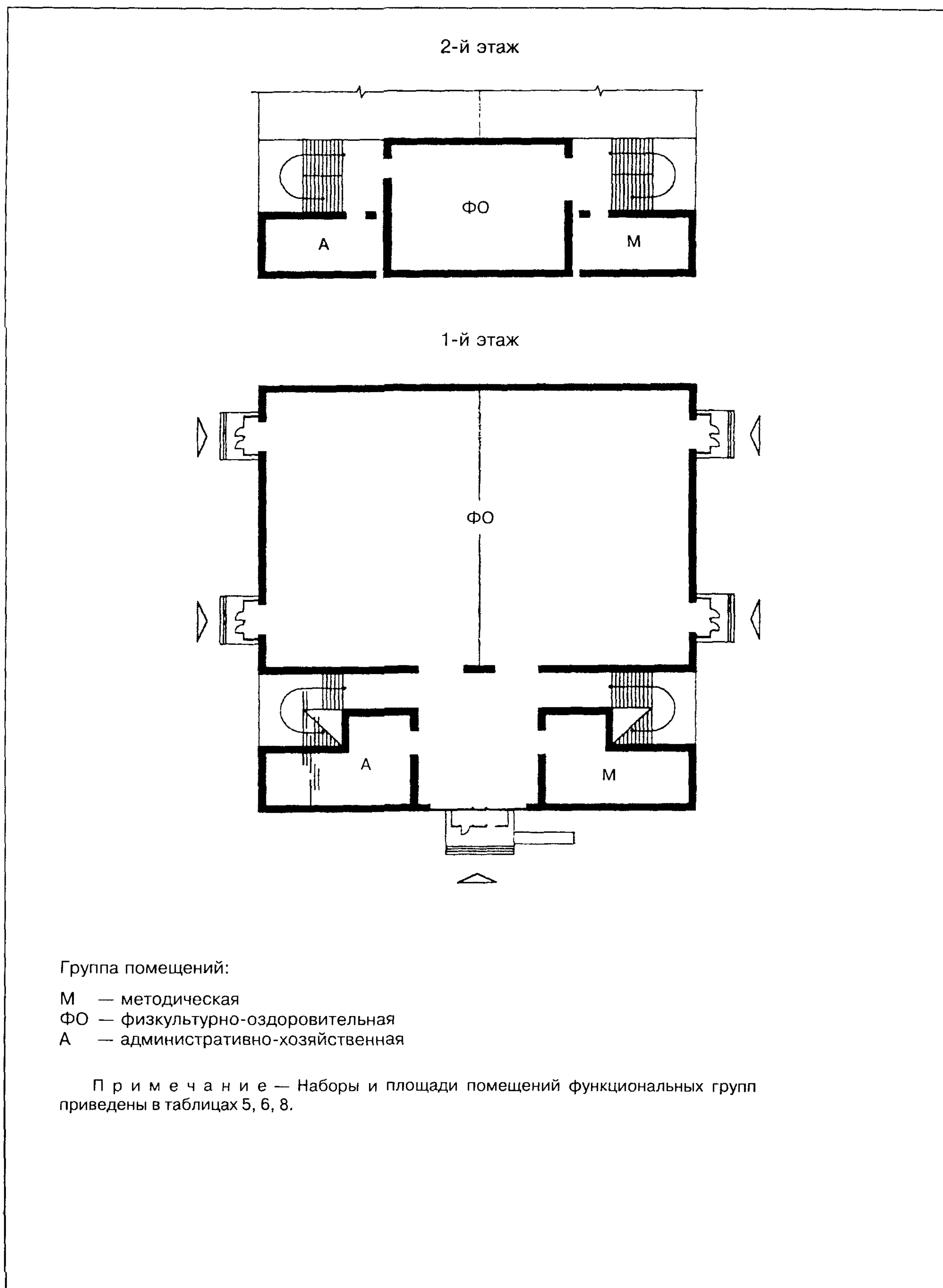
Рисунок Б.3 — Проектное решение консультационно-методического центра
