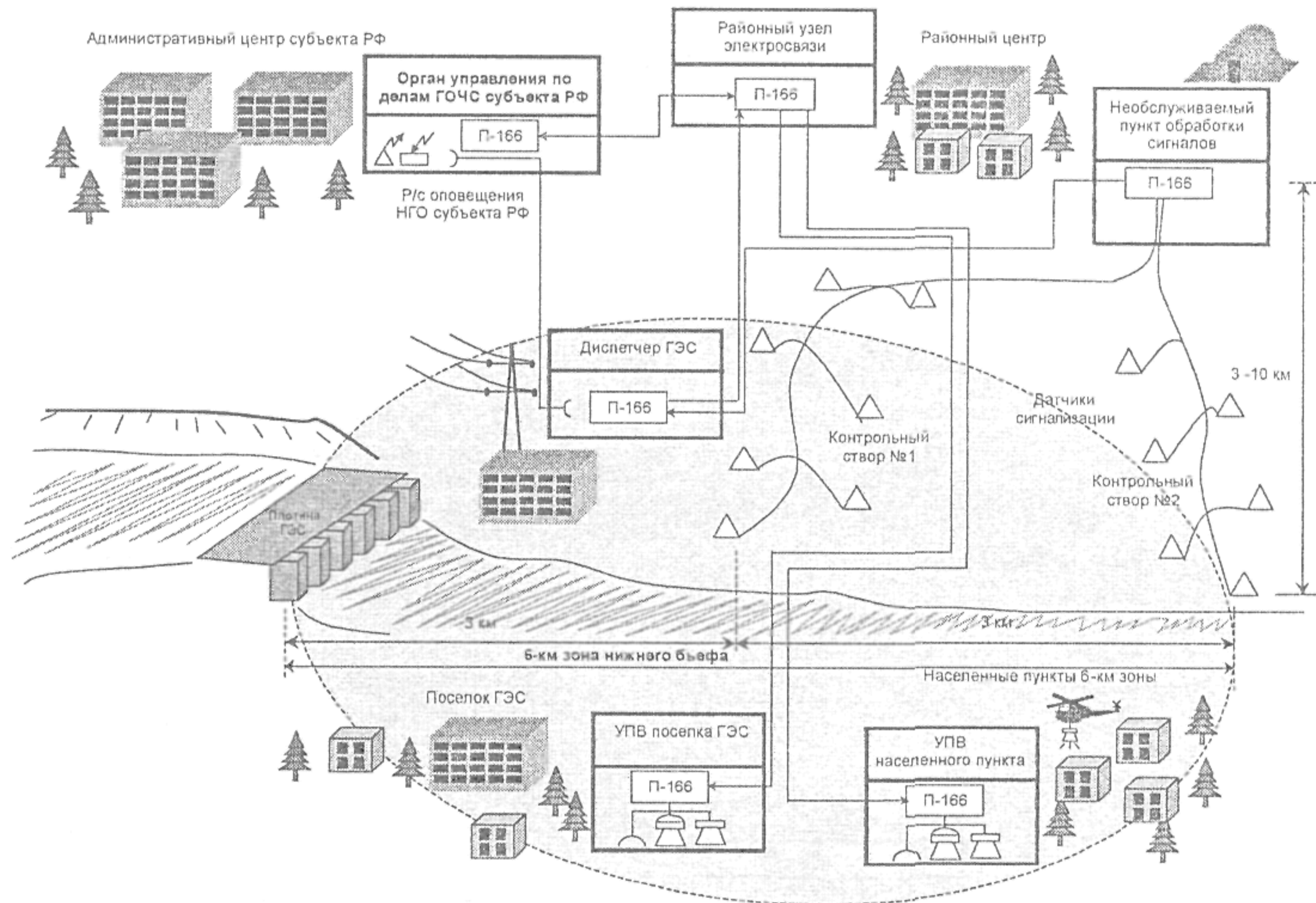
Рис.2.3. Организация локальной системы оповещения в районе размещения ГЭС
