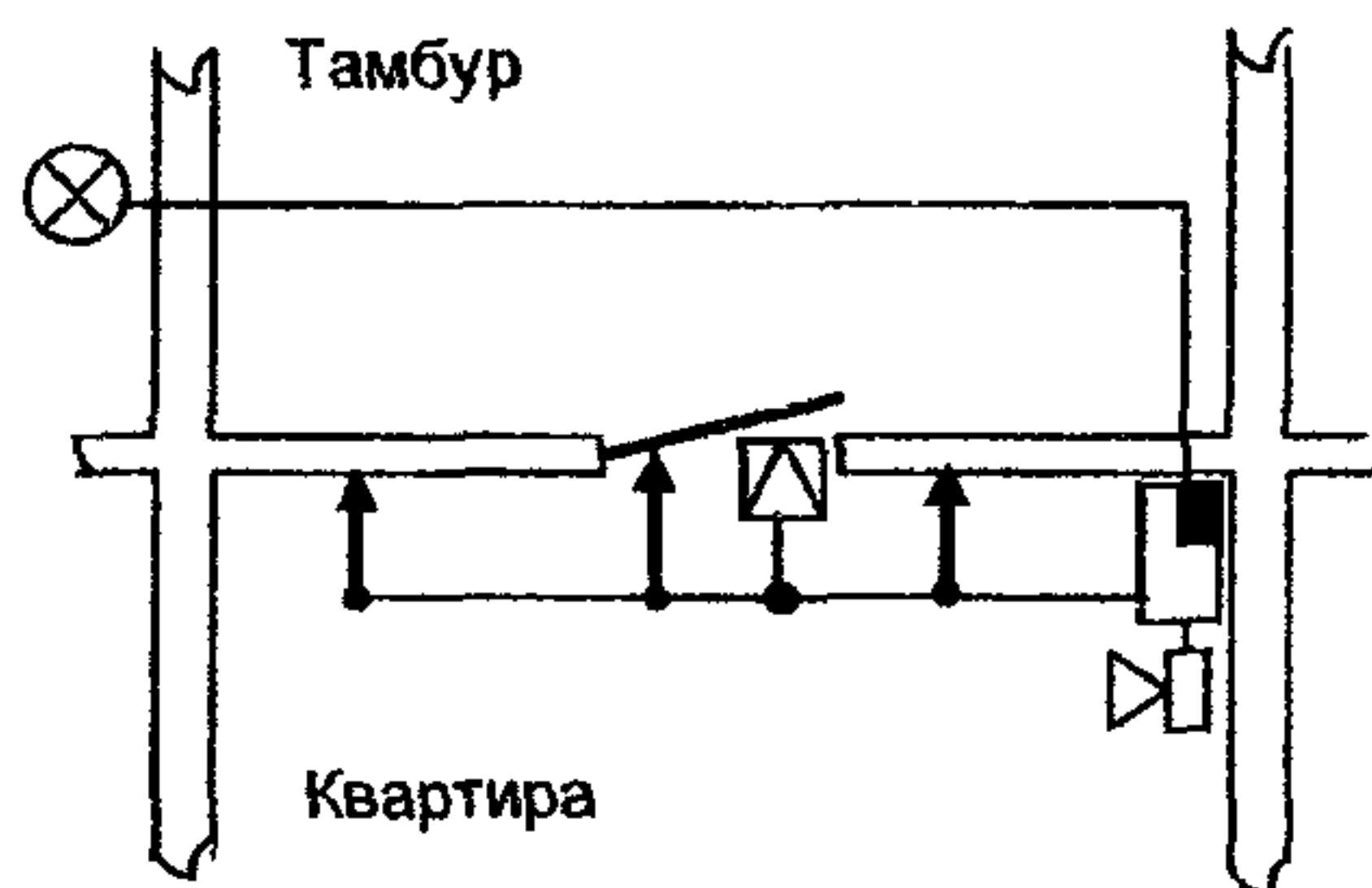
Рисунок 14 - Солидарная охрана входной двери квартиры
