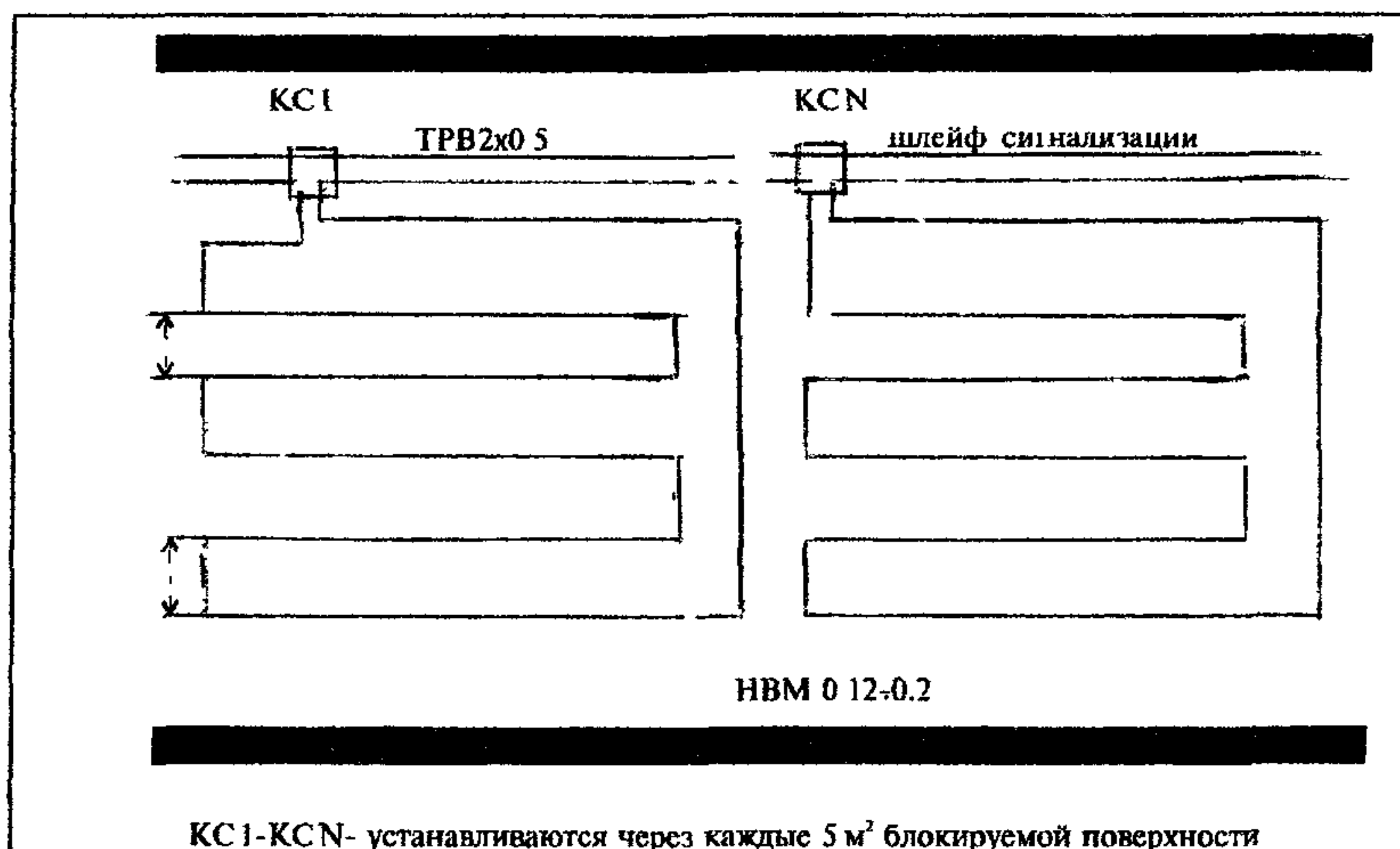
Рисунок 8 - Блокировка стен извещателем омическим типа "Провод"
