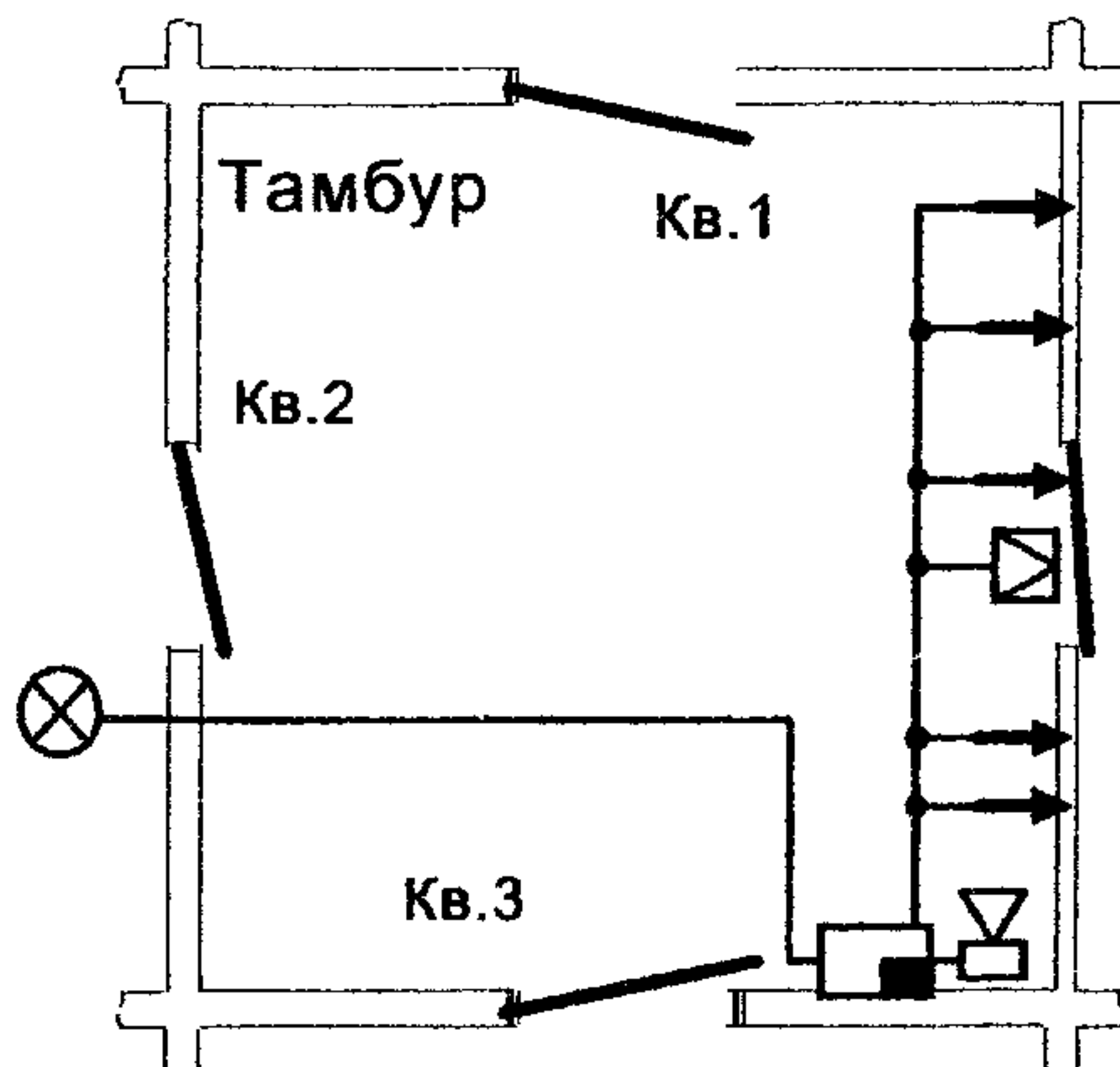
Рисунок 11 - Солидарная охрана двери квартирного тамбура
