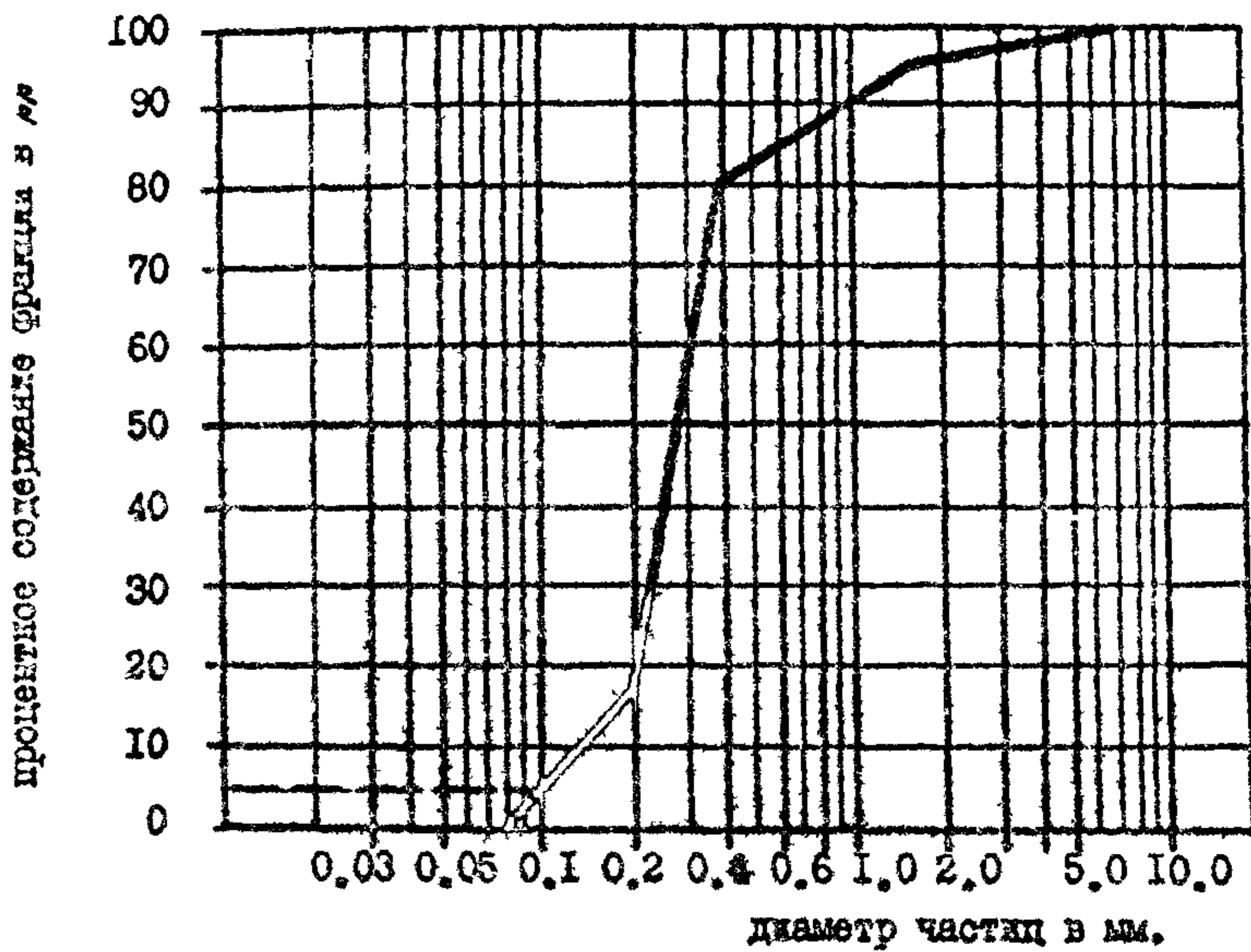
Рис. 5 КРИВАЯ ГРАНУЛОМЕТРИЧЕСКОГО СОСТАВА ГРУНТА (пример)
