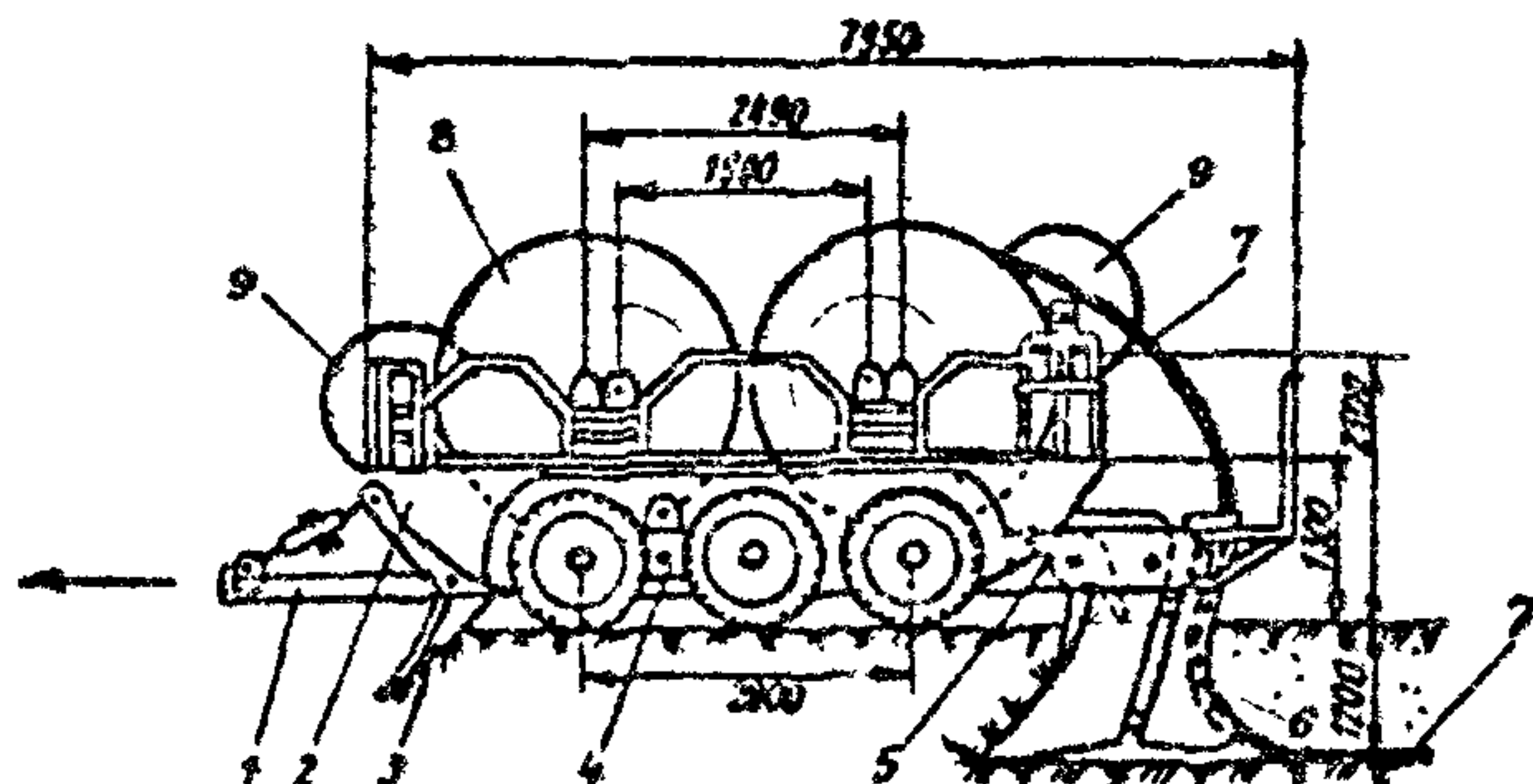
Рис. 3.3. Кабелеукладчик КУ-К-3
