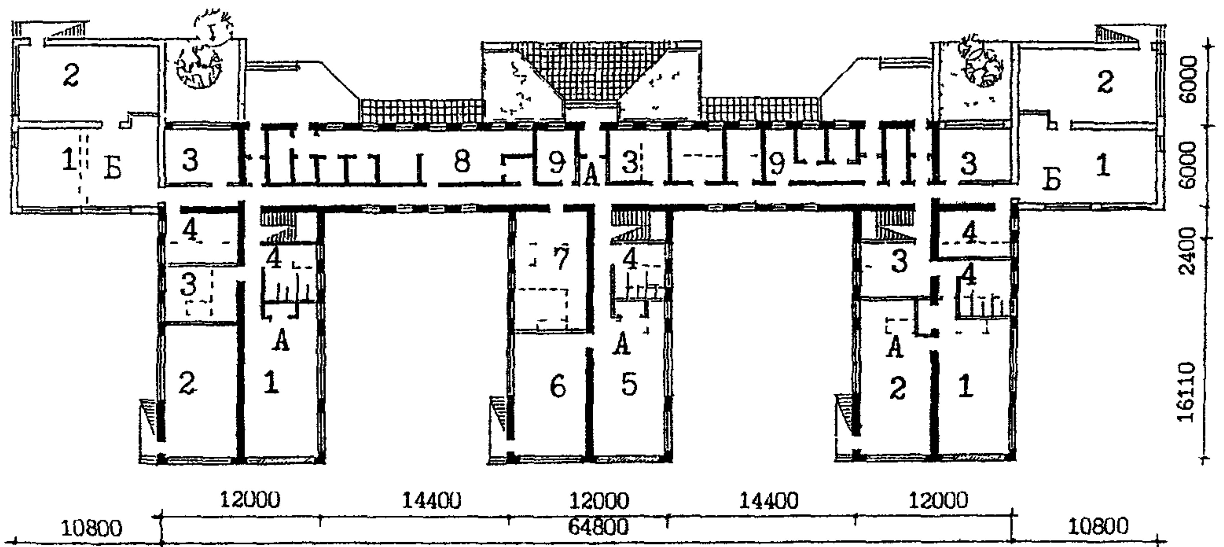
план 1 этажа
