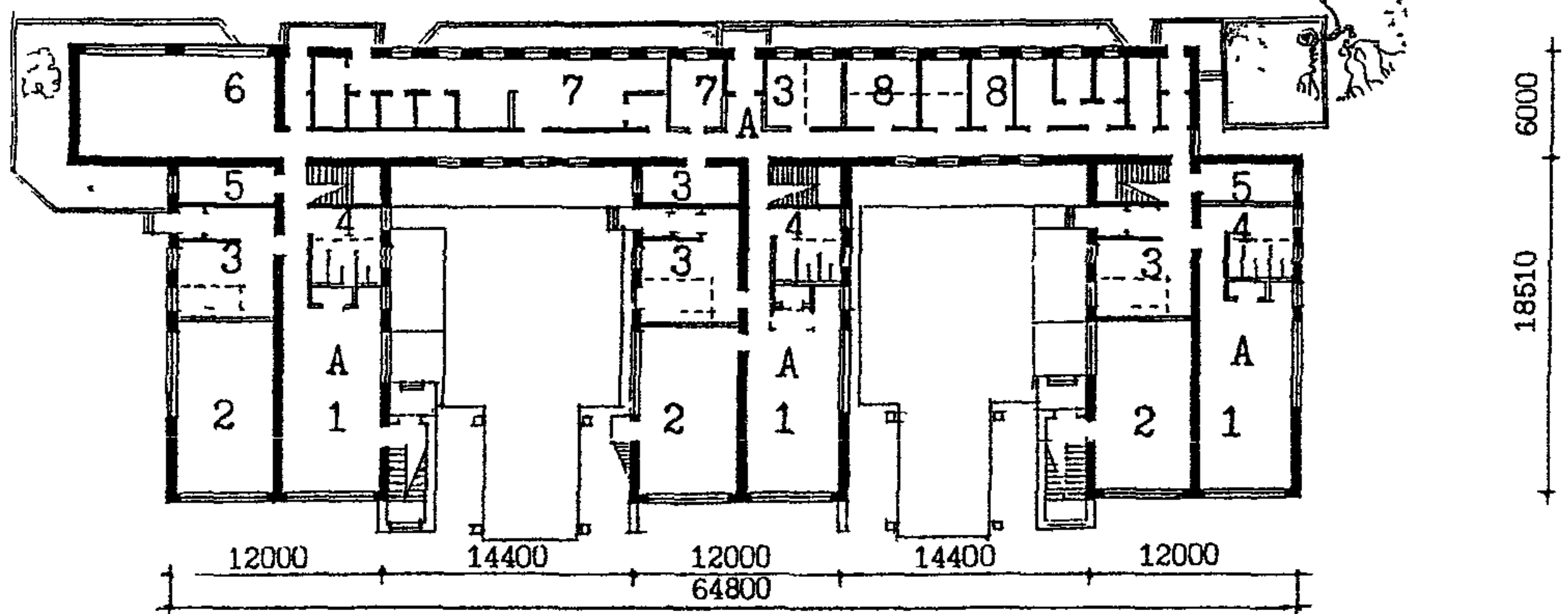
Рис 32 Пример архитектурно-планировочного решения реконструкции здания детского сада типа У1-13 для ДООУ на 10 групп 200 мест (для затесненных участков) Планы 1, 2 и 3 этажей.
