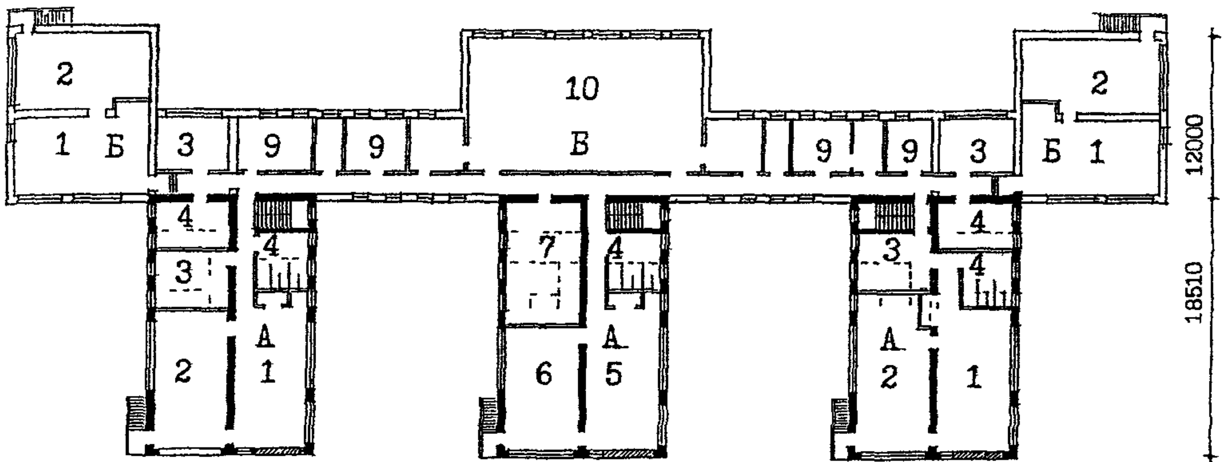
план 2 этажа
