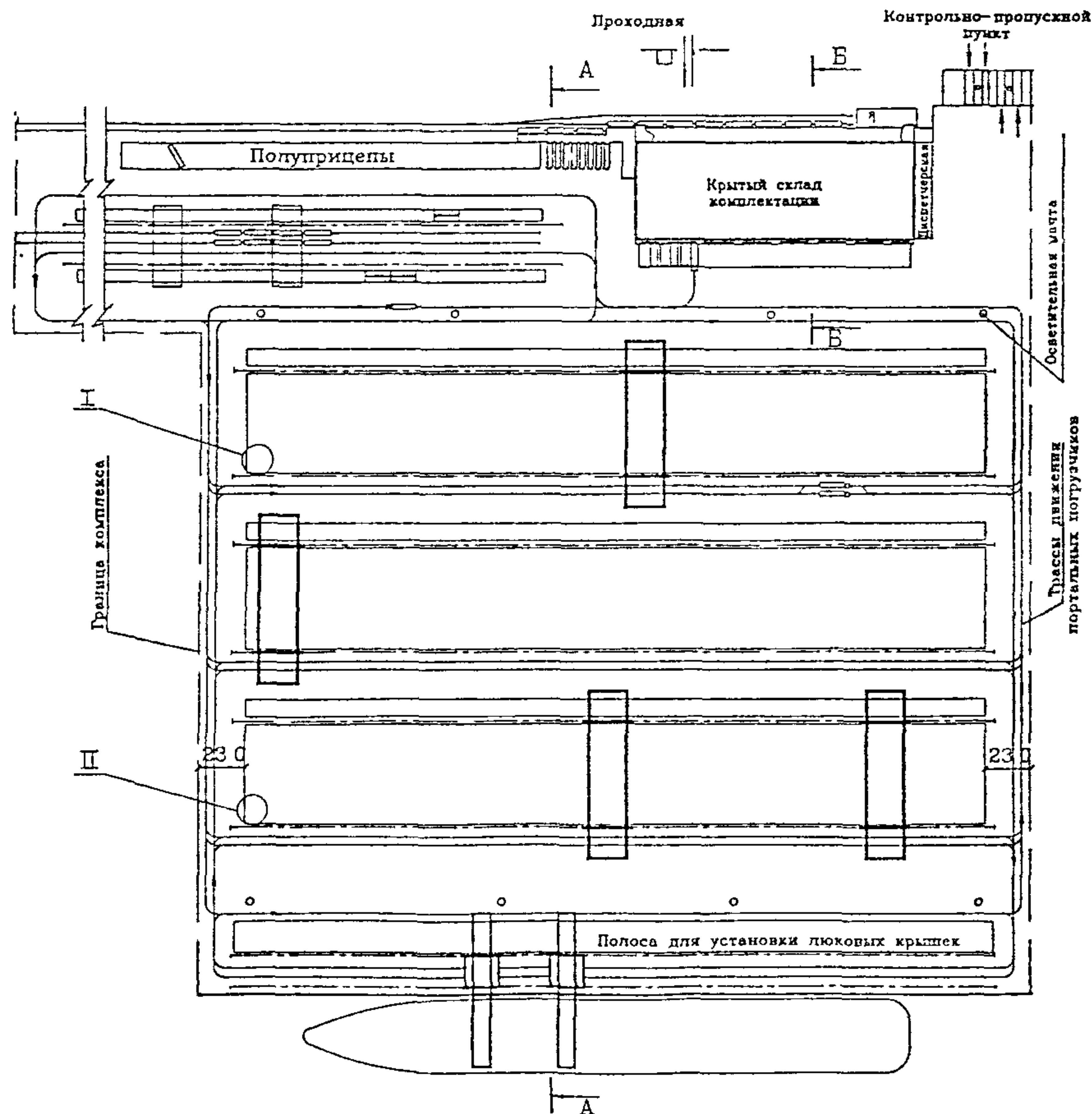
Рис. 7 Схема механизации НЗ с козловыми перегружателями на рельсовом ходу План
