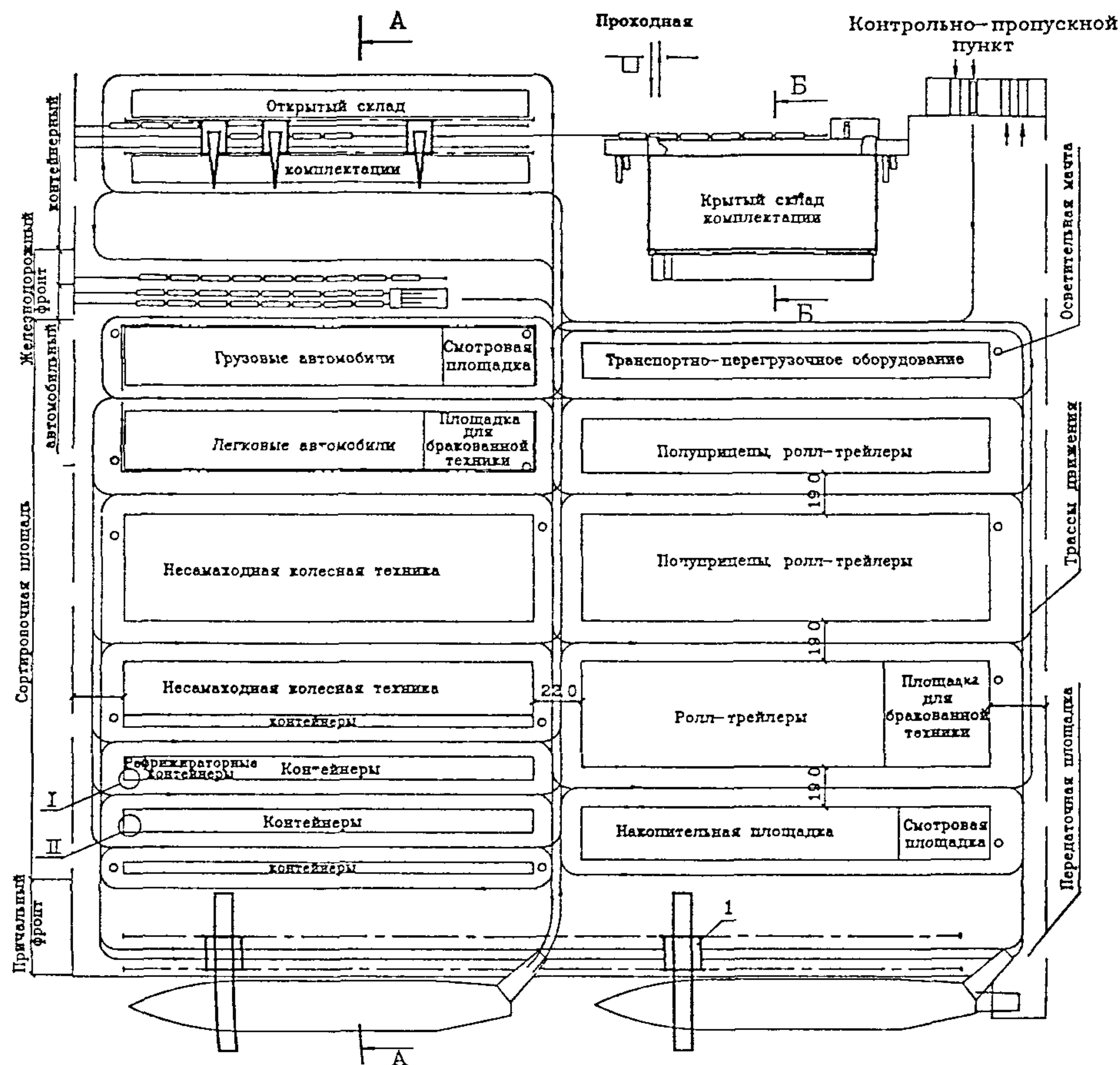
Рис. 3 Схема механизации N2 с использованием фронтальных погрузчиков. План
