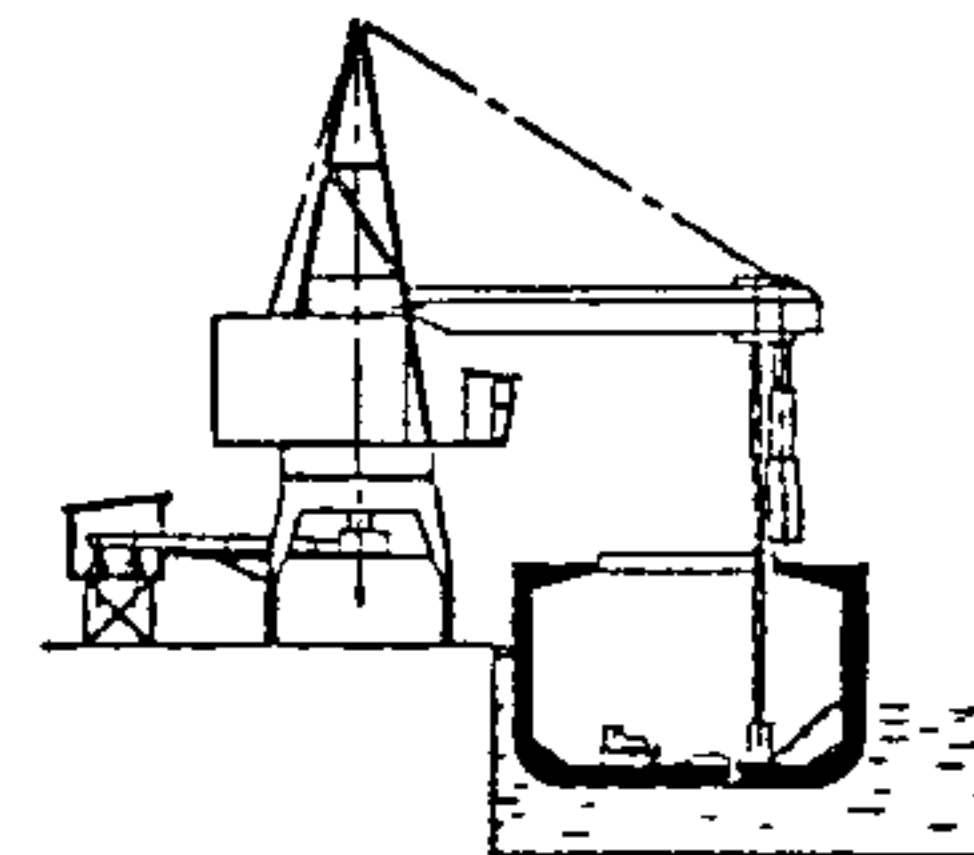
комбинированный пневмо-механический перегружатель
