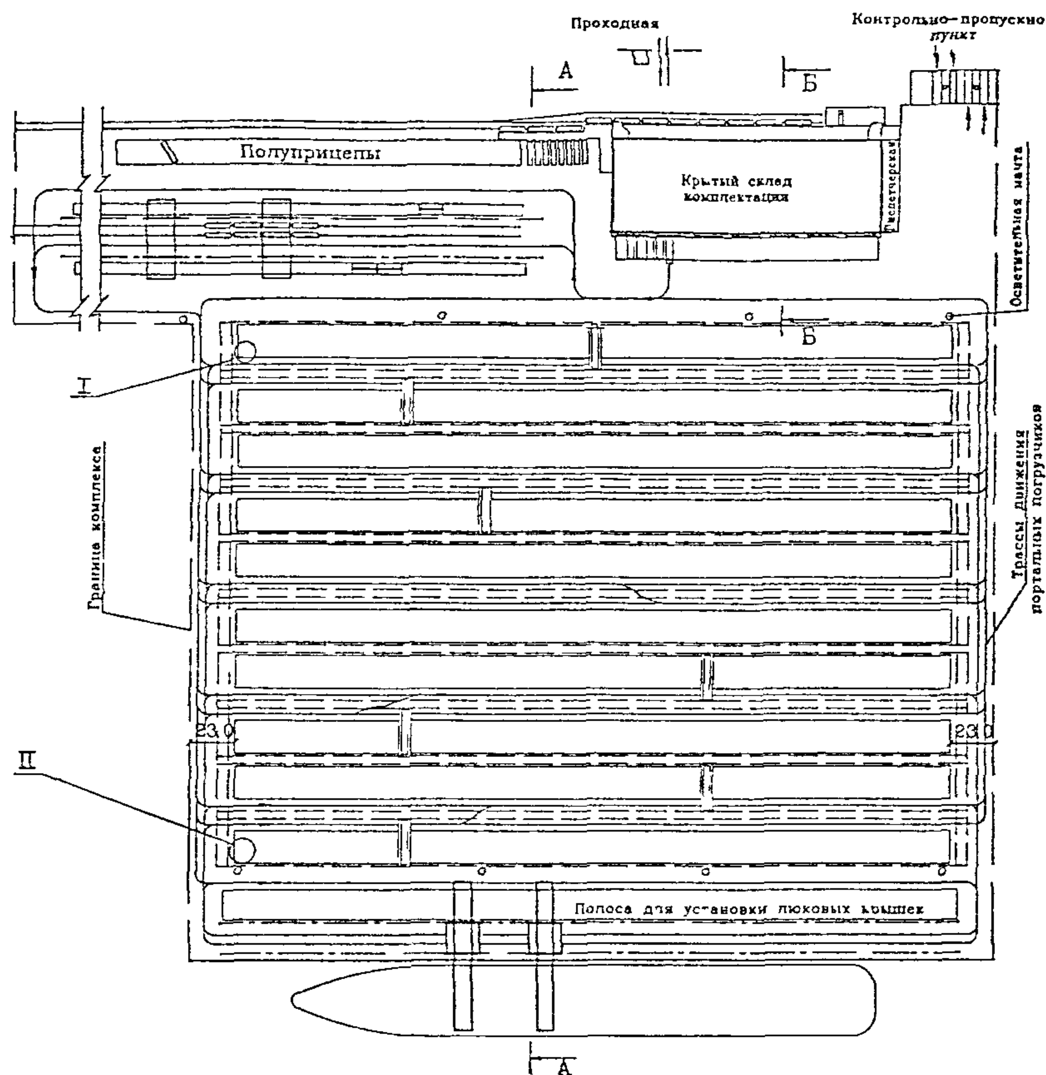
Рис. 5 Схема механизации №2 с пневмоколесными кранами. План
