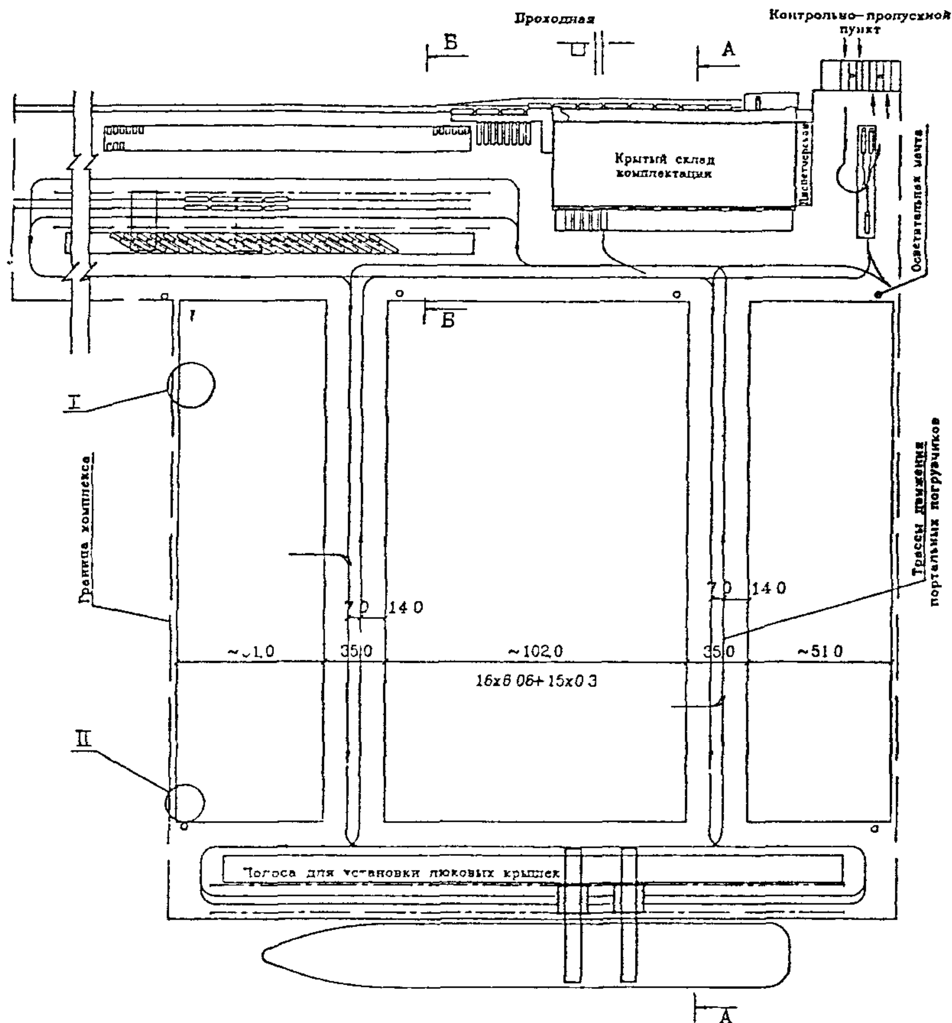
Рис. 3 Схема механизации N1 с портальными погрузчиками и размещением контейнеров параллельно линии кордона. План
