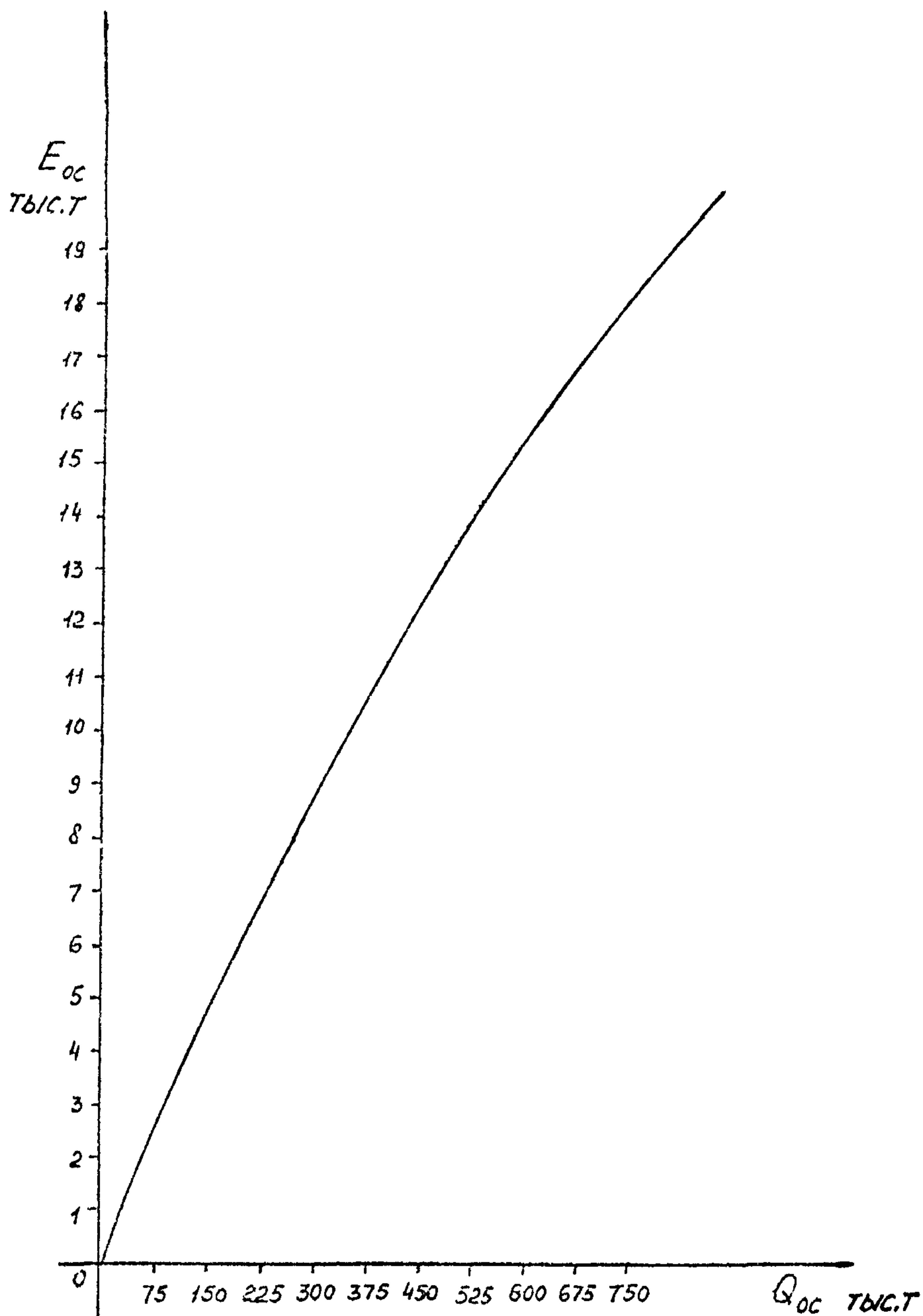
Рис.18. Зависимость потребной вместимости открытого склада от грузооборота
