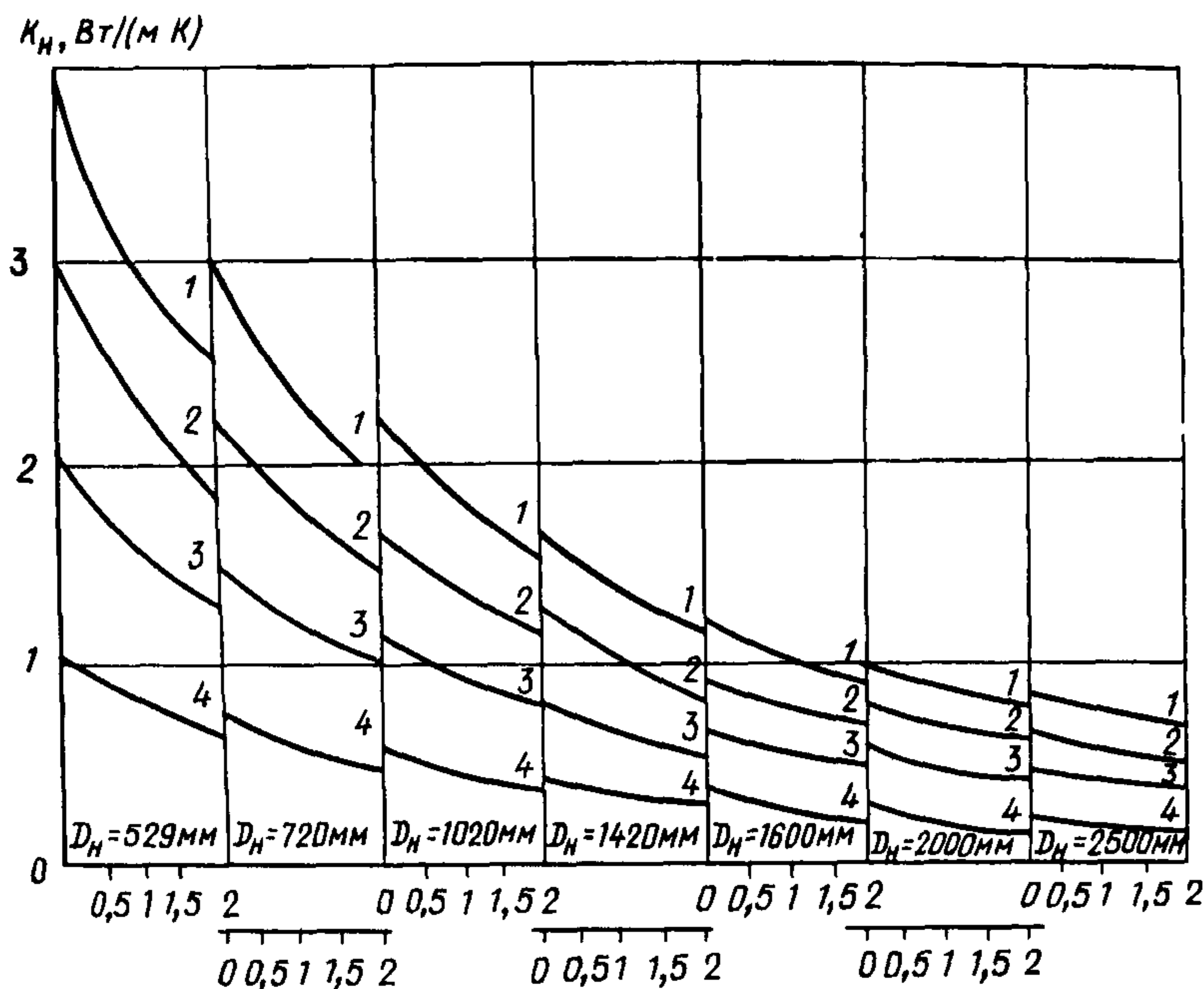
Рис. 1. Номограмма для определения коэффициента теплопередачи подземного трубопровода k_H в зависимости от глубины заложения трубопровода h_\delta и внешнего диаметра трубопровода D_H 1 — \lambda = 2 Вт/(м·К); 2 — \lambda = 1,5 Вт/(м·К); 3 — \lambda = 1 Вт/(м·К); 4 — \lambda = 0,5 Вт/(м·К)
