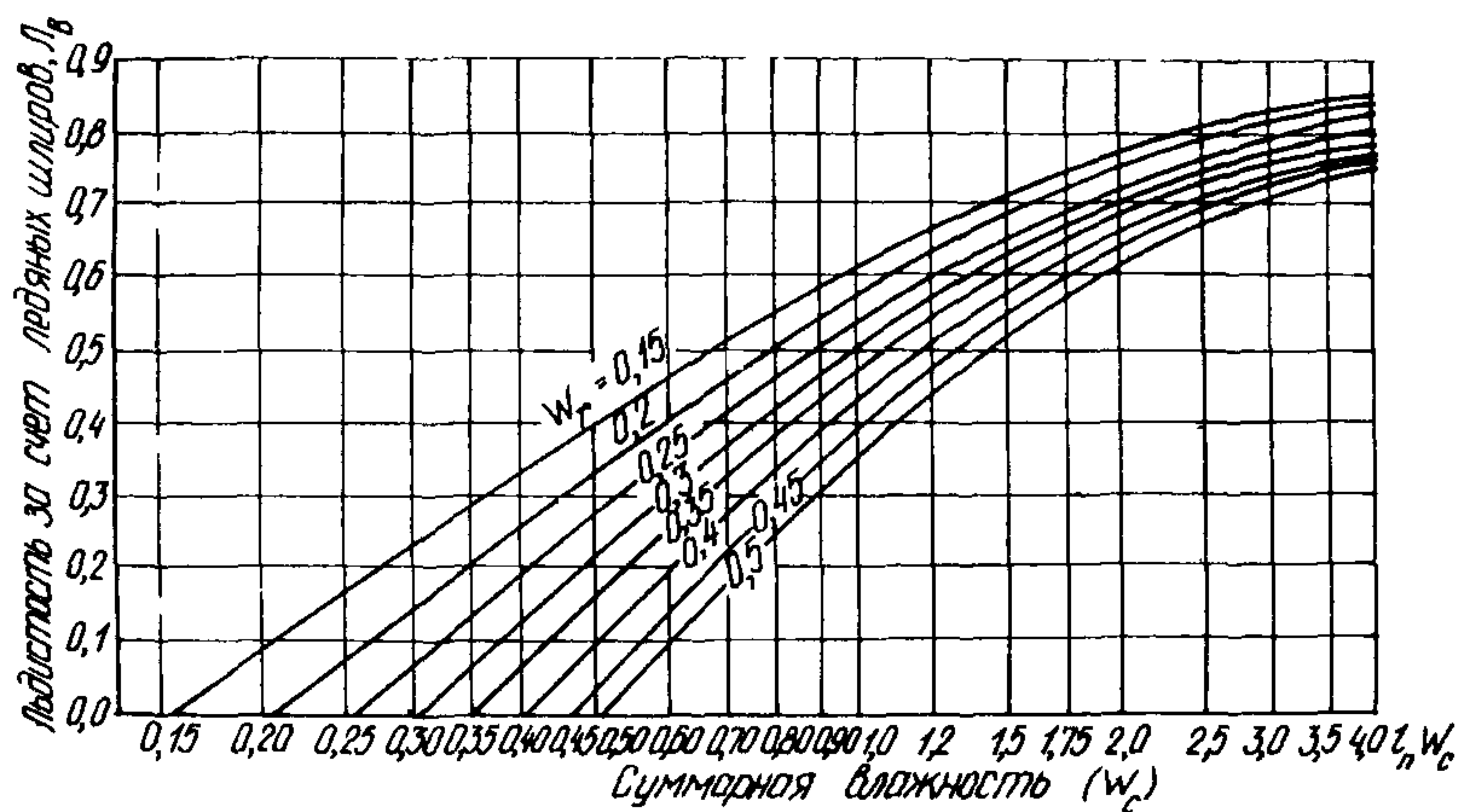
Рис. 1. Номограмма для определения суммарной влажности W_c за счет объемной льдистости J_v и влажности минеральных прослоев W_r .
