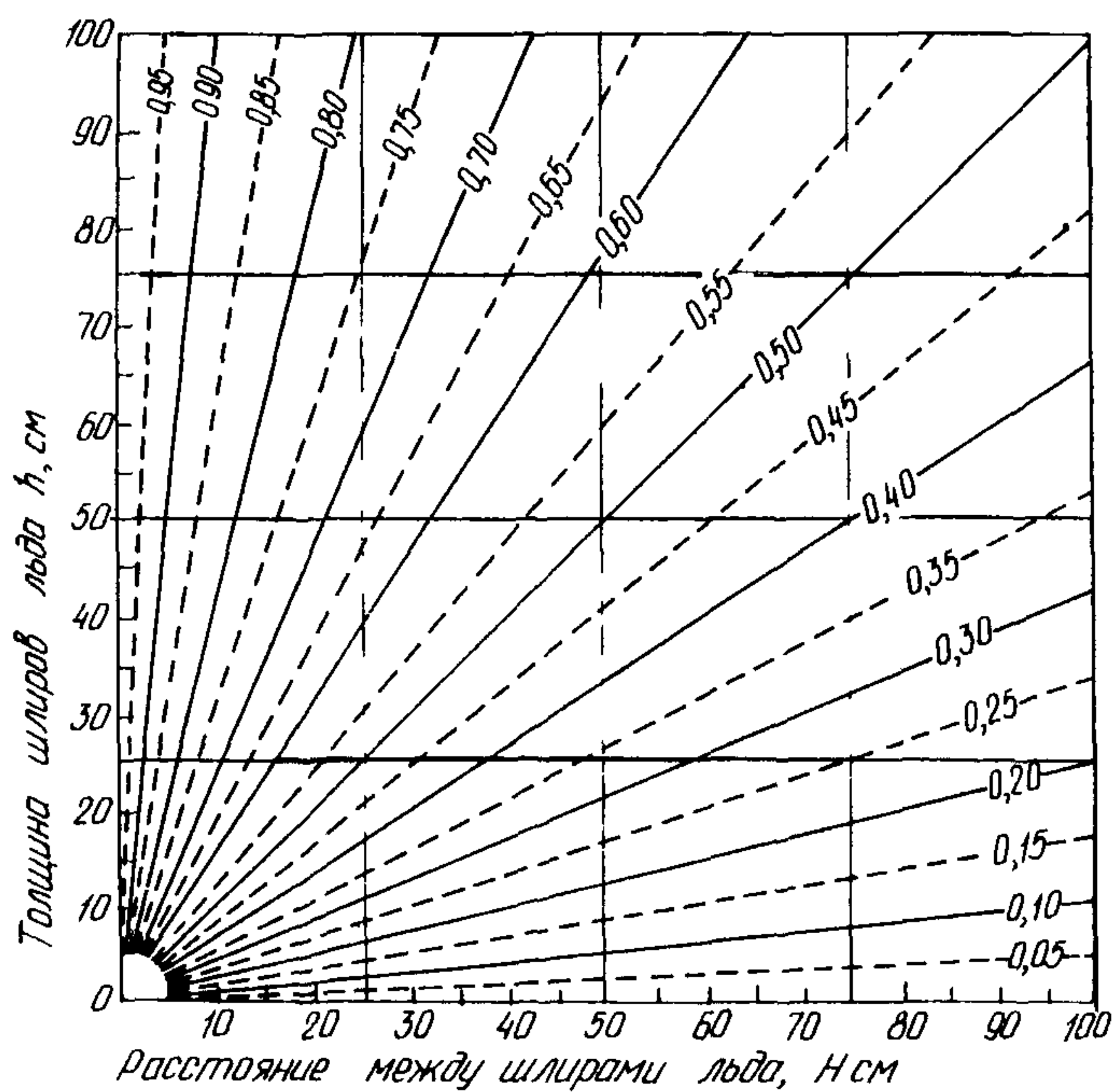
Рис. 2. Номограмма для определения объемной льдистости ( J_v ) мерзлых грунтов со слоистой криогенной текстурой.
