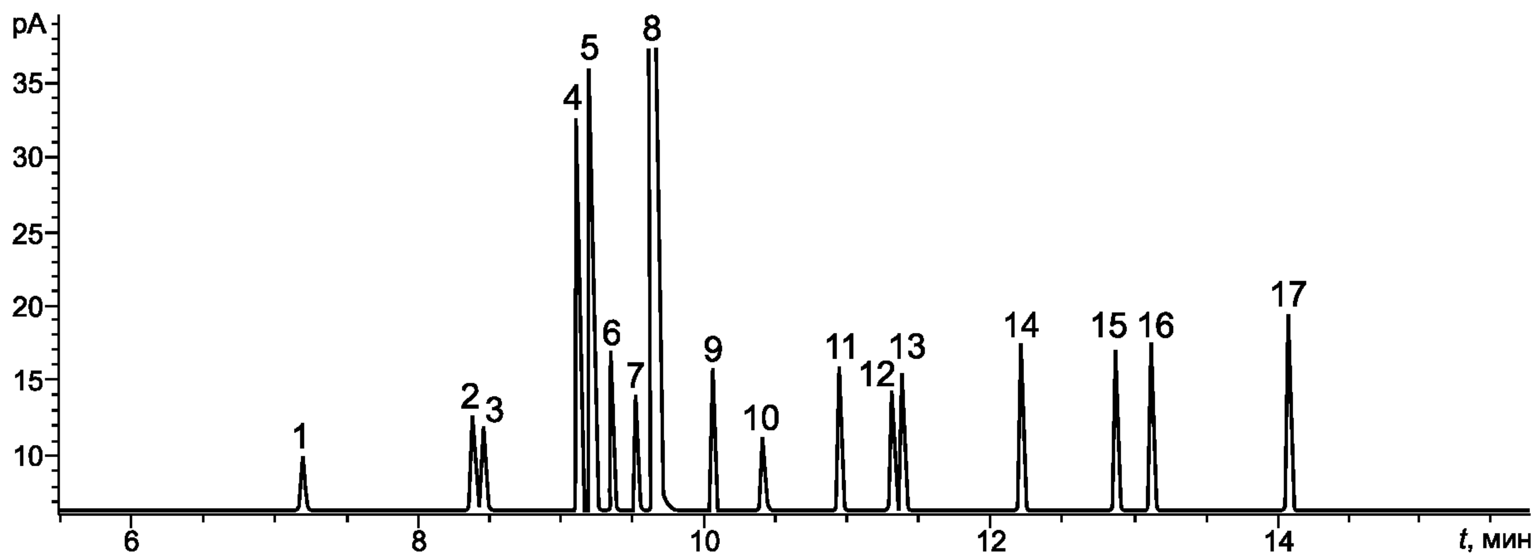
1 — уксусный альдегид; 2 — ацетон; 3 — этилформиат; 4 — этилацетат; 5 — метанол; 6 — 2-бутанон; 7 — 2-пропанол; 8 — этанол; 9 — этилпропионат; 10 — диацетил; 11 — изобутилацетат; 12 — 1-пропанол; 13 — этилбутират; 14 — изобутиловый спирт; 15 — изоамилацетат; 16 — 1-бутанол; 17 — изоамиловый спирт
