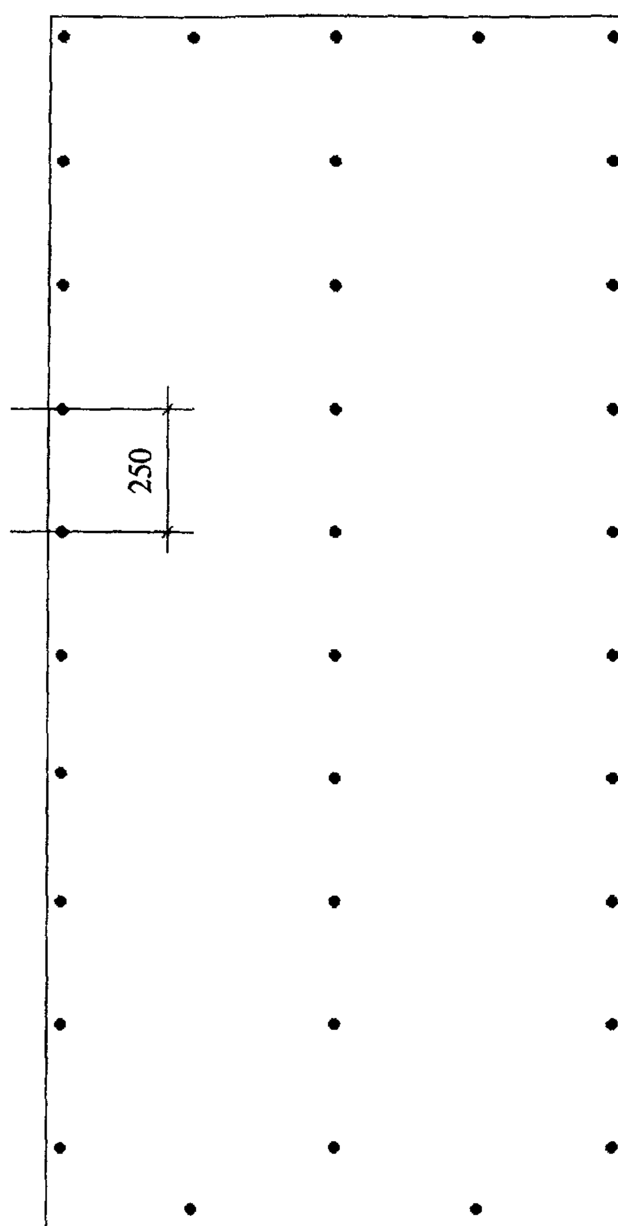
Рисунок 9 — Схема расположения самонарезающих винтов при однослойной облицовке
