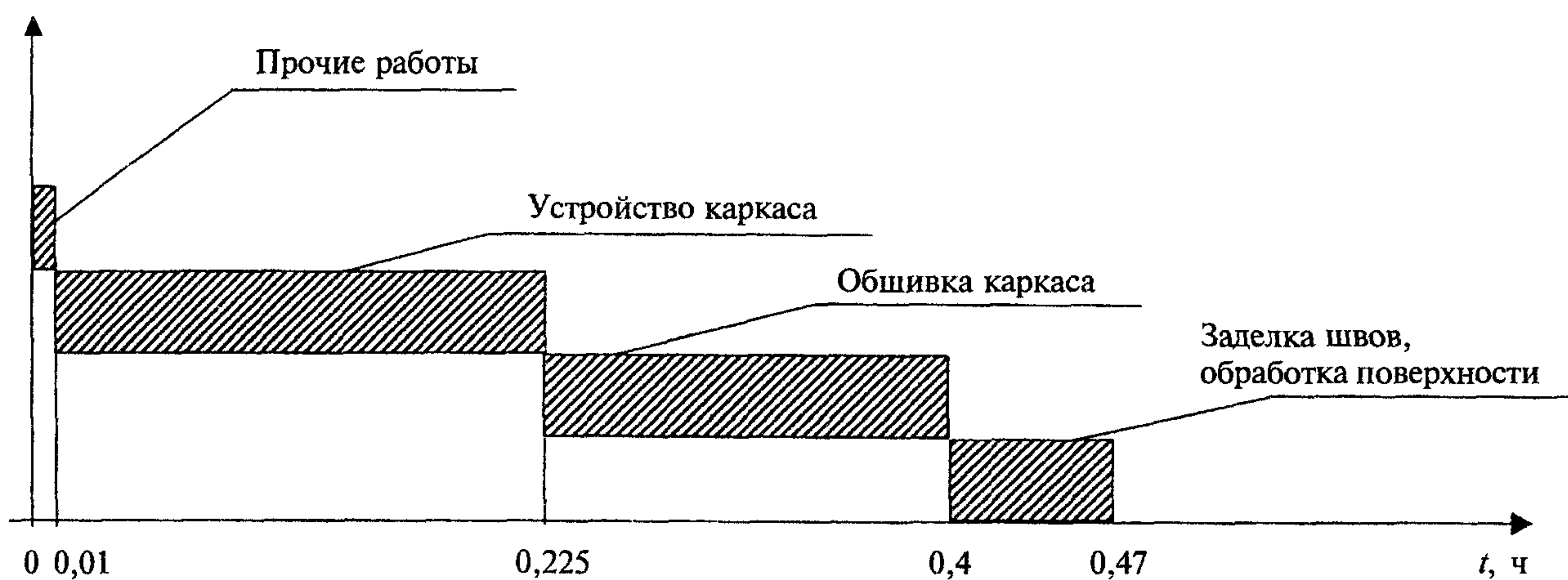
Рисунок 4.1 — График движения рабочей силы
