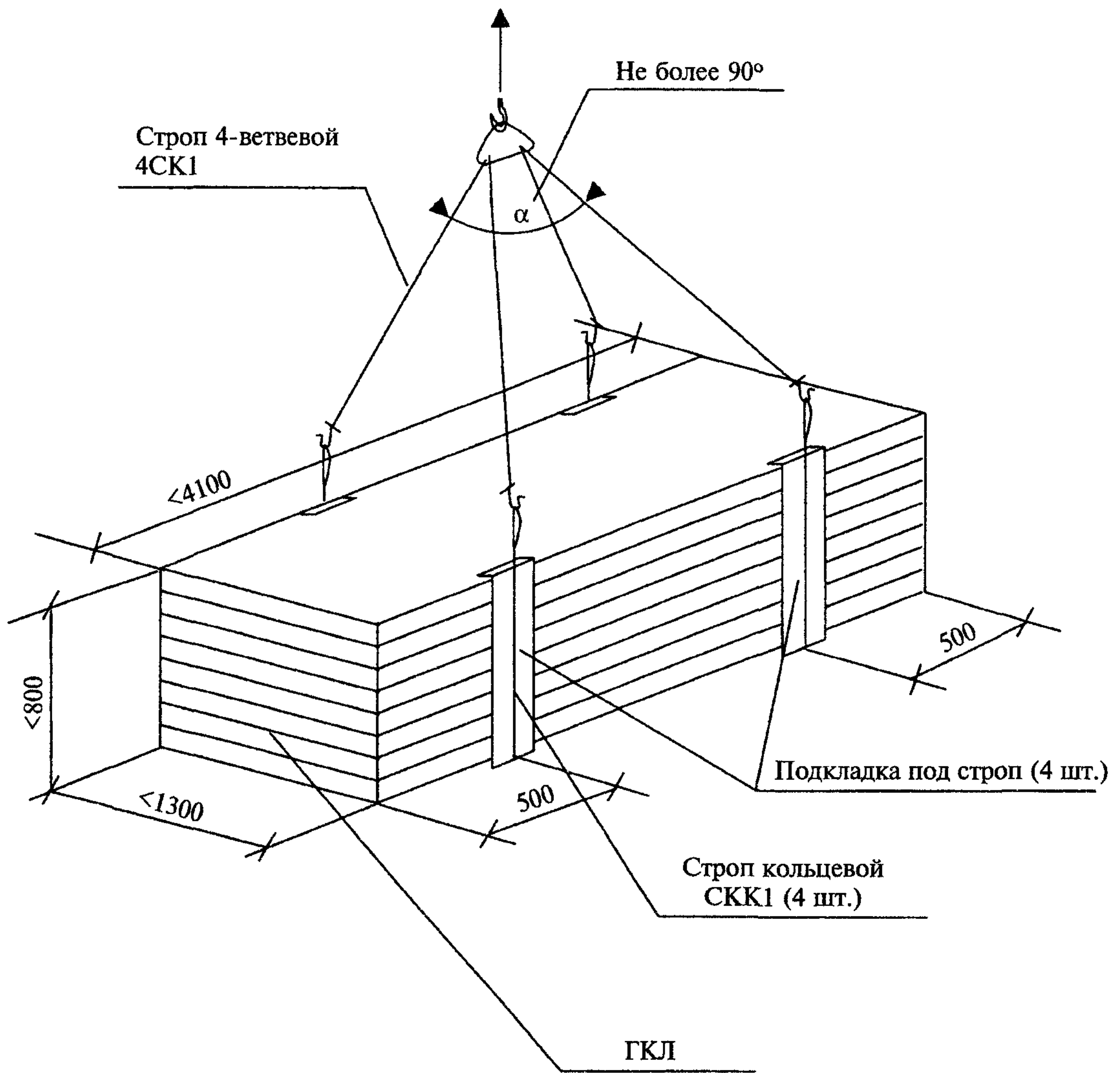
Рисунок 1 – Схема строповки пакета ГКЛ
