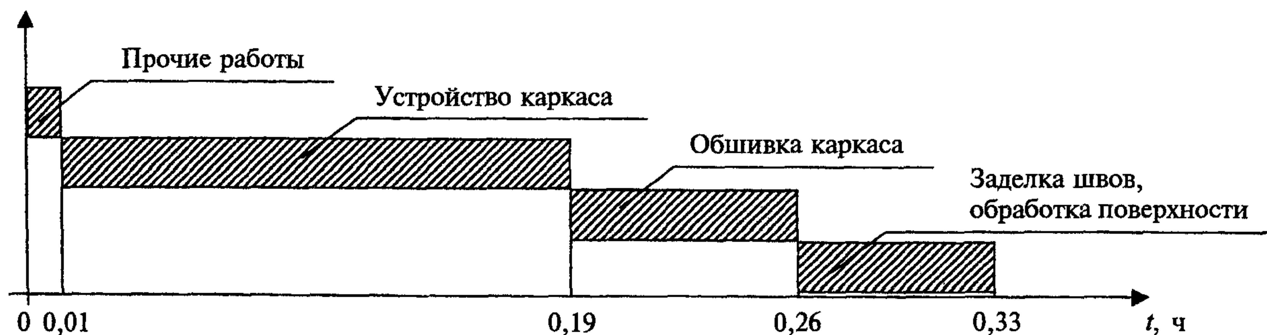
Рисунок 4.1 — График движения рабочей силы
