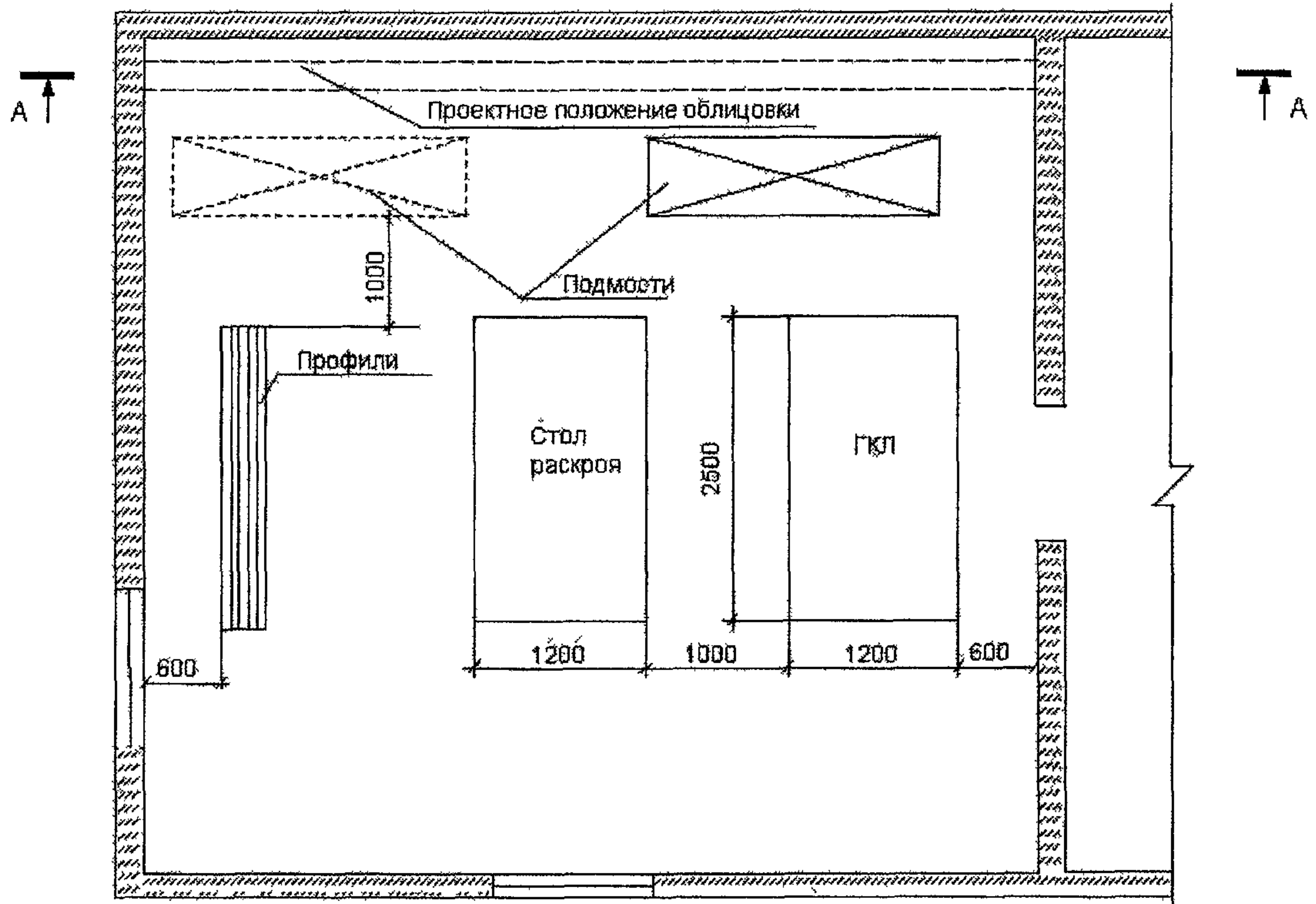
Рисунок 22 — Схема организации рабочего места при облицовке стен
