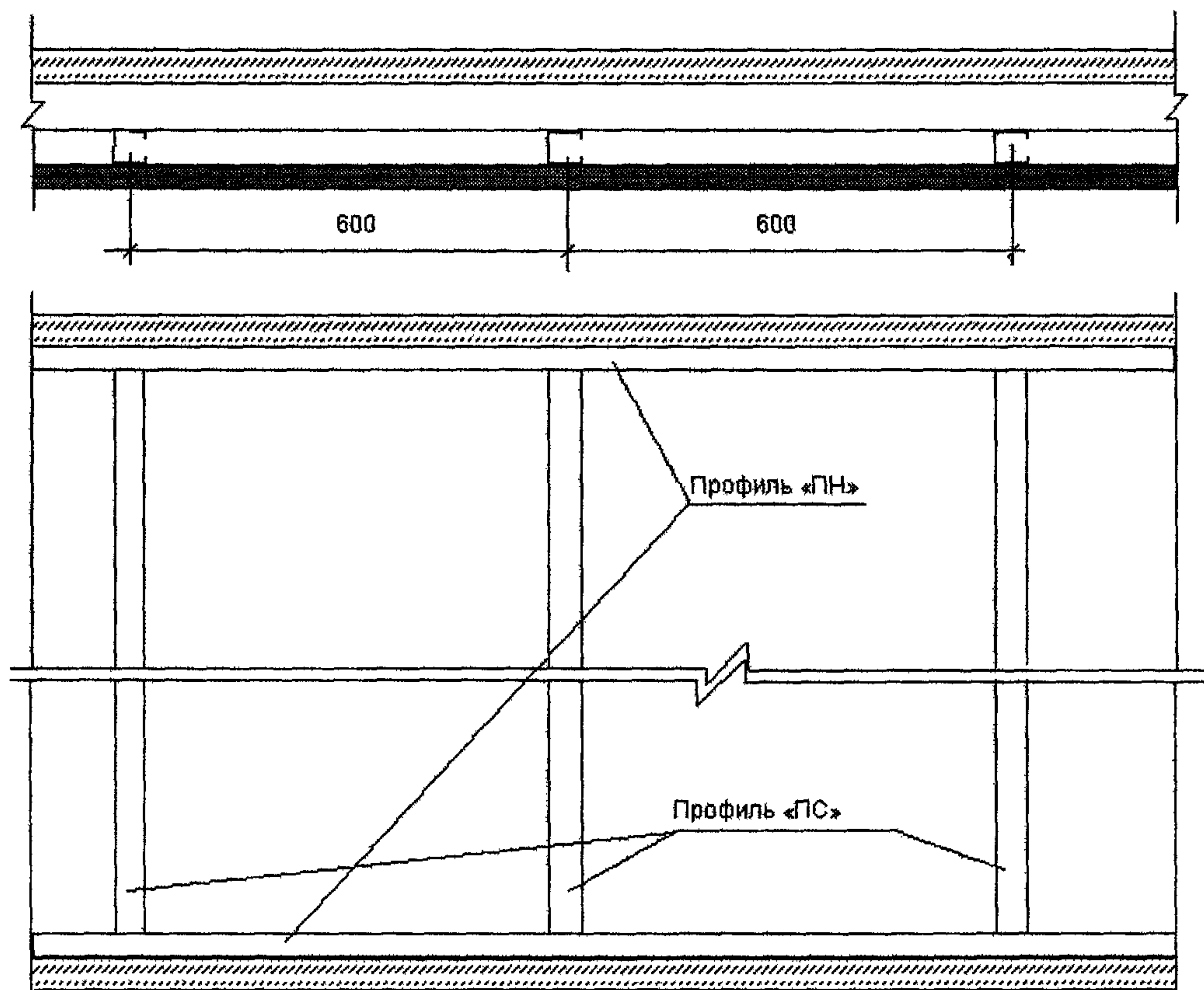
Рисунок 27 — Схема монтажа каркаса в облицовке С 626
