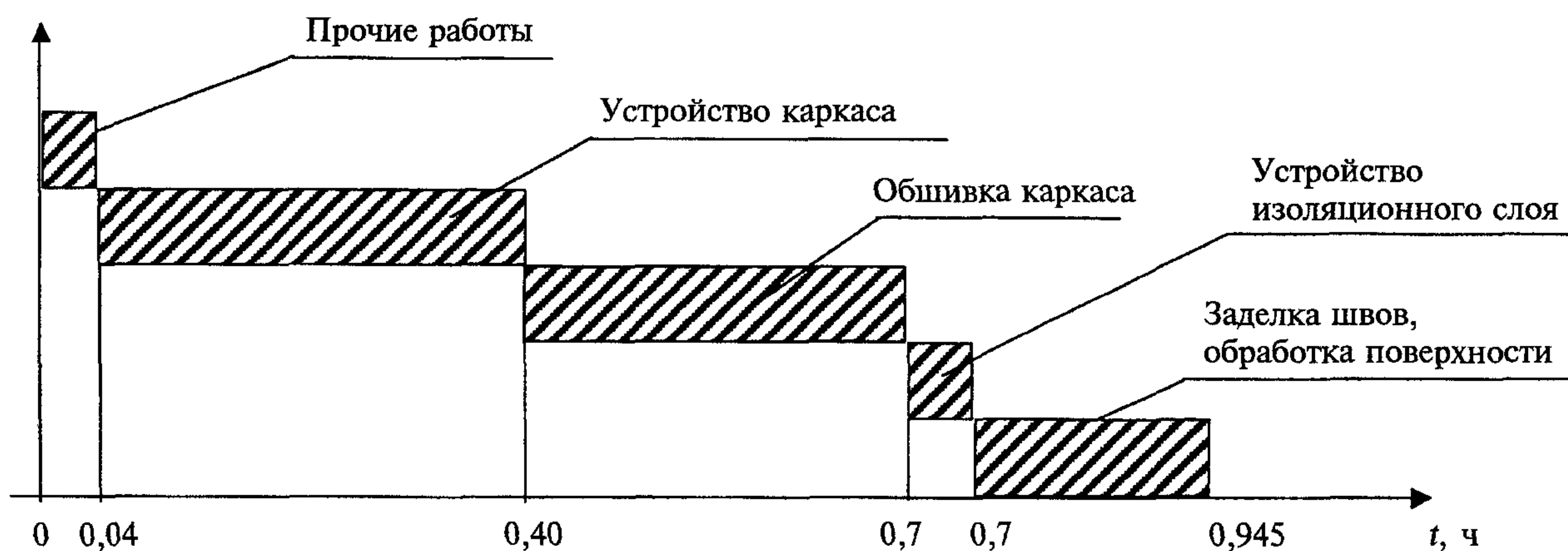
Рисунок 4.1 — График движения рабочей силы
