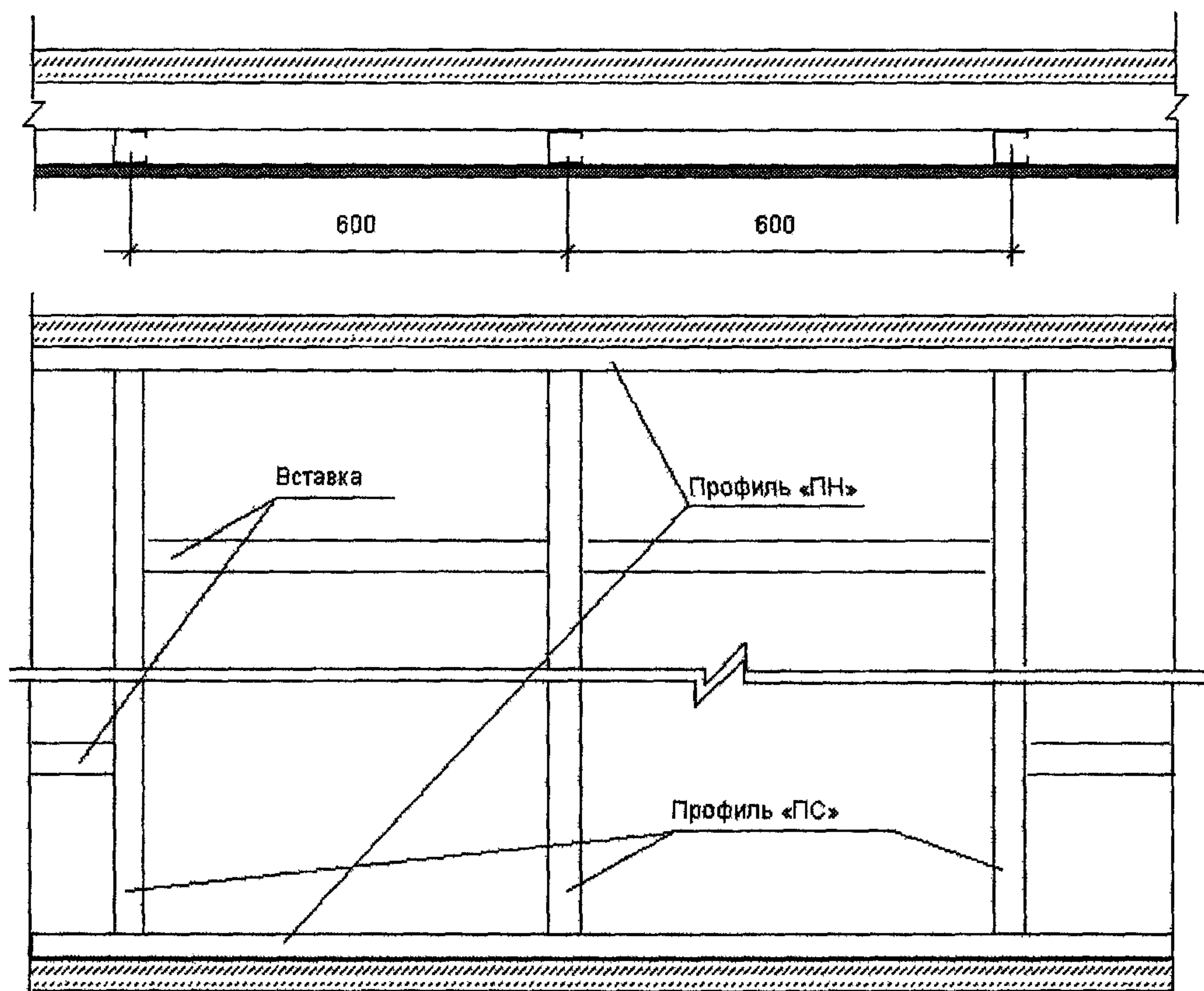
Рисунок 26 — Схема монтажа каркаса в облицовке С 625
