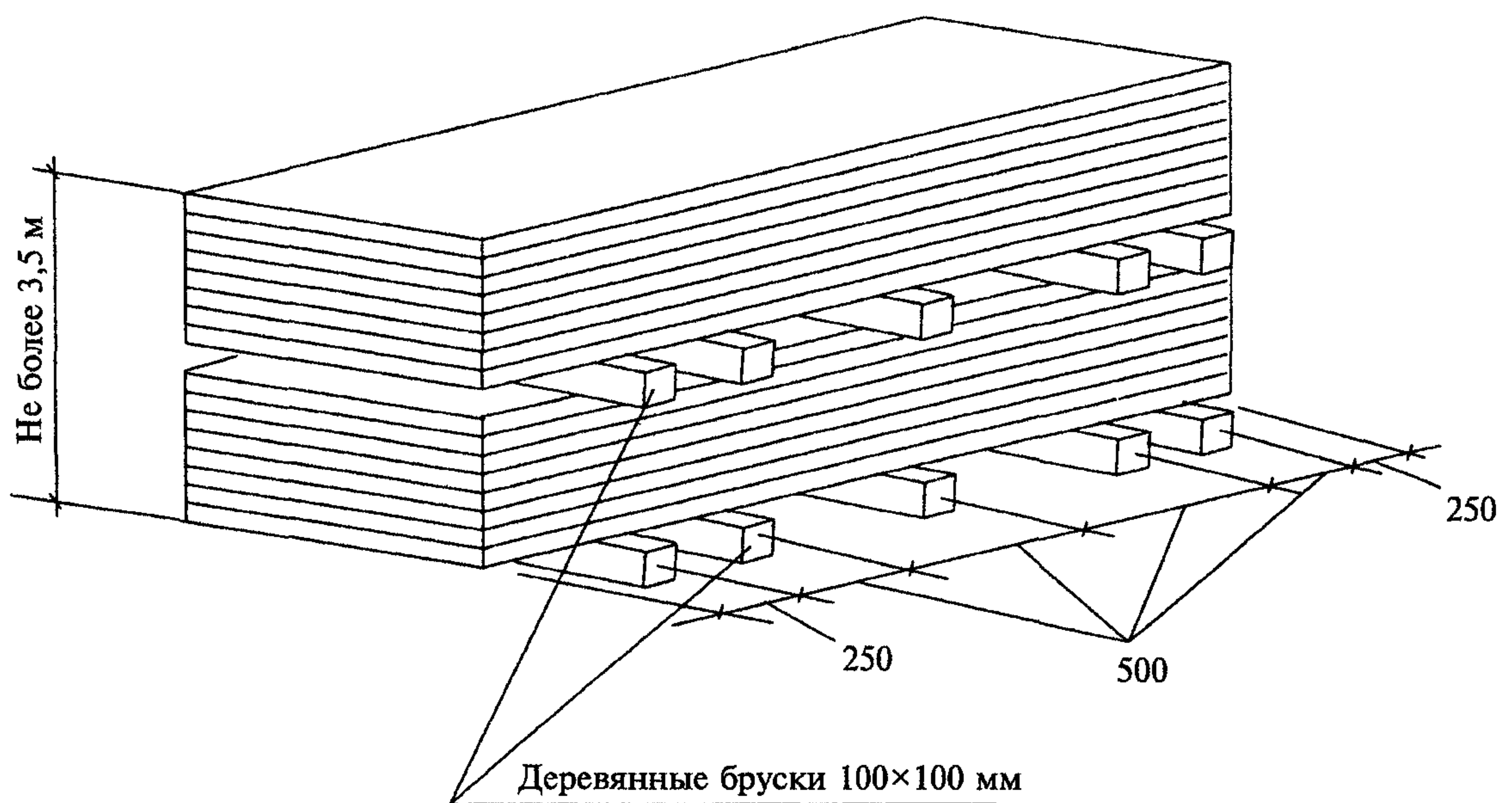
Рисунок 2 – Схема складирования ГКЛ на объекте
