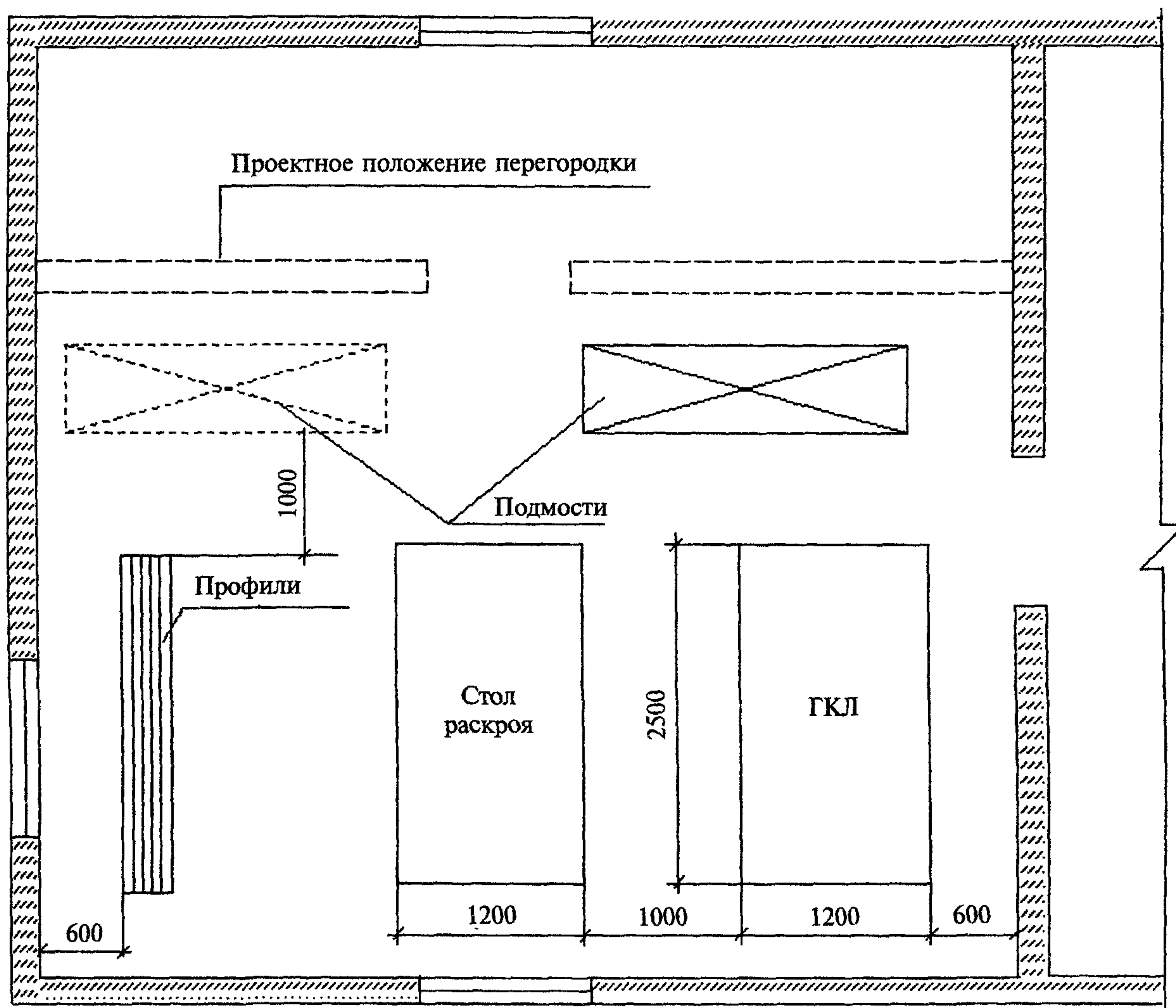
Рисунок 3 — Схема организации рабочего места
