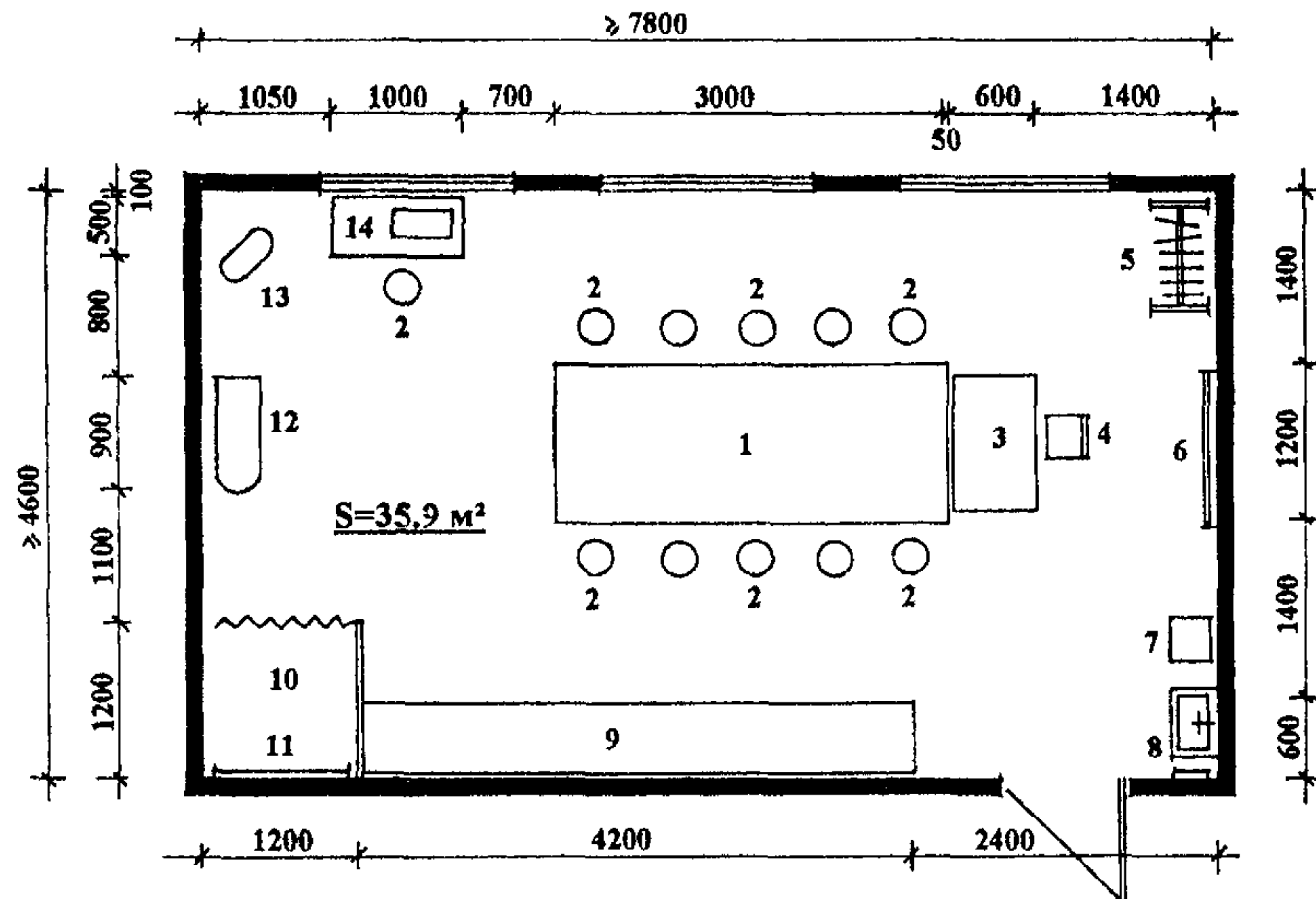
Экспликация оборудования
