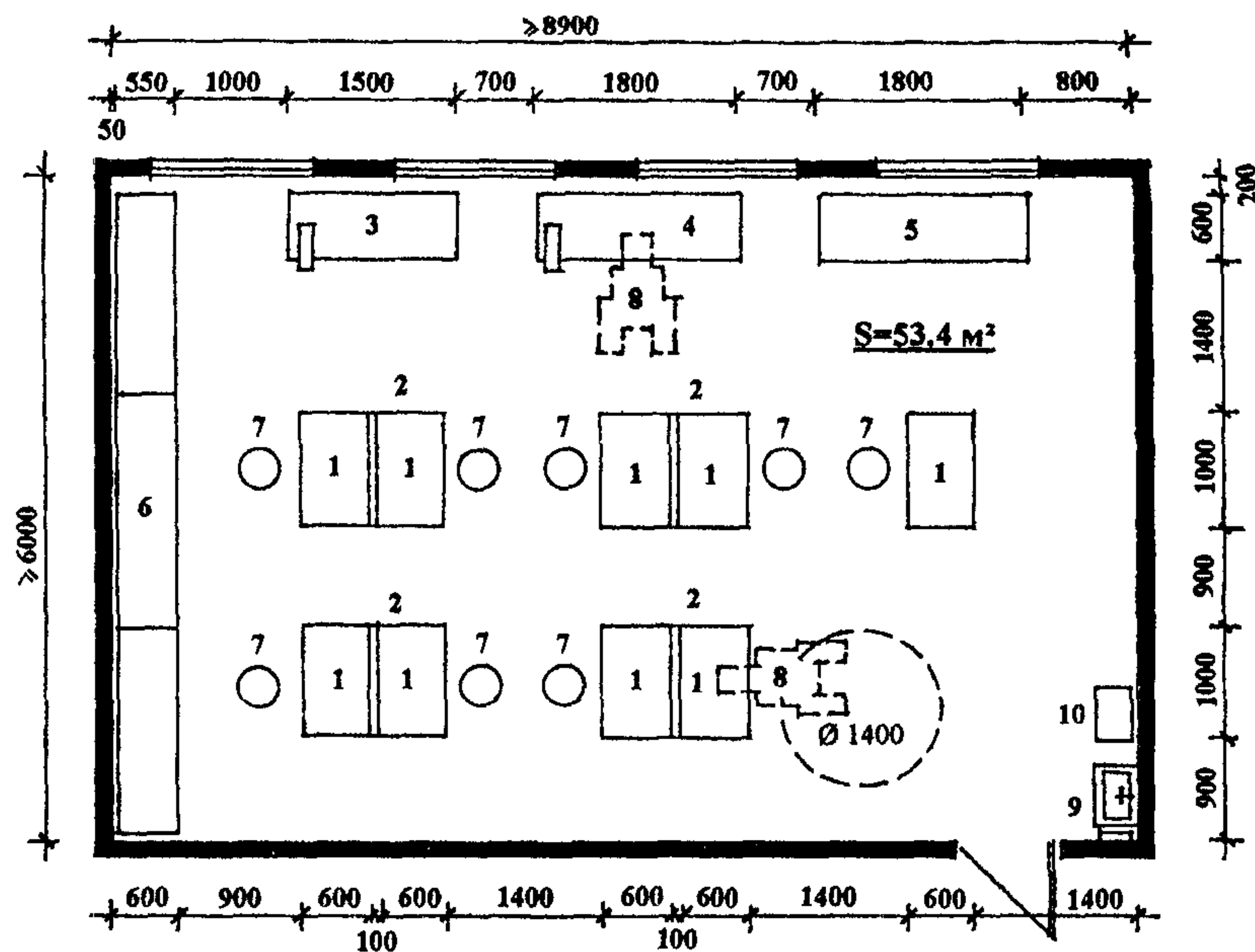
Экспликация оборудования
