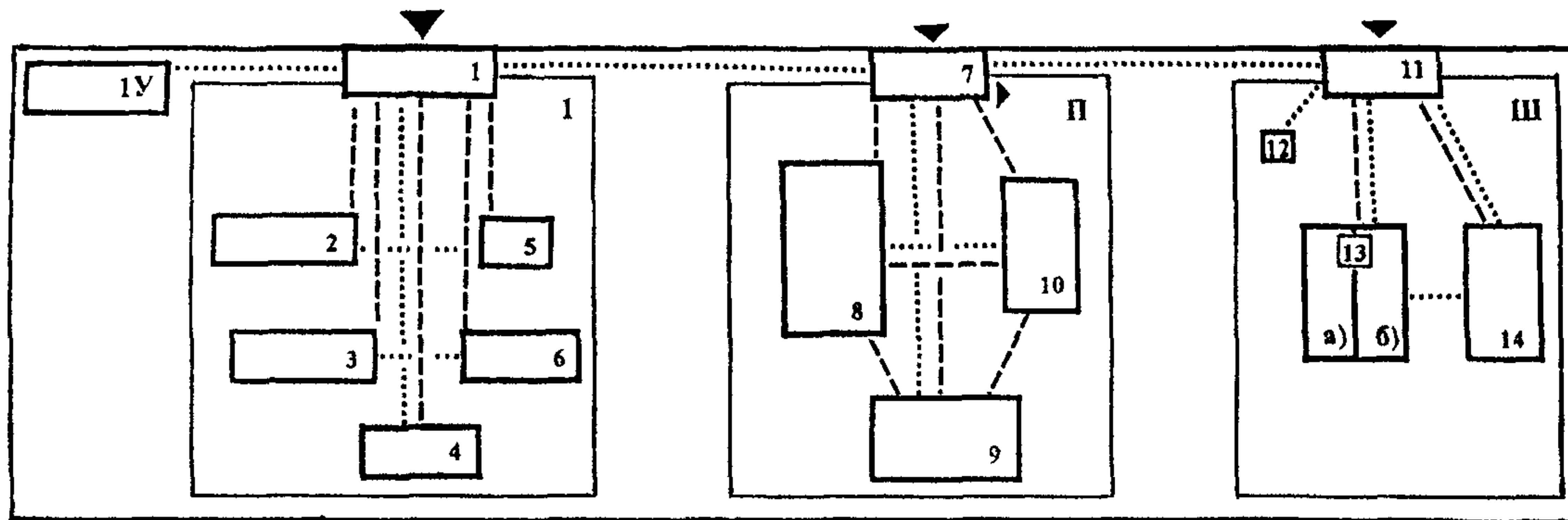
Рис. 1. Функционально-планировочная схема ЦСПСиД.
