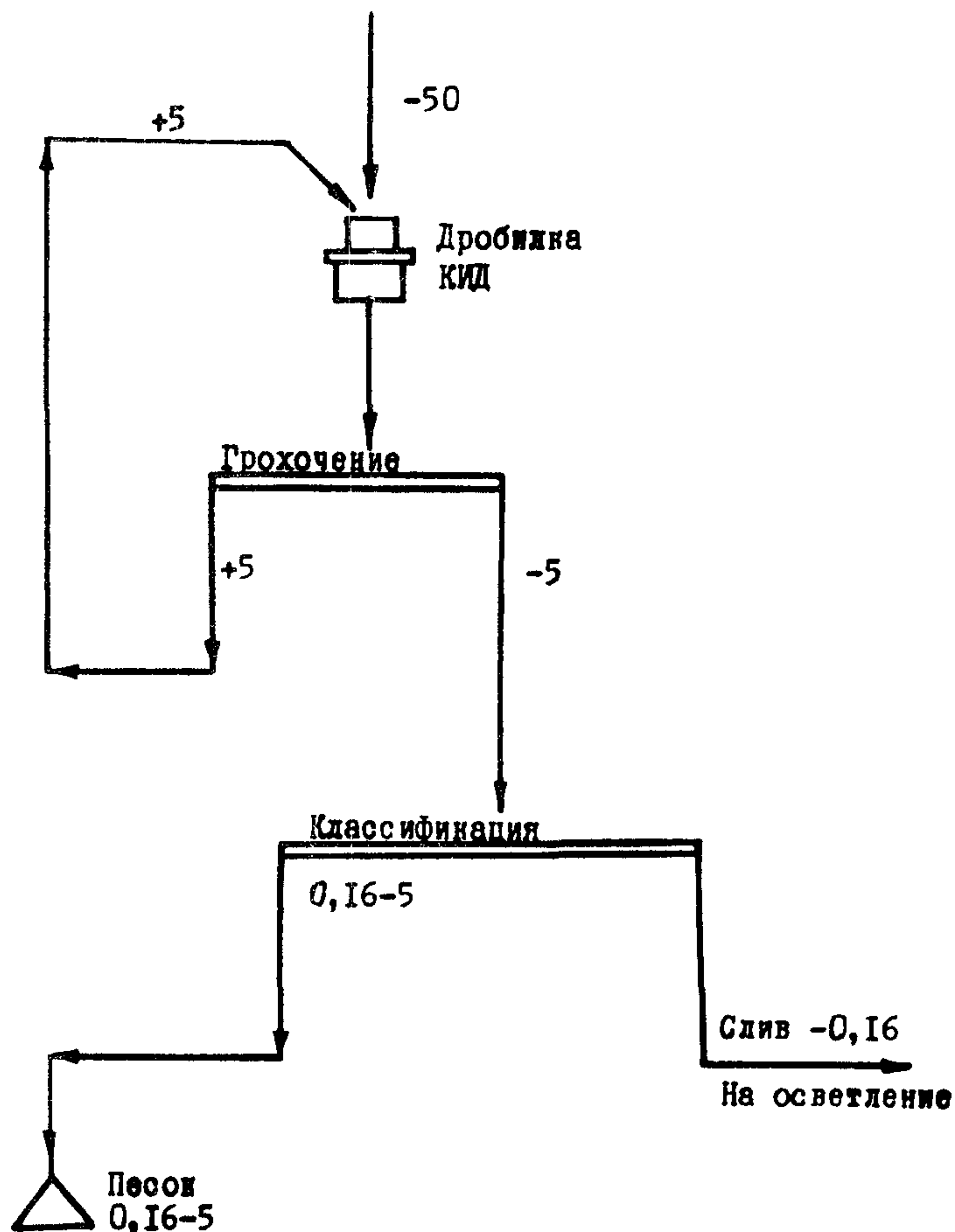
Рис.3. Технологическая схема получения песка дробленого с использованием Дробилки КИД-600
