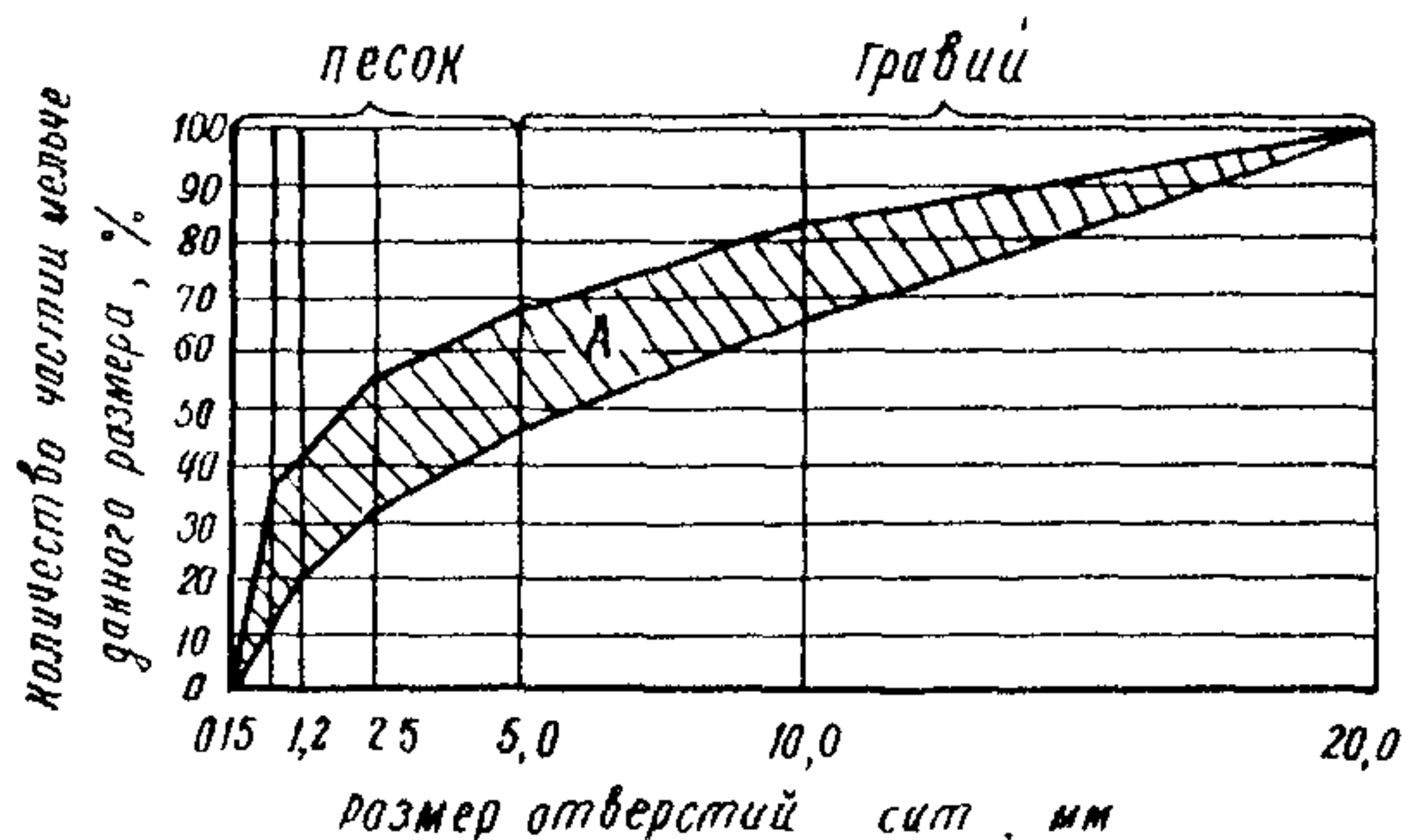
Рис. 5. Требуемый зерновой состав естественной гравийно-песчаной смеси
