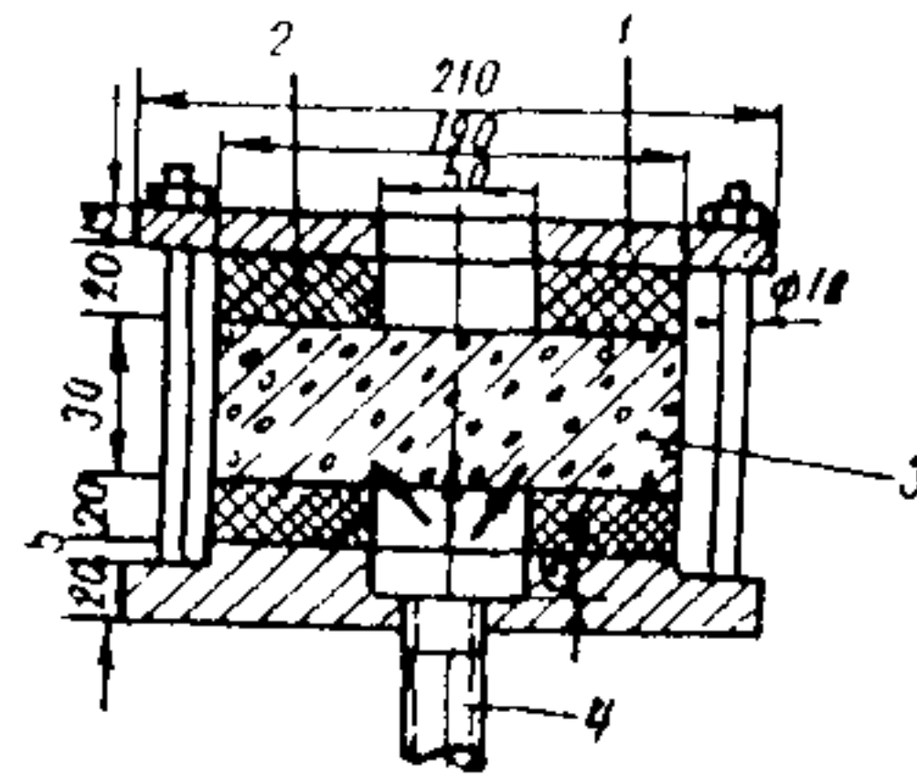
Прибор для испытания набрызг-материалов на водонепроницаемость:
