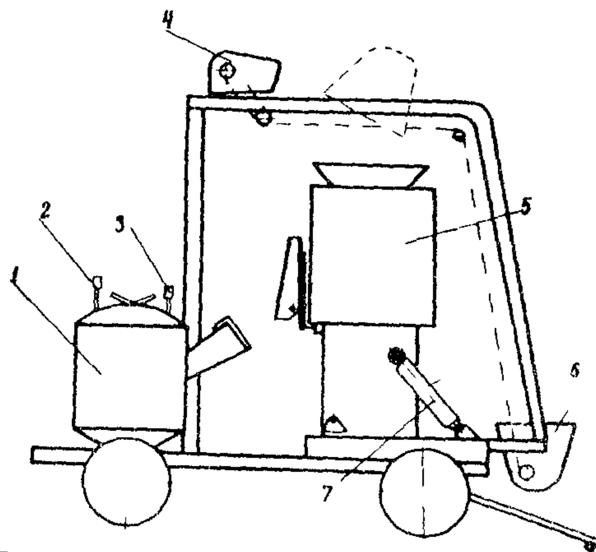
Рис. 13. Схема установки для приготовления и укладки аэроцемя:
