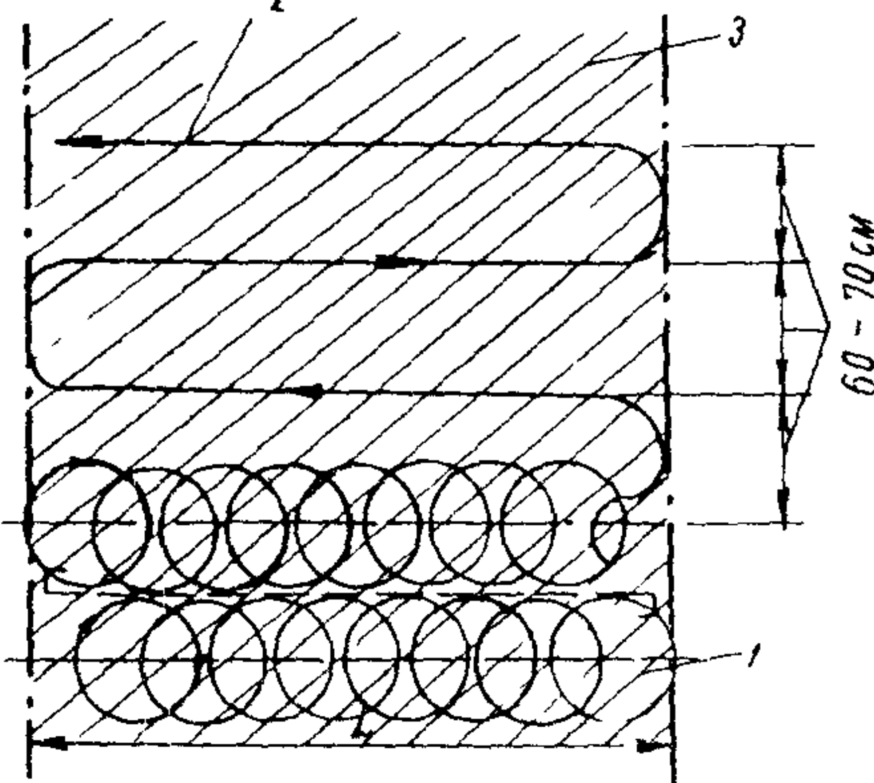
Рис.18. Порядок перемещения сопла при пневмонабрызге:
