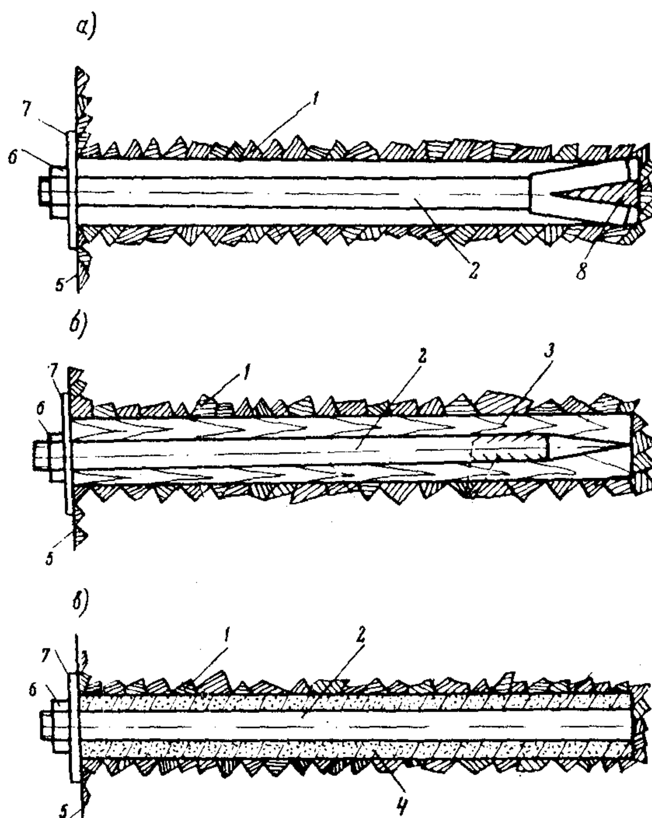
Рис. 6. Конструкции монтажных анкеров: а - клино-щелевой; б - в деревянной пробке; в - в монолитном цементобетоне (растворе);
