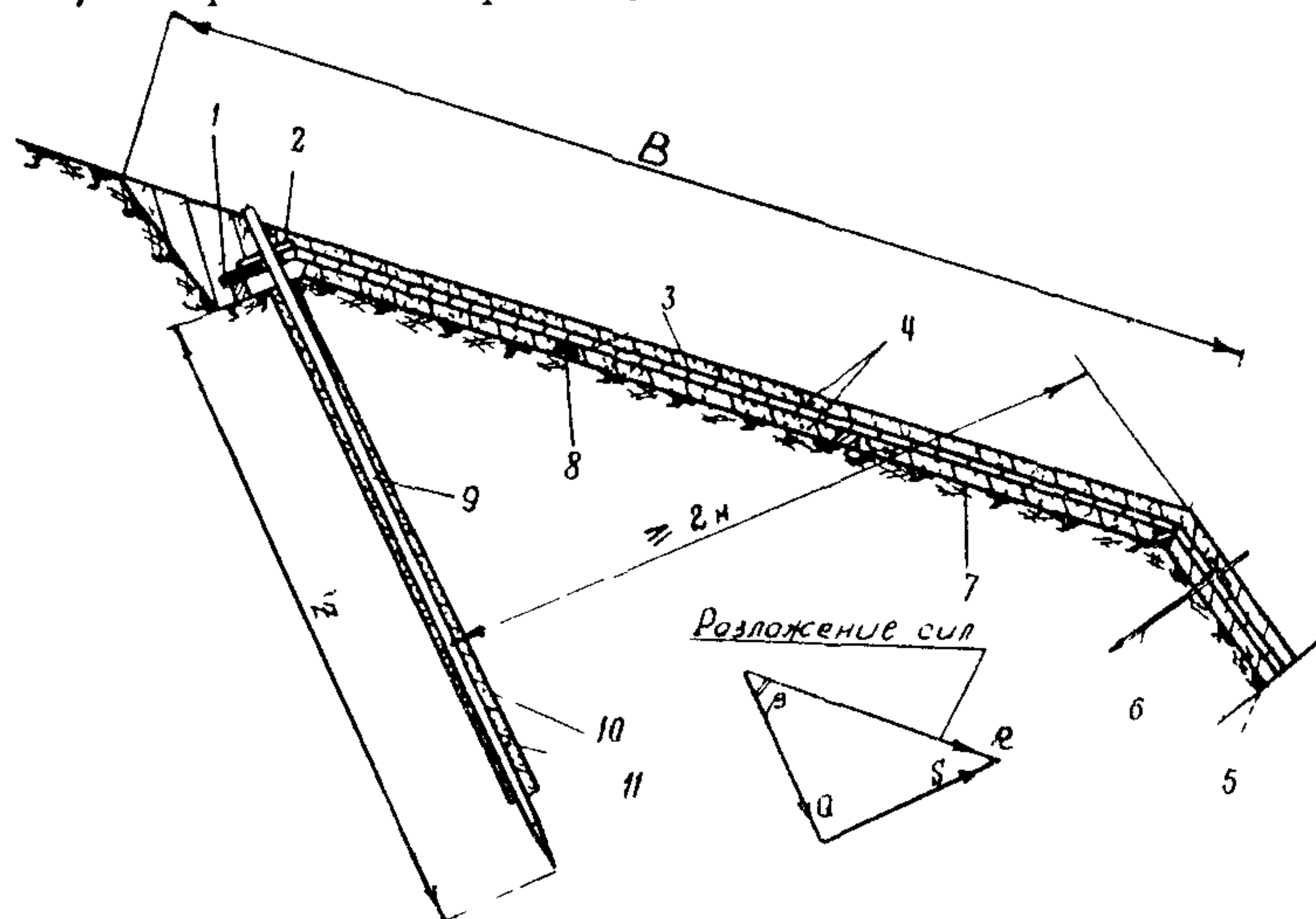
Рис. 2. Конструктивная схема защитного покрытия из пневмонабрызга:
