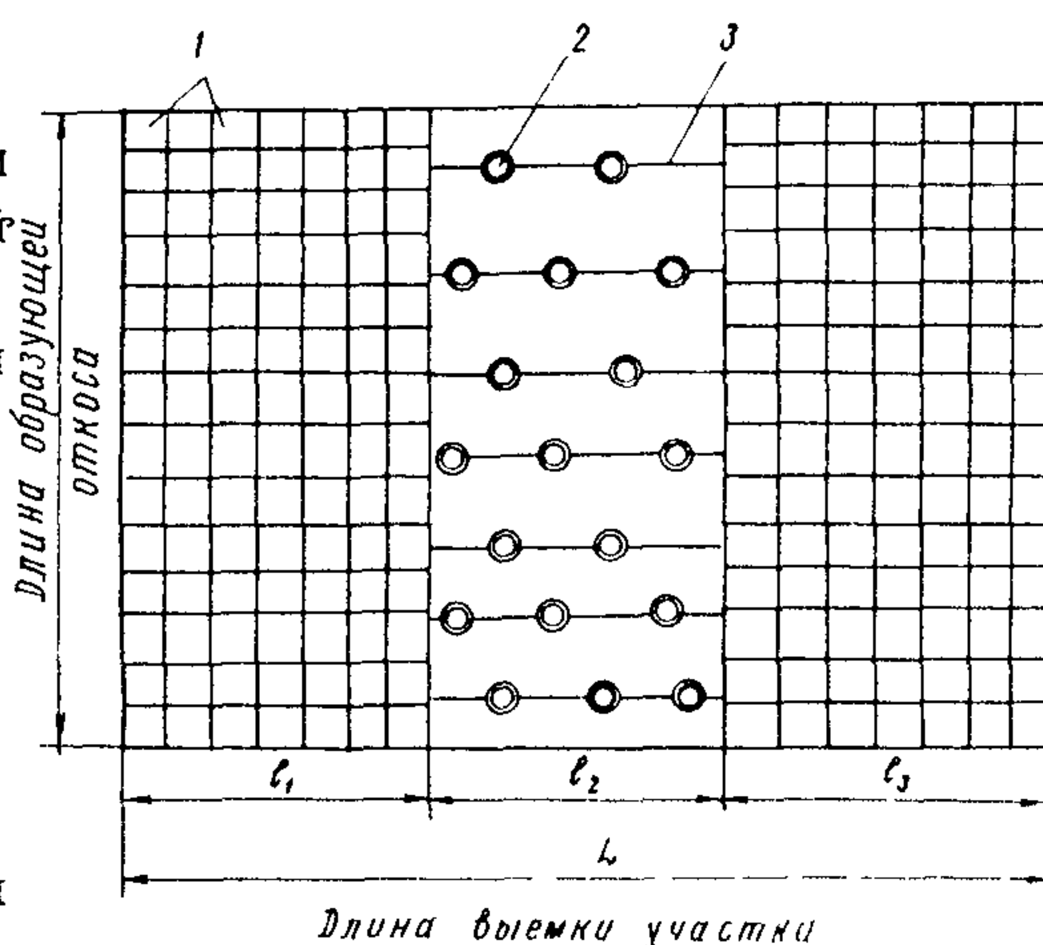
Рис. 3. Распределение монтажной сетки на поверхности скального откоса:
