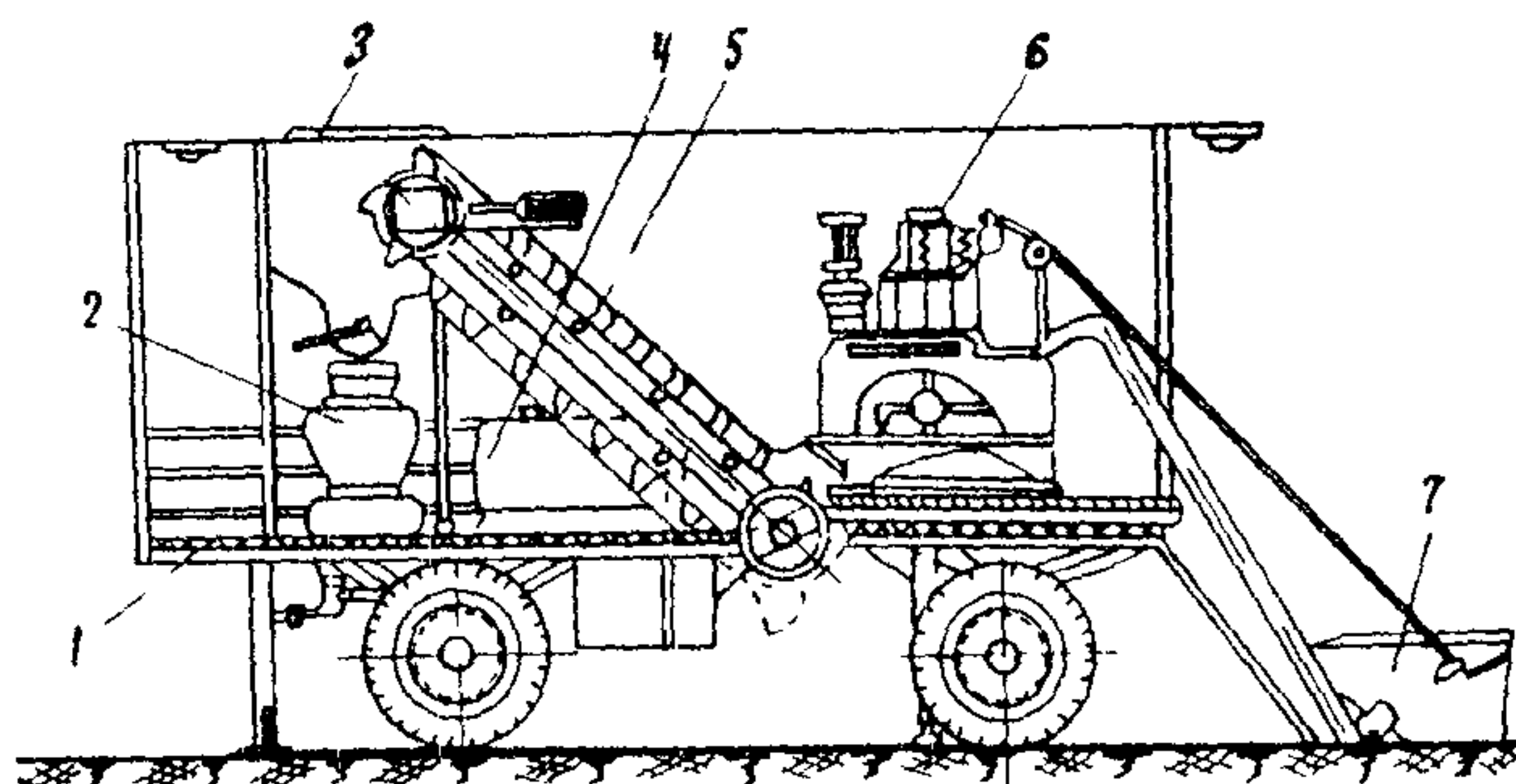
Рис. 15. Передвижная бетонировочная станция (ПБС):
