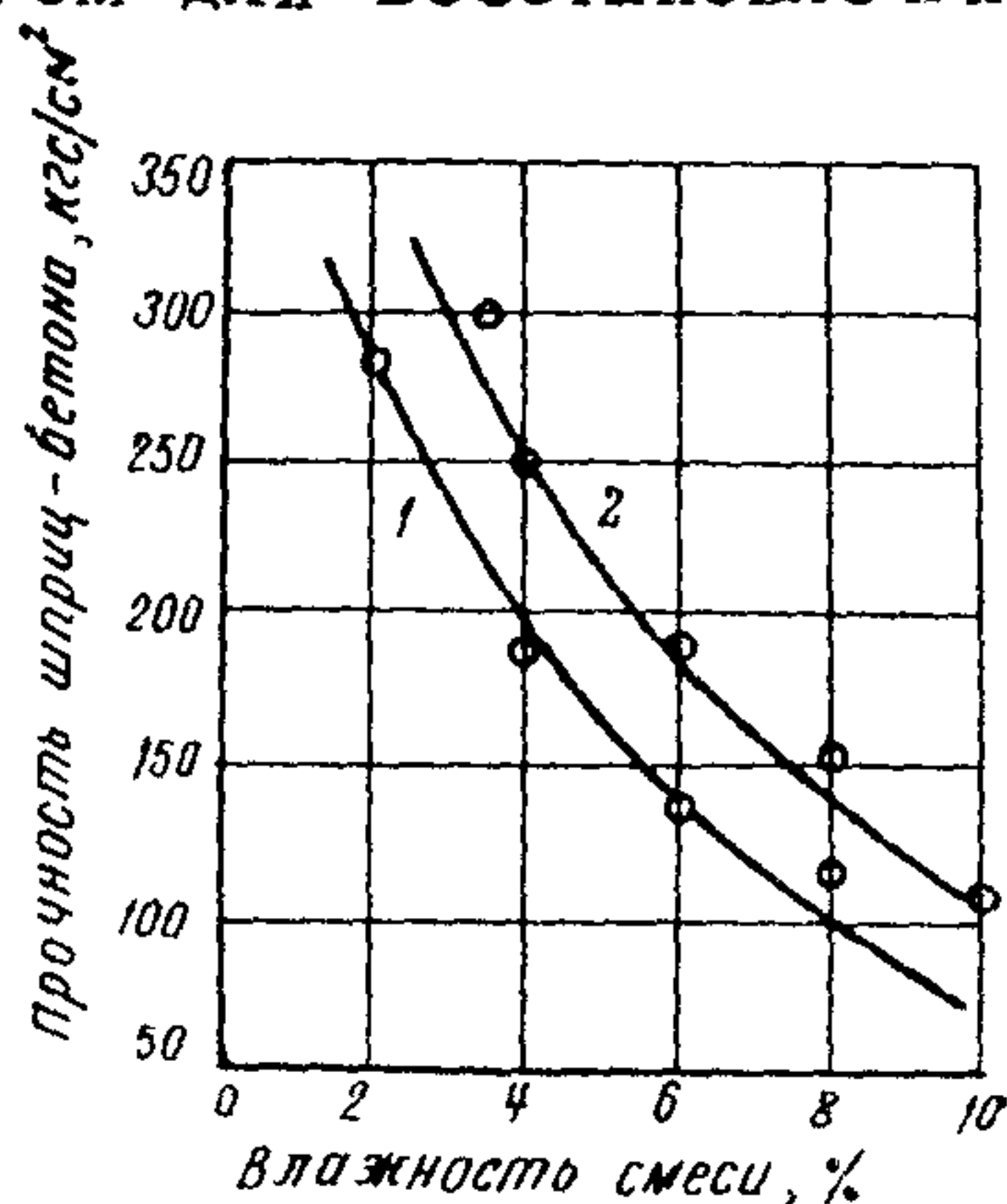
Рис. 8. Изменение прочности шприц-бетона в зависимости от влажности сухой смеси при ее шестичасовом хранении:
