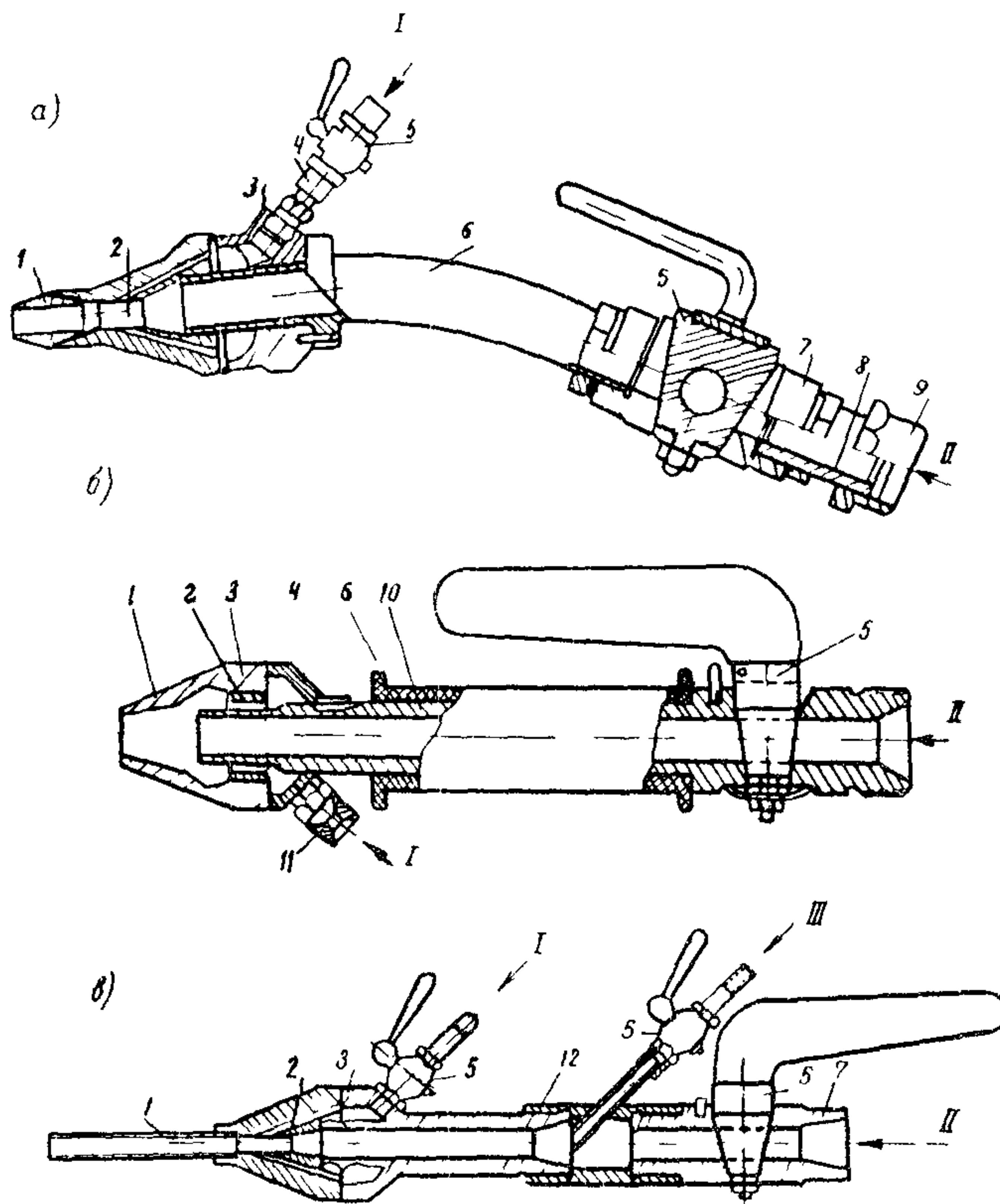
Рис. 9. Схема конструкции пистолета:
