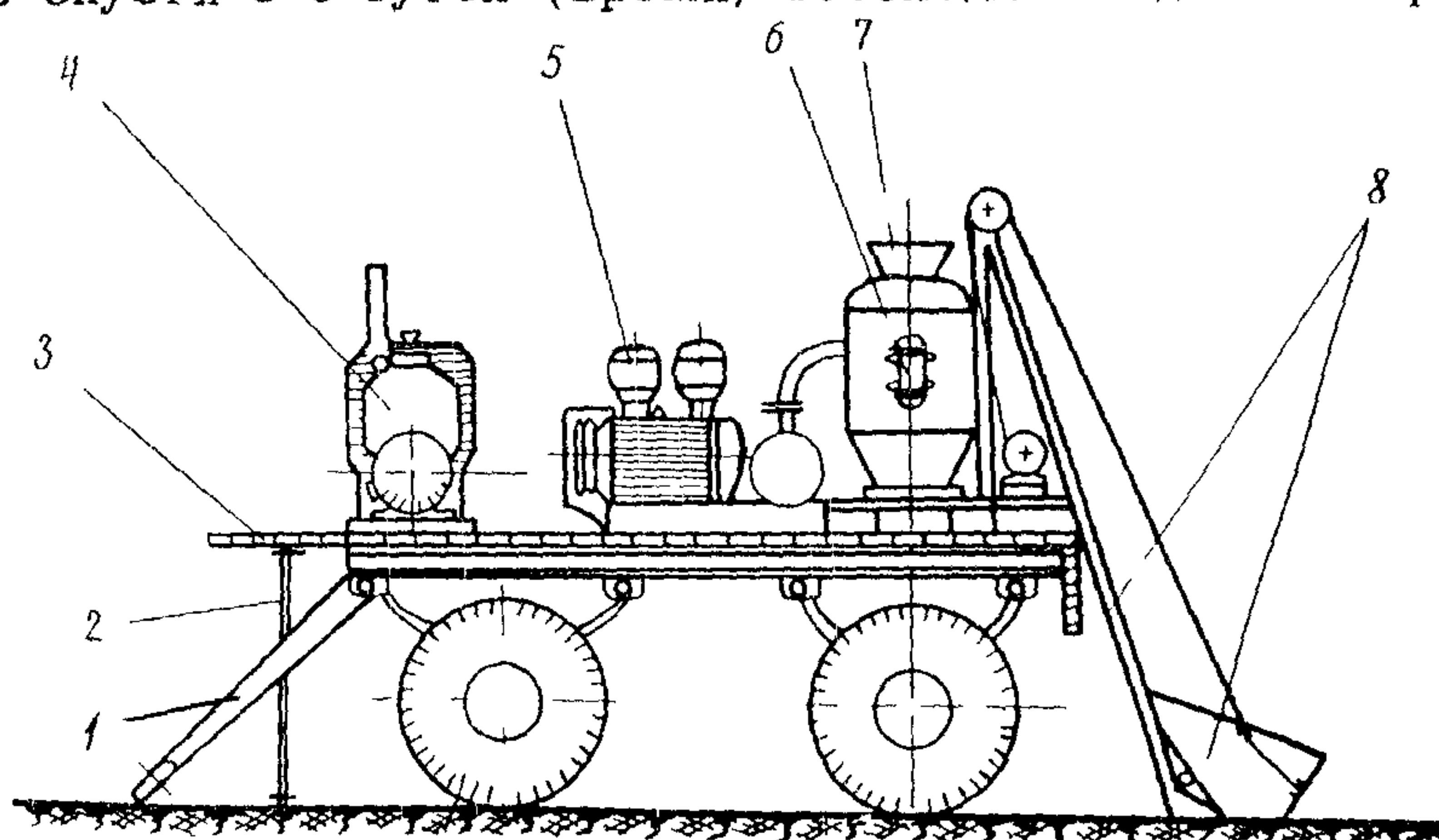
Рис. 16. Передвижной комплект Союздорнии для пневмо-набрызга:
