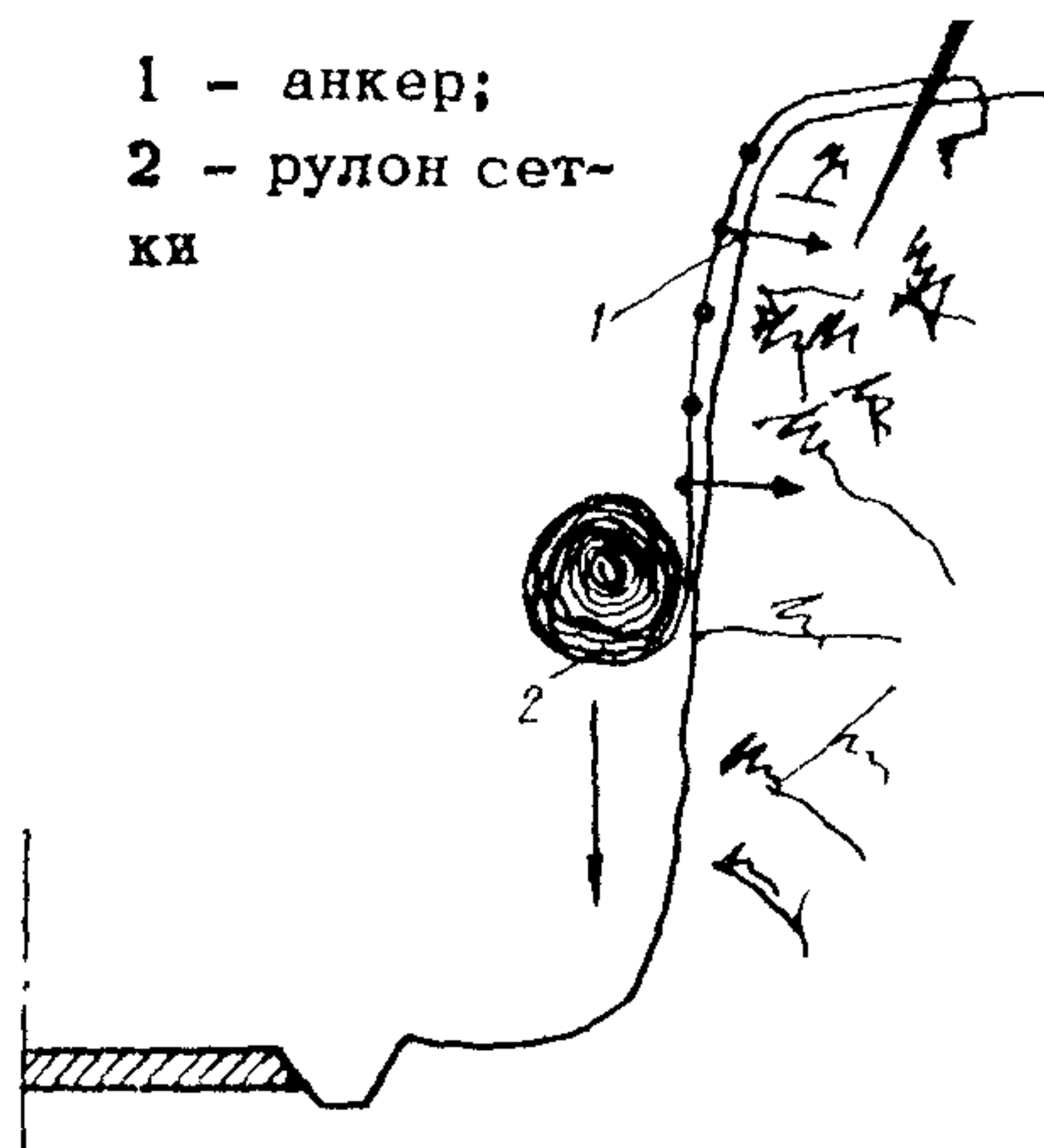
Рис. 7. Монтаж сетки:
