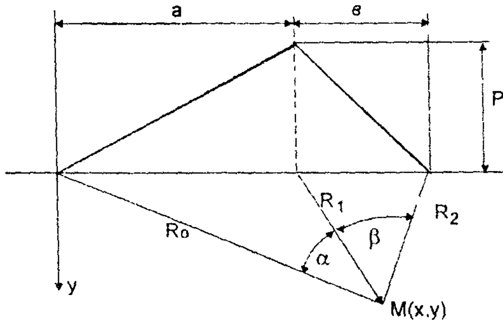
Рис. 3. Оценка напряженного состояния при нагрузке в виде разностороннего треугольника (несимметричного клина)
