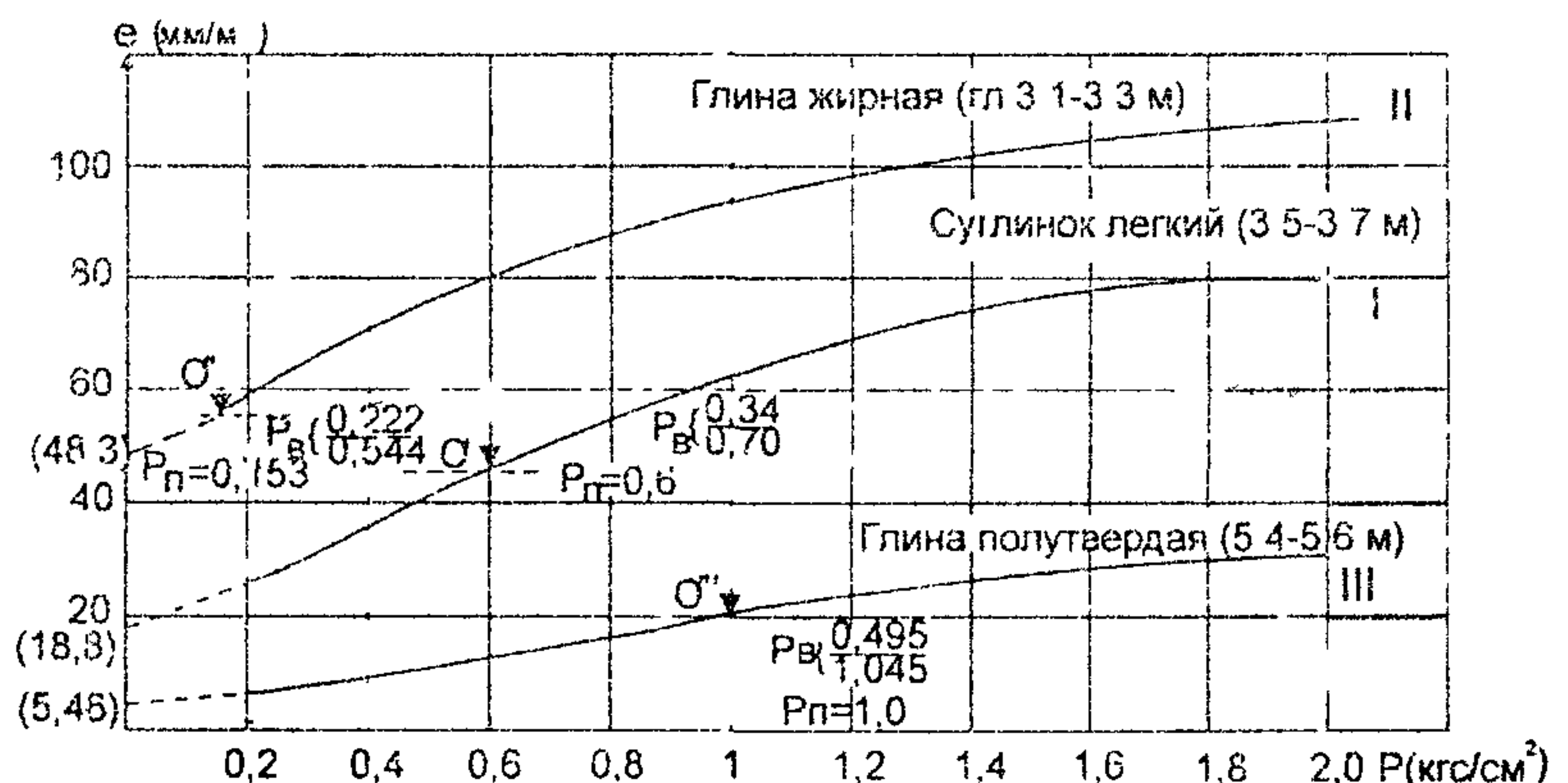
Рис. 5. Результаты компрессионных испытаний образцов грунта
