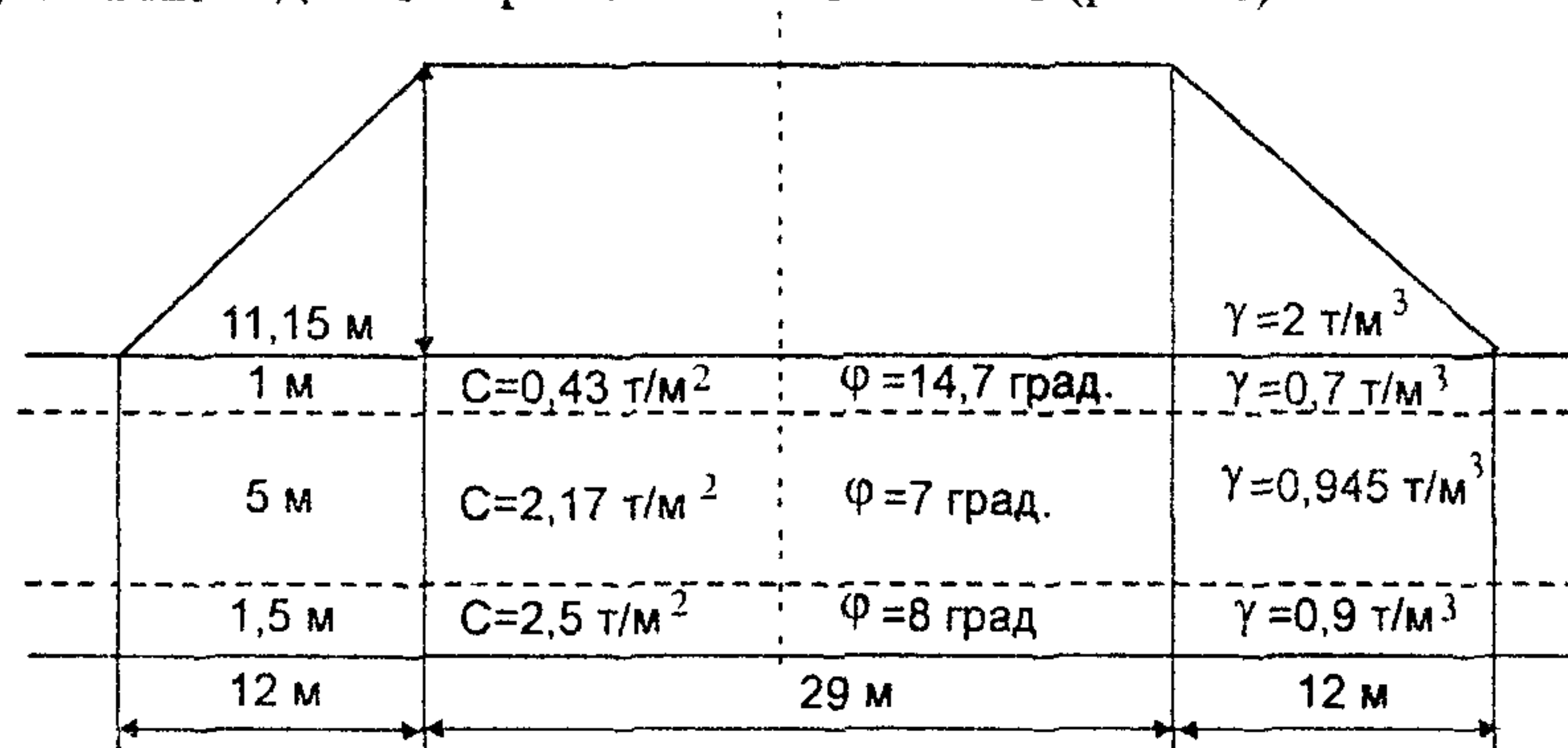
Рис. 6. Схема насыпи на слабом слоистом основании: вариант I – K_{без}=0,56 , S=49,92 см, T=45,96 мес; вариант II – соответственно 0,56, 26,21 см, 3,40 мес
