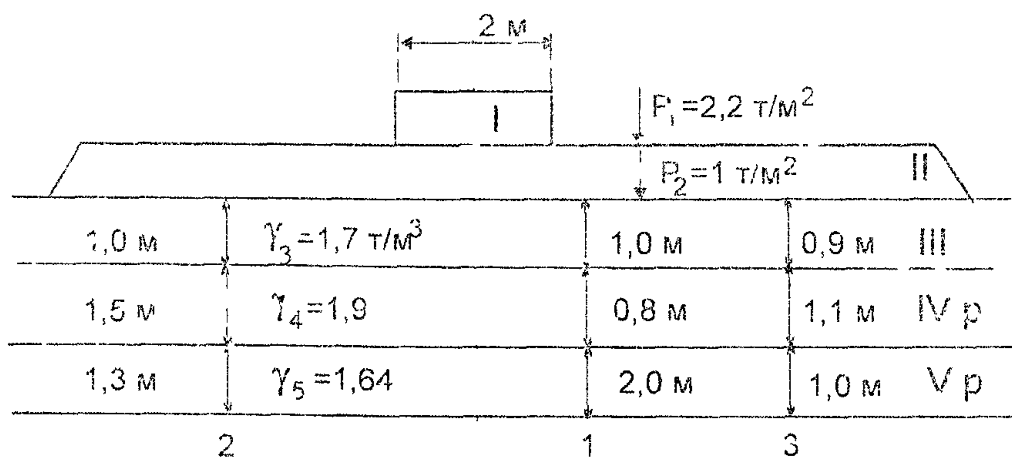
Рис 8. Расчетные схемы для контрольных точек 1, 2 и 3
