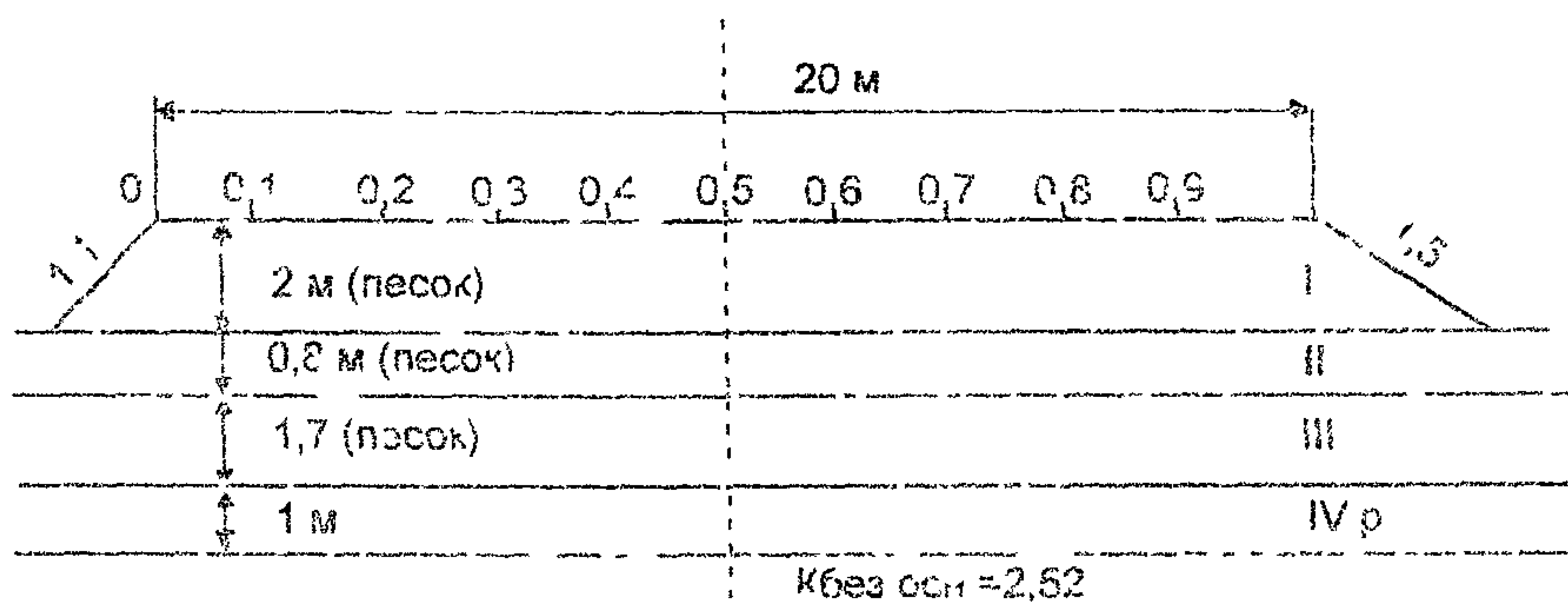
Рис. 7 Схема расчета осадки насыпи в разных точках
