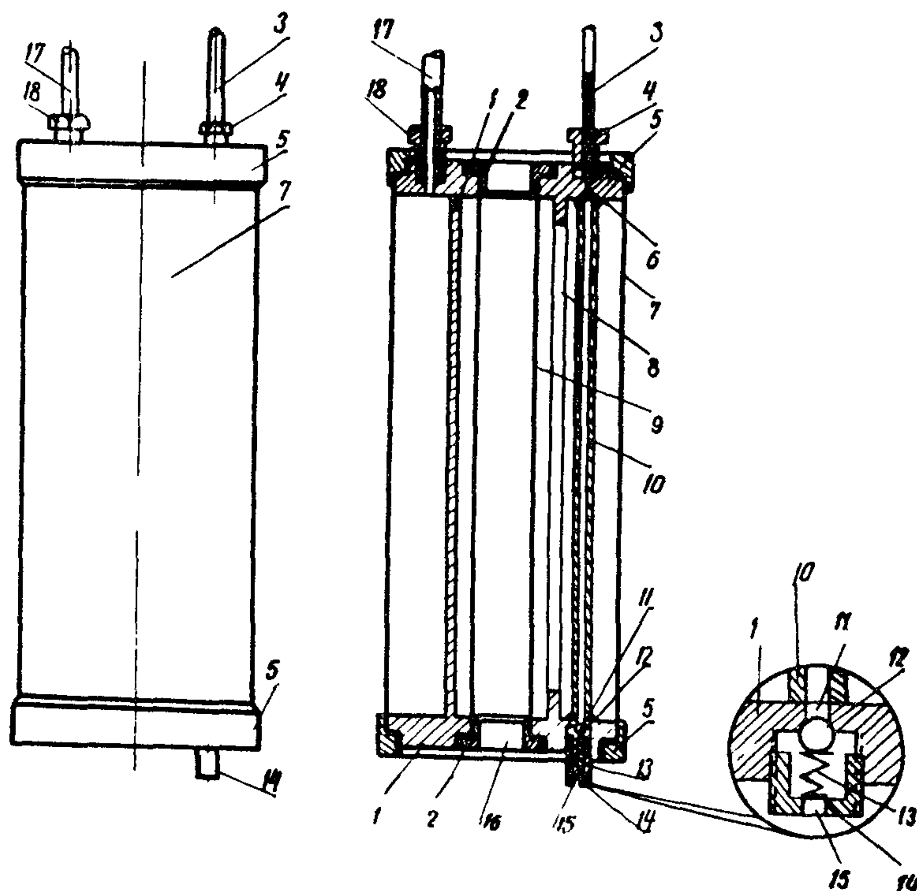
Рис.1. Схема конструкции иньектора:
