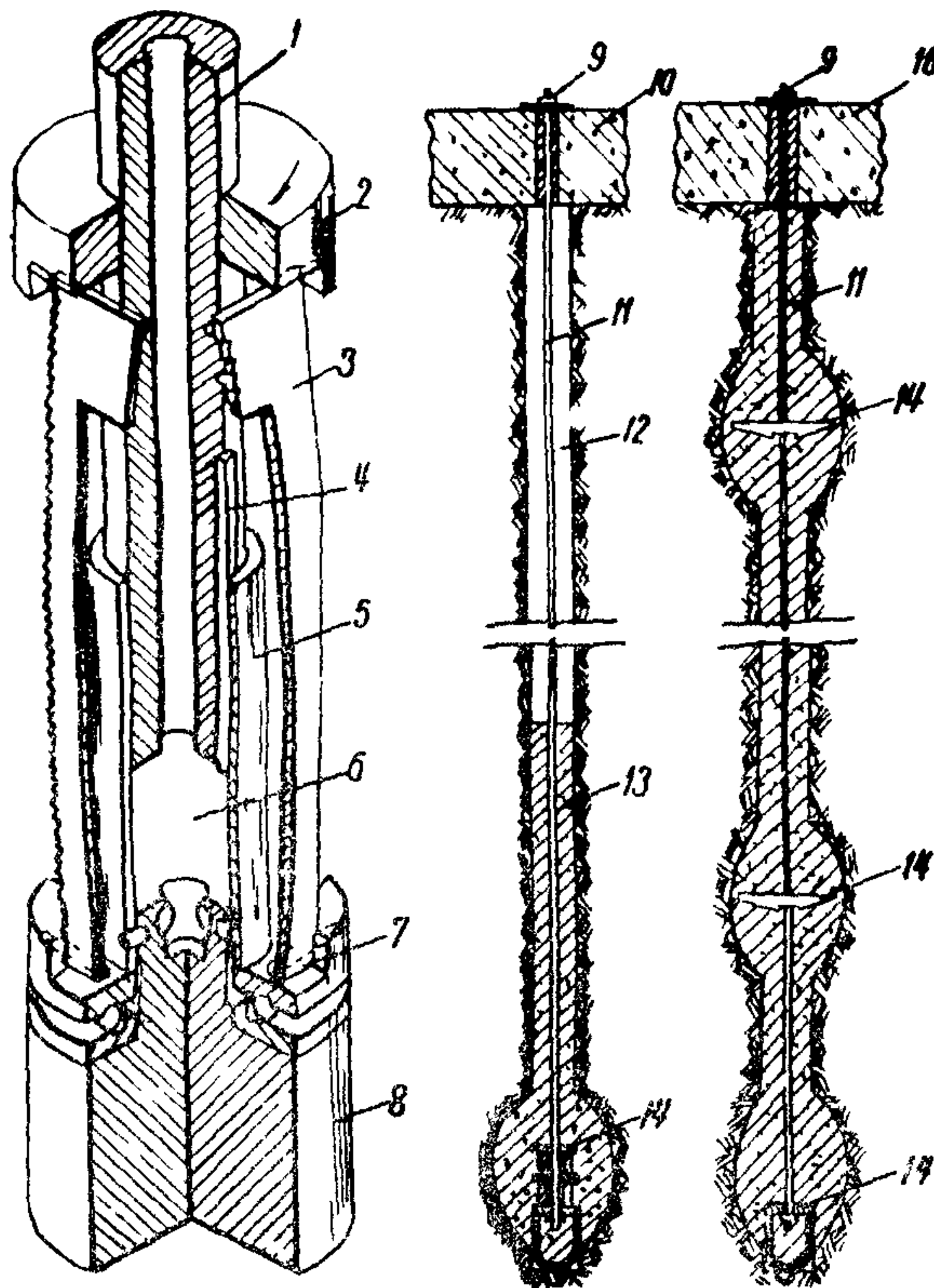
Рис.5. Уширитель скважины и анкерное крепление (патент США № 320075, кл. 81-39) : 1-сердечник; 2-верхний фланец; 3-нож; 4-замковое соединение; 5-направляющая труба; 6-полость; 7-ролковая опора; 8-нижний фланец; 9-верхний анкер; 10-бетонная плита; 11-стержень; 12-скважина; 13-бетонный раствор; 14-нижний анкер
