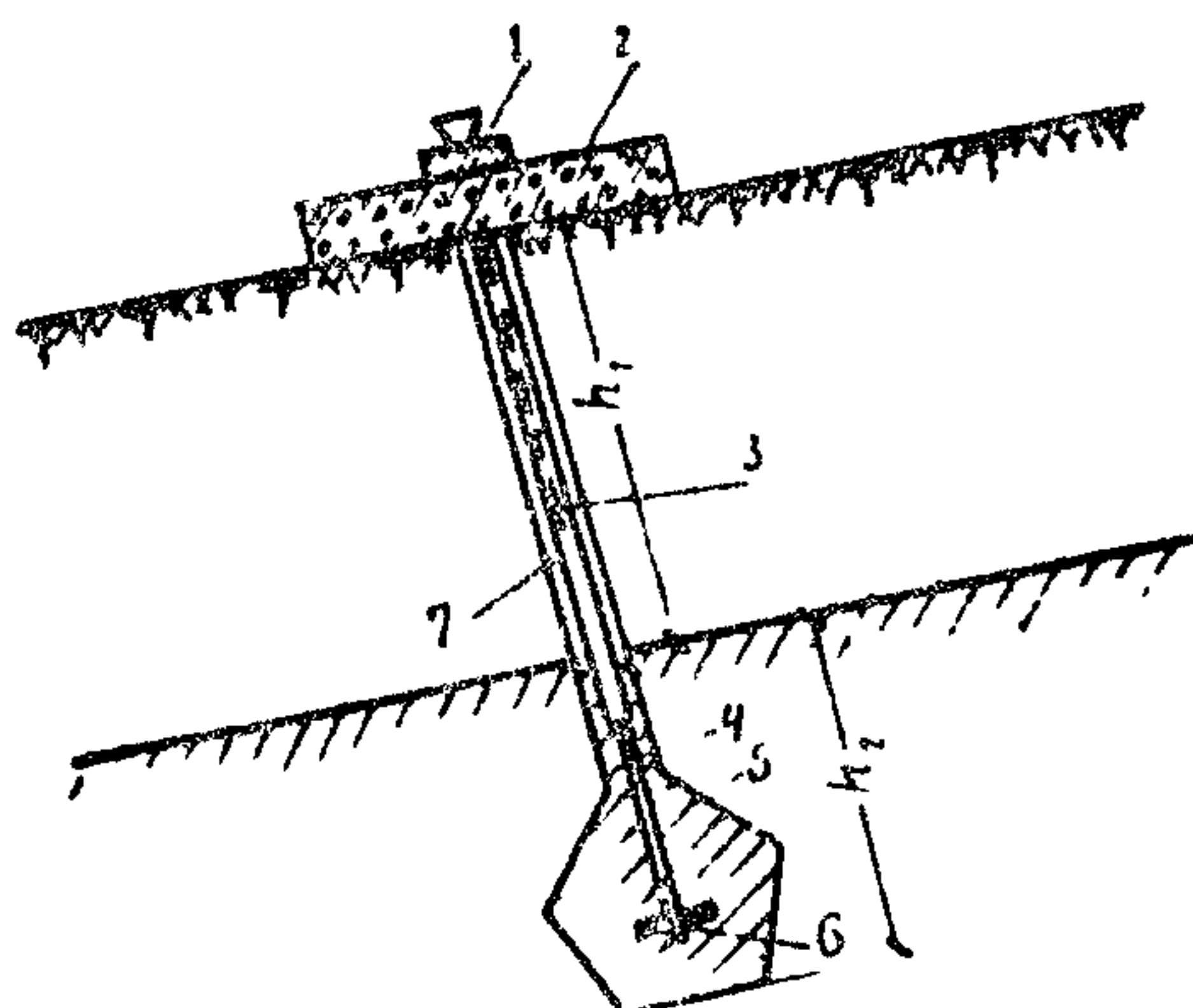
Схема анкерной затяжки:
