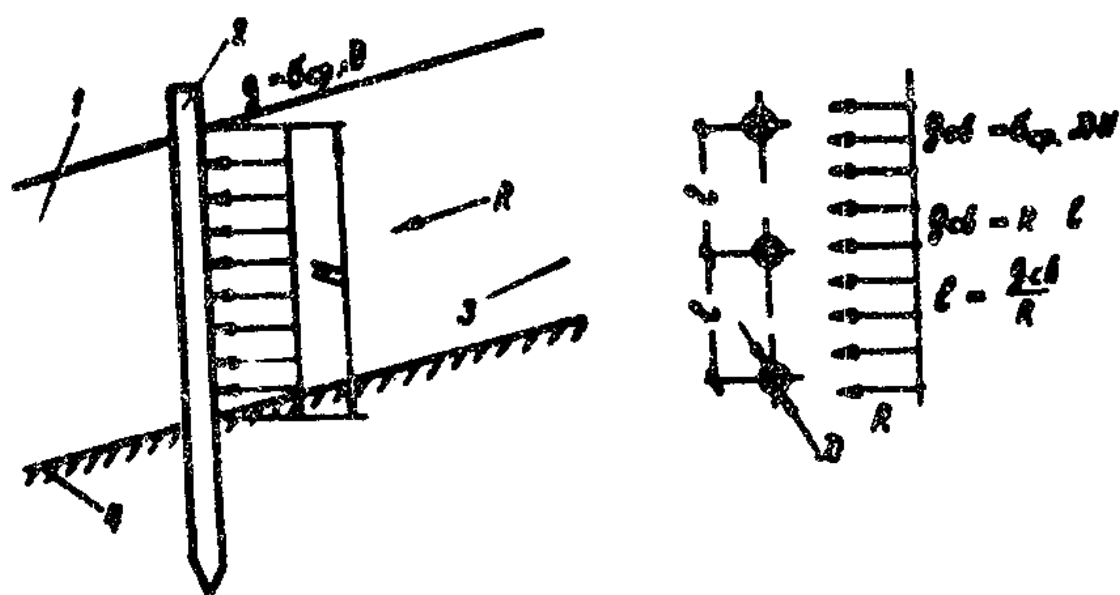
Рис.1. Расчетная схема к определению расстояний между осями свай в рядах :
