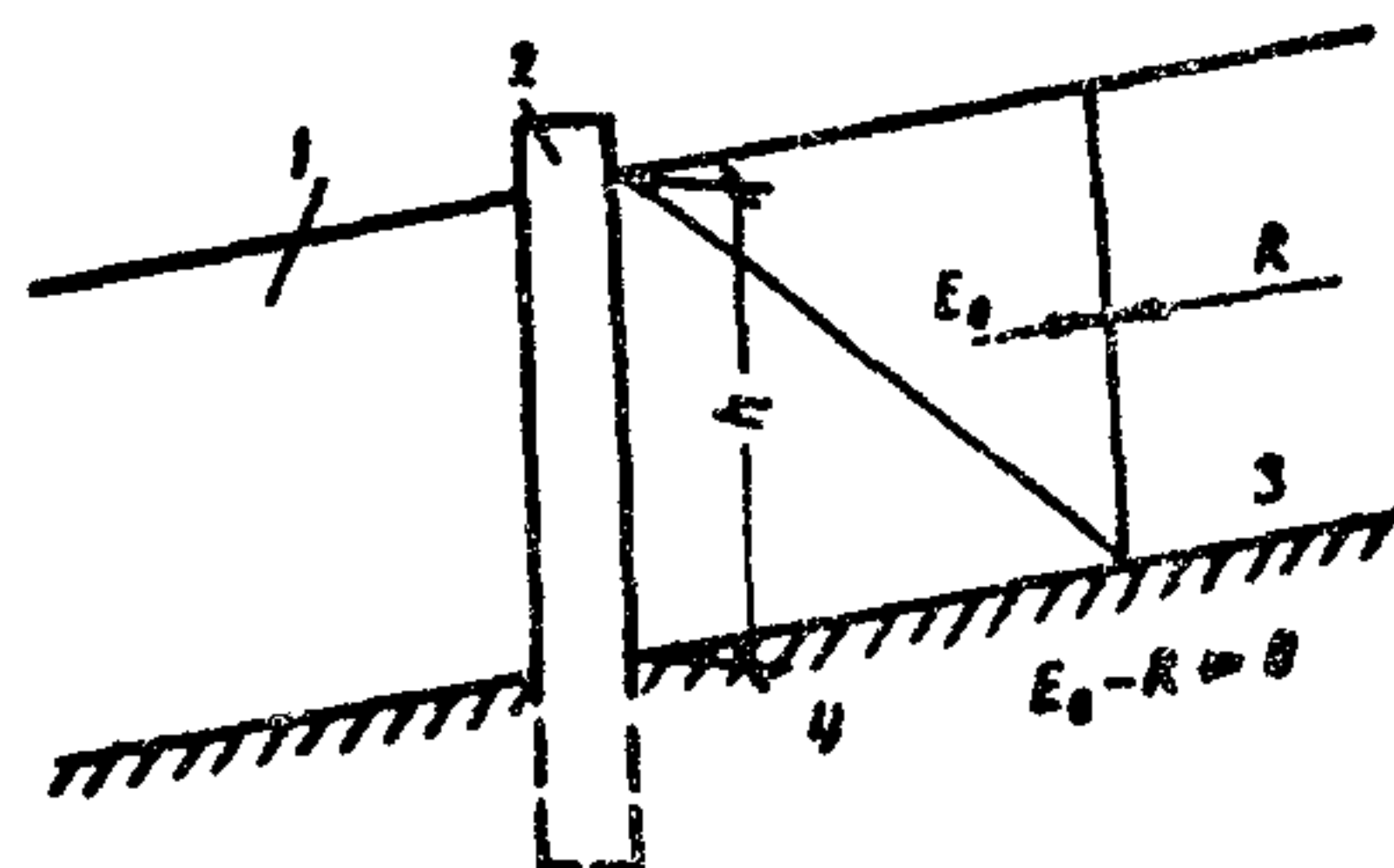
Рис.2. Расчетная схема к проверке свайной удерживающей конструкции на возможность переползания ее грунтом оползневого массива : 1—оползневое тело; 2—свая; 3—поверхность скольжения; 4—коренные породы
