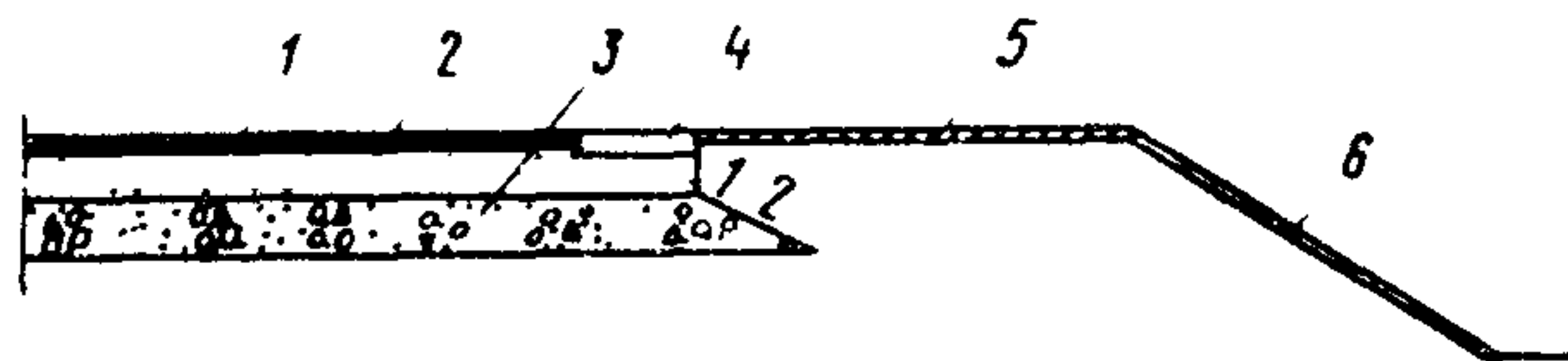
Рис.5. Двухслойная теплоизоляция из битуминированного аглопорита:
