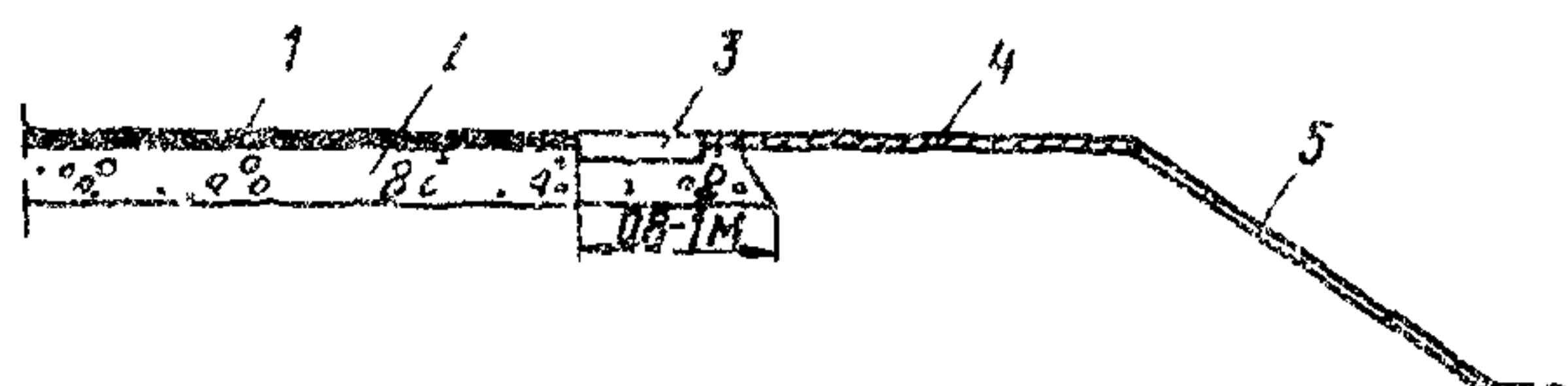
Рис.4. Теплоизоляция из битумоминеральной смеси;
