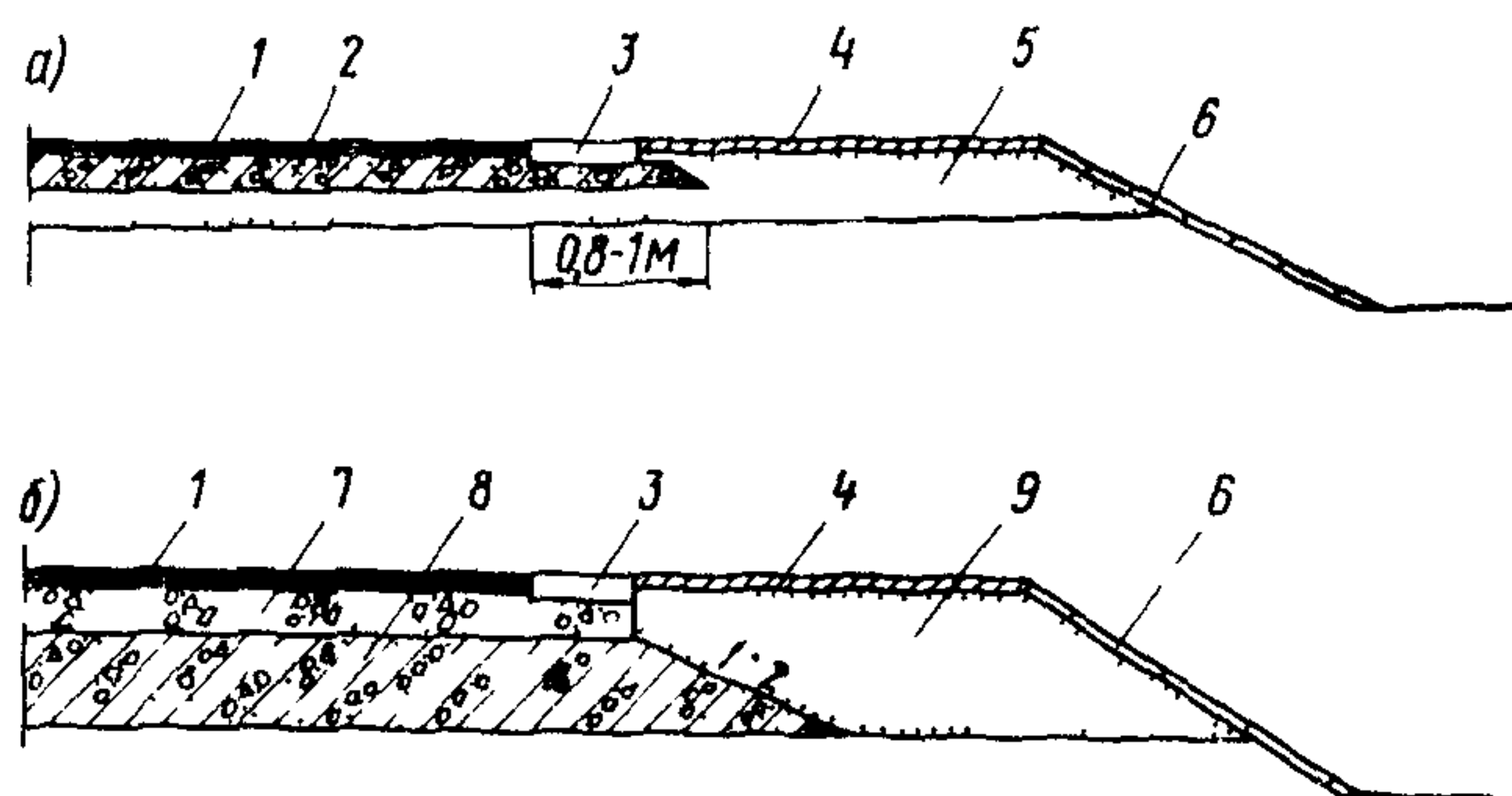
Рис.2. Конструкции с теплоизоляцией из легкого бетона (а); из битумоминеральной смеси и крупнопористого бетона (б):
