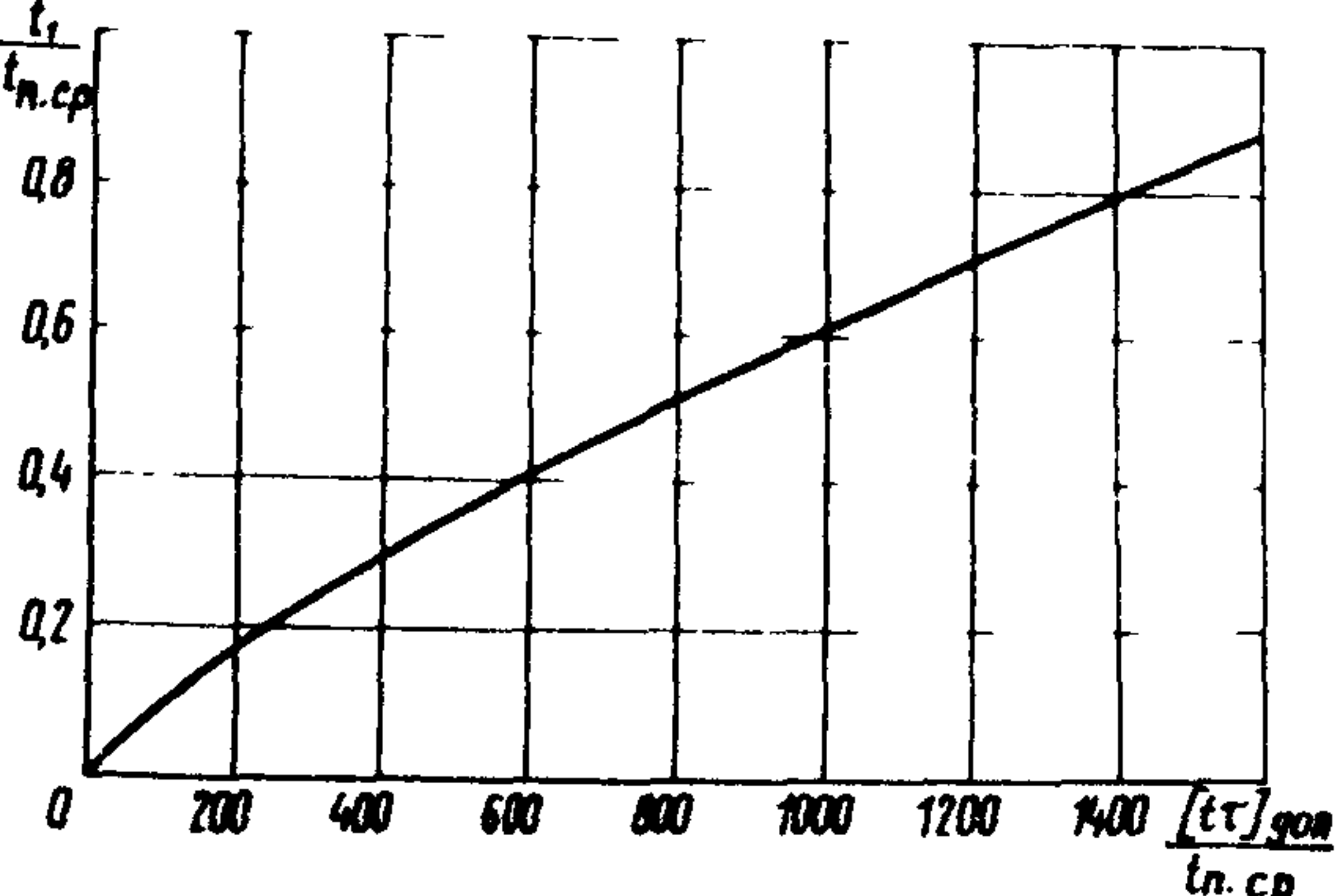
Рис.8. График для определения допускаемой суммы отрицательных температур на поверхности земляного полотна под теплоизоляцией за зиму (градусо-сутки)
