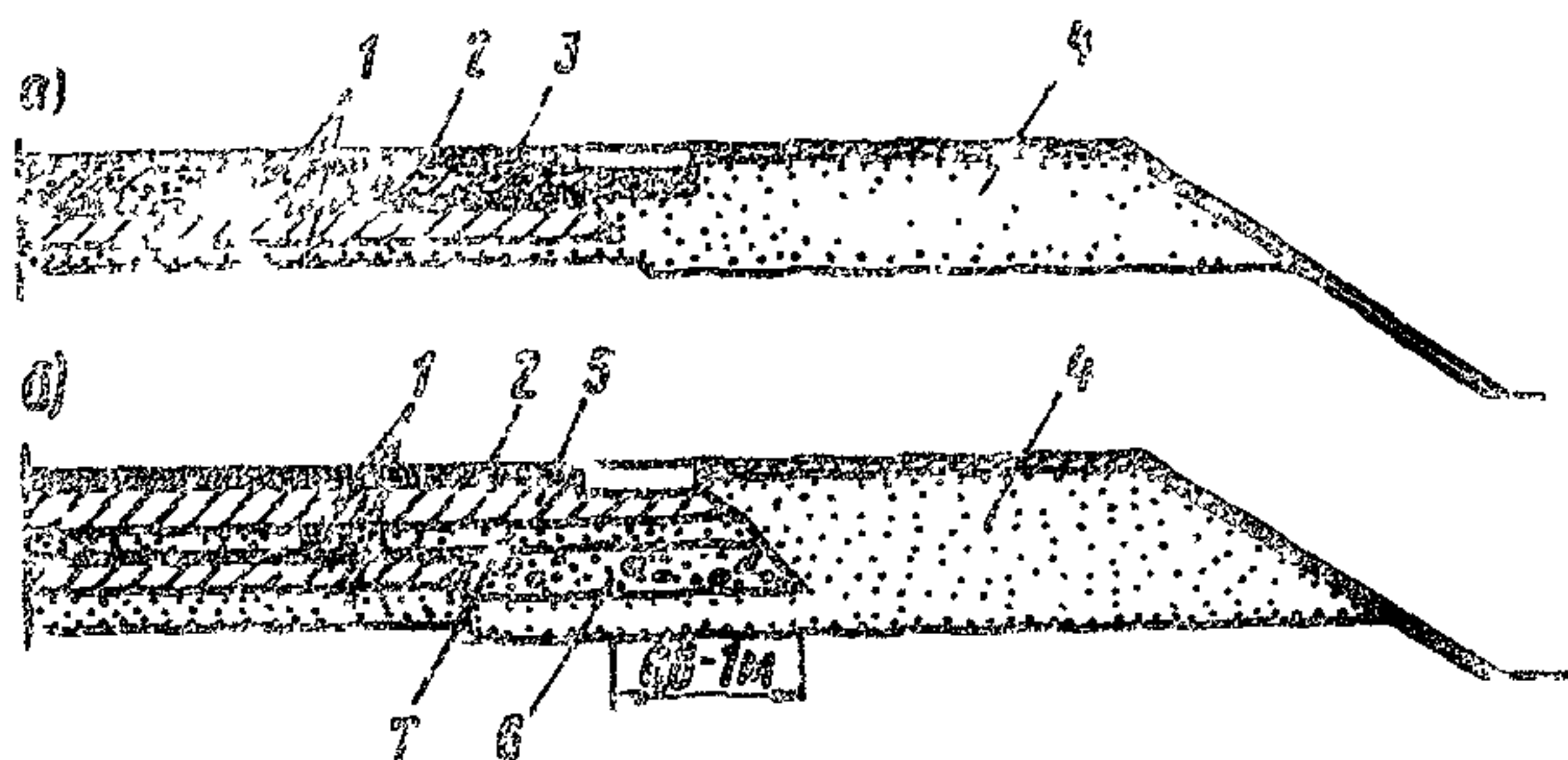
Рис. 6. Теплоизоляция, устраиваемая при усилении дорожной одежды (а) и при реконструкции дорог с уширением и усилением дорожной одежды (б): 1—старая дорожная одежда; 2—новое покрытие; 3—легкий бетон; 4—новый дренажный слой; 5—основание; 6—укрепление основания под уширением; 7—теплоизоляция
