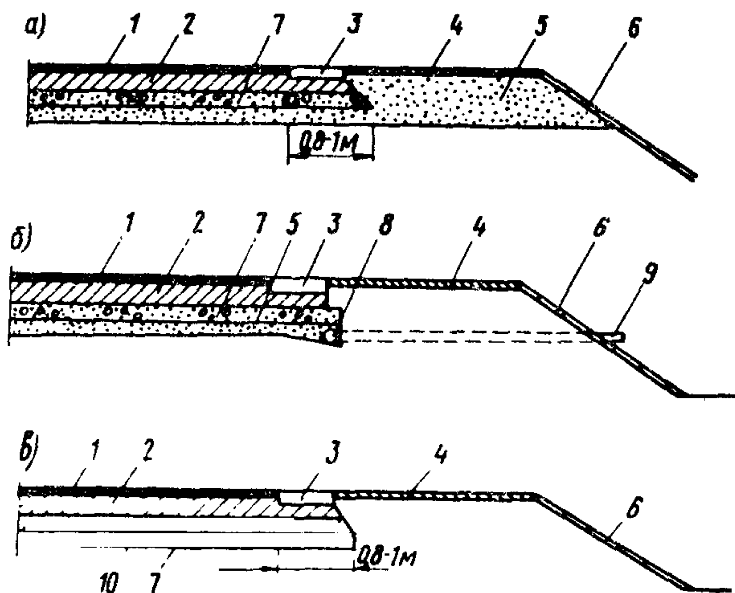
Рис.3. Конструкции с теплоизолирующим слоем из укрепленных материалов и грунтов с легкими заполнителями (а), то же с трубчатыми дренами (б) и с морозозащитным слоем из битумоминеральной смеси (в):
