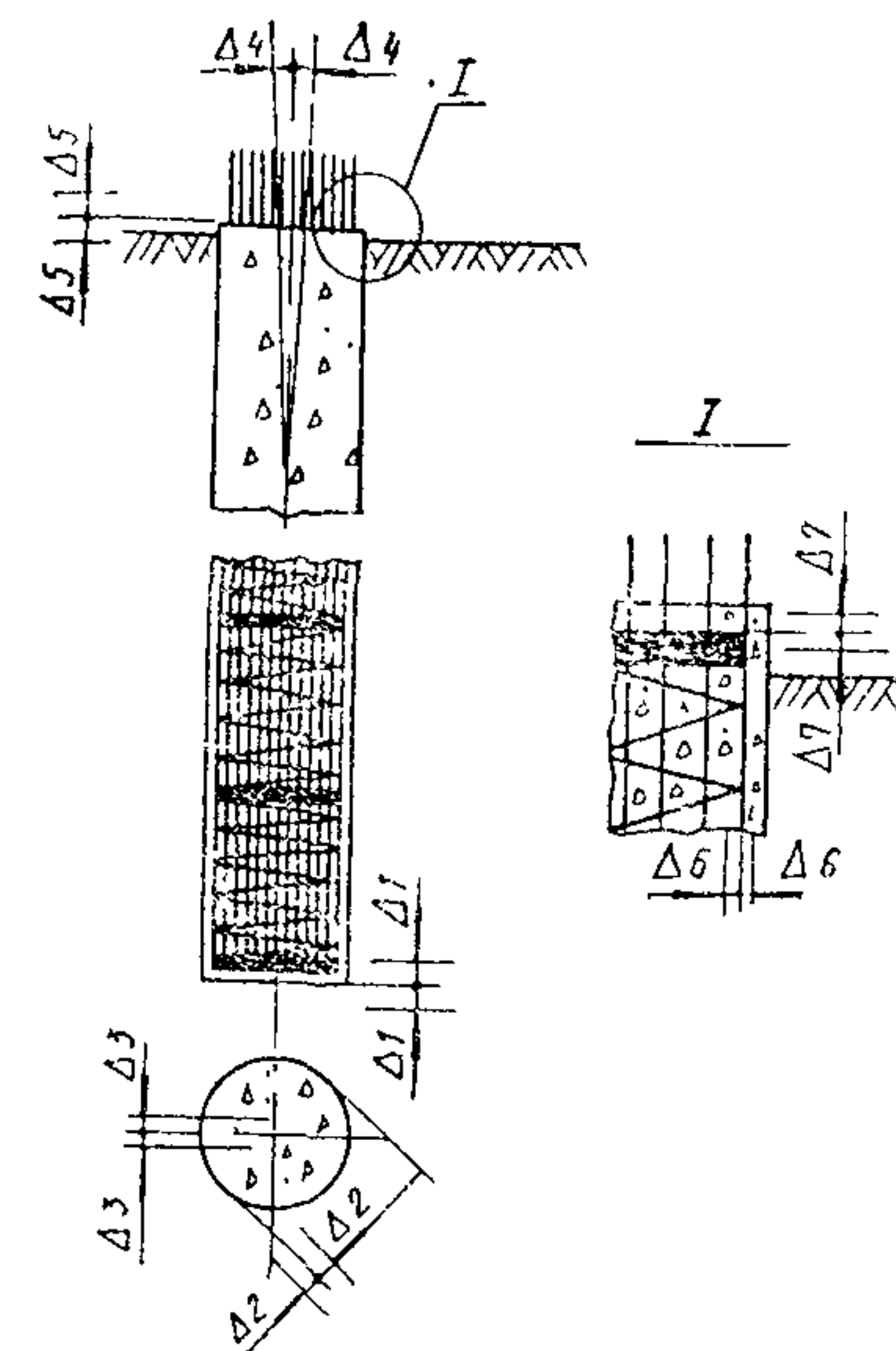
Схема буронабивной свай с указанием предельных отклонений
