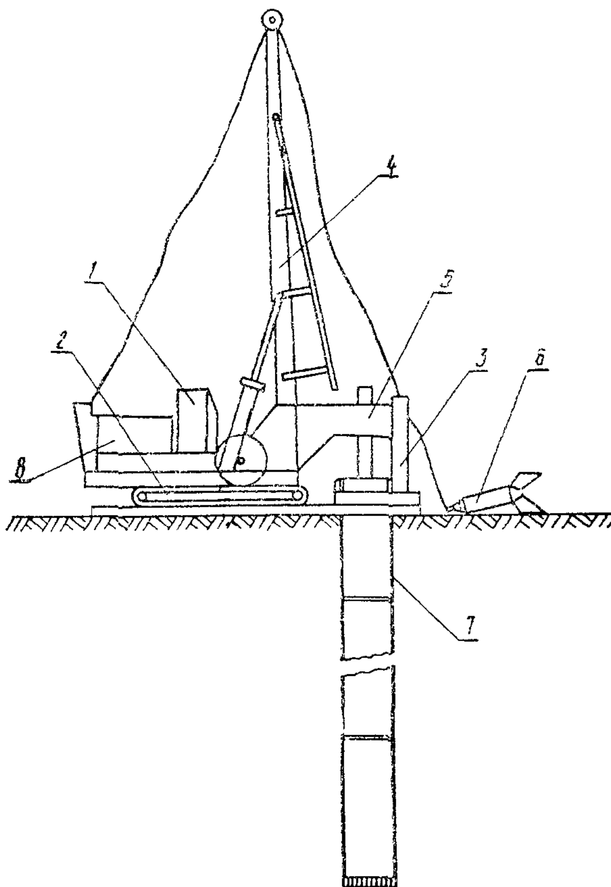
Рис. 1. Схема буровой установки «Като» 30THC-VS:
