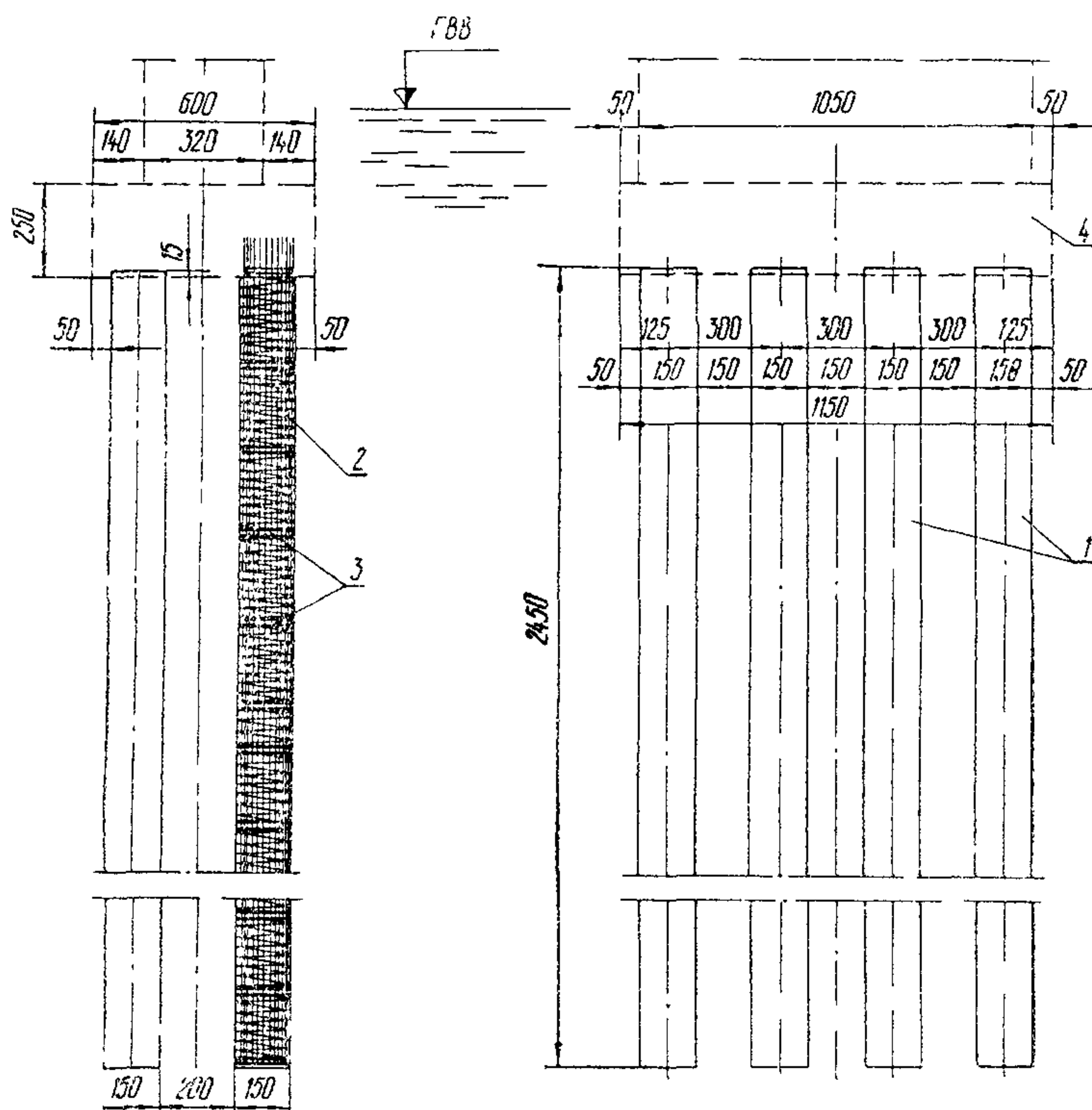
Рис. 2. Конструкция буронабивных свай фундамента опоры моста:
