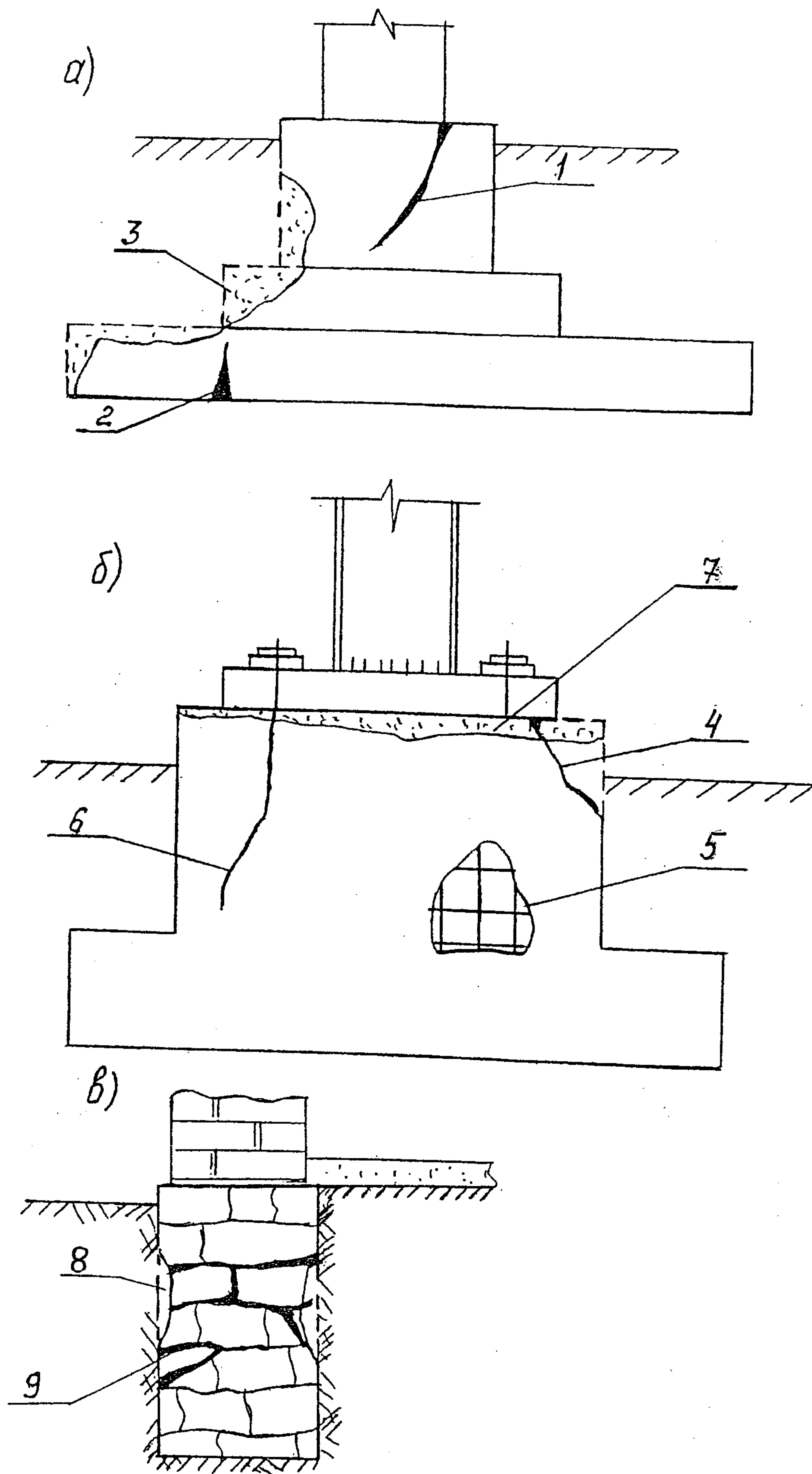
Рис. 13. Повреждения фундаментов
