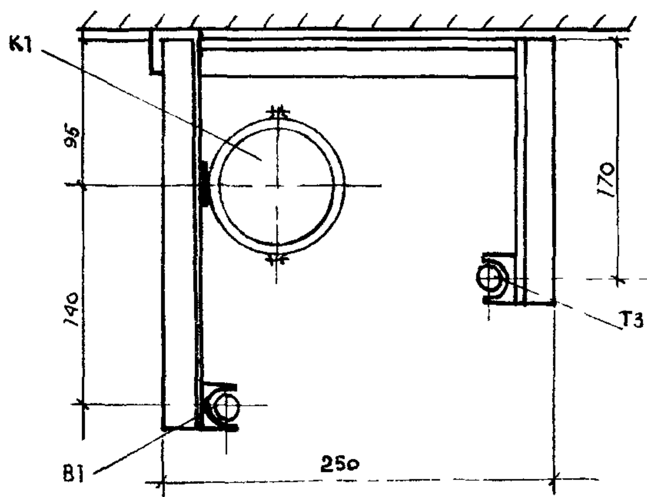
Рис.1. Планы расположения стояков внутреннего водопровода и канализации из полипропиленовых труб в шахт-пакетах
