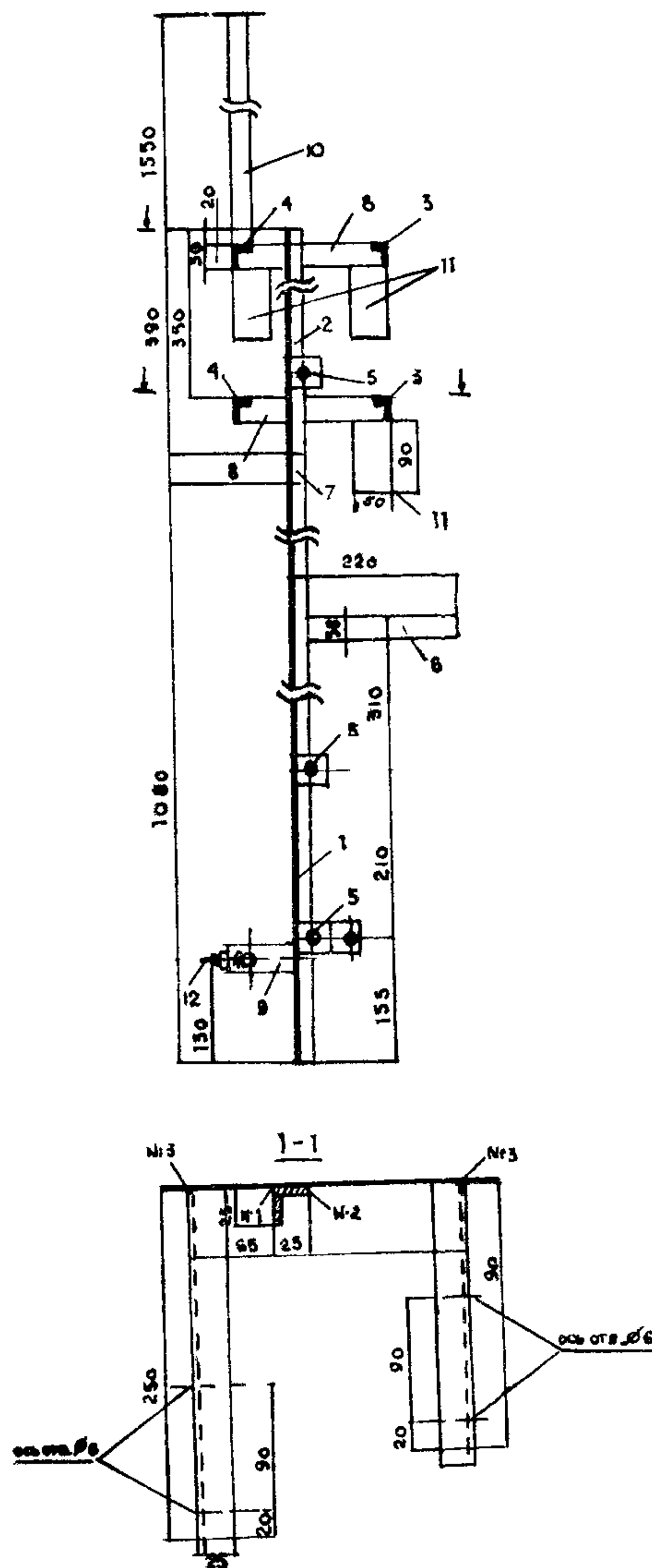
Рис.8. Внешний вид каркаса шахт-пакета для санузла жилого дома серии КОПЭ
