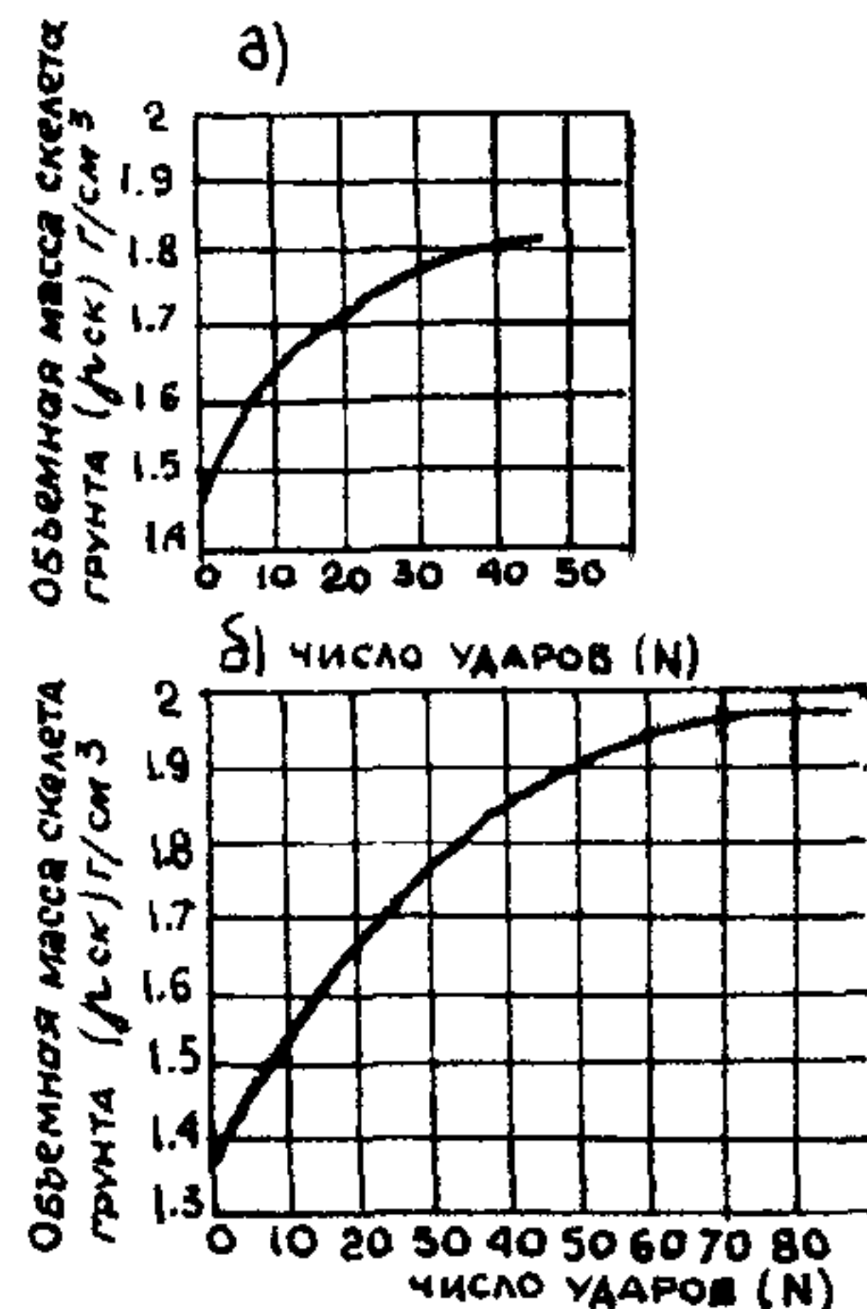
Рис. 2. Тарифовочные графики зависимости числа ударов от степени плотности грунтов в пределах их оптимальной влажности:
