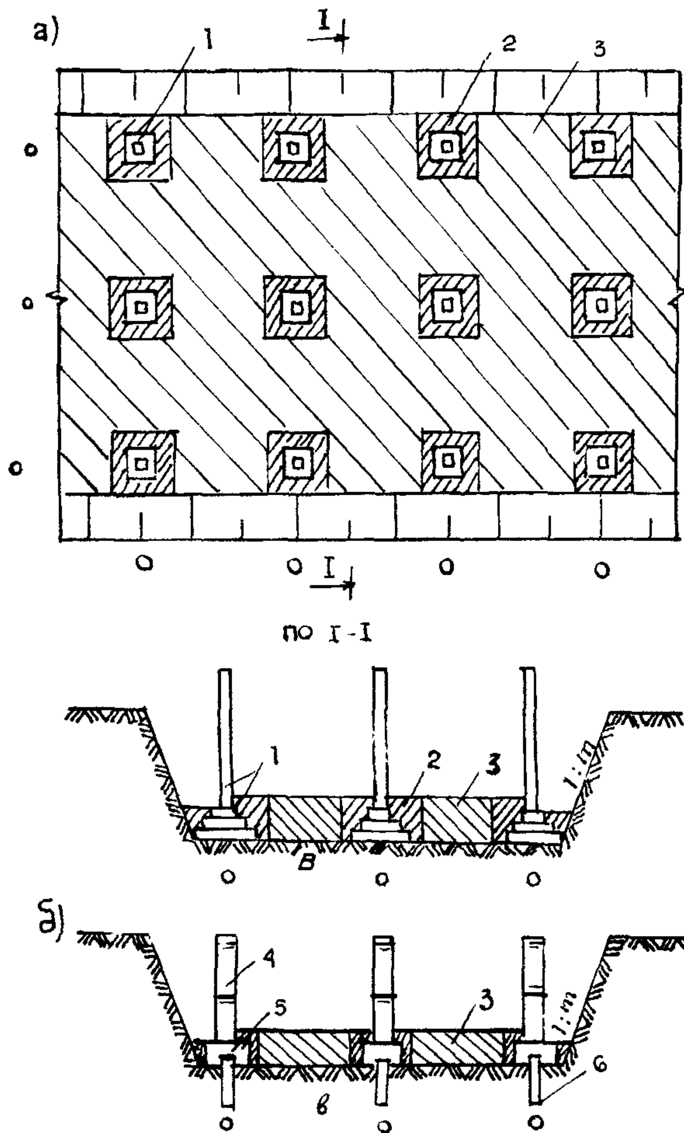
Рис. 7.1. Схема засыпки грунта под полы в подвале здания:
