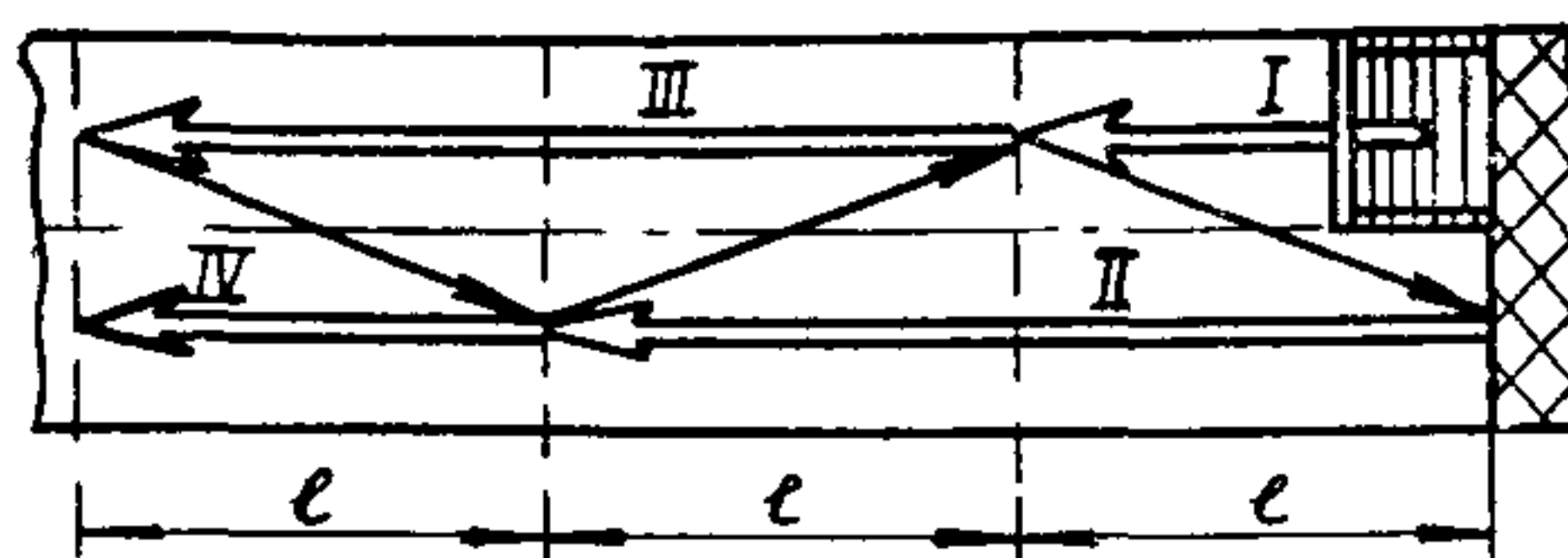
Рис 1 Схема движения асфальтоукладчика
