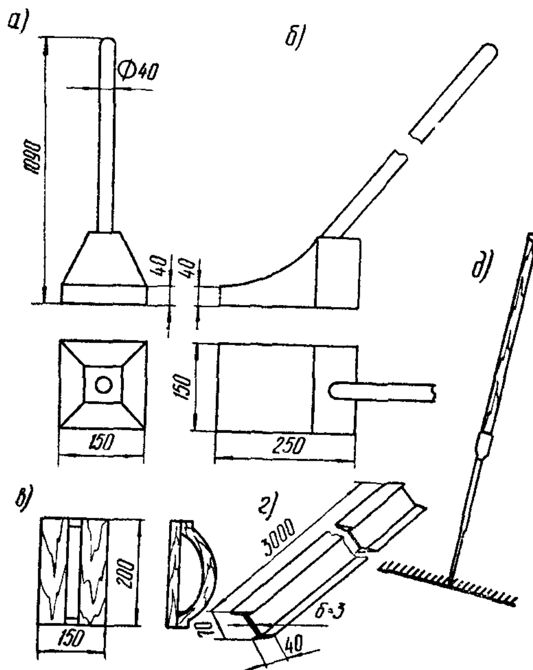
Рис. 2. Инструменты для устройства асфальтобетонных покрытий:
