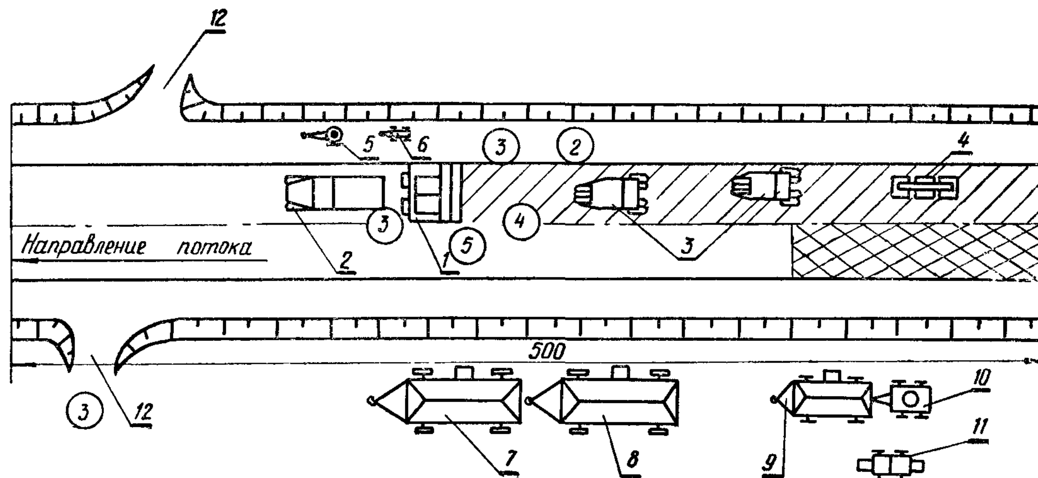
Рис. 3 Технологическая схема устройства асфальтобетонных покрытий на захватке длиной 500 м:
