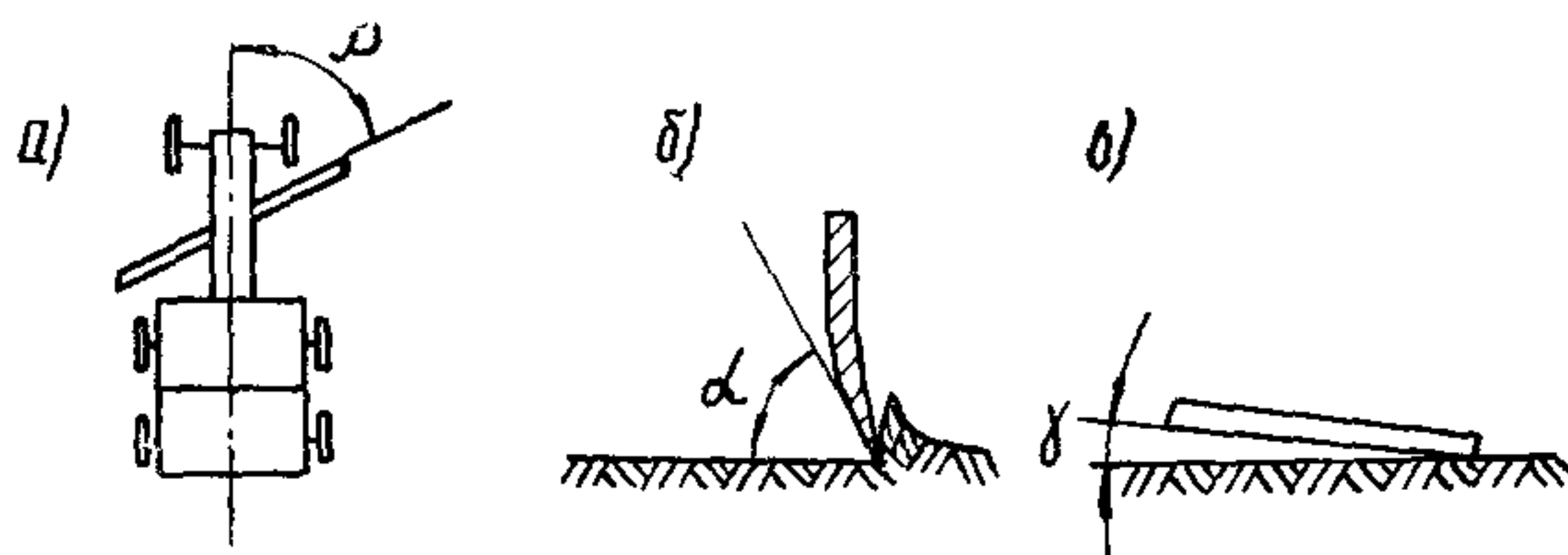
Рис. 3. Углы установки отвала автогрейдера в рабочее положение: а—угол захвата \beta ; б—угол резания \alpha ; в—угол наклона \gamma
