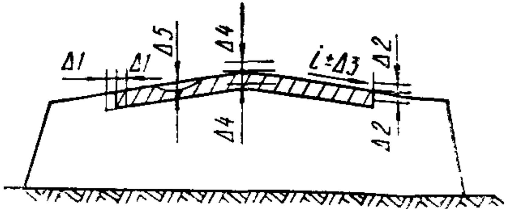
Схема конструкции основания с обозначением предельных отклонений
