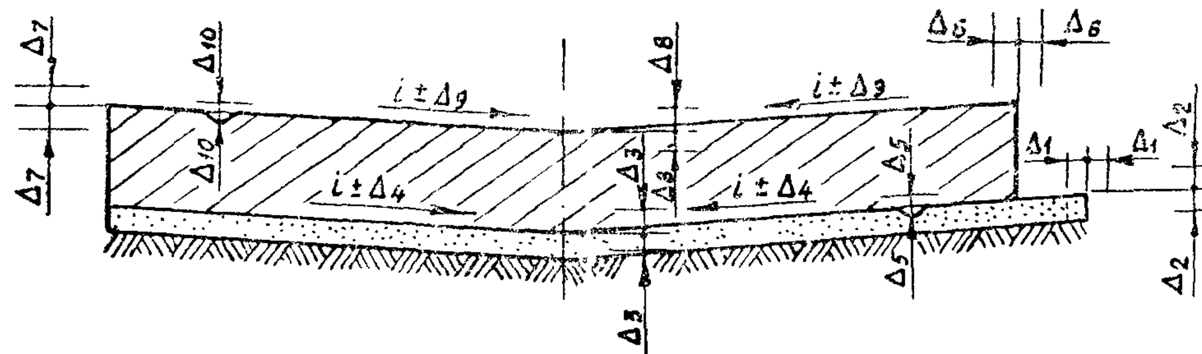
Рис. 6. Схема предельных отклонений
