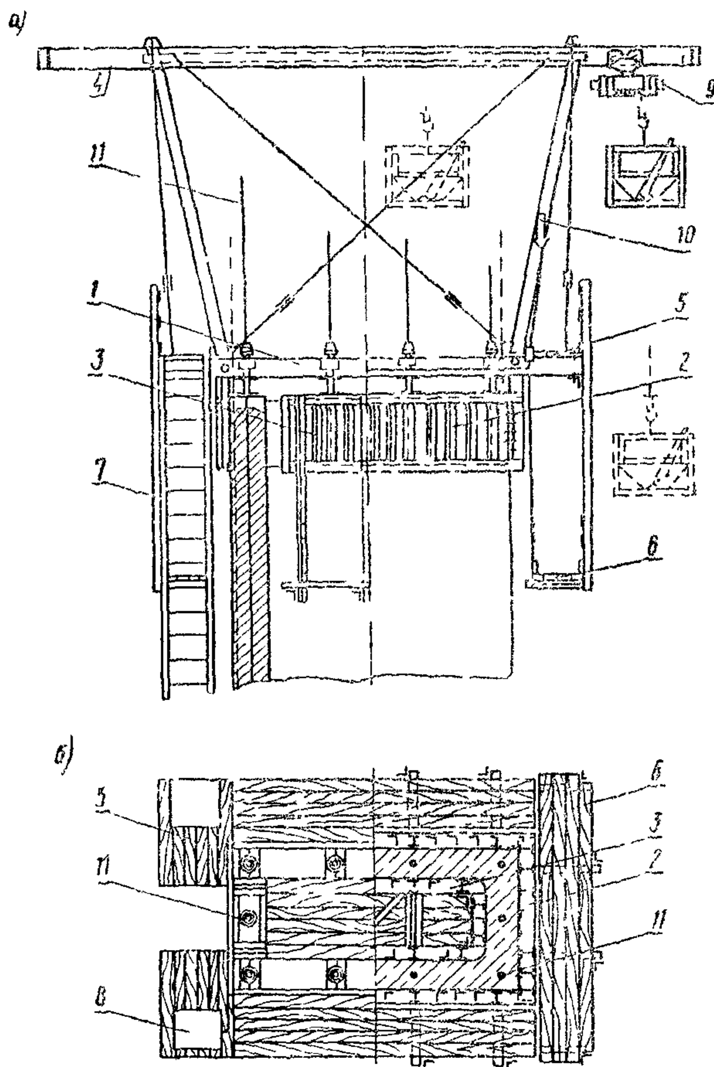
Рис. 2. Агрегат скользящей опалубки:
