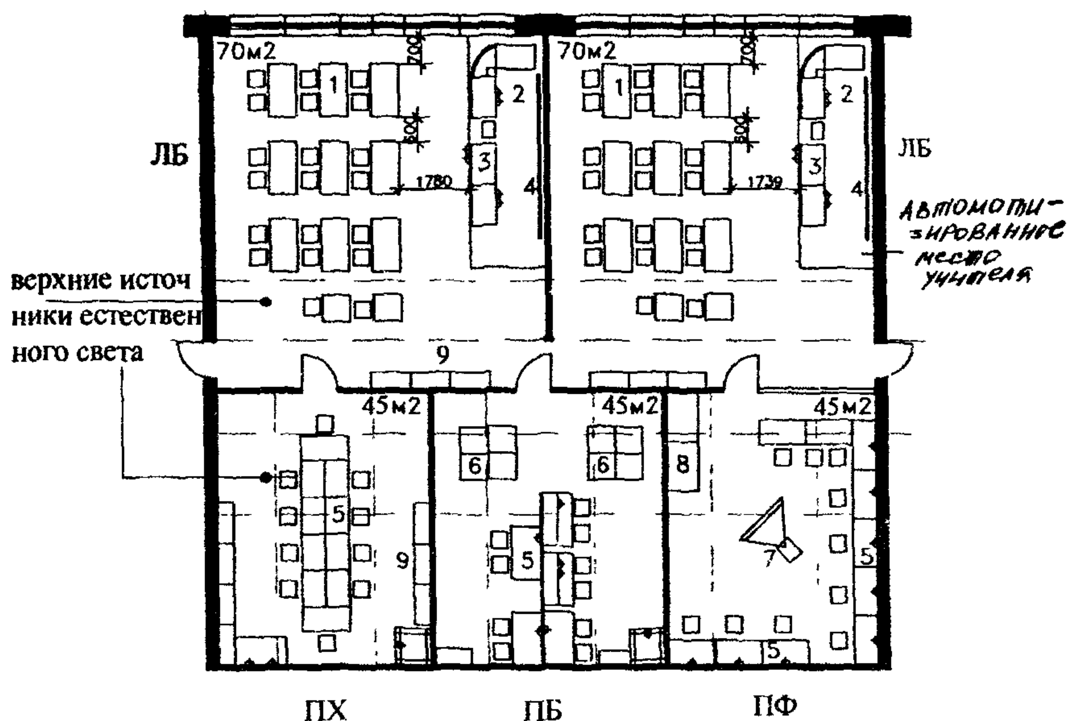
Рис. 8 Учебный специализированный кабинет - лаборатория с практикумами (КТ-III).
