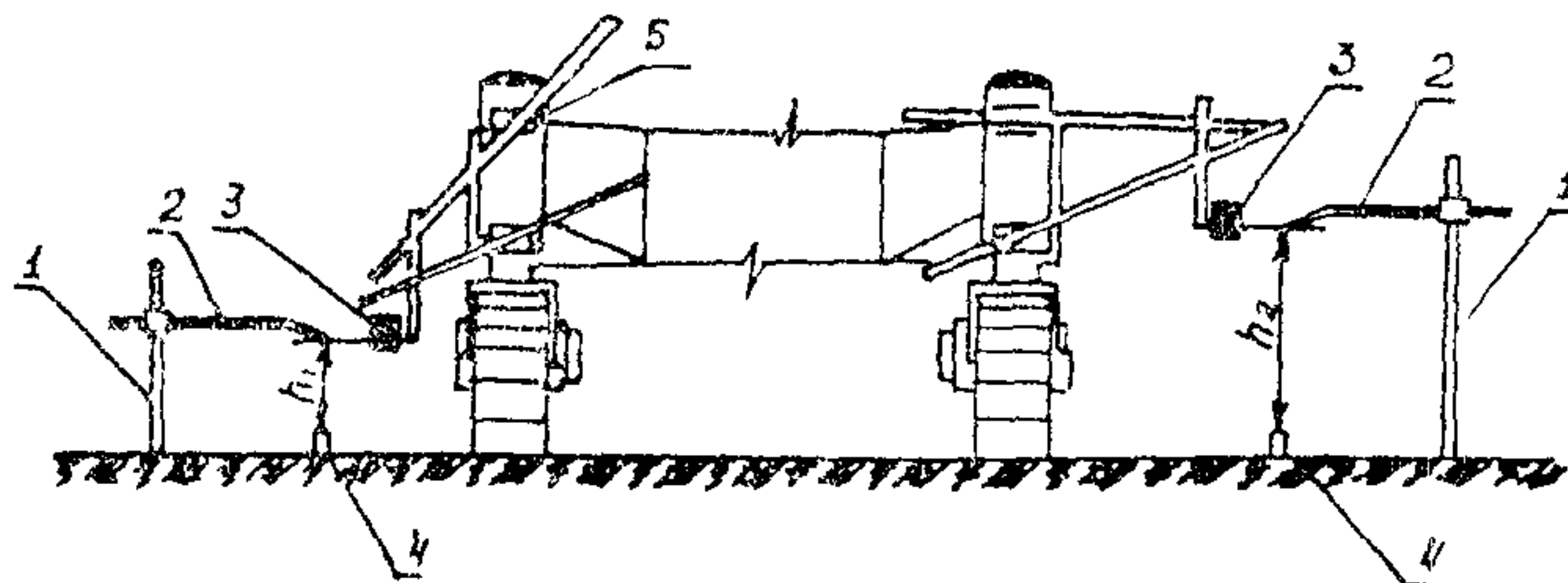
Рис. 5. Установка копирных струн в разных уровнях: 1—металлическая стойка; 2—кронштейн; 3—датчик уровня с копиром; 4—нивелирная рейка; 5—рама профилировщика; h_1 —постоянная высота левой струны; h_2 —постоянная высота правой струны
