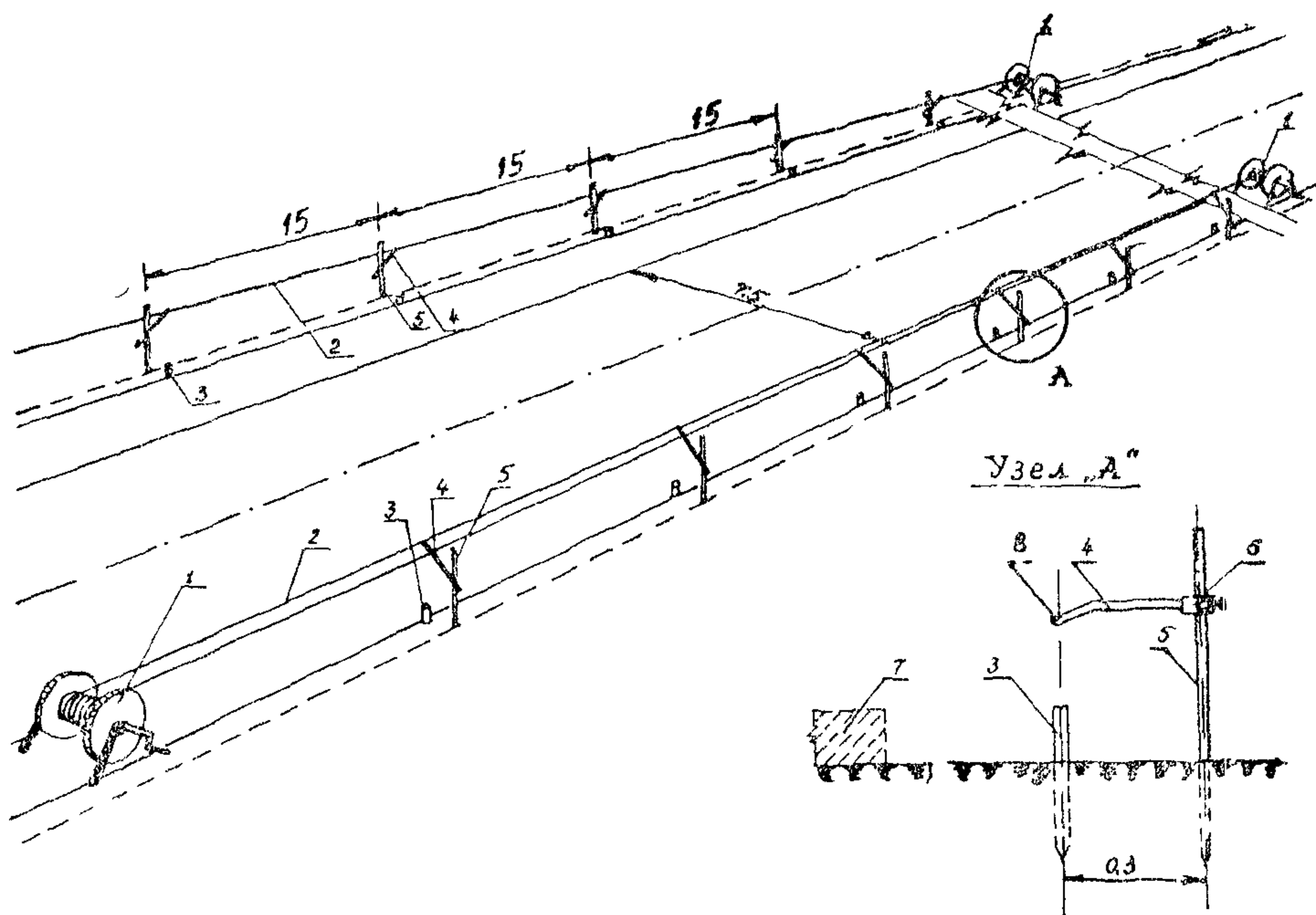
Рис. 1. Схематичный план участка установки копирных струн: 1—натяжной барабан, 2—копирная струна; 3—ливельная рейка; 4—кронштейн, 5—стойка-стержень; 6—струбцина; 7—устанавливаемое покрытие (основание); 8—прорез для струны
