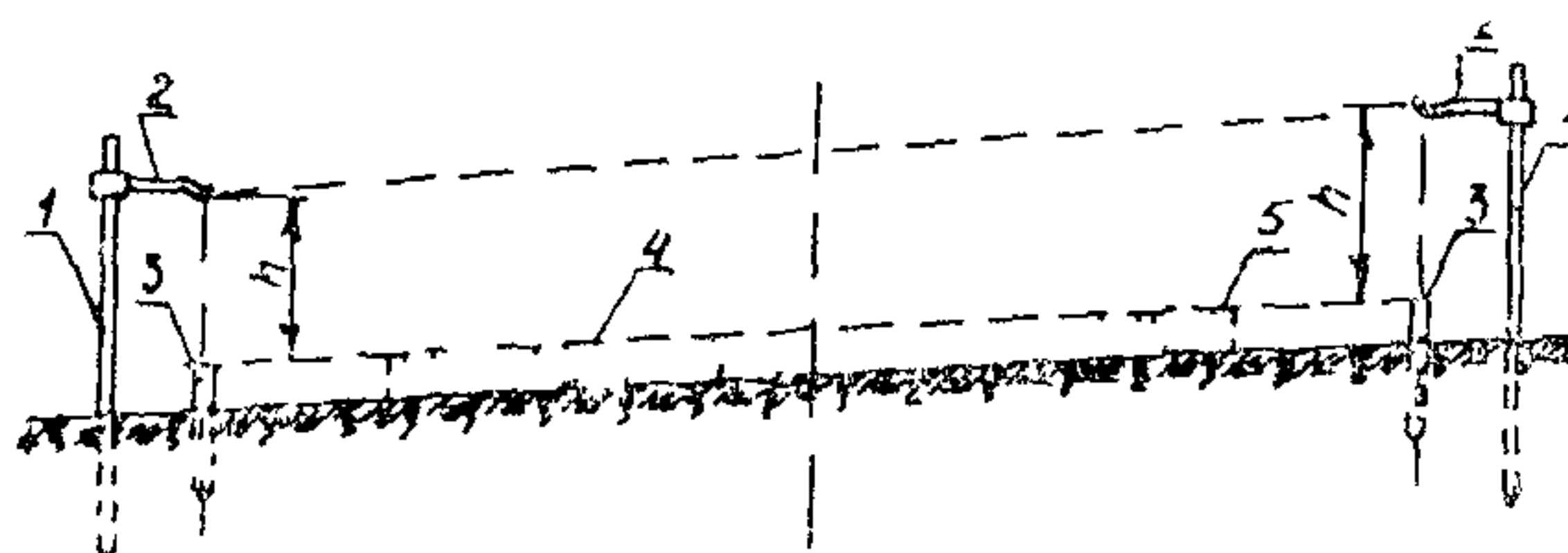
Рис. 2. Расположение струн при односкатном профиле.
